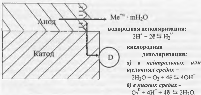
Рис. 11.6. Схема электродных процессов
