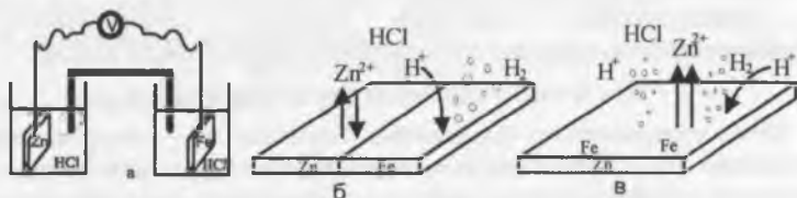
Рис. 11.5. Виды железо - цинковых гальванических элементов а) макрогальванический элемент, б) короткозамкнутый макрогальванический элемент, в) микрогальванический элемент.
