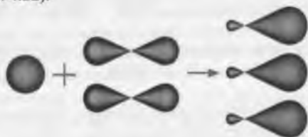
Рис. 4.22. Формы орбиталей при sp^2 -гибридизации
