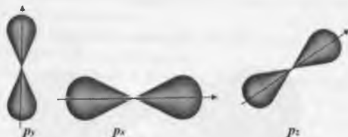
Рис. 4.4. Ориентация в пространстве p_x , p_y и p_z орбиталей
