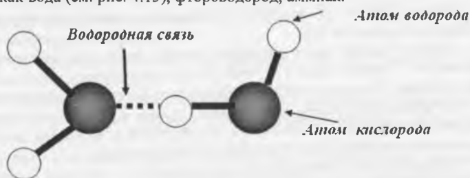
Рис. 4.13. Возникновение водородной связи в молекуле воды
