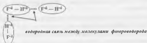
Рис. 4.12. Схема образования водородных связей между молекулами фтороводорода
