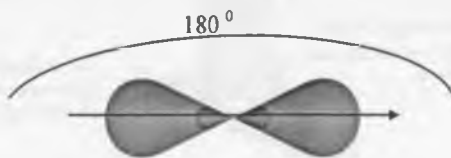
Рис. 4.20. Расположение двух и sp - гибридизованных орбиталей в пространстве
