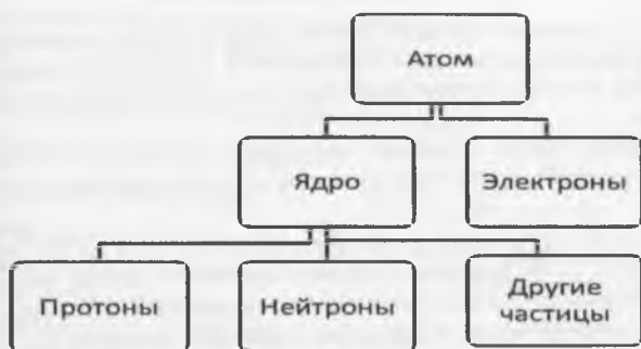
Рис. 4.1. Схема строения атома элемента
