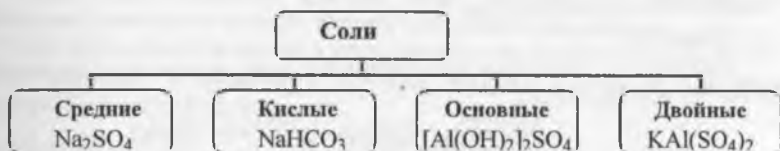
Рис. 2.5. Схема классификации солей
