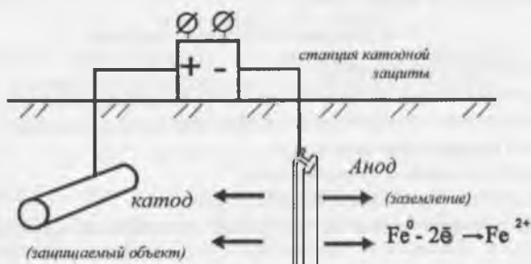
Рис. 11.11. Катодная защита металлов от коррозии
