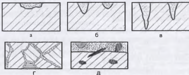
Рис. 11.4. Местная коррозия
