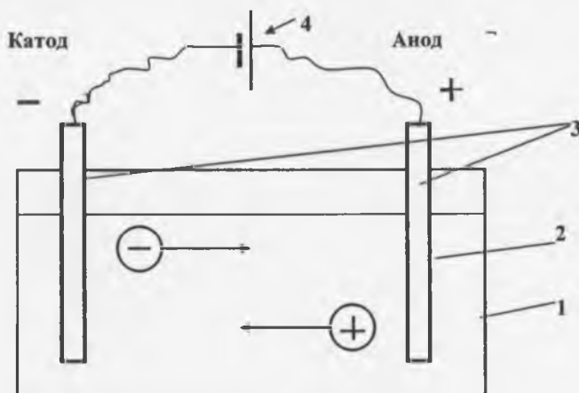
Рис. 12.1. Схема электролизера
