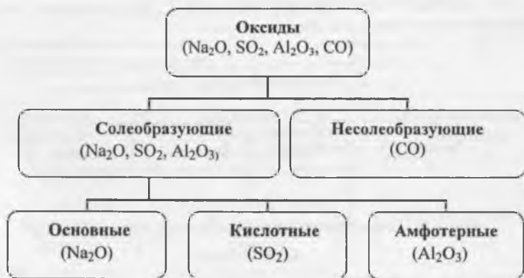
Рис. 2.3. Схема классификации оксидов
