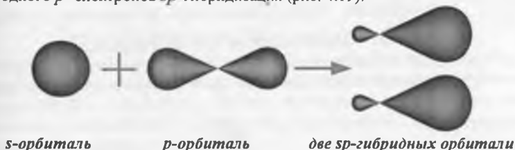
Рис. 4.19. Формы исходных и гибридизованных орбиталей атома бериллия
