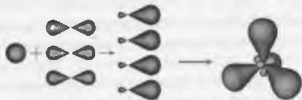
Рис. 4.25. Образование sp^3 -гибридных орбиталей
