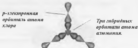
Рис. 4.24. Перекрывание атомных орбиталей в молекуле \text{AlCl}_3 Форма молекулы, имеющей три гибридные sp^2 -орбитали, представляет
