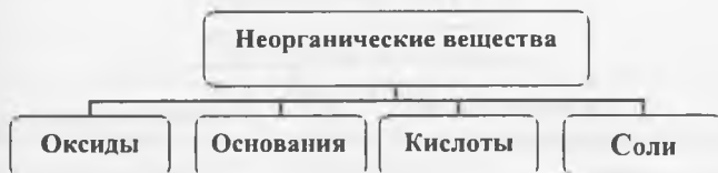
Рис. 2.2. Схема классификации неорганических веществ.
