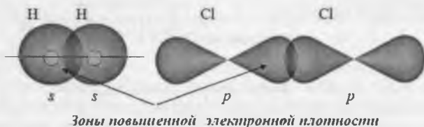
Рис. 4.10. Образование молекул водорода и хлора при перекрытии двух сферических – s и двух гантелеобразных – p атомных орбиталей
