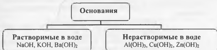
Рис. 2.4. Классификация оснований.
