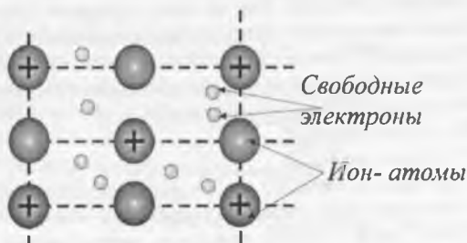
Рис. 4.27. Металлическая связь
