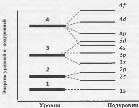
Рис. 4.8. Энергия атомных орбиталей
