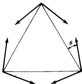
Рис. 4.5. Перекрытие орбиталей в циклопропане. Стрелки направлены к центру электронной плотности.
