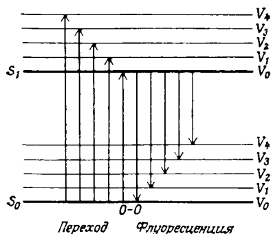
Рис. 7.5. Переход и флуоресценция между состояниями S_1 и S_0 .
