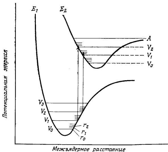
Рис. 7.2. Диаграммы энергии двухатомной молекулы. Показаны два возможных перехода. Если электрон возбужден до уровня А, молекула может распадаться (разд. 7.5).
