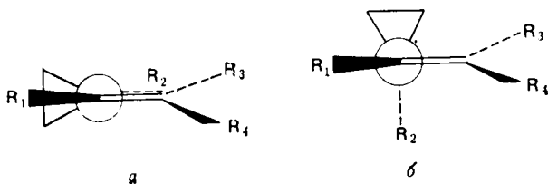
Рис. 4.6. Конформации \alpha -циклопропилалкенов. В конформации a сопряжение максимально, в конформации б — минимально.
