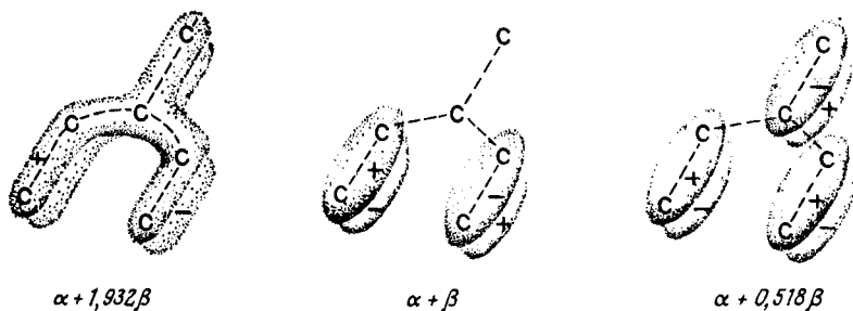
Рис. 2.5. Три связывающие орбитали 3-метилена-1,4-пентадиена (9).
