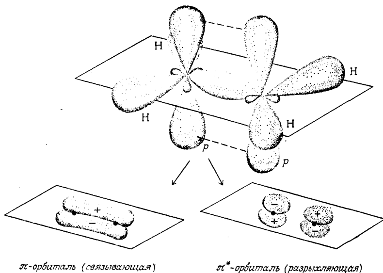
Рис. 1.5. Перекрывающиеся p -орбитали образуют \pi - и \pi^* -орбитали. Для удобства \sigma -орбитали показаны отдельно в верхней части рисунка.
