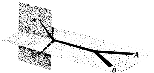
Рис. 4.2. Взаимно перпендикулярные несимметричные плоскости.
