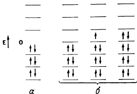
Рис. 2.6. Энергетические уровни четно альтернантных (а) и нечетно альтернантных (б) углеводородов [94].
