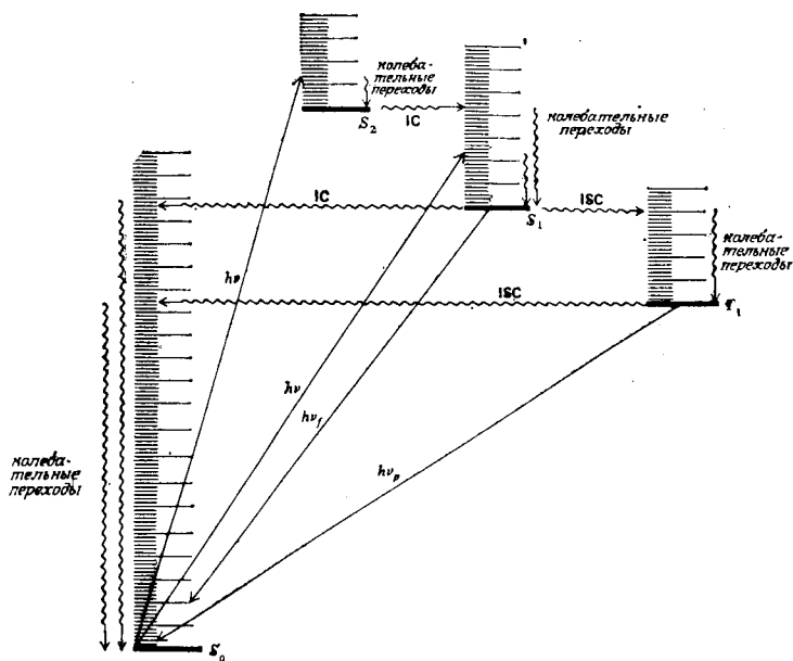
Рис. 7.4. Модифицированная диаграмма Яблонского, показывающая переходы из основного состояния в возбужденные.
