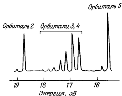
Рис. 1.8. Фотоэлектронный спектр молекулы азота ( N_2 ) [12].
