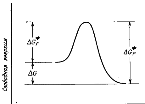
Рис. 6.1. Диаграмма свободной энергии для реакции, в ходе которой интермедиат не образуется. Продукты обладают меньшей свободной энергией, чем реагенты.
