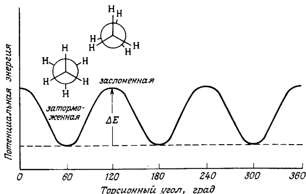
Рис. 4.3. Диаграмма потенциальной энергии конформаций этана.
