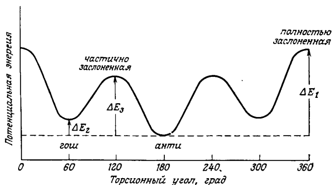
Рис. 4.4. Диаграмма потенциальной энергии конформаций систем \text{YCH}_2\text{—CH}_2\text{Y} или \text{YCH}_2\text{—CH}_2\text{X} .
