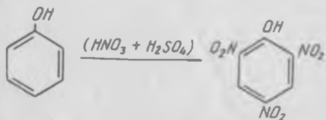
2,4,6-тринитрофенол-пикрин кислота
