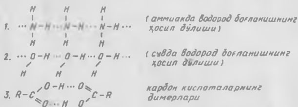
6-расм. Аммиак, сув ва карбон кислоталарда водород боғланишнинг ҳосил бўлиши.
