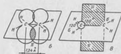
9-расм. Этилен молекуласининг ҳосил бўлиши.
