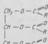
триглицерид
