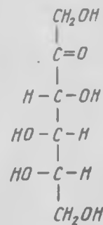
\beta -L-фруктоза
