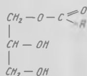
моноглицерид
