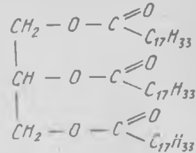
триолеин
