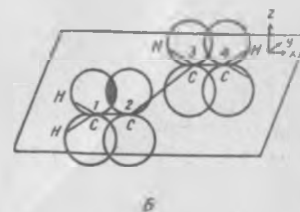
10-расм. Пропилен ва бутаден молекуласининг электрон тузилиши
