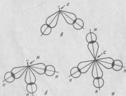
4-расм. Метан (а), аммиак (б) ва сув (в) молекулаларида туртала электрон жуфтининг фазода узаро жойлашиши (Р — электрон булутларининг ярмиси, яъни гантелининг бир томони) курсатилган.
