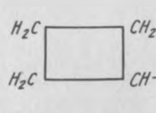
циклобутил
