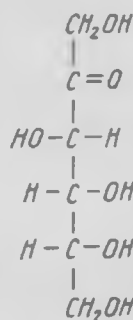
\alpha -D-фруктоза
