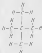
неопентан
