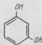
резорцин m-диоксибензол
