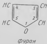
ФУРАН ГРУППАСИ
