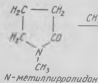
N-метилпирролидон
