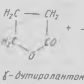
\delta -бутиролактон
