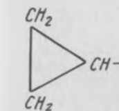
циклопропил
