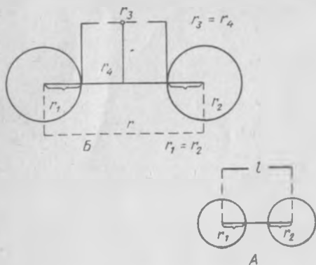
2-рasm. Атом ковалент радиусининг бог узунлигининг ярмига тенглиги.
