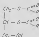
диглицерид
