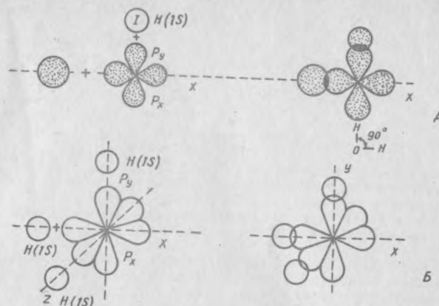
7-расм. Сув (А) ва аммиак (В) молекулларнинг ҳосил бўлиши.
