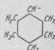
циклогексил
