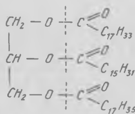
олеин кислота қолдиғи
