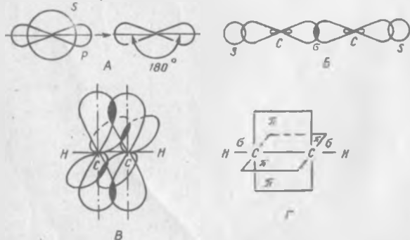
11-расм. sp — гибридланиш ва ацетилен молекуласининг электрон тўзлиши.
