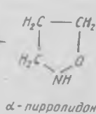
\alpha -пирролидон
