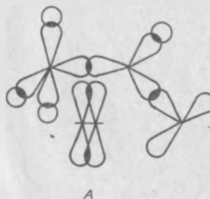
10-расм. Пропилен ва бутаден молекуласининг электрон тузилиши
