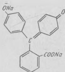
қизил фенолфталеин
