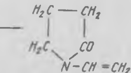
N-винил- \alpha -пирролидон
