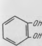
пирокатехин o-диоксибензол
