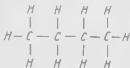
н-бутан
