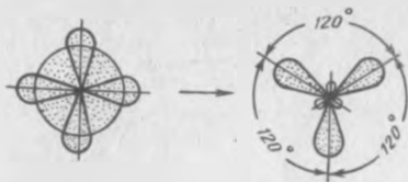
8-расм. sp^2 — гибрид орбиталларнинг ҳосил бўлиши.
