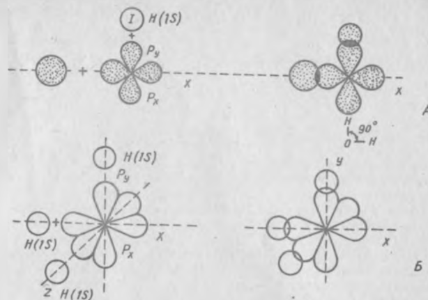
7-расм. Сув (А) ва аммиак (В) молекуляр орбиталларининг ҳосил бўлиши.
