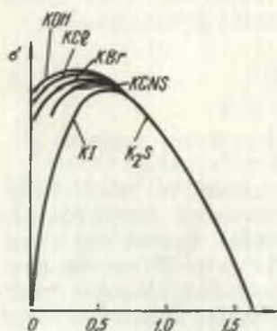
33-расм. Анионлар адсорбиланган шароитда электрокапилляр диаграмма максимумларининг ўзгариши.
