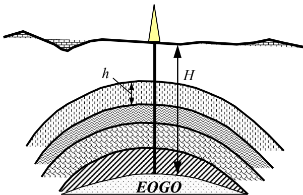
6-rasm. Yer osti gaz ombori qirqimi
