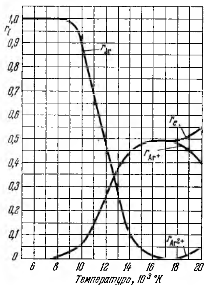
Рис. 24. Изменение объемных долей r_i ионизованного аргона в зависимости от температуры при p = 10^{-1} \text{ кг/см}^2 .
