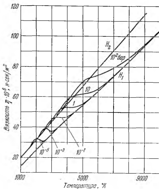
Рис. 4. Вязкость \eta диссоциированного водорода ( H_1 — атомарный и H_2 — молекулярный водород).
