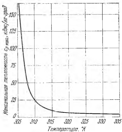
Рис. 11. Изменение максимальной теплоемкости c_{p\max} двуокиси углерода в зависимости от температуры на различных изобарах.
