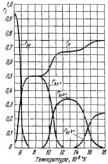
Рис. 32. Изменение объемных долей r_i ионизованного аргона в зависимости от температуры при p = 10^{-9} \text{ кг/см}^2 .
