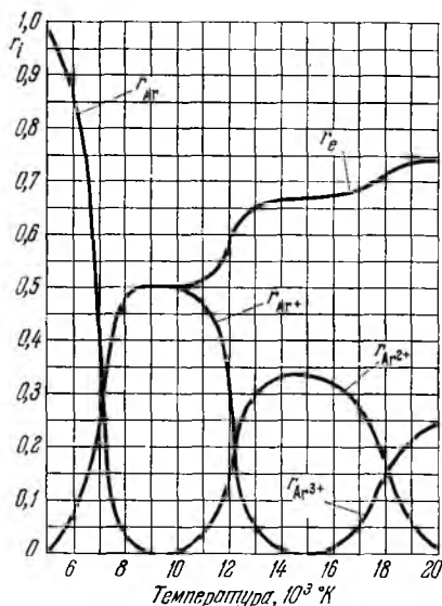
Рис. 30. Изменение объемных долей r_i ионизованного аргона в зависимости от температуры при p = 10^{-7} \text{ кг/см}^2 .
