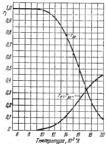
Рис. 22. Изменение объемных долей r_i ионизованного аргона в зависимости от температуры при p = 10 \text{ кг/см}^2 .
