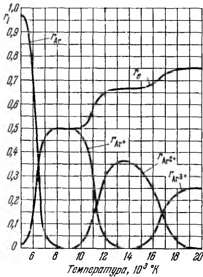
Рис. 31. Изменение объемных долей r_i ионизованного аргона в зависимости от температуры при p = 10^{-8} \text{ кг/см}^2 .
