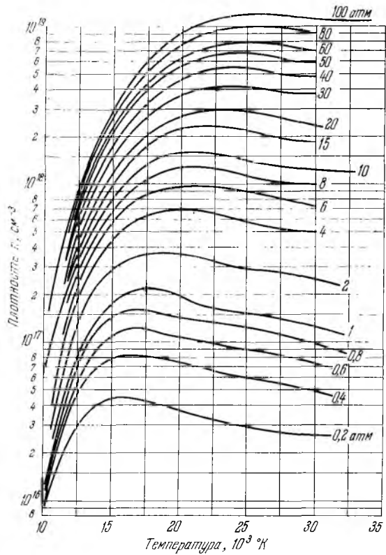
Рис. 16. Изменение плотности n электронов (ионов) в ионизованном азоте в зависимости от температуры на различных изобарах.
