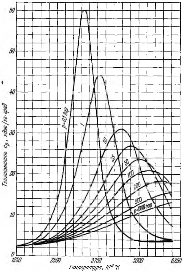
Рис. 6. Изменение теплоемкости c_p диссоциированного водяного пара в зависимости от температуры на различных изобарах.
