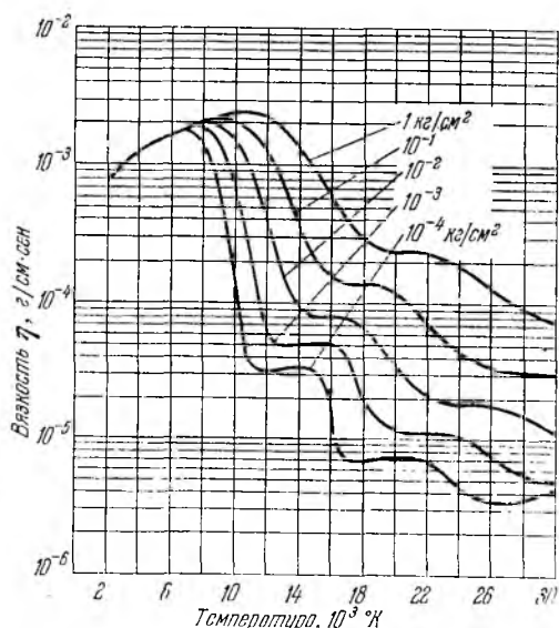
Рис. 38. Изменение вязкости \eta ионизованного аргона в зависимости от температуры на различных изобарах.
