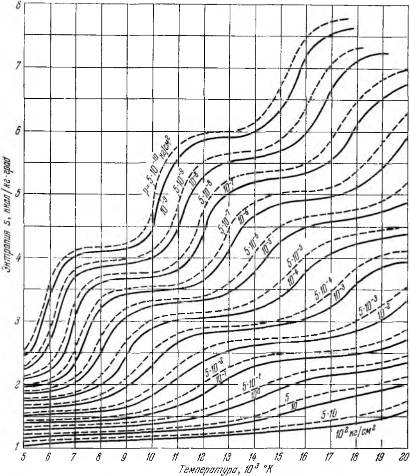
Рис. 36. Изменение энтропии s ионизованного аргона в зависимости от температуры на различных изобарах.
