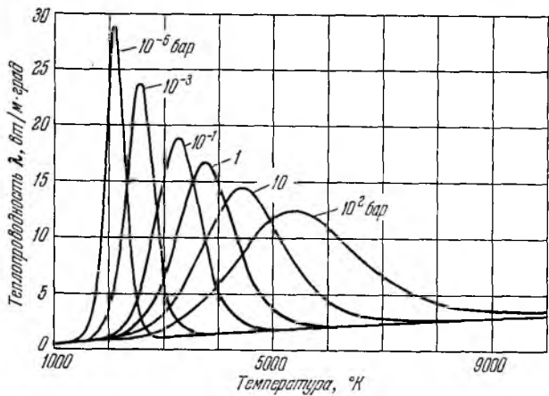
Рис. 5. Изменение теплопроводности \lambda диссоциированного водорода в зависимости от температуры на различных изобарах.
