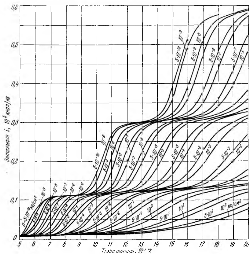
Рис. 35. Изменение энтальпии i ионизованного аргона в зависимости от температуры на различных изобарах.
