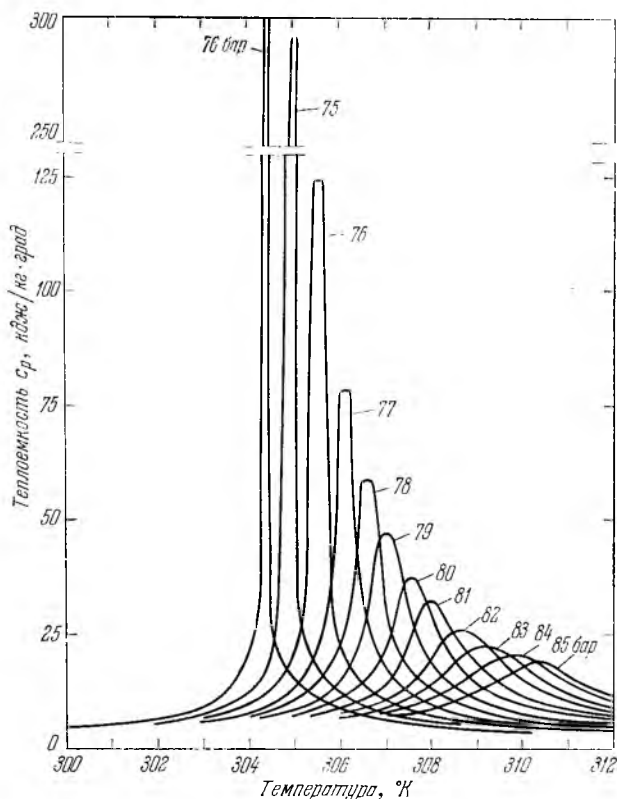
Рис. 10. Теплоемкость c_p двуокиси углерода вблизи критического состояния ( p_{кр}=73,815 бар; T_{кр}=304,19 °K). Температуры, при которых теплоемкость c_p двуокиси углерода достигает максимальной величины на различных изобарах:
