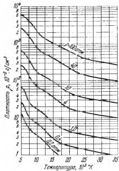
Рис. 15. Изменение плотности \rho ионизованного азота в зависимости от температуры на различных изобарах.
