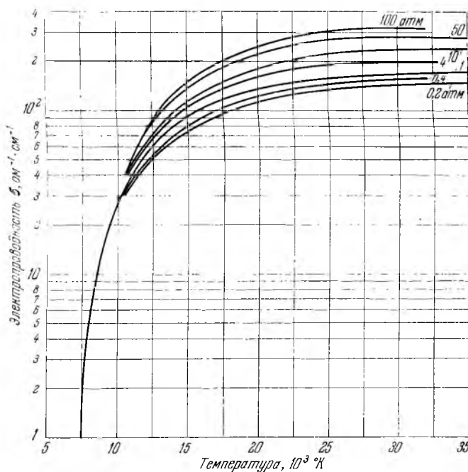
Рис. 17. Изменение электропроводности \sigma ионизованного азота в зависимости от температуры.
