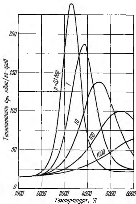
Рис. 3. Изменение теплоемкости c_p диссоциированного водорода в зависимости от температуры и различных изобар.
