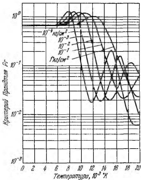
Рис. 40. Изменение критерия Прандтля Pr ионизованного аргона в зависимости от температуры на различных изобарах.
