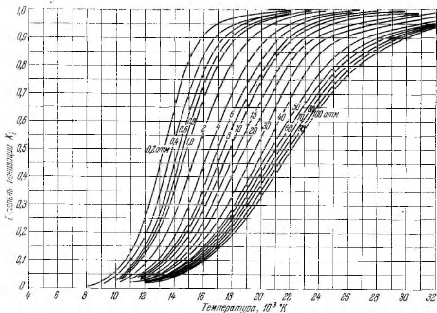
Рис. 14. Изменение степени ионизации X_i азота в зависимости от температуры на различных изобарах.
