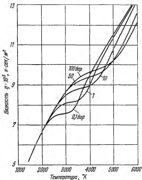
Рис. 7. Изменение вязкости \eta диссоциированного водяного пара в зависимости от температуры на различных изобарах.
