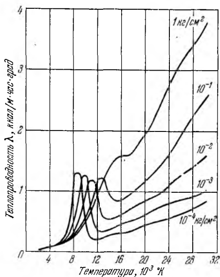
Рис. 39. Изменение теплопроводности \lambda ионизованного аргона в зависимости от температуры на различных изобарах.
