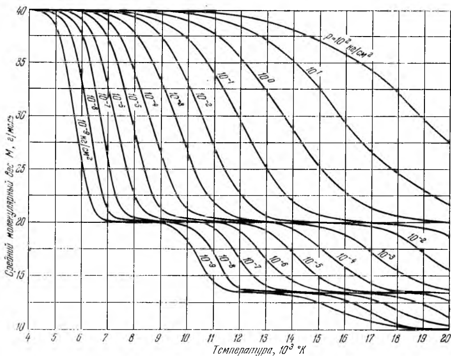
Рис. 33. Изменение среднего молекулярного веса M ионизованного аргона в зависимости от температуры на различных изобарах.
