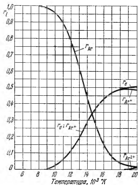
Рис. 23. Изменение объемных долей r_i ионизованного аргона в зависимости от температуры при p = 1 \text{ кг/см}^2
