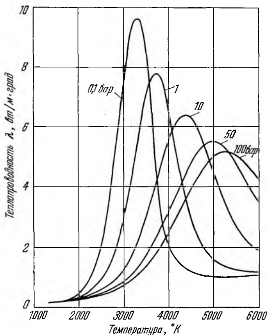
Рис. 8. Изменение теплопроводности \lambda диссоциированного водяного пара в зависимости от температуры на различных изобарах.
