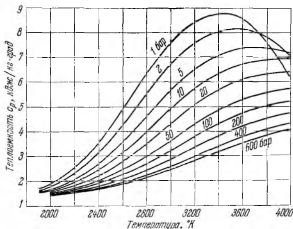
Рис. 12. Изменение теплоемкости c_p диссоциированной двуокиси углерода в зависимости от температуры на различных изобарах.
