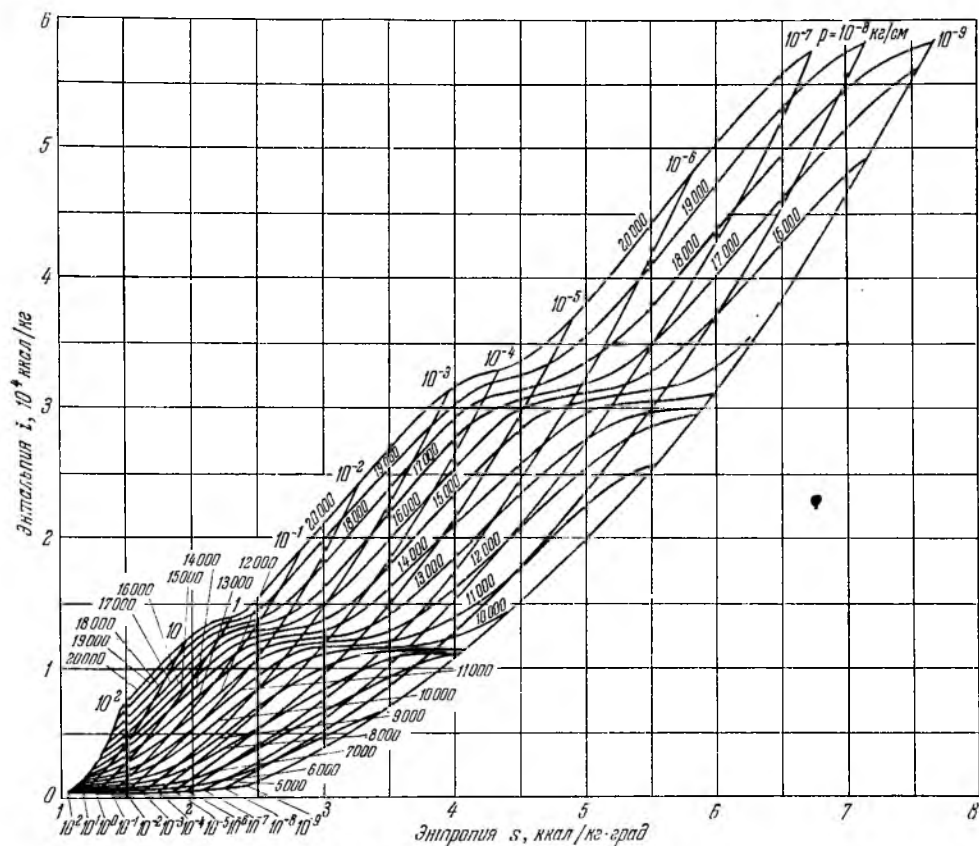
Рис. 37. Диаграмма i-s для аргона.
