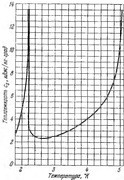
Рис. 18. Изменение теплоемкости c_p жидкого гелия на линии насыщения в зависимости от температуры.
