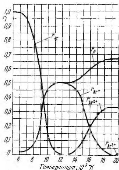
Рис. 27. Изменение объемных долей r_i ионизованного аргона в зависимости от температуры при p = 10^{-4} \text{ кг/см}^2 .
