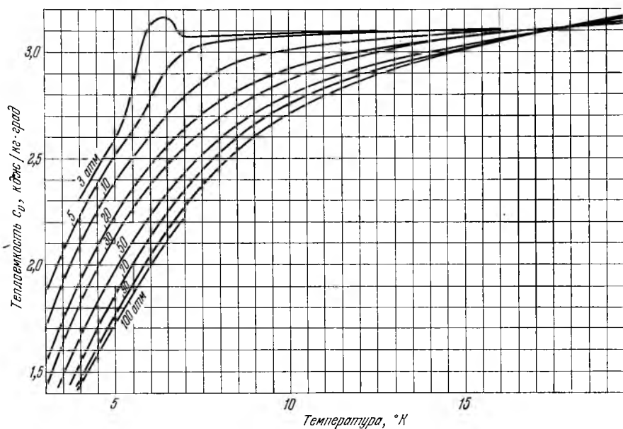
Рис. 19. Изменение теплоемкости c_p гелия в зависимости от температуры на различных изобарах.
