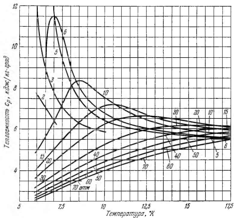
Рис. 20. Изменение теплоемкости c_p гелия в зависимости от температуры на различных изобарах.
