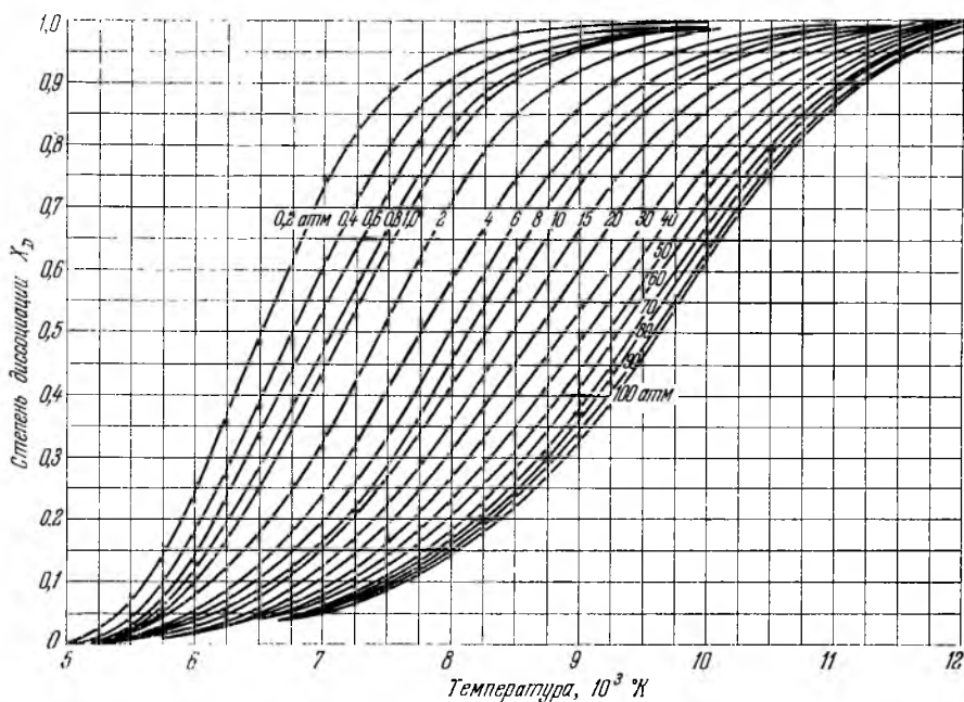
Рис. 13. Изменение степени диссоциации X_2 азота в зависимости от температуры на различных изобарах.
