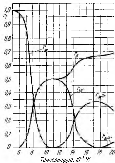
Рис. 28. Изменение объемных долей r_i ионизованного аргона в зависимости от температуры при p = 10^{-5} \text{ кг/см}^2 .
