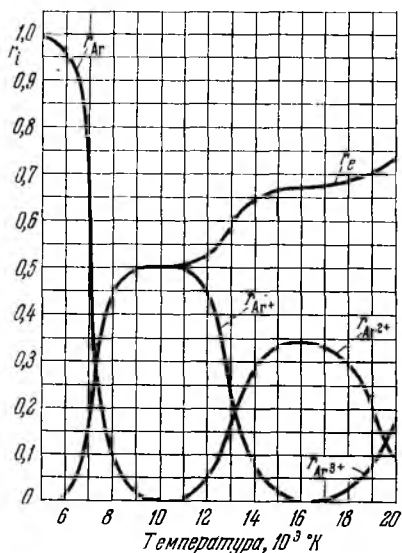
Рис. 29. Изменение объемных долей r_i ионизованного аргона в зависимости от температуры при p = 10^{-6} \text{ кг/см}^2 .
