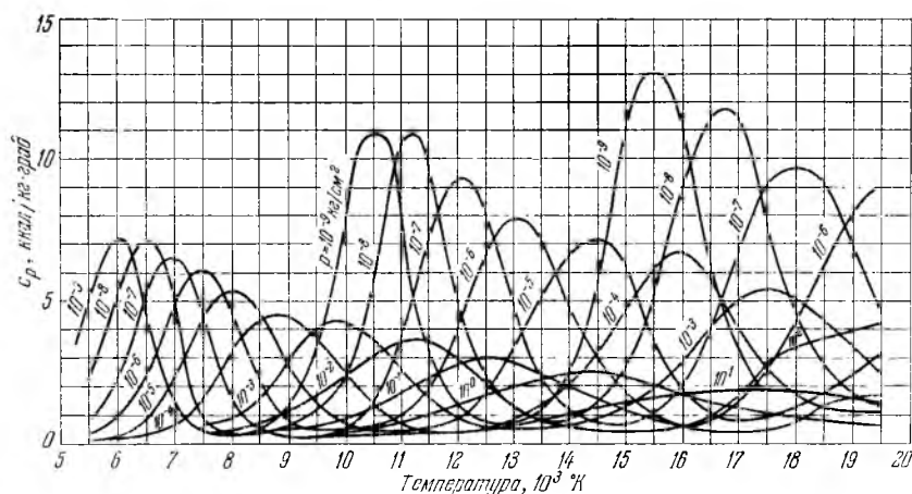
Рис. 34. Изменение теплоемкости c_p ионизованного аргона в зависимости от температуры на различных изобарах.
