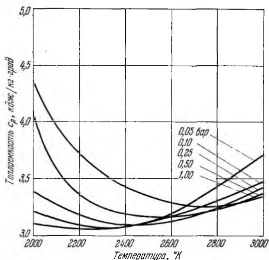
Рис. 9. Теплоемкость c_p диссоциированного и частично ионизованного лития.
