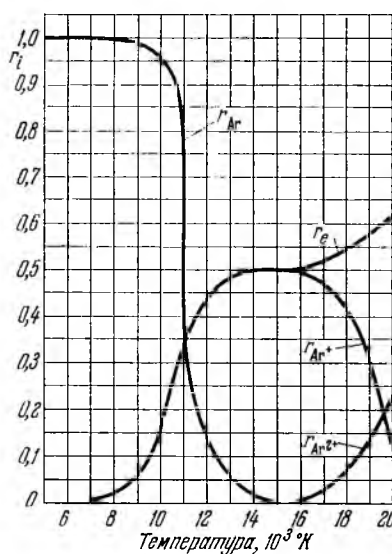
Рис. 25. Изменение объемных долей r_i ионизованного аргона в зависимости от температуры при p = 10^{-2} \text{ кг/см}^2 .
