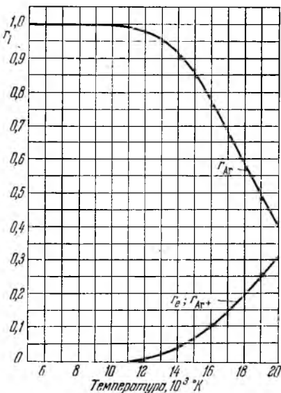
Рис. 21. Изменение объемных долей r_i ионизованного аргона в зависимости от температуры при p = 10^2 \text{ кг/см}^2 .
