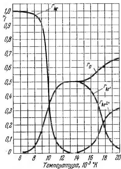
Рис. 26. Изменение объемных долей r_i ионизованного аргона в зависимости от температуры при p = 10^{-3} \text{ кг/см}^2 .
