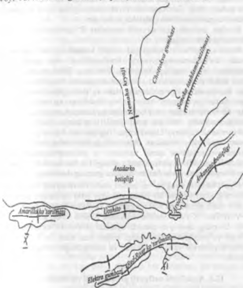
12.2.1-rasm. Uoshito – Uoshito burmahanligi (Okloxoma shtati) va yondosh rayonlardagi yirik geostruktura elementlarining joylashish sxemasi (Ver-Vibe, 1952-y.)
