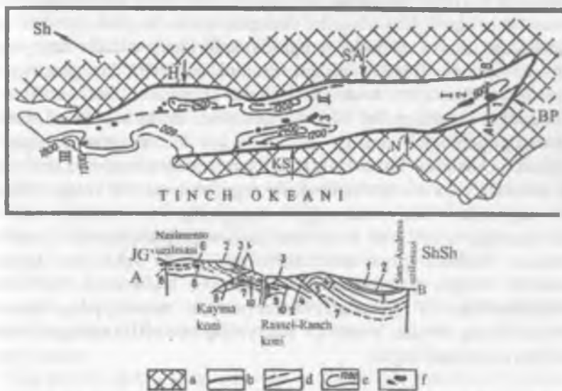
9.3.2- rasm. Xaf – Mun – Salinas – Kayama NGO va uning ko'ndalang kesimi sxemalari («Spravochnik», 1976 bo'yicha)
