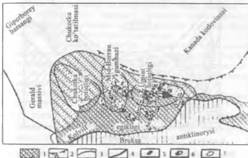
10.1.1-rasm. Alyaskaning Arktika qiyaligi neftgazli provinsiyasi
