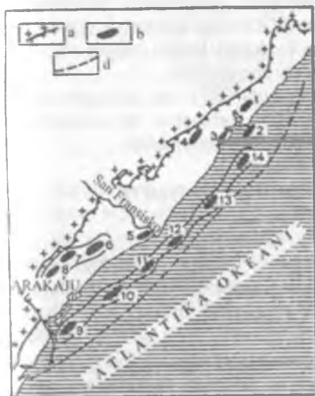
35.2.1-rasm. Serjipi-Alagoas neftgazli oblastida asosiy neft konlarining joylashishi sxematik xaritasi.
