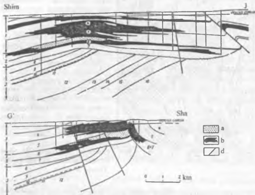
33.1.2-rasm. La-Sira-Infantas konlarining kesimi Uisk, 1954 y., bo'yicha. a – gaz; b – neft; d – tektonik buzilishlar.
