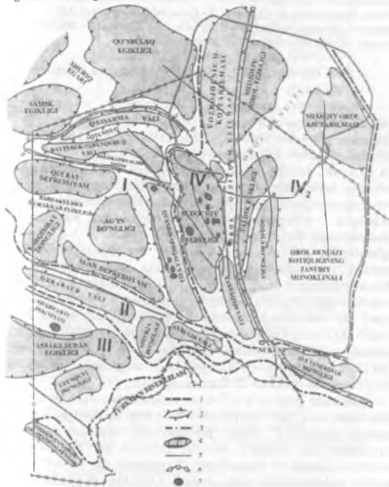
15.2.1-rasm. Ustyurt o‘lkasi. Geotektonik rayonlashtirish sxemasi
