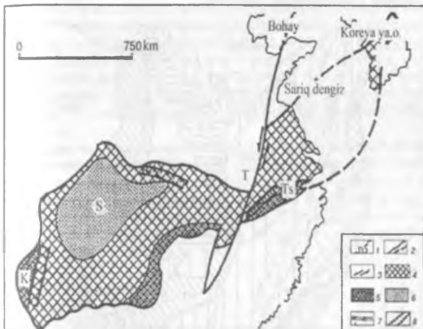
58.1-rasm. Yanszi platformasini tektonik rayonlashtirish (V.ye.Xain bo'yicha)
