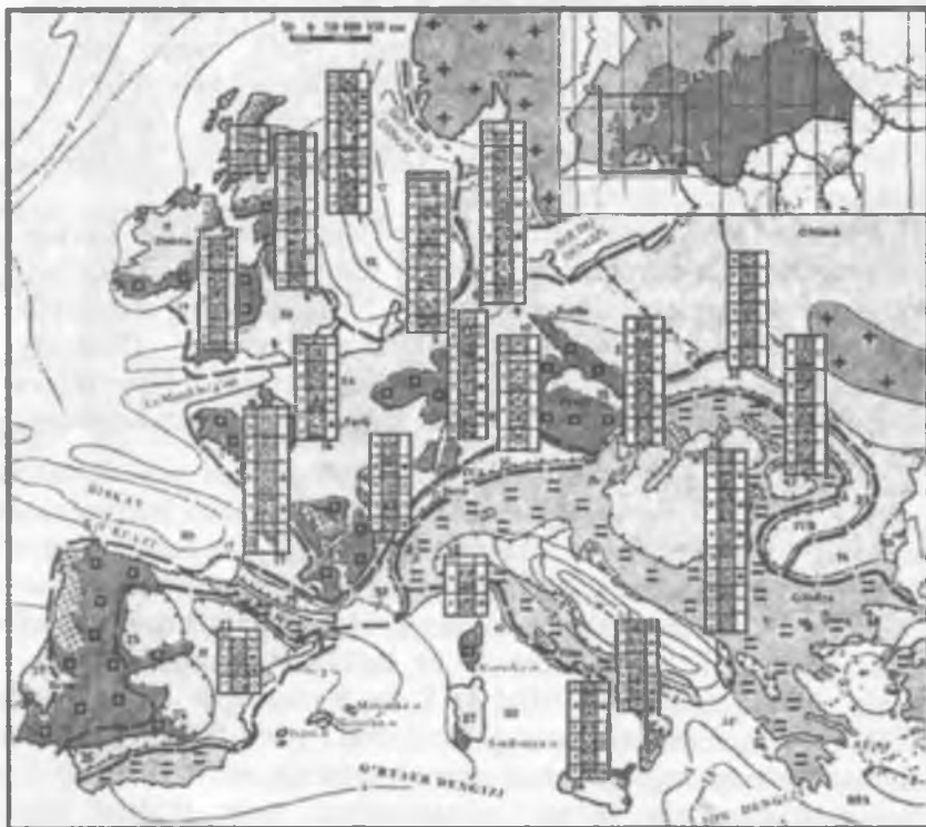
22.1-rasm. Evrosiyo litosfera plitasi (G'arbiy qismi) Neftgazgeologik elementlarning joylashish sxemasi
