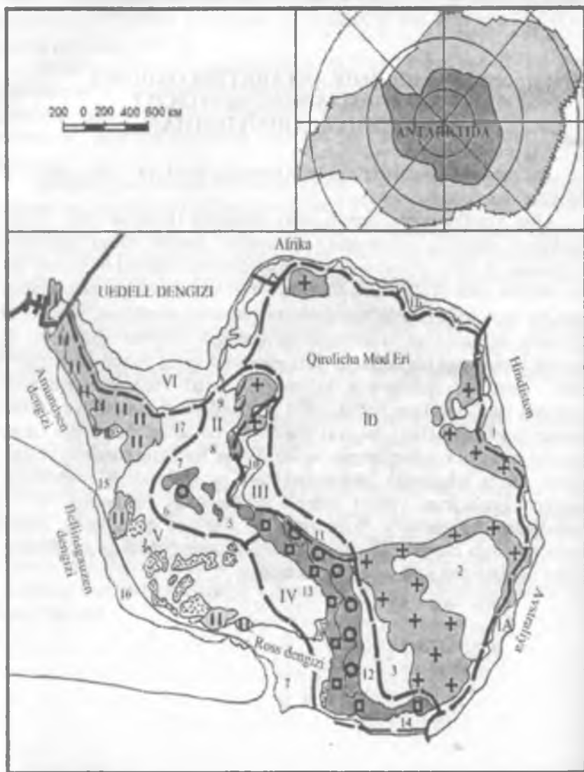
55.1-rasm. Antarktika litosfera plitasi. Neftgazgeologik elementlarning joylashish sxemasi.
