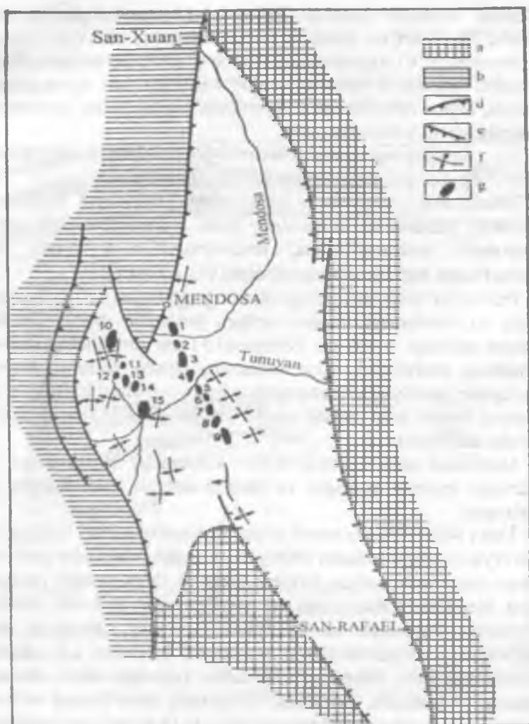
33.2.1-rasm. Mendoza neftgazli oblastining joylashishi
