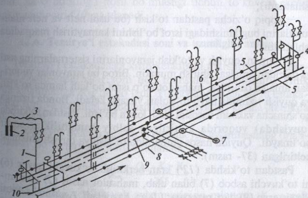
36- rasm. Temiryo'l estakadasi va qurilmalarining chizmasi: 1- to'kuvchi-quyuvchi ustun (stoyak); 2- ustunning oxirgi qismi; 3- rezinali qo'li; 4- vantuz; 5- to'kuvchi kollektor; 6- nosoz sisternalar uchun to'kuvchi kollektor; 7- kanalizatsiya quduqlari; 8- tarnov; 9- havo kollektori; 10- havo chiqaruvchi ventil.
