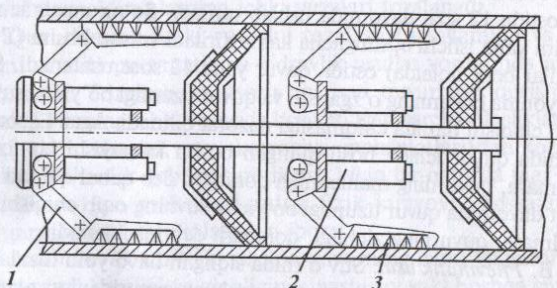
31- rasm. Metall taroqli «skrepka» chizmasi:
