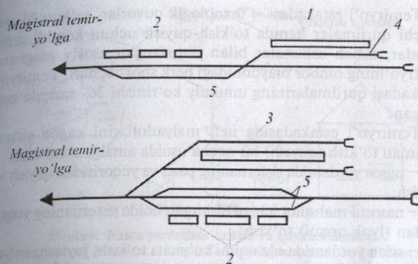
35- rasm. Temiryo'l berk estakadalarining umumiy chizmalari: 1- bir tomonli estakada; 2- idish mahsulotlarni saqlovchi omborlar; 3- ikki tomonli estakada; 4- to'kish tomoni; 5- manyovr uchun yo'l.
