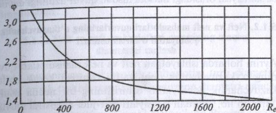
10- rasm. Laminar rejim uchun \xi — koeffitsiyenti qiymatlarining grafiqi.
