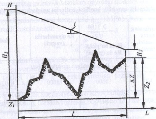
9- rasm. Quvurning gidravlik nishablik chizig'i.
