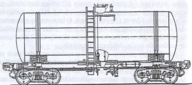
27- rasm. To'rt o'qli (60 t) vagon-sisternaning umumiy chizmasi.
