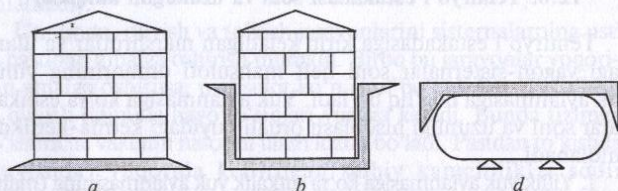
38- rasm. Rezervuarlarning yer yuzasiga nisbatan joylashishi: a— yer usti; b— yarim yer osti; d— yer osti.
