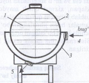
28- rasm. Sisterna ichidagi mahsulotni bug' «ko'ylagi» yordamida isitish: 1- neft mahsuloti; 2- sisterna; 3- isituvchi «ko'ylak»; 4- suv bug'ining kirishi; 5- suv kondensatining chiqishi.
