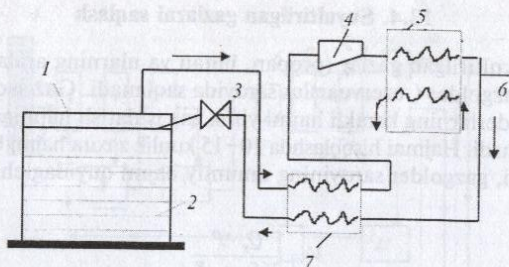
44- rasm. Suyultirilgan gazni izotermik sharoitda saqlash chizmasi: 1- issiqlik izolatsiyasi qoplangan yupqa devorli rezervuar; 2- suyuq gaz; 3- rostlash (drossellash) krani; 4- kompressor; 5- issiqlik almashtirgich; 6- sovitish uchun suv; 7- issiqlik almashtirgich.
