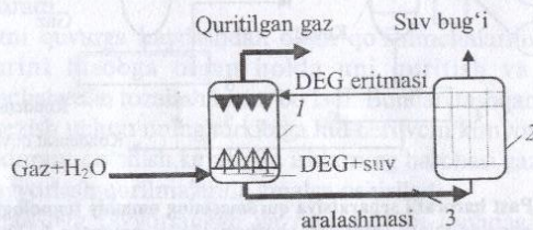
6- rasim. Gazni absorbent yordamida quritishning umumiy chizmasi: 1- absorber; 2- desorber; 3- aralashmani oqizuvchi quvur.
