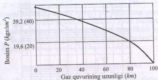
13- rasm. Gaz quvuridagi bosimlarning o'zgarish grafiqi.
