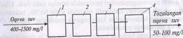
45- rasm. Mexanik tozalash tizimi qurilmalarining prinsipial chizmasi: 1- bufer rezervuari; 2- qum ushlagichi; 3- neft ushlagichi; 4- qo'shimcha hovuz (qum yoki neft ushlagichlar ishlamaganda undan foydalaniladi).
