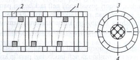
20- rasm. Spiral ko'rinishdagi ariqchasi bo'lgan quvurda suv va neftning oqish holati chizmasi: 1- quvur; 2- quvur ichidagi spiral ko'rinishdagi ariqcha; 3- suv oqimi; 4- neft oqimi.
