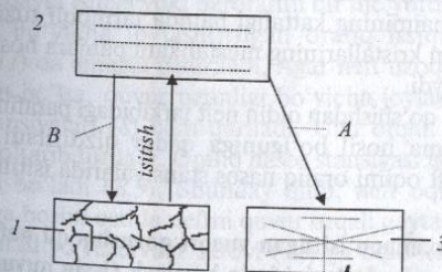
21- rasm. Yuqori qovushqoqli neftni issiqlik bilan ishlash rejimining prinsipial chizmasi: 1- yuqori qovushqoqli birlamchi neft tuzilishi; 2- qizdirishdan keyingi neft (bir jinsli eritma); 3- maxsus rejimda sovitilgan keyingi neft tuzilishi.
