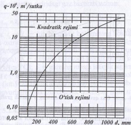
12- rasm. Quvur bo'yicha gazning oqish rejimlari grafigi.
