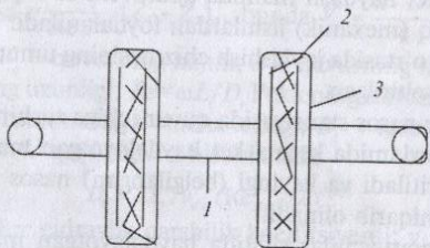
16- rasm. Diskli ajratuvchi: 1- shtanga (o'q); 2- elastik materialdan yasalgan disk; 3- metall disk.
