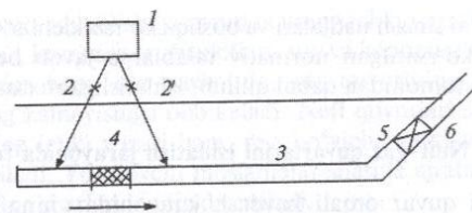
30- rasm. Gidravlik usulda tozalashning umumiy chizmasi: 1- suv bilan ta'minlovchi manba; 2, 2' - berkituvchi va ochuvchi kranlar; 3- magistrallik quvur; 4- ajratuvchi (tozalovchi) porshen; 5- kran; 6- potrubok (asosiy quvur uchiga o'rnatilgan quvur bo'lagi).
