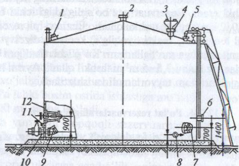
40- rasm. Po'lat rezervuar jihozlarning joylashish chizmasi:
