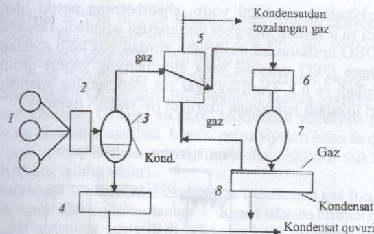
5- rasm. Past haroratli separatsiya qurilmasining umumiy texnologik chizmasi: 1— gaz quduqlari; 2— drossel shaybasi; 3— tik separator; 4— kondensat yig'uvchi idish; 5— gaz sovitgich; 6— bosimni moslab turuvchi shtutser; 7— tik separator, 8— yotiq past haroratli separator.
