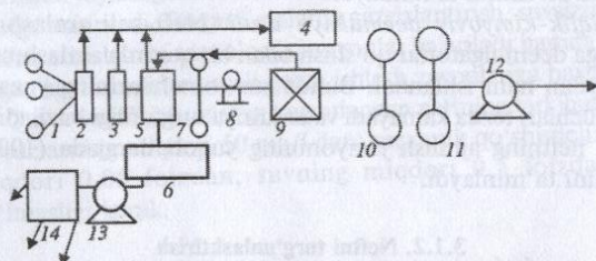
4- rasm. Neftni kompleks tayyorlash qurilma va jihozlarining umumiy texnologik chizmasi:
