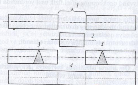
33- rasm. Quvur uzilishini bartaraf etish sxemasi: 1- jarohatlangan quvur bo'limi; 2- yangi quvur (potrubka); 3- loy to'sig'i; 4- avariya bartaraf qilingandan keyingi quvur.
