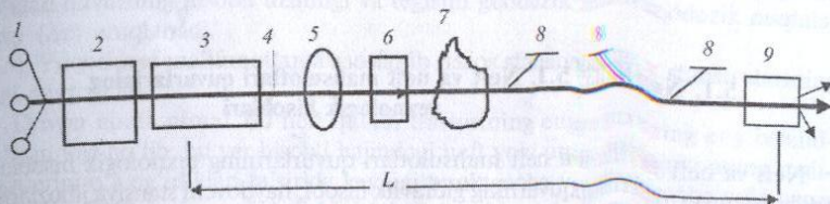
8- rasm. Magistral neft quvuri tarkibining umumiy chizmasi: 1- neft quduqlari; 2- bosh qurilmalar; 3- bosh nasos stansiyasi (BNS); 4- quvurning chiziqli bo'limi; 5 - sun'iy to'siqlar; 6- oraliq nasos stansiyalari (ONS); 7- tabiiy to'siqlar; 8- EKH vositalari; 9- neftni qayta ishlash zavodi yoki uzatuvchi neft ombori; L- magistral neft quvurining uzunligi.
