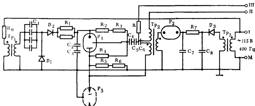
Рис. VIII.26. Принципиальная электрическая схема скважинного генератора: Tr — трансформатор; C — конденсатор; P — разрядная камера
