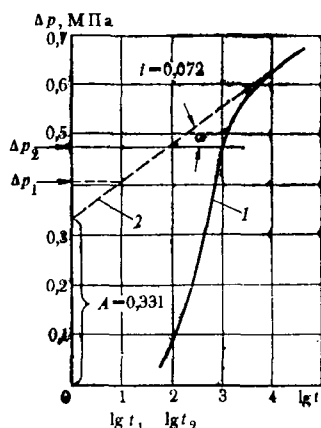
Рис. 1.6. Обработка кривой восстановления давления без учета дополнительного притока:
