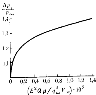
Рис. VIII.16. График зависимости \Delta p_c/p_{\infty} от E^2 Q \mu / q^3 V_{ж}
