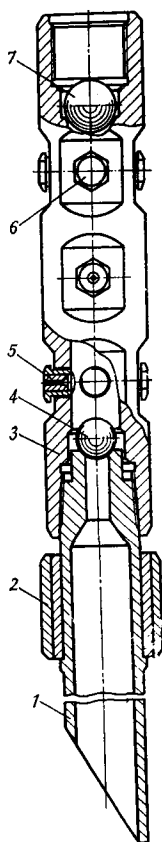
Рис. VIII.8. Перфоратор АП-6М100:
