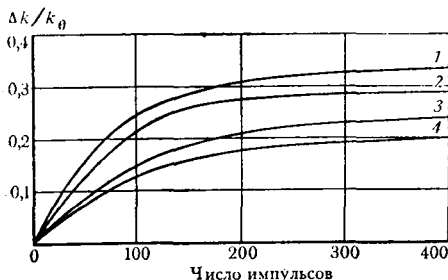
Рис. VIII.24. Изменение проницаемости образцов песчанника в зависимости от числа импульсов ( \Delta k/k_0 — отношение прироста проницаемости образцов к начальной их проницаемости):
