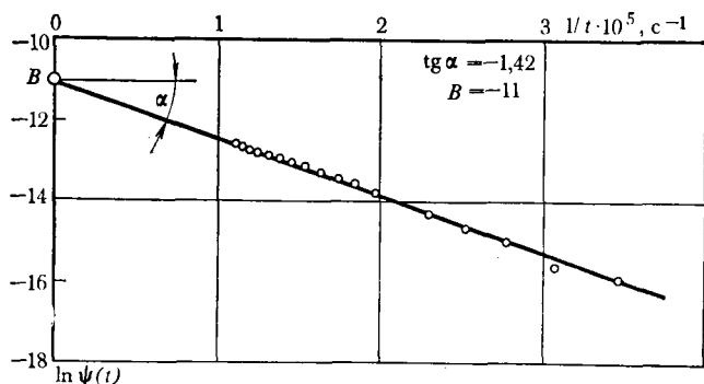
Рис. I.15. Обработка кривой реагирования при однократном скачкообразном изменении дебита возмущающей скважины интегральным методом
