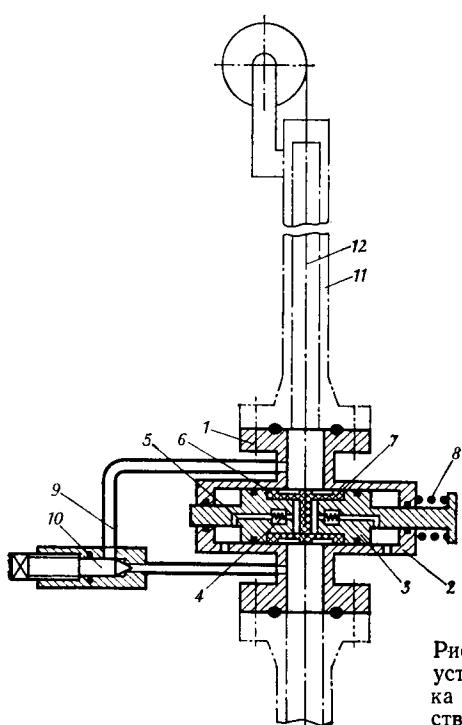
Рис. П.3. Устройство для предотвращения и ликвидации аварий
