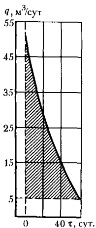
Рис. VII.15. Изменение дебита скважины после термоакустической обработки
