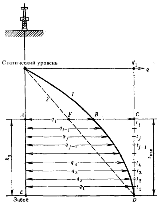
Рис. IV.9. Восстановление уровня при нелинейном (1) и линейном (2) притоке:
