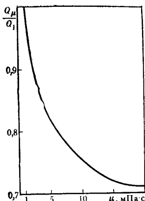
Рис. III.2. Зависимость отнoсительного дебитa ( Q_\mu/Q_1 ) от абсолютной вязкости \mu .
