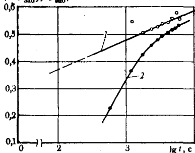
Рис. I.8. К примеру обработки кривой восстановления давления с учетом дополнительного притока дифференциальным методом:
