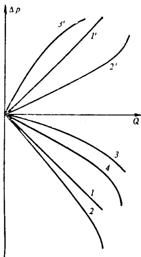
Рис. I.1. Характерные типы индикаторных диаграмм:
