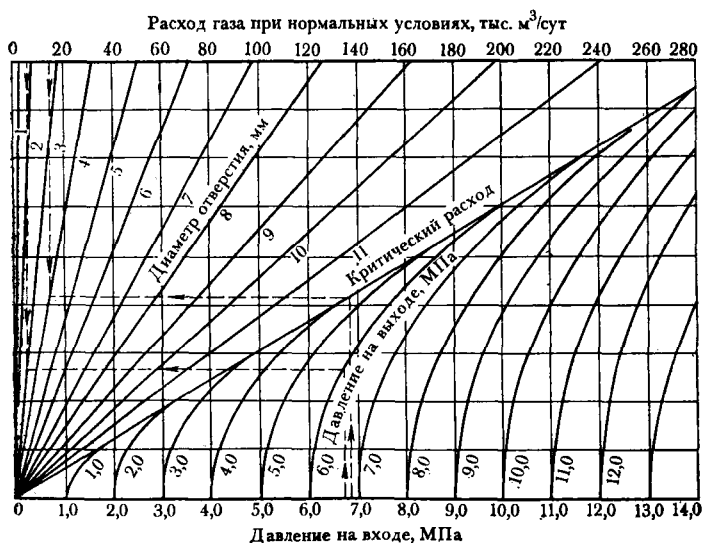
Рис. III.22. Номограмма для определения диаметра седла клапана
