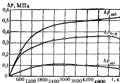
Рис. 1.7. Промысловые графики изменения забойного, межтрубного и буферного давления
