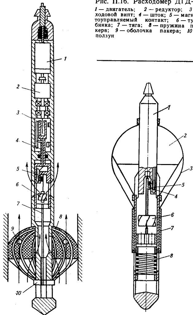
Рис. II.17. Расходомер «Терек-3» с бесприводным пакером:
