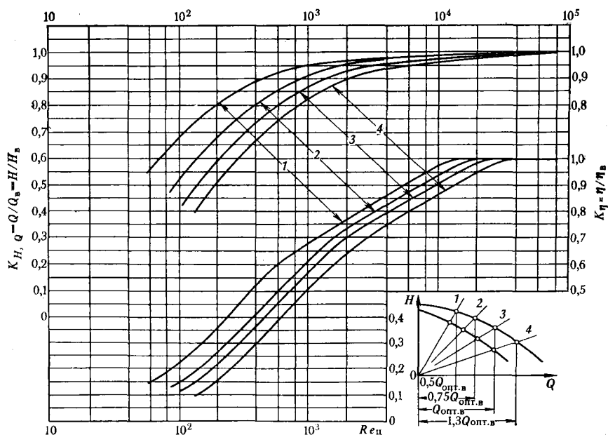
Рис. VI.8. Зависимость относительных подачи и напора K_{QH} и относительного к. п. д. K_{\eta} погружного центробежного насоса от модифицированного числа Re_{\text{ц}} потока в его межлопаточных каналах для различных соответственных режимов Q_{\text{в}}/Q_{\text{опт.в}} :
