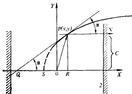
Рис. VIII.27. Схема строения отражателя:
