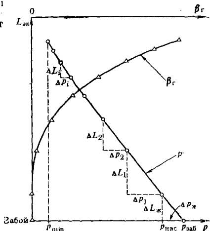
Рис. VI.6. Изменение давления и объемной расходной доли свободного газа \beta_{\text{г}} в потоке вдоль ствола скважины при постоянном дебите жидкости
