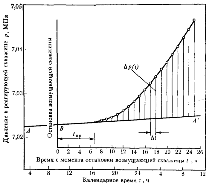
Рис. I.14. Изменение давления в реагирующей скважине при скачкообразном однократном изменении дебита возмущающей скважины
