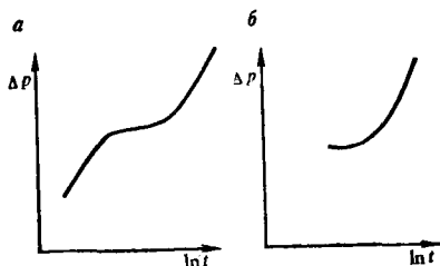
Рис. 1.10. Формы кривых восстановления давления для трещиноватых коллекторов
