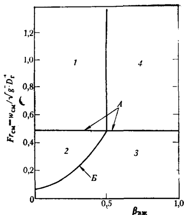
Рис. VI.1. Карта структурных форм водонефтяного и водонефтегазового потоков в колонне подъемных труб и в стволе скважины. 1 — \omega_{\text{см}} \geq 0,487 \sqrt{g d_g} , \beta_{\text{вж}} \leq 0,5 ; эмульсионная структура водонефтяного потока типа В/Н; эмульсионно-пузырьковая структура водонефтегазового потока типа (B+G)/H , если \varphi_r \leq 0,65 или p \geq 7 МПа; эмульсионно-снарядная структура водонефтегазового потока типа (B+G)/H , если \varphi_r \leq 0,65 при p \leq 7 МПа;
