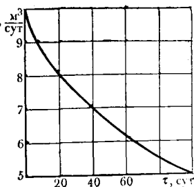
Рис. VII.7. Изменение дебита скважины после обработки
