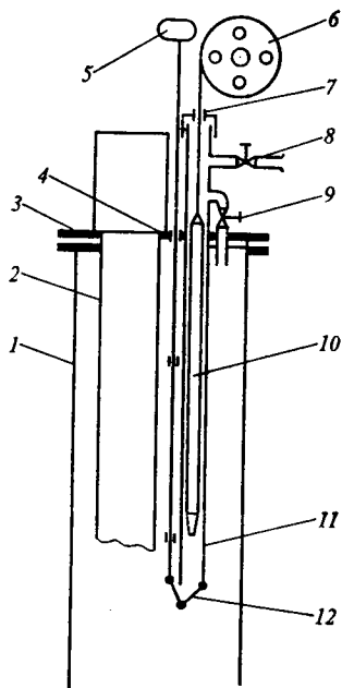
Рис. П.4. Схема оборудования устья насосной скважины для спуска приборов в межтрубное пространство:
