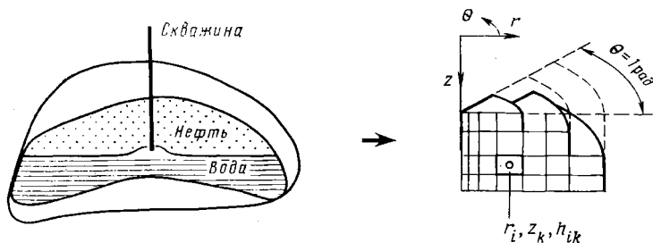
Рис. 9.3. Представление пласта сеткой в цилиндрических координатах
