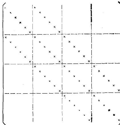
Рис. 8.13. Матрица V в уравнении (8.68) при использовании упорядочения по строкам. Элементы, не равные нулю, обозначены \times . К примеру, для десятой строки эти элементы следующие: g_{3,2} ; ay_{3,2} ; f_{3,2}
