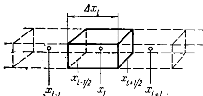
Рис. 3.1. Разбиение на блоки в од- номерном случае
