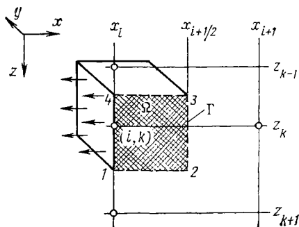
Рис. 7.9. Типичный граничный блок сетки в профильной модели
