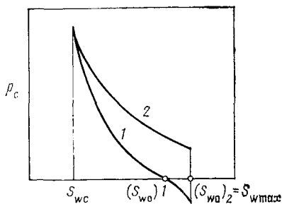
Рис. 5.16. Определение S_{w0} для двух различных кривых P_c
