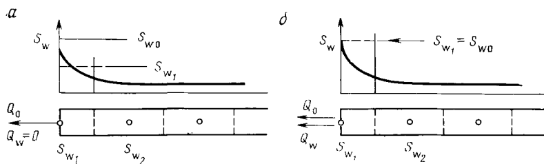
Рис. 5.19. Профиль насыщенности до (а) и после (б) прорыва воды
