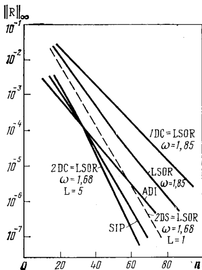
Рис. 8.21. Результаты тестовых расчетов для задачи 4 (Сеттари и Азиз, 1973)
