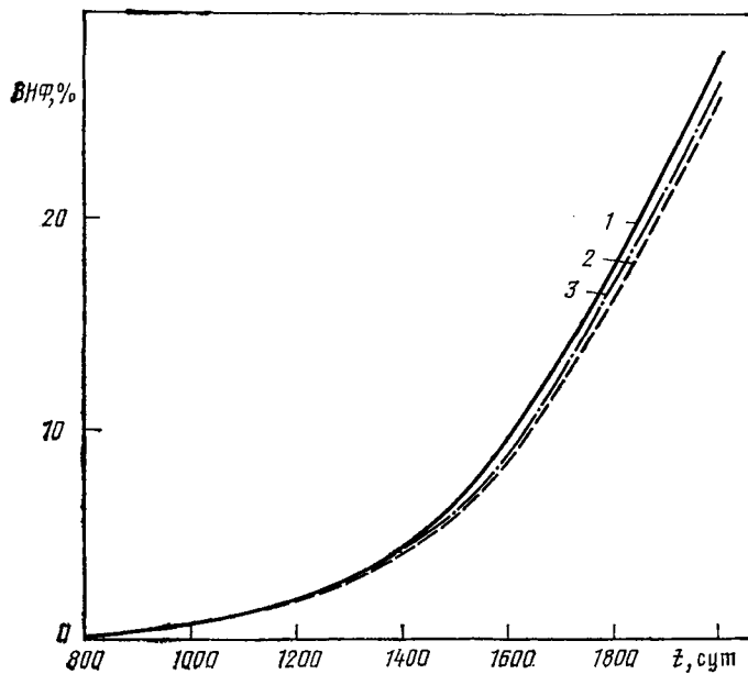
Рис. 9.22. Сравнение SS и SEQ-моделей для задачи Блэра и Уэйнауга. Модели: 1 — SS; 2 — SEQ (модель I); 3 — SEQ (модель II)
