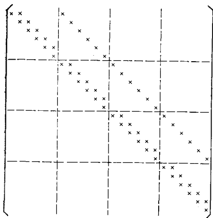
Рис. 8.15. Вид матрицы U по методу Стоуна. Элементы, не равные нулю, обозначены \times . К примеру, для десятой строки эти элементы следующие: 1; b_{3,2}; f_{3,2}
