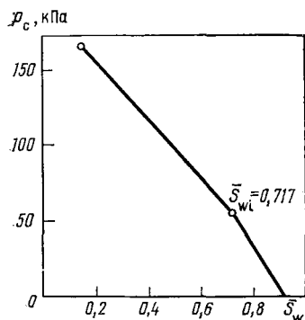
Рис. 12.2. Зависимость псевдокапиллярного давления от средней насыщенности (Коутс и др., 1971)
