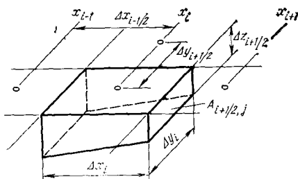
Рис. 7.5. Типичный блок сетки, приведенной на рис. 7.4
