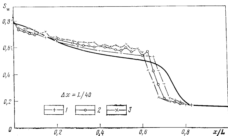
Рис. 5.13. Оценка устойчивости SEQ-метода при учете P_c по методу касательных для модифицированной контрольной задачи 1 при больших значениях P_c 1—3 — см. рис. 5.12
