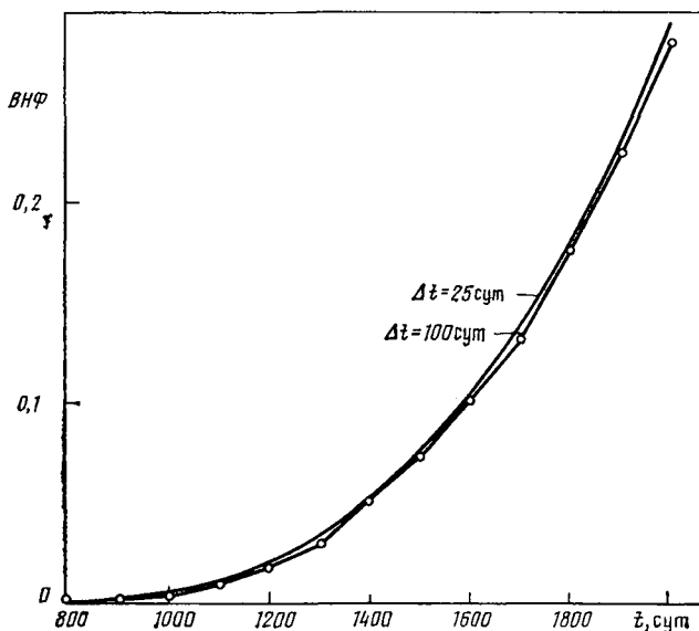
Рис. 9.21. Чувствительность модели Сеттари и Азиза к временному шагу для задачи Блэра и Уэйнауга
