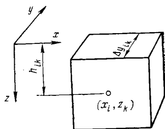
Рис. 7.2. Типичный блок профильной модели
