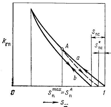
Рис. 12.10. Модель гистерезиса для k_{rn}
