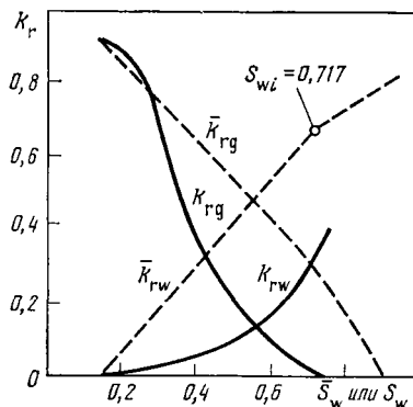
Рис. 12.3. Зависимость относительных и псевдоотносительных проницаемостей от насыщенностей (Коутс и др., 1971)
