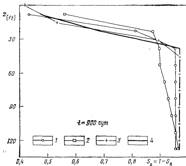
Рис. 5.9. Сравнение результатов по трем методам для контрольной задачи 2 Маккрири при просачивании газа (Сеттари и Азиз, 1975)
