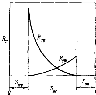
Рис. 2.6. Типичные кривые относительных фазовых проницаемостей
