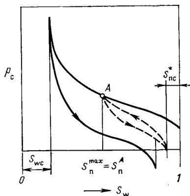
Рис. 12.9. Промежуточная кривая P_c , берущая начало на кривой первичного вытеснения
