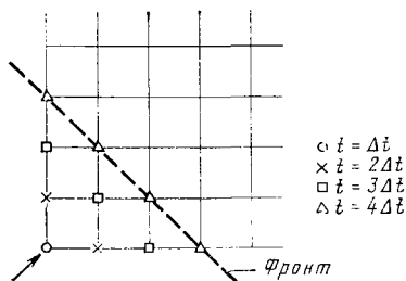
Рис. 9.18. Распространение подвижного состояния при явном определении проводимостей
