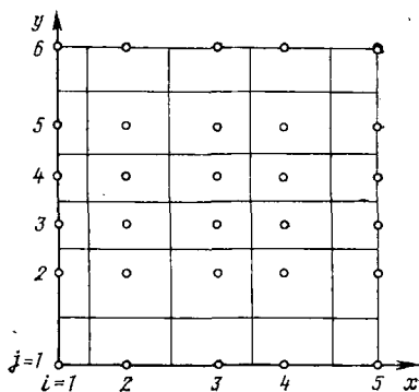
Рис. 7.4. Типичная сетка двумерных моделей с координатами x, y
