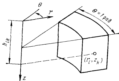
Рис. 7.3. Типичный блок модели со скважиной в координатах r, z
