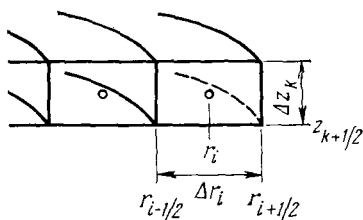
Рис. 7.6. Границы блока в радиальном направлении
