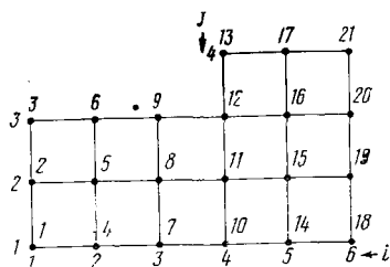
Рис. 8.3. Сетка, состоящая более чем из одного прямоугольника
