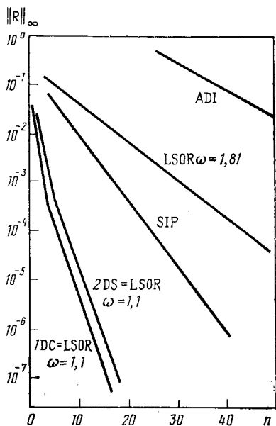
Рис. 8.19. Результаты тестовых расчетов для задачи 2 (Сеттари и Азиз, 1973)
