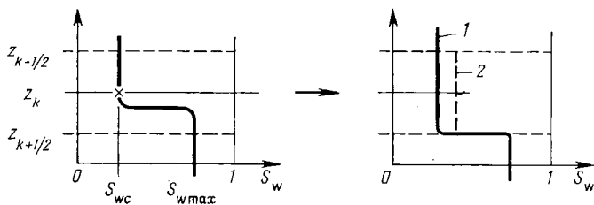
Рис. 9.8. Дискретизация начальных условий: 1 — задание начального состояния модели; 2 — фактическая средняя насыщенность в блоке
