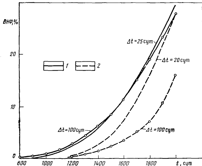
Рис. 9.20. Чувствительность моделей Леткемана и Ридингса, а также Нолен и Берри к временному шагу для задачи Блэра и Уэйнауга Модели: 1 — Нолен и Берри (полунеявный метод); 2 — Леткемана и Ридингса
