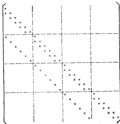
Рис. 8.16. Вид матрицы L по методу Стоуна. Элементы, не равные нулю, обозначены \times . К примеру, для десятой строки эти элементы следующие: g_{3,2}; c_{3,2}; a_{3,2}
