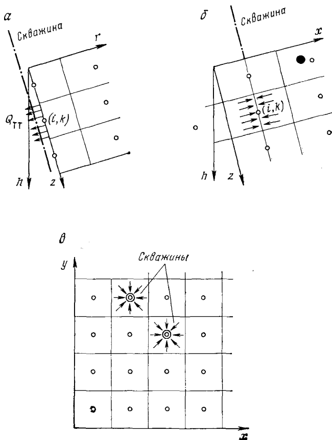
Рис. 9.6. Представление скважин в сетках различного типа Модели: а — одиночной скважины; б — профильная; в — площадная
