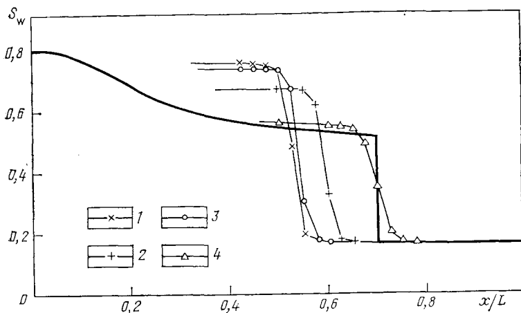
Рис. 5.2. Результаты решения по «средневзвешенной схеме» при различных P_c (контрольная задача 1: \Delta x=L/40 ; \Delta t=10 сут; t=1500 сут) 1 — P_c — измеренное; 2 — P_c \times 10 ; 3 — P_c \times 50 ; 4 — P_c \times 200
