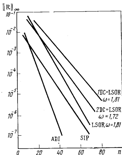
Рис. 8.18. Результаты тестовых расчетов для задачи 1 (Сеттари и Азиз, 1974)
