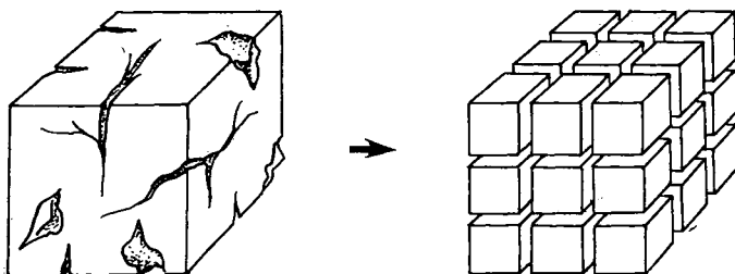
Рис. 12.12. Идеализированное представление трещиноватого пласта
