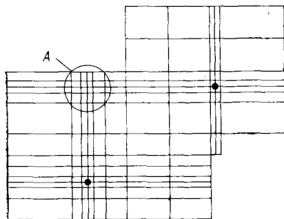
Рис. 7.14. Типичная неравномерная сетка для площадной модели
