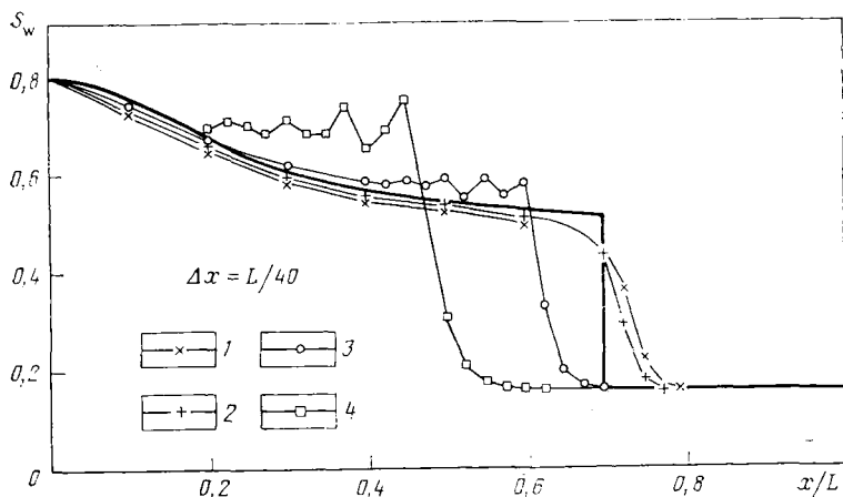
Рис. 5.5. Оценка устойчивости линеаризованного неявного SS-метода для контрольной задачи 1 при t=1500 сут (Сеттари и Азиз, 1975) Шаг \Delta t в сут: 1 — 25; 2 — 50; 3 — 100; 4 — 187,5
