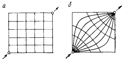
Рис. 7.17. Сетка для моделирования пятиточечной системы заводнения
