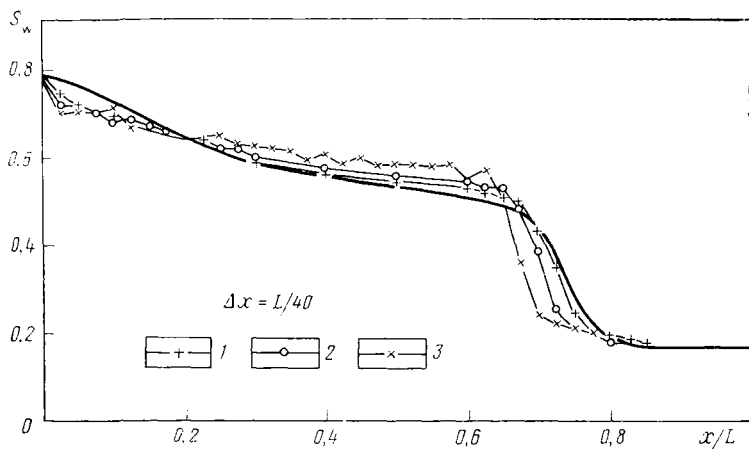
Рис. 5.14. Оценка устойчивости SEQ-метода при учете P_c по методу секущих для модифицированной контрольной задачи 1 при больших значениях P_c 1—3 — см. рис. 5.12
