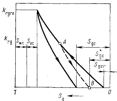
Рис. 12.11. Гистерезис k_{rn} по Коутсу (1976 а)
