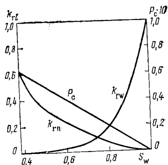
Рис. 2.10. Типичные зависимости свойств породы для системы газ — нефть, когда нефть — смачивающая фаза (Сеттари и Азиз, 1975)
