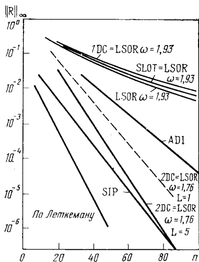
Рис. 8.20. Результаты тестовых расчетов для задачи 3 (Сеттари и Азиз, 1973)
