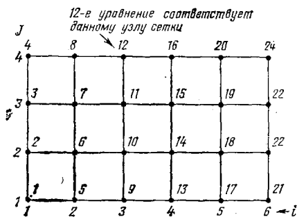
Рис. 8.1б. Стандартное упорядочение по столбцам (или по индексу j )
