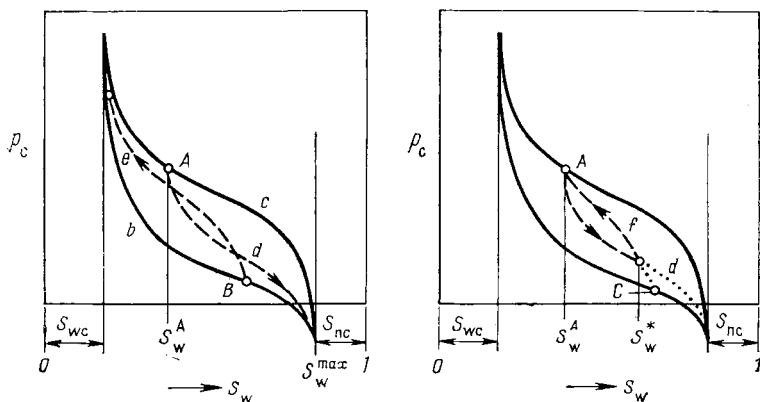
Рис. 12.8. Промежуточные кривые P_c . Слева возврат начинается на предельных кривых, справа — возврат начинается на промежуточной кривой
