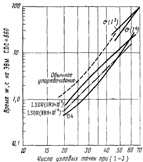
Рис. 8.26. Сравнение эффективности прямых методов (D4 и обычное упорядочение) и метода LSOR
