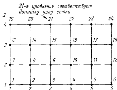
Рис. 8.1а. Стандартное упорядочение по строкам (или по индексу i )
