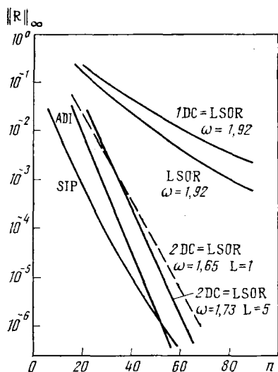
Рис. 8.24. Результаты тестовых расчетов для задачи 7 (Сеттари и Азиз, 1973)
