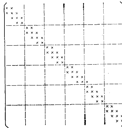
Рис. 8.14. Матрица V в уравнении (8.68) при использовании упорядочения по столбцам. Элементы, не равные нулю, обозначены \times . К примеру, для десятой строки эти элементы следующие: g_{3,2} ; ay_{3,2} ; f_{3,2}
