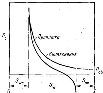
Рис. 2.5. Типичная кривая капиллярного давления
