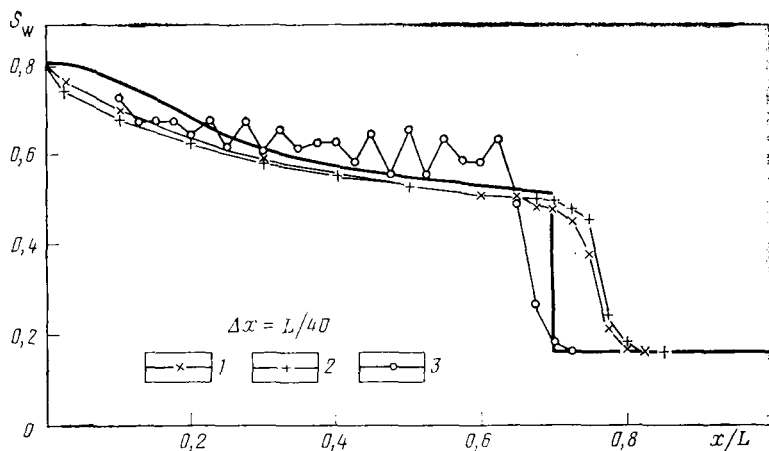
Рис. 5.11. Оценка устойчивости SEQ-метода при проводимостях, линейризованных по методу секущих, и \delta S_w = 0,32 (контрольная задача 1) 1—3 см. рис. 5.10
