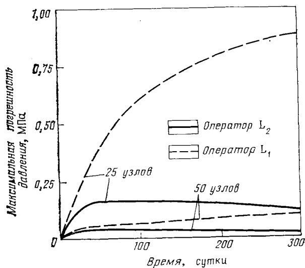
Рис. 3.13. Влияние уменьшения шага сетки на погрешность, полученную для операторов L_1 и L_2
