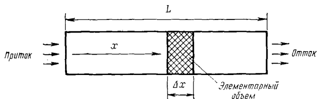
Рис. 2.1. Схема линейной фильтрации в цилиндрическом образце длины \Delta x
