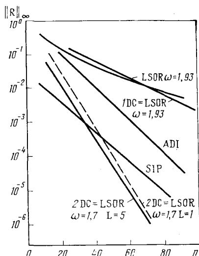
Рис. 8.23. Результаты тестовых расчетов для задачи 6 (Сеттари и Азиз, 1973)
