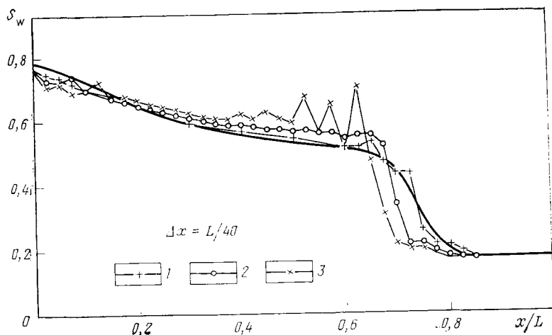
Рис. 5.12. Оценка устойчивости SEQ-метода при явном учете P_c для модифицированной контрольной задачи 1 при больших значениях P_c Шаг \Delta t в сут: 1 — 75; 2 — 100; 3 — 125
