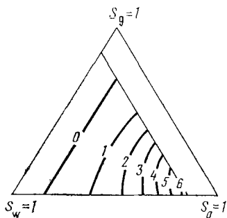
Рис. 2.11. Относительные проницаемости при трехфазной фильтрации, определенные по моделям Стоуна (I и II).
