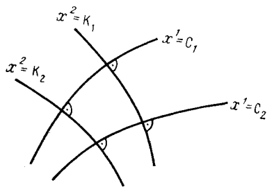
Рис. 7.18. Ортогональная система координат
