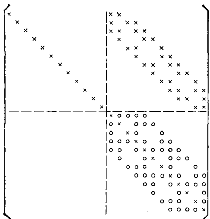
Рис. 8.10. Преобразованная матрица для упорядочения по схеме D4
