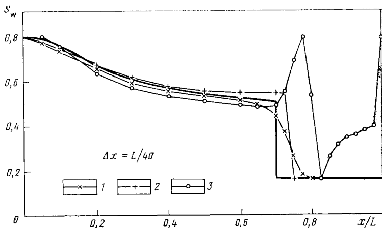
Рис. 5.6. Оценка устойчивости полунеявного SS-метода с использованием касательных для контрольной задачи 1 при t=1500 сут (Сеттари и Азиз, 1975) 1—3 — см. рис. 5.4
