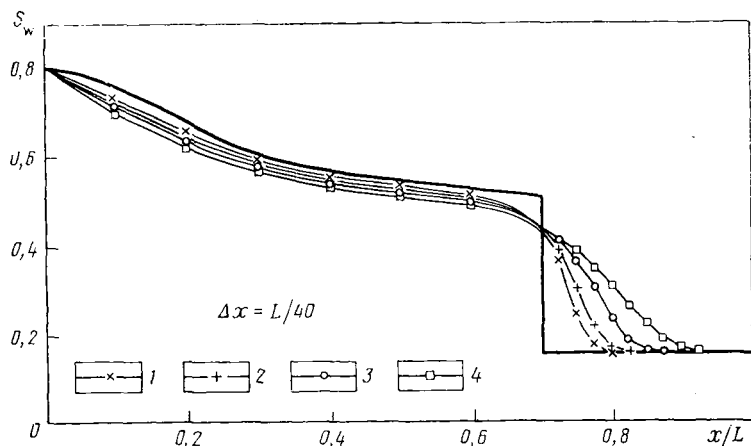
Рис. 5.8. Оценка устойчивости неявного метода для контрольной задачи 1 при t=1500 сут (Сеттари и Азиз, 1975).
