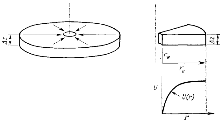
Рис. 3.17. Одномерная радиальная фильтрация: r_w и r_e соответственно радиус скважины и внешний радиус дренирования
