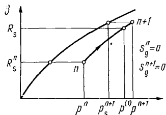
Рис. 12.6. Схема моделирования переменного давления насыщения (Страйт и др., 1977)
