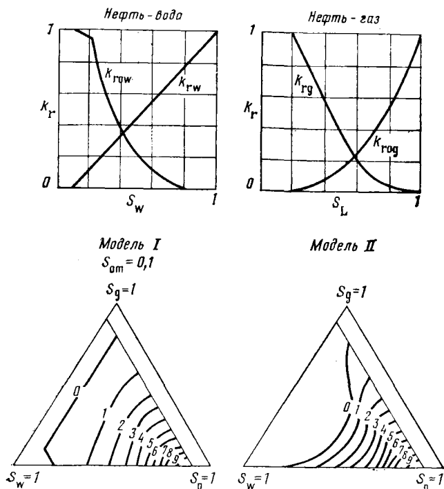
Рис. 2.12. Относительные проницаемости при трехфазной фильтрации, определенные по моделям Стоуна (I и II)
