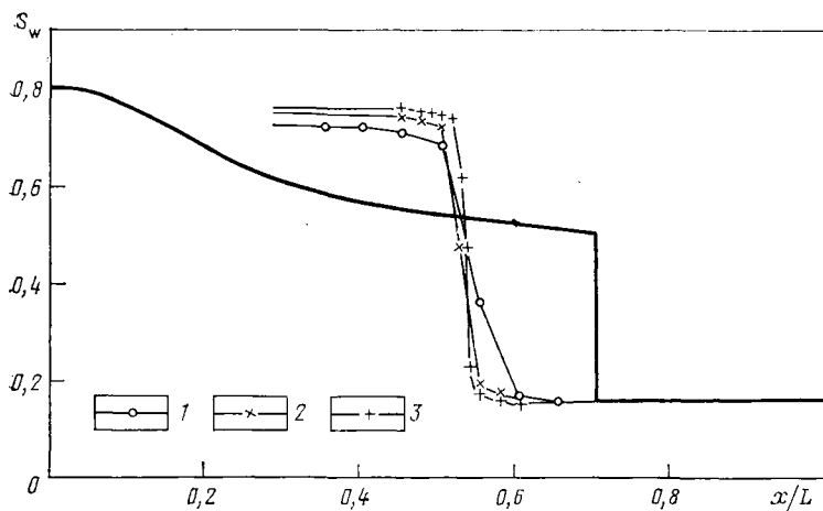
Рис. 5.1. Результаты сходимости «средневзвешенной» схемы — задача, близкая к гиперболической (контрольная задача 1) t=1500 сут) 1 — N=20 , \Delta t=10 сут; 2 — N=40 , \Delta t=10 сут; 3 — N=60 , \Delta t=5 сут
