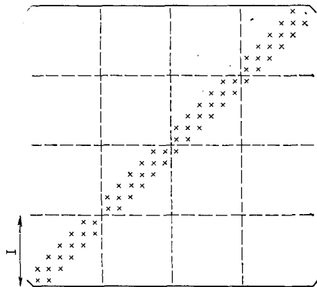
Рис. 8.12. Матрица H в уравнении (8.68) при использовании упорядочения по строкам. Элементы, не равные нулю, обозначены \times . К примеру, для десятой строки эти элементы следующие: c_{3,2} ; ax_{3,2} ; b_{3,2}
