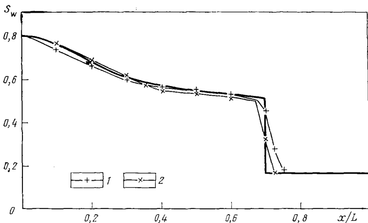
Рис. 5.3. Сравнение схем «взвешивания по потоку» (контрольная задача 1: \Delta x = L/40 ; \Delta t = 10 сут; t = 1500 сут (Сеттари и Азиз, 1975)) 1 — «одноточечное взвешивание» вверх по потоку; 2 — «двухточечное взвешивание вверх по потоку»
