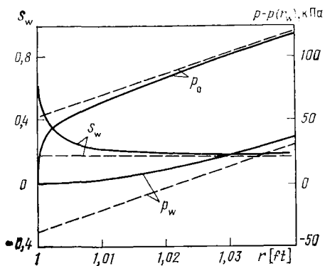
Рис. 5.18. Вычисленные распределения давления и насыщенности у скважины при наличии и отсутствии конечного эффекта (Азиз и Сеттари, 1974)
