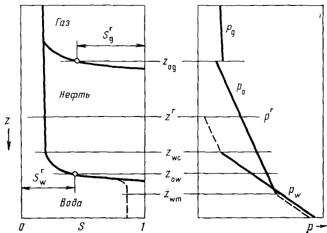
Рис. 9.7. Распределение начальной насыщенности и давления в пласте
