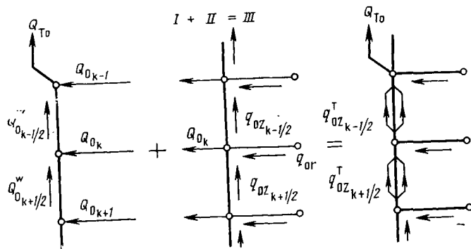
Рис. 9.19. Комбинация уравнений для ствола скважины и уравнений для пласта (II), I — уравнение для ствола скважины; II — уравнение для пласта; III — модифицированное уравнение
