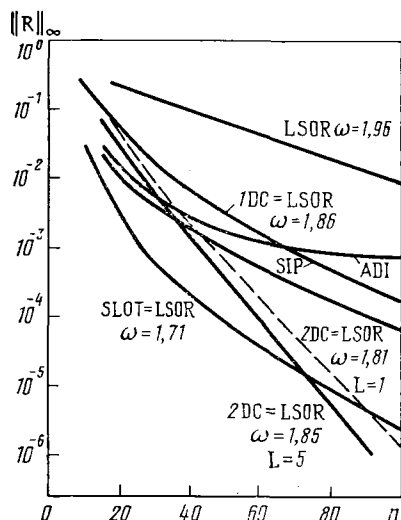
Рис. 8.22. Результаты тестовых расчетов для задачи 5 (Сеттари и Азиз, 1973)
