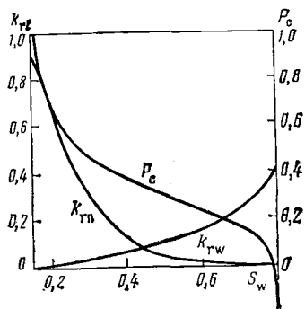
Рис. 2.9. Типичные зависимости свойств породы для системы вода — нефть, когда вода — смачивающая фаза (Сеттари и Азиз, 1975)
