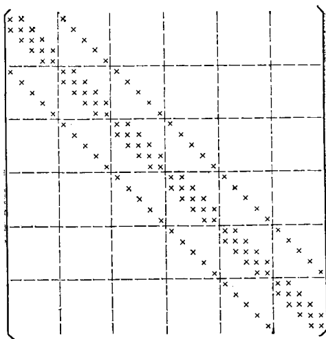
Рис. 7.13. Вид матрицы коэффициентов уравнения (7.84)
