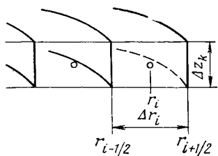
Рис. 9.5. Типичный элемент цилиндрической сетки
