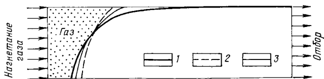
Рис. 9.17. Эффект численной дисперсии в профильной задаче о нагнетании газа. 1 — точное решение; 2 — конечно-разностное решение, грубая сетка; 3 — конечно-разностное решение, мелкая сетка
