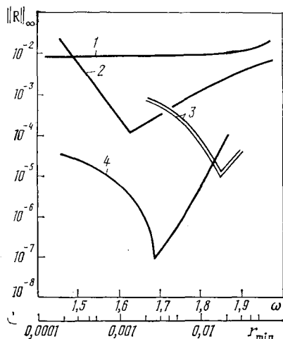
Рис. 8.25. Оптимальные итерационные параметры, определенные опытным способом с помощью графиков \|R\| для фиксированного числа итераций
