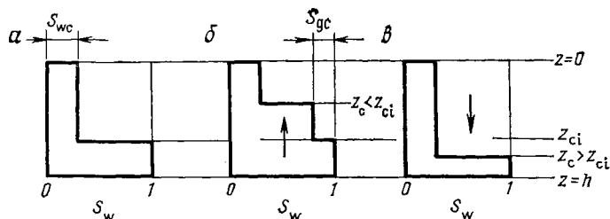
Рис. 12.1. Распределение флюидов по вертикали в состоянии гравитационного равновесия
