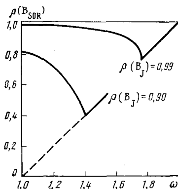
Рис. 8.11. Зависимость спектрального радиуса \rho B_{SOR} от \omega
