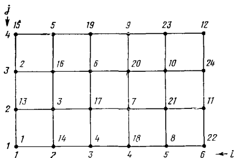
Рис. 8.7а. Схема упорядочения D4 Рис. 8.7б. Матрица A для упорядочения D4
