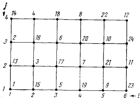
Рис. 8.8а. Схема двухциклического упорядочения Рис. 8.8б. Матрица A для двухциклического упорядочения
