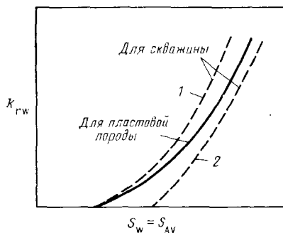
Рис. 9.12. Псевдоотносительные проницаемости для скважины
