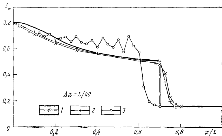
Рис. 5.10. Оценка устойчивости SEQ-метода при проводимостях линейризованных по методу касательных (контрольная задача 1) Шаг \Delta t в сут: 1 — 25; 2 — 50; 3 — 100
