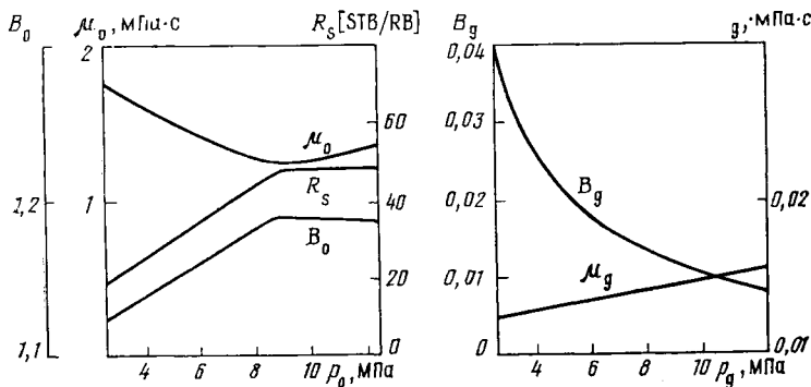
Рис. 2.4. Типичные зависимости свойств нефти (слева) и газа (справа) от давления (Сеттари Азиз, 1975)
