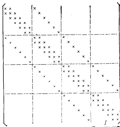
Рис. 8.2а. Вид матрицы А для стандартного упорядочения неизвестных по строкам, показанного на рис. 8.1,а. Элементы, не равные нулю, отмечены знаками \times . К примеру, для девятой строки ( i=3 , j=2 ) эти элементы следующие: g_{3,2} ; c_{3,2} ; a_{3,2} ; b_{3,2} ; f_{3,2}
