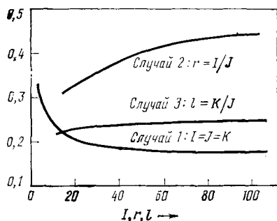
Рис. 11.2. Отношение объемов вычислений для различных трехмерных задач
