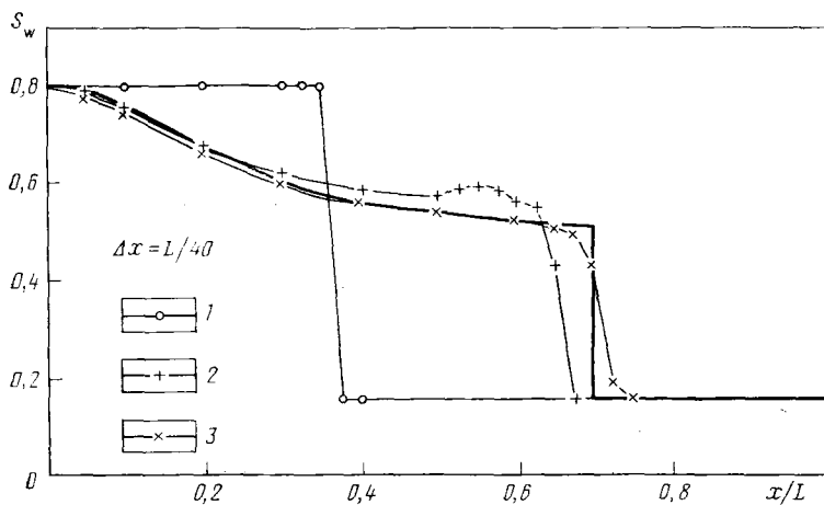
Рис. 5.4. Оценка устойчивости SS-метода с явными проводимостями для контрольной задачи 1 при t=1500 сут. Шаг \Delta t — в сут: 1 — 25; 2 — 50; 3 — 100
