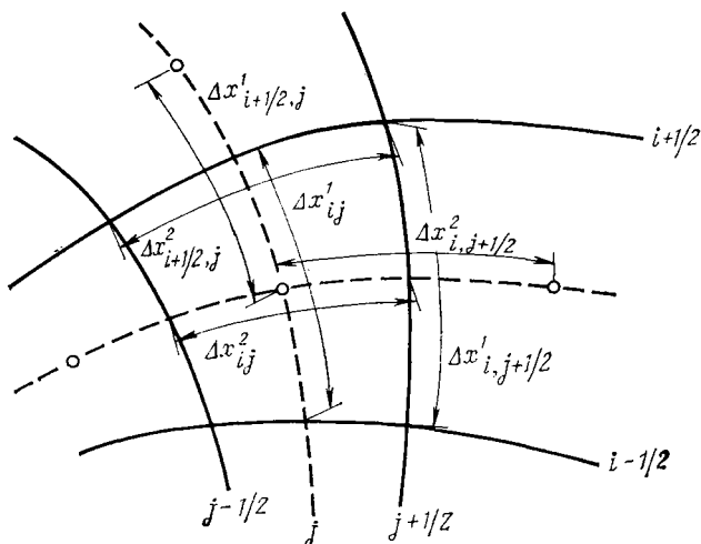
Рис. 7.19. Сетка в криволинейной системе координат
