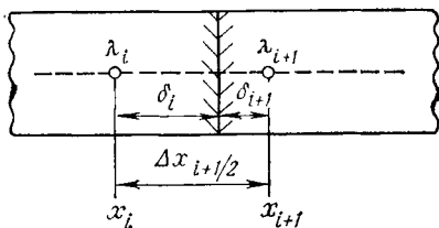
Рис. 3.14. Осреднение проводимости для вертикального раздела
