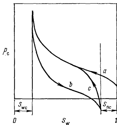
Рис. 12.7. Кривые гистерезиса капиллярного давления
