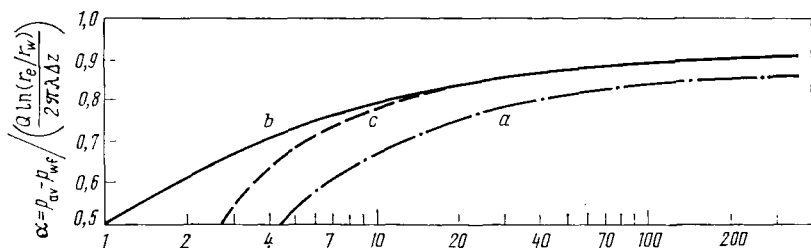
Рис. 7.11. Различные способы определения давления на скважине по среднему давлению: (а) уравнение (7.60); (б) уравнение (7.63); (с) уравнение (7.64)
