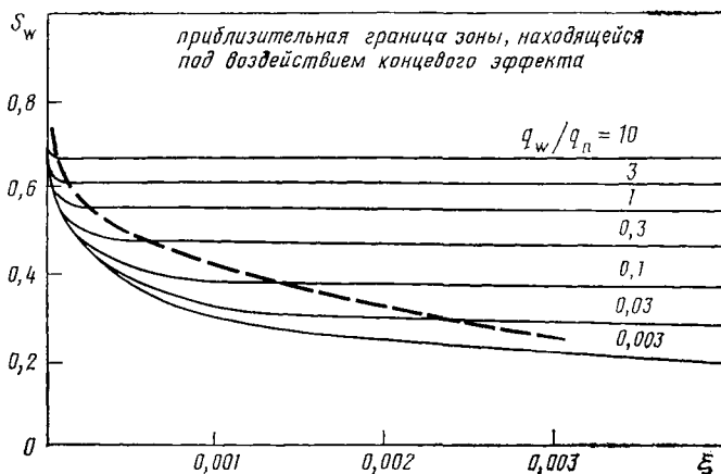
Рис. 5.17. Результаты расчета насыщенности на выходе при одномерном радиальном течении по данным Блэра и Уэйнауга (Сеттари и Азиз, 1974)
