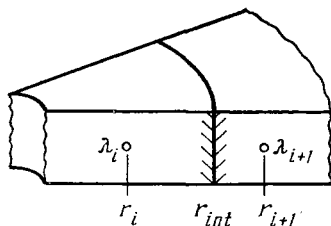
Рис. 3.18. Осреднение проводимости для вертикальной поверхности раздела
