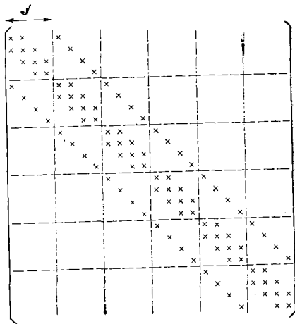
Рис. 8.2,б. Вид матрицы А, показанной на рис. 8.1,б для стандартного упорядочения неизвестных по столбцам. Элементы, не равные нулю, отмечены знаком \times . К примеру, для десятой строки ( i=3 , j=2 ) эти элементы следующие: c_{3,2} ; g_{3,2} ; a_{3,2} ; f_{3,2} ; b_{3,2}
