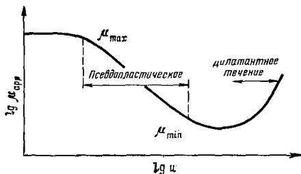
Рис. 2.3. Кажущаяся вязкость для неньютоновских флюидов (Бондору и др., 1972)
