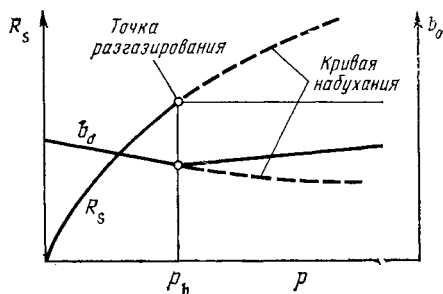
Рис. 12.4. Зависимость растворимости газа в нефти от давления
