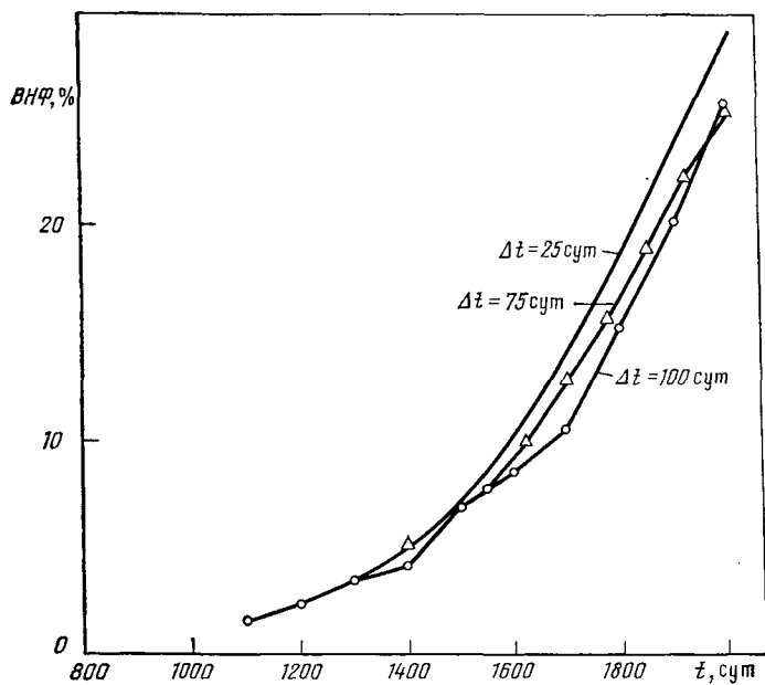
Рис. 9.23. Чувствительность SEQ-модели I к временному шагу
