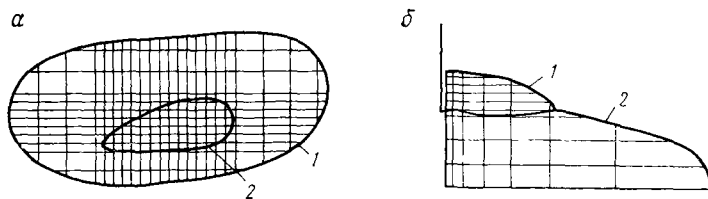
Рис. 9.9. Примеры сеток, охватывающих продуктивный и водоносный пласты 1 — граница продуктивного пласта; 2 — граница водоносного пласта; а — площадная сетка; б — цилиндрическая сетка
