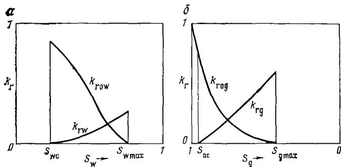
Рис. 2.7. Кривые относительных фазовых проницаемостей а — система нефть — вода; б — система газ — нефть
