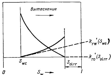
Рис. 9.24. Схема учета наклона кривых k_r в конечных точках
