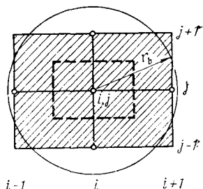
Рис. 7.12. К определению r_b в уравнении (7.71)
