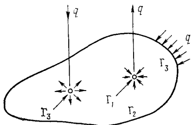
Рис. 7.7. Границы в площадных системах
