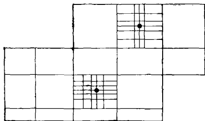
Рис. 7.15. Локальное измельчение сетки
