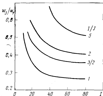
Рис. 8.9. Сравнение объемов вычислений при упорядочении по схеме D4 и стандартном упорядочении
