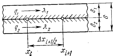
Рис. 3.15. Осреднение проводимости для слоистой системы
