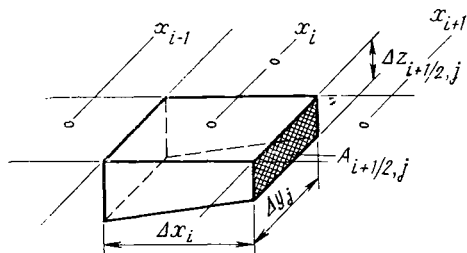
Рис. 9.4. Типичный элемент площадной сетки
