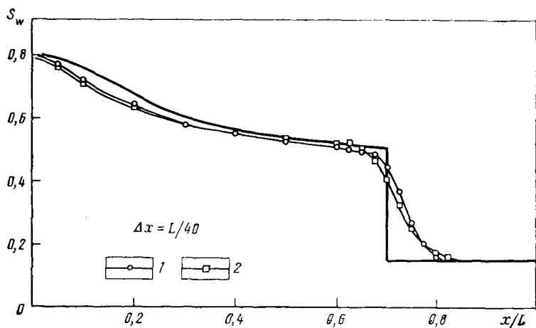
Рис. 5.7. Оценка устойчивости полунявного SS-метода с использованием секущих для контрольной задачи 1 при t=1500 сут (Сеттари и Азиз, 1975) Шаг \Delta t в сут: 1 — 100; 2 — 187.5
