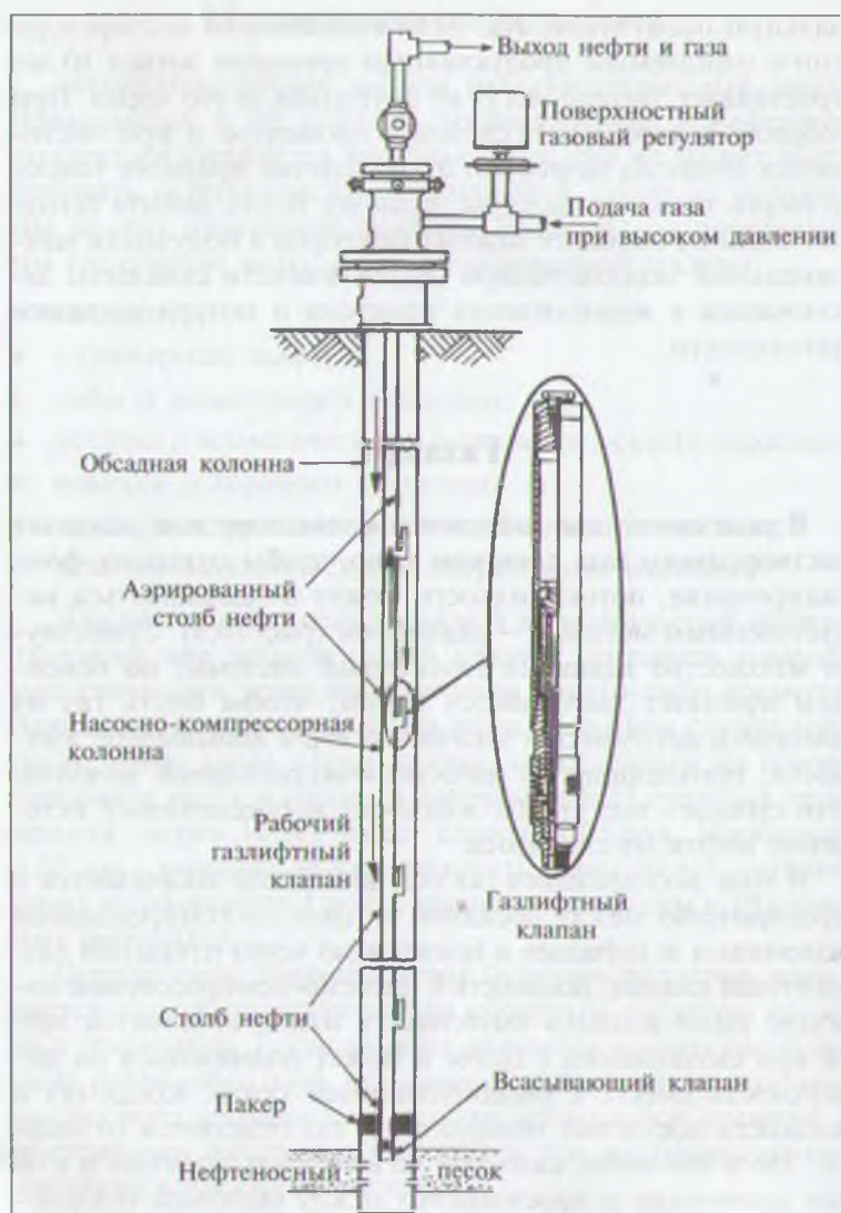
Рис. 10.3. Газлифтная установка. Газ закачивается в скважину в пространство между обсадной и насосно-компрессорной колоннами, проникает в насосно-компрессорную колонну через рабочий газлифтный клапан, там смешивается с нефтью и поднимает ее на поверхность
