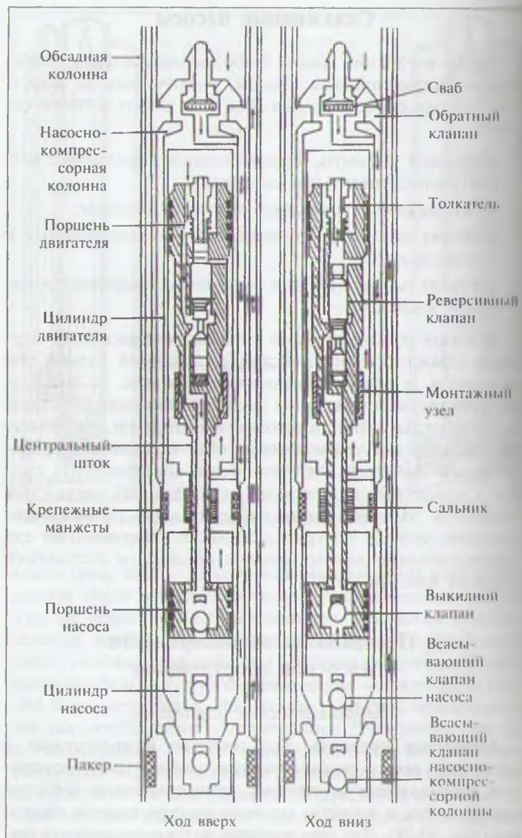
Рис. 10.26. Свободный гидравлический насос другого типа
