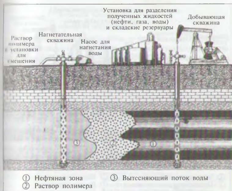
Рис. 14.3. Нагнетание раствора полимера (по оригинальным рисункам Joe R. Lindley, министерство энергетики США, представлено Национальным советом США по нефти)
