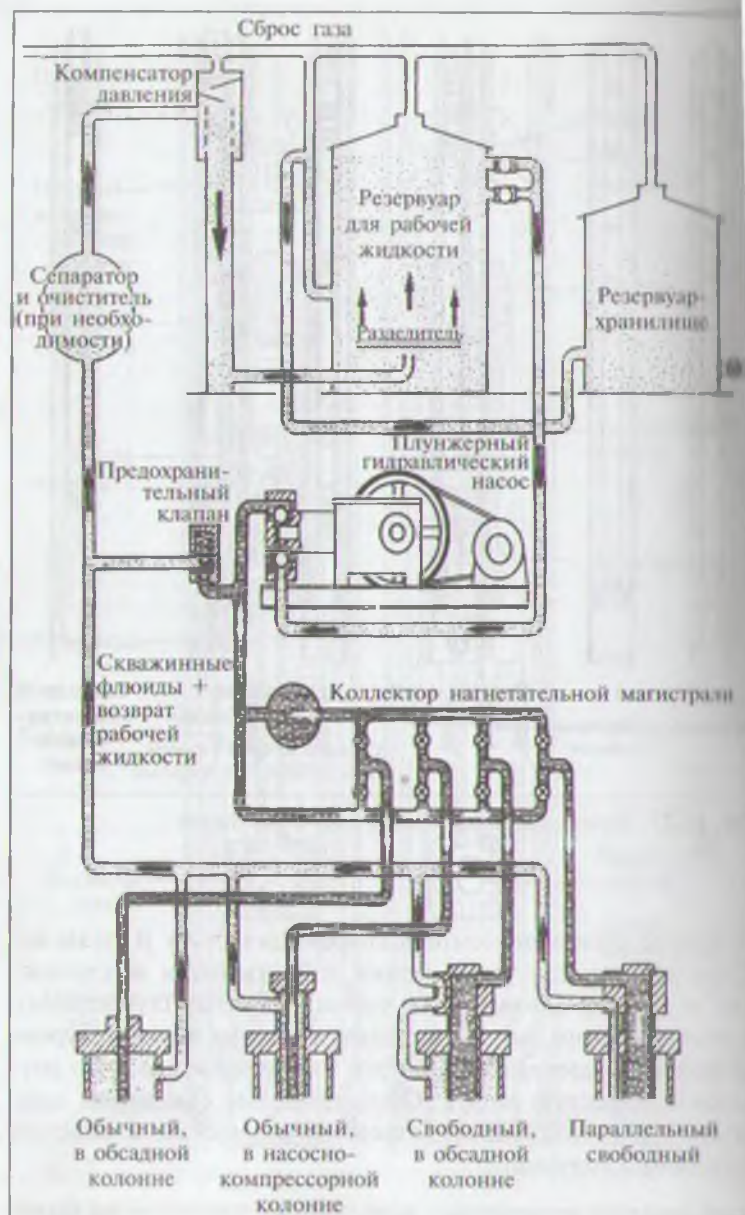
Рис. 10.28. Открытая гидравлическая система для перскачивания
