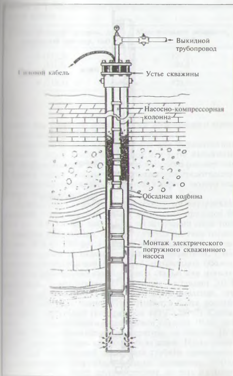
Рис. 10.32. Электрический погружной скважинный насос
