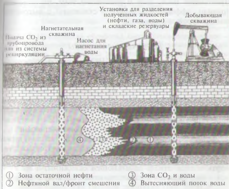
Рис. 14.5. Нагнетание \text{CO}_2 (по оригинальным рисункам Joe R. Lindley, министерство энергетики США, предоставлено Национальным советом США по нефти)
