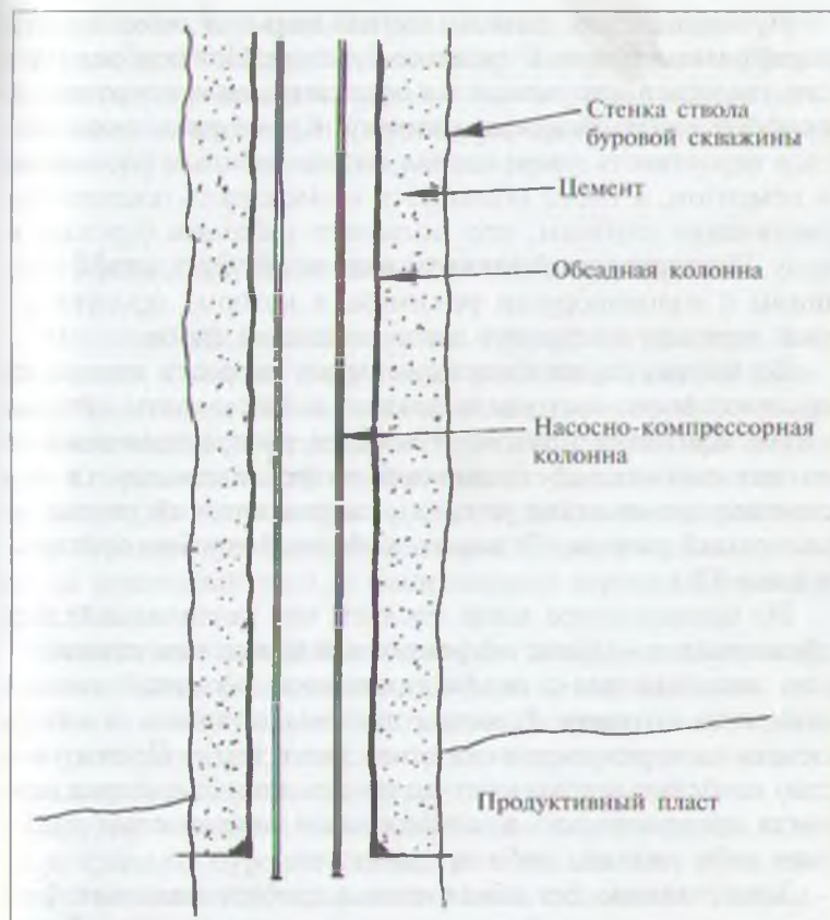
Рис. 7.5. Заканчивание скважины без спуска обсадной колонны в продуктивную зону
