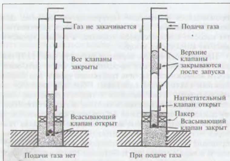
Рис. 10.7. Газлифт периодического действия
