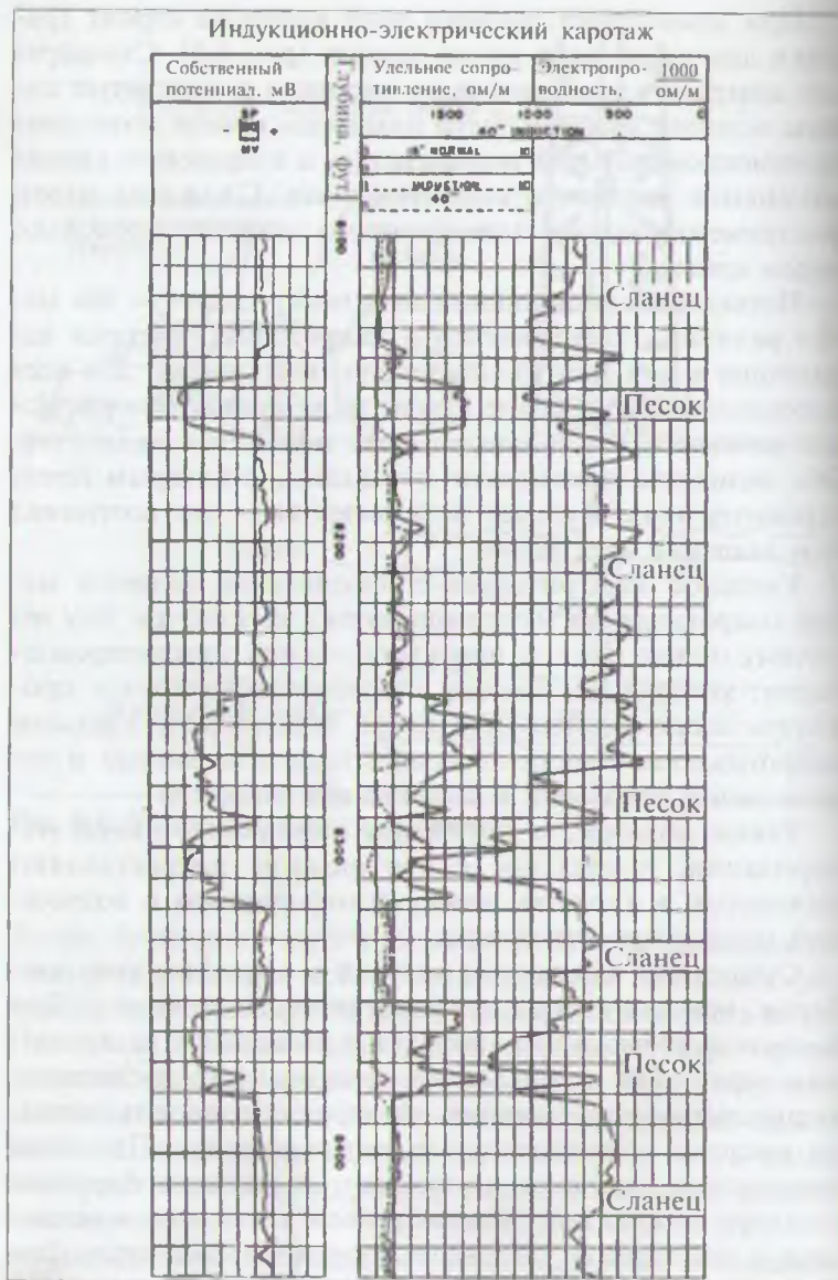
Рис. 6.5. Диаграмма электрического каротажа скважины. Левая кривая показывает изменение потенциала самопроизвольной поляризации, а правая — изменение удельного сопротивления
