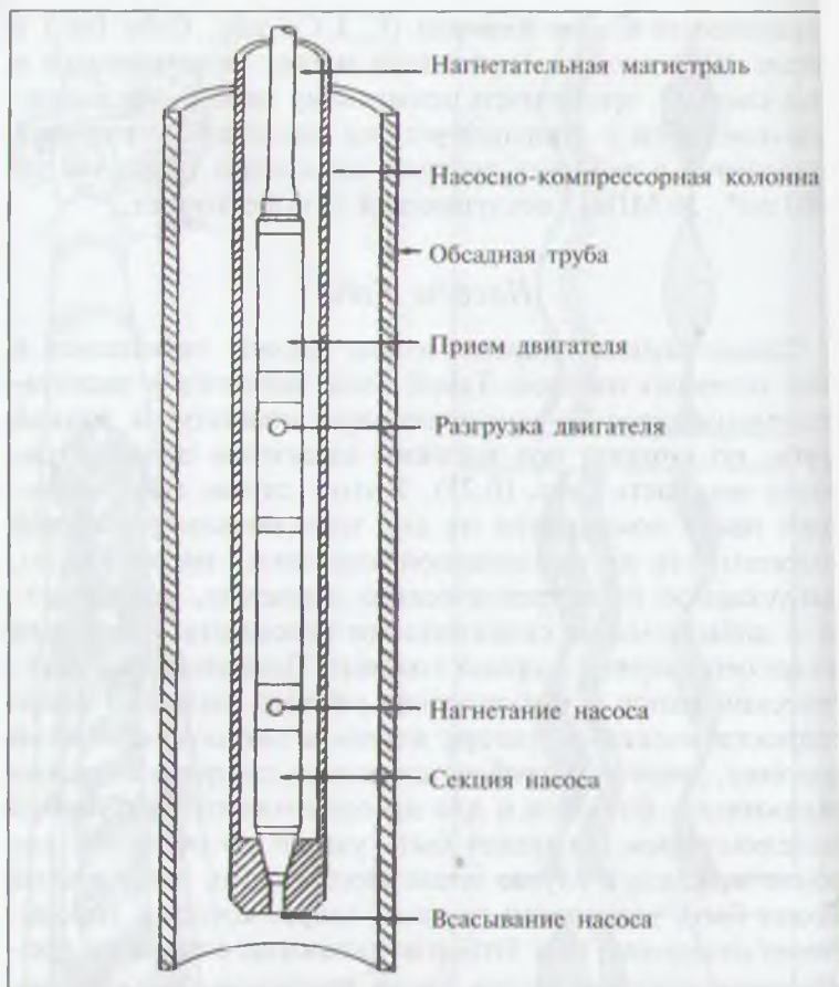
Рис. 10.23. Гидравлический насос вставного типа
