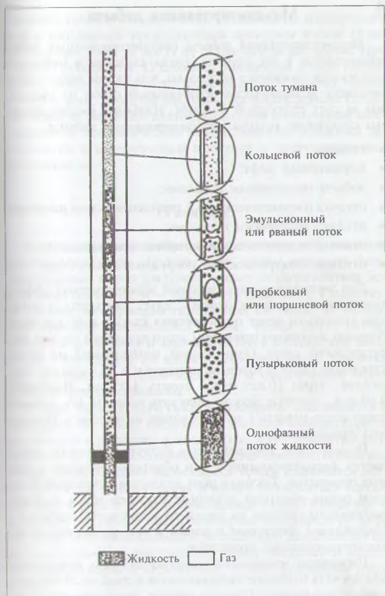
Рис. 10.2. Разделение жидкостей по мере протекания по насосно-компрессорной колонне
