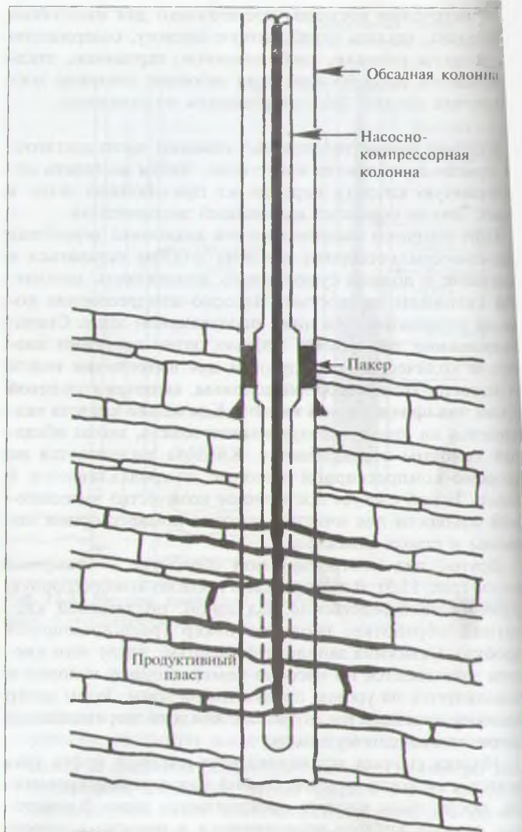
Рис. 13.3. Кислотная обработка скважины по пакерному способу
