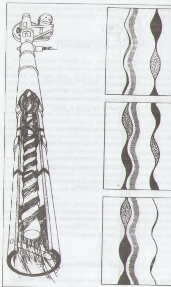
Рис. 10.22. Полостной насос
