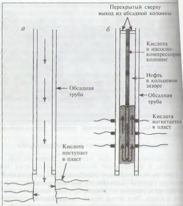
Рис. 13.2. Методы кислотной обработки: а — неконтролируемый; б — контролируемый
