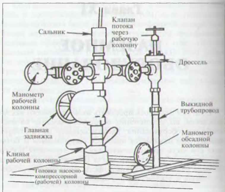
Рис. 11.1. Таким простым оборудованием оснащаются насосные скважины
