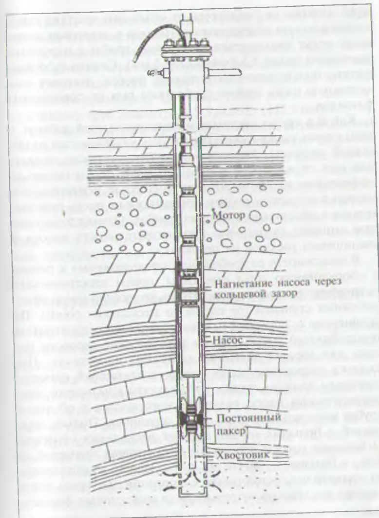
Рис. 10.36. Погружной насос с пакером
