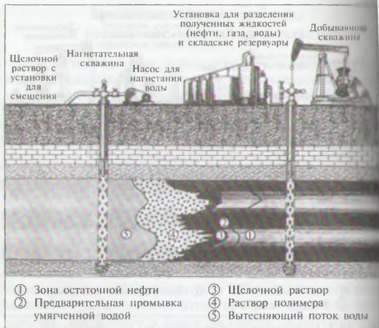
Рис. 14.4. Нагнетание щелочного раствора (по оригинальным рисункам Joe R. Lindley, министерство энергетики США, предоставлено Национальным советом США по нефти)
