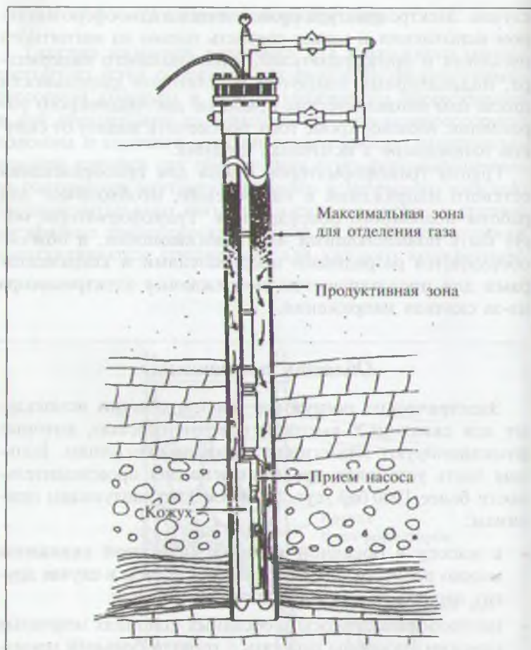
Рис. 10.35. Погружной насос в кожухе
