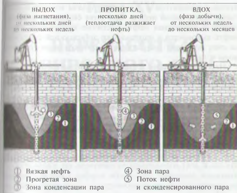
Рис. 14.6. Циклическая обработка паром (технология выдох—вдох) или паровая пропитка (по оригинальным рисункам Дж. R. Lindley, министерство энергетики США, предоставлено Национальным советом США по нефти)
