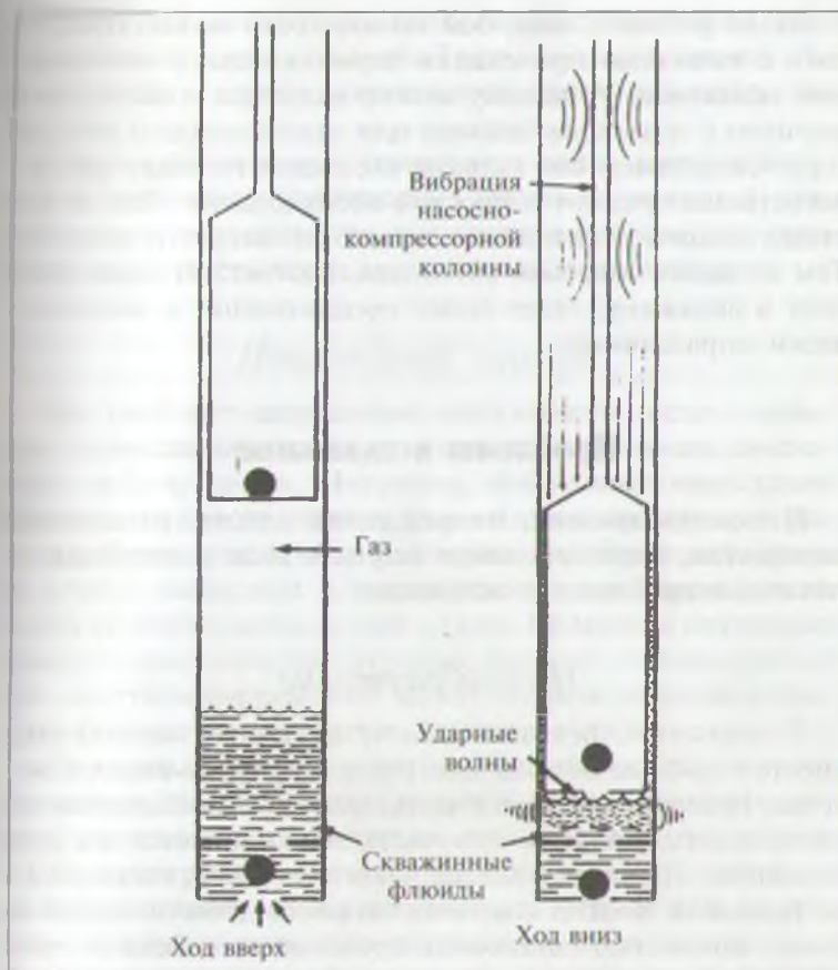
Рис. 12.3. Бой поршня по жидкости
