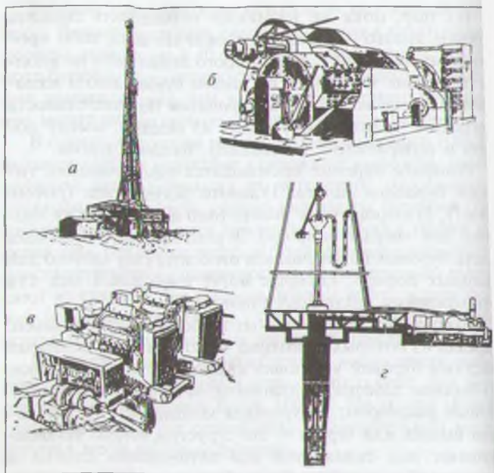
Рис. 5.4. Детали установки для роторного бурения: а — мачтовая вышка; б — буровые лебедки; в — двигатели системы промывки буровым раствором; г — система промывки буровым раствором и бурильная колонна
