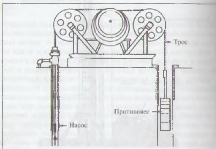
Рис. 10.20. Один из видов насосной установки с тросами
