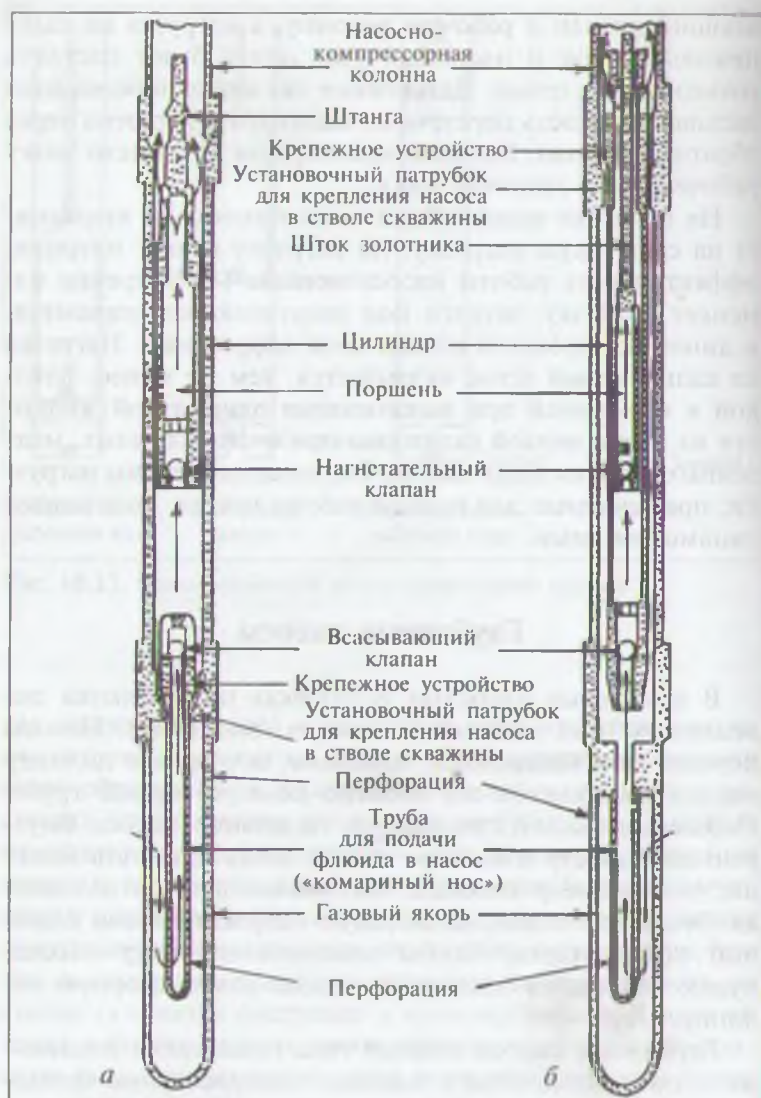
Рис. 10.14. Два типа насосов для штанговых насосных установок: a — трубный насос, б — стационарный цилиндр вставного типа с верхним креплением штока. Вставной насос и цилиндр можно извлечь из скважины, не поднимая насосно-компрессорную колонну
