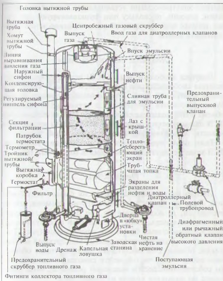
Рис. 11.4. Диаграмма потоков в вертикальной установке тепловой обработки
