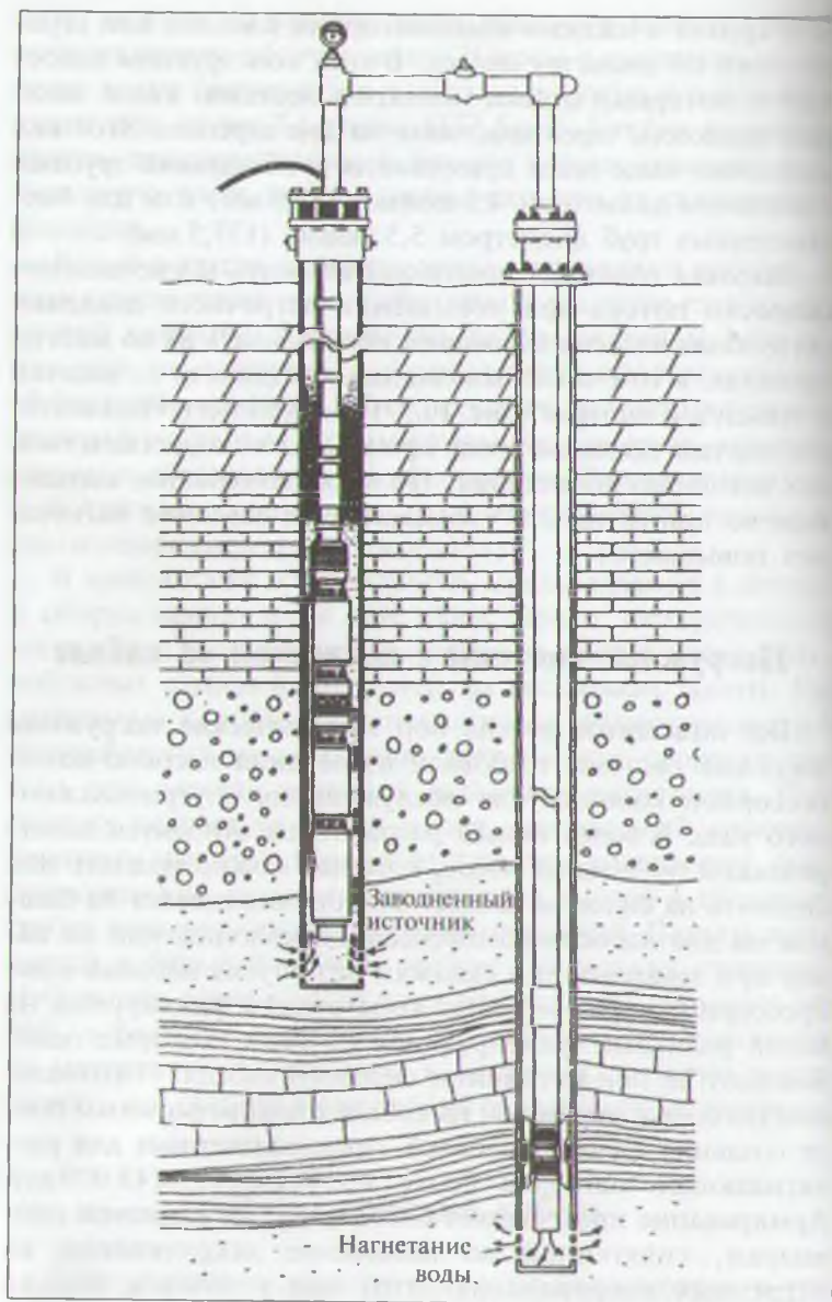
Рис. 10.37. Повышение нефтеотдачи посредством заводнения в замкнутой системе добычи—закачки
