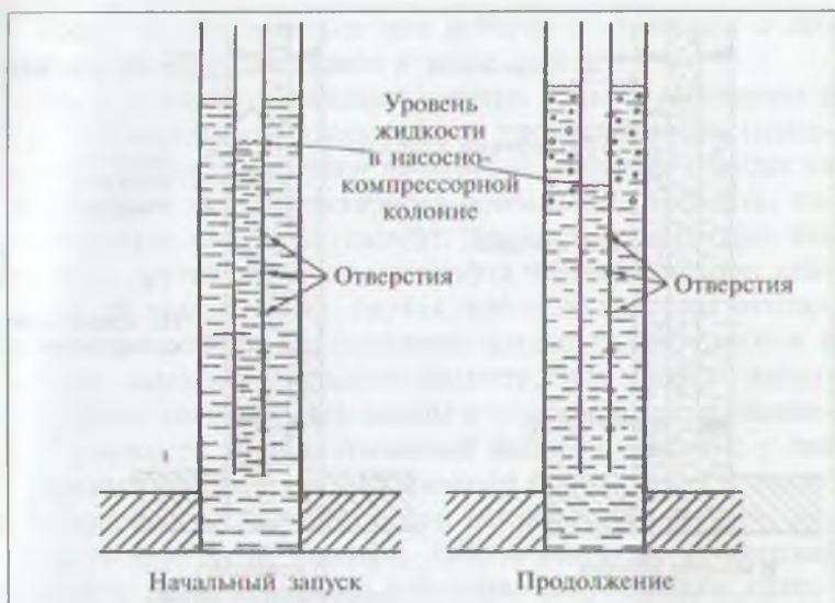
Рис. 10.5. Насосно-компрессорная колонна с отверстиями
