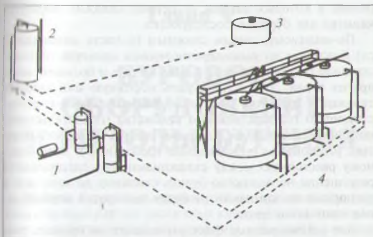
Рис. 4.6. Упрощенная схема монтажа наземного оборудования: 1 — сепараторы; 2 — нефтеочистители; 3 — емкость для утилизации; 4 — резервуары для товарной нефти
