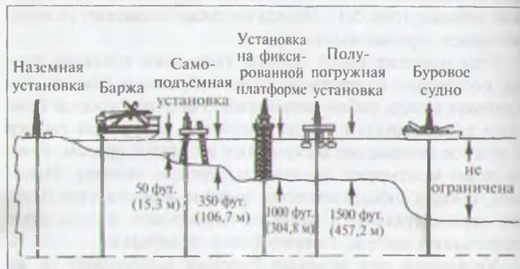
Рис. 5.2. Типы морских буровых установок
