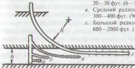
Рис. 16.2. Типы горизонтальных скважин (собственность Halliburton Energy Services)
