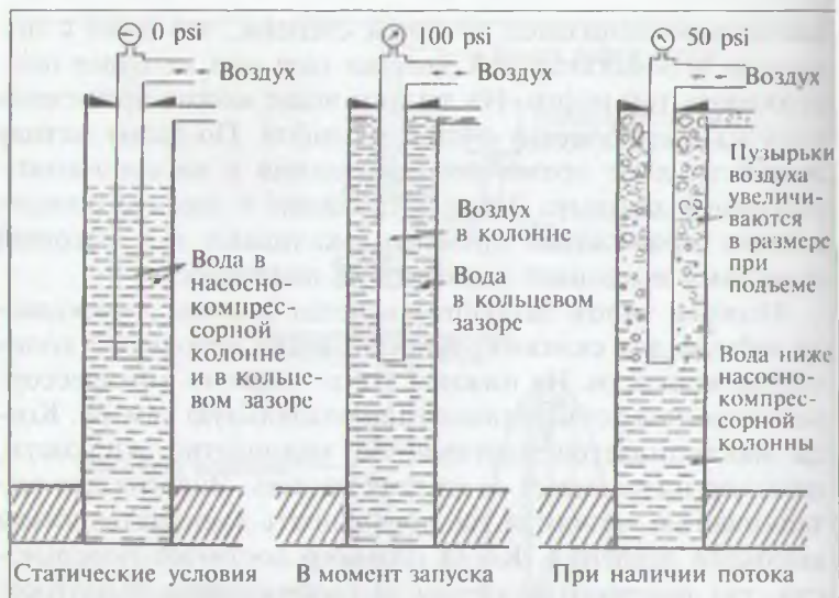
Рис. 10.4. Газлифт с использованием колонны с открытым концом в водяной скважине
