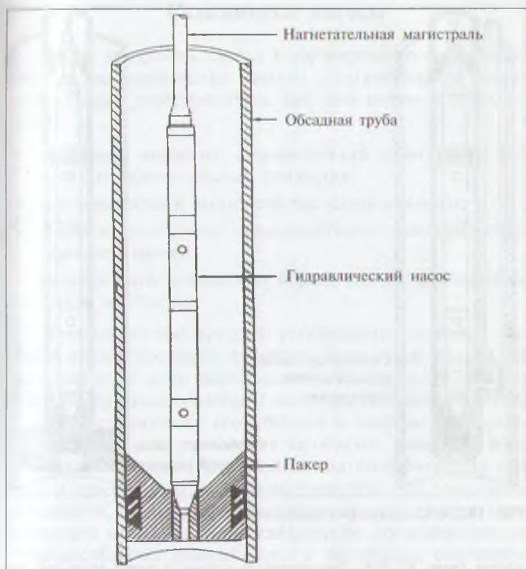
Рис. 10.24. Гидравлический насос в обсадной колонне
