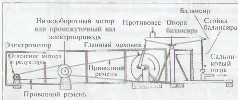
Рис. 10.15. Старинная качалка
