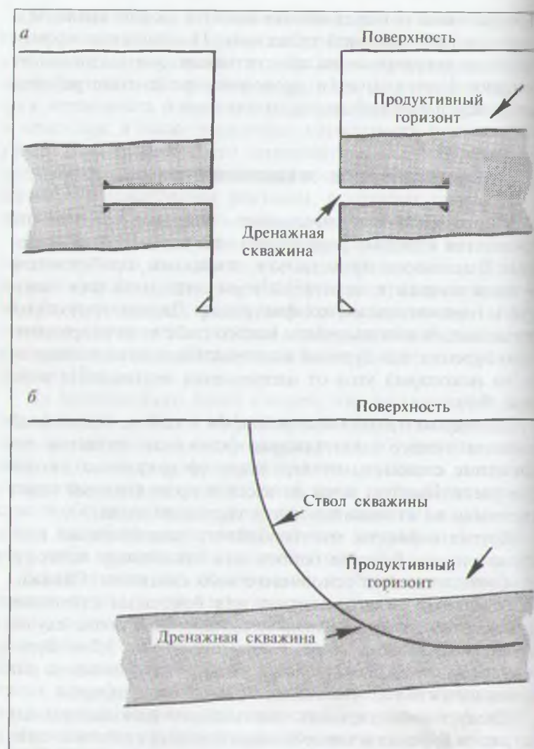
Рис. 7.6. Два типа многозабойного заканчивания скважины: а — бурение в пласт происходит в горизонтальном направлении при вертикальном стволе скважины; б — бурение ведется под углом, так чтобы проникновение в пласт оказалось горизонтальным. В результате увеличивается срок продуктивности данного горизонта, т.е. в целом продуктивность повышается
