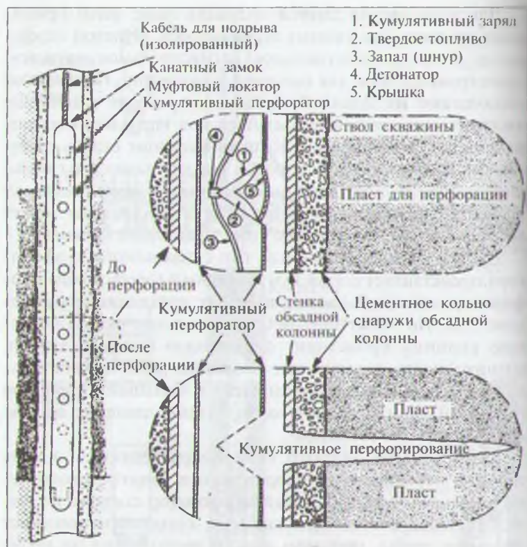
Рис. 7.2. Схема процесса кумулятивного перфорирования
