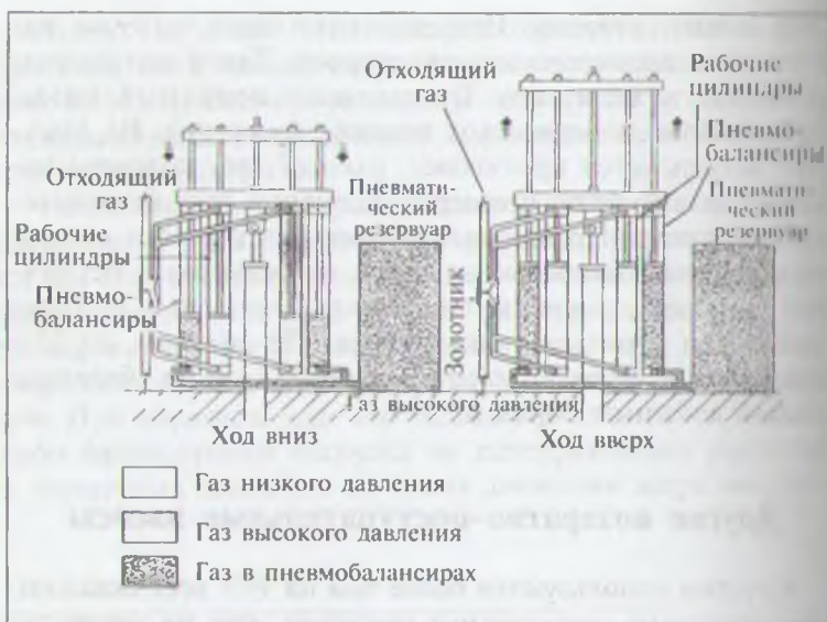
Рис. 10.18. Пневматический штанговый насос
