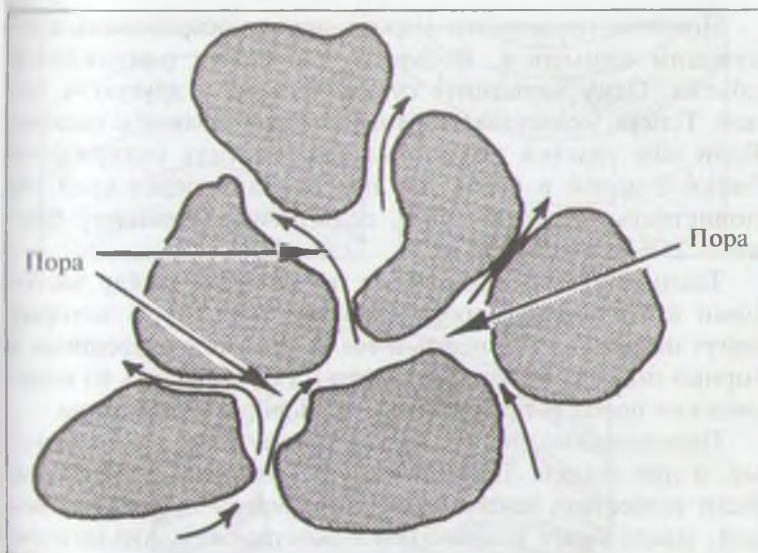
Рис. 3.3. Нефть собирается в пустотах или порах в горной породе и проходит через крошечные трещины и каналы. Это называется пористостью
