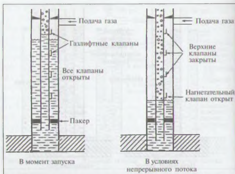
Рис. 10.6. Схема монтажа газлифтных клапанов
