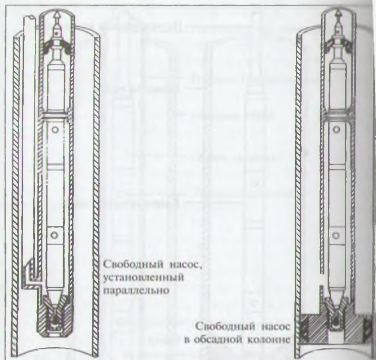
Рис. 10.25. Свободный гидравлический насос
