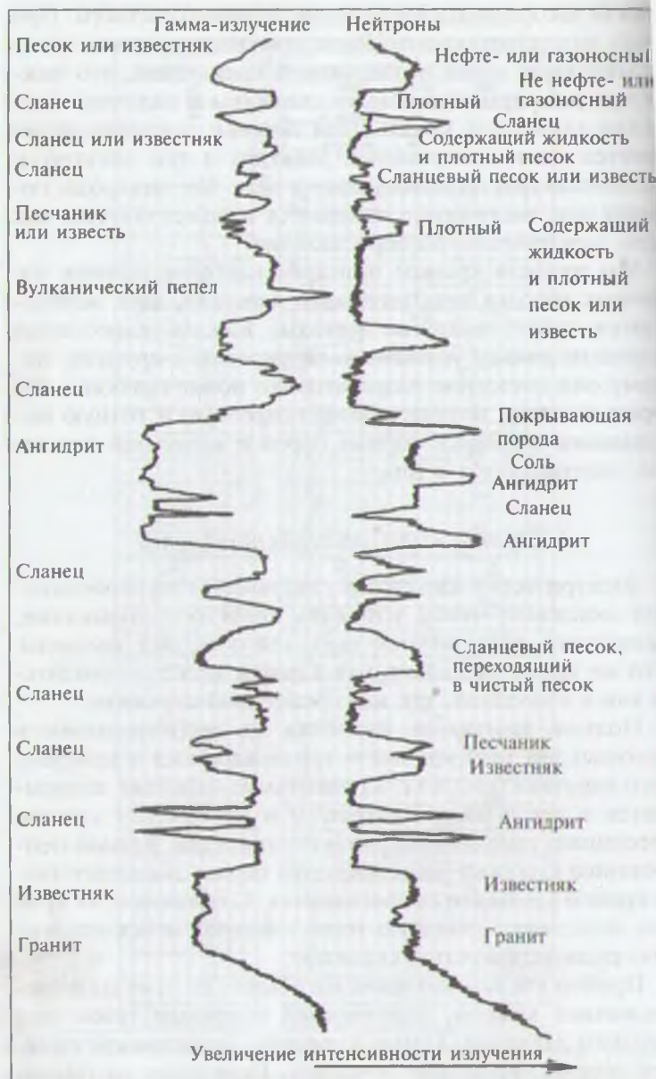
Рис. 6.6. Каротажная диаграмма по радиоактивности
