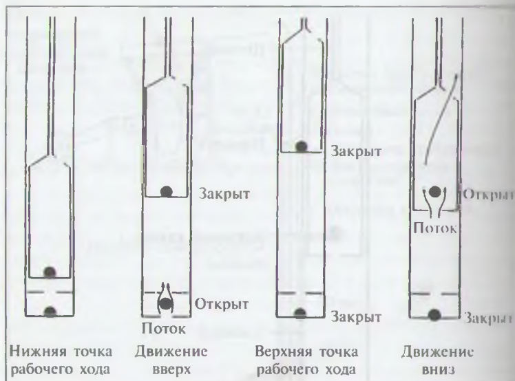
Рис. 10.13. Схема рабочего цикла штангового насоса
