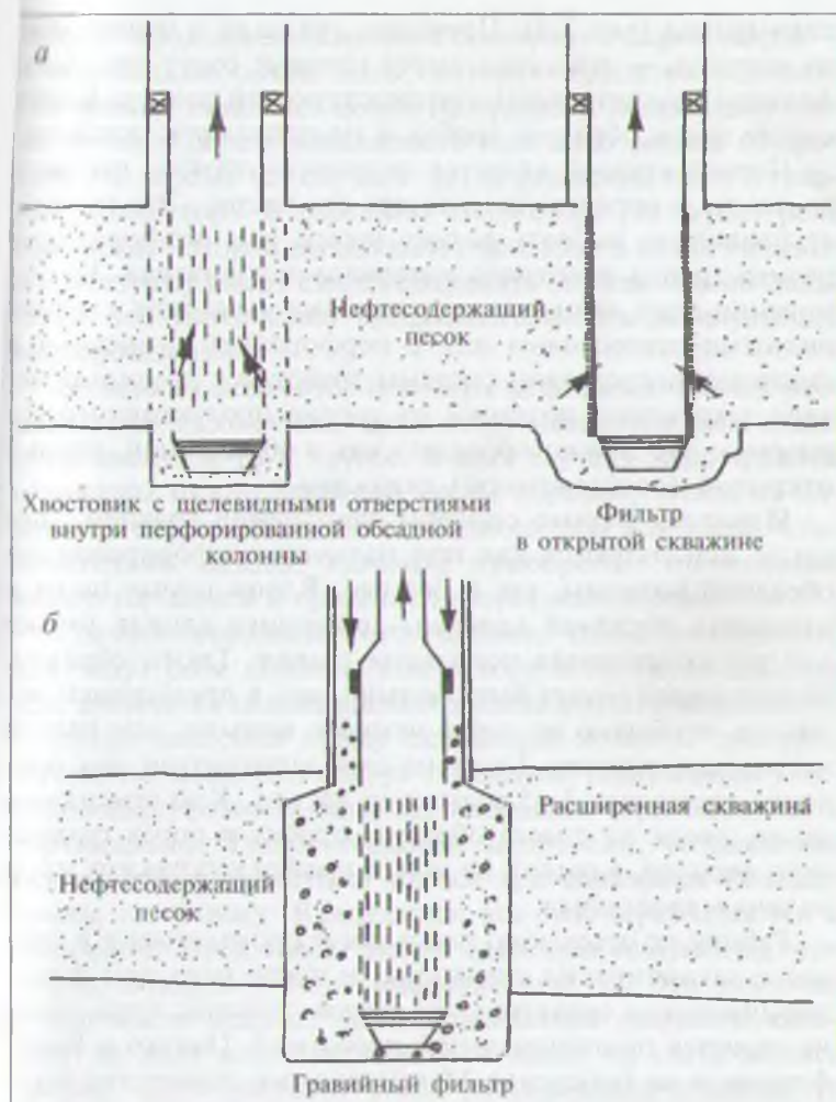
Рис. 7.4. Два метода борьбы с песком: а — применение хвостовиков; б — заполнение гравием
