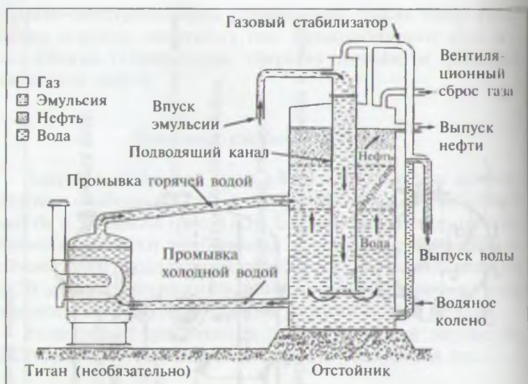
Рис. 11.6. Схематическое изображение промывочного бака или отстойника
