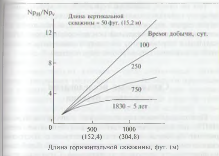
Рис. 16.3. Сравнение добычи из горизонтальных и вертикальной скважин (собственность Halliburton) (Отношение объемов добычи нефти из вертикальной и горизонтальных скважин в течение разных периодов времени и при разной длине горизонтальных скважин.)
