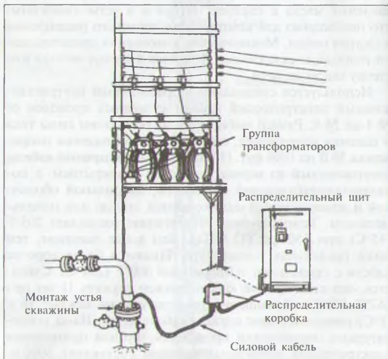
Рис. 10.34. Наземное оборудование для погружного электронасоса
