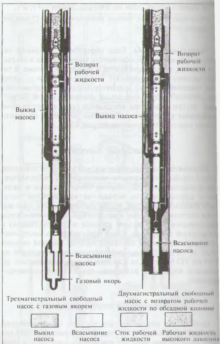
Рис. 10.29. Внутрискважинные гидравлические насосные установки с замкнутыми гидравлическими системами
