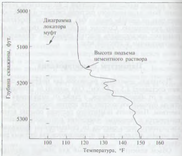
Рис. 8.6. Температурный график высоты подъема цементного раствора
