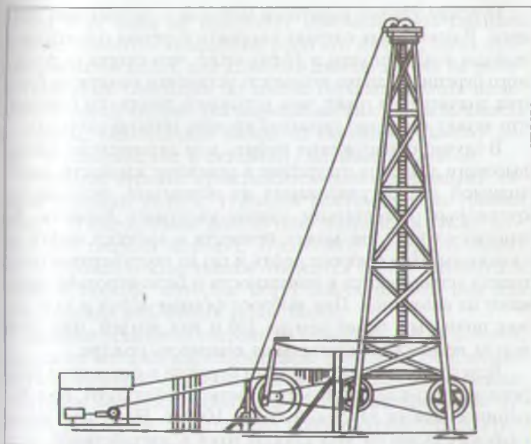
Рис. 5.3. Схема станка канатного бурения
