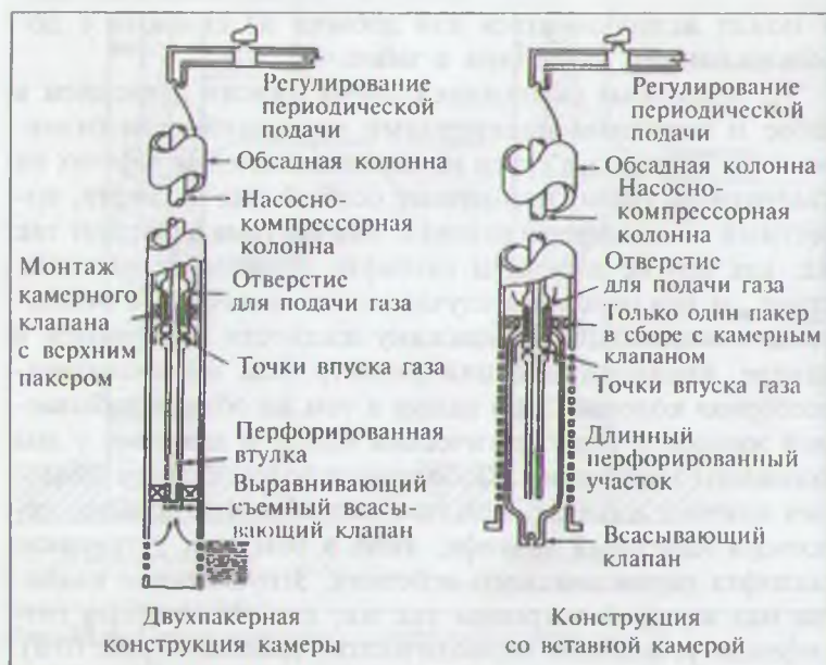
Рис. 10.8. Два вида камерного газлифта
