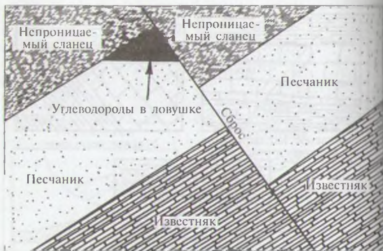
Рис. 3.7. Комбинированная ловушка. Углеводороды накапливаются по структурному механизму в результате наличия сброса и по стратиграфическому за счет непроницаемого слоя сланцевой породы
