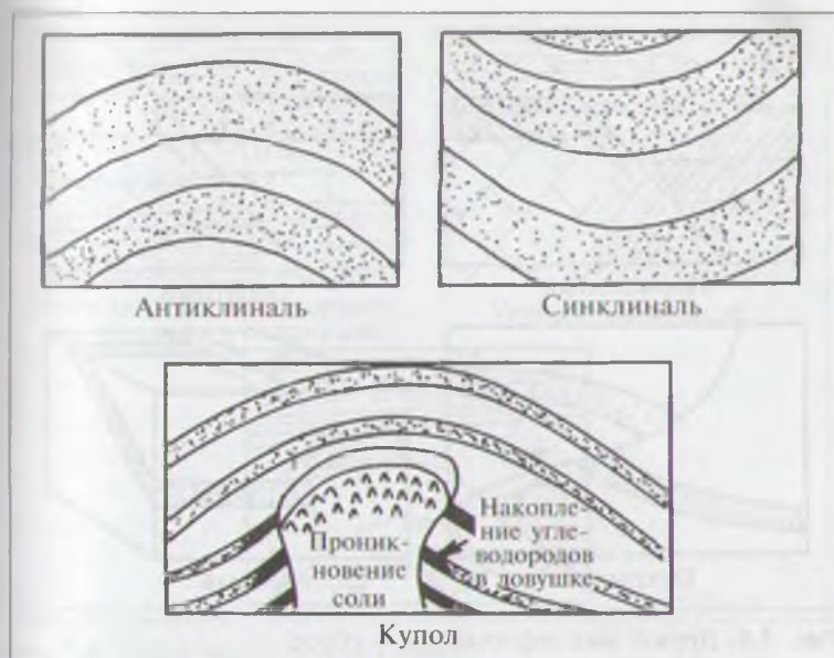
Рис. 3.4. Некоторые типичные виды складок
