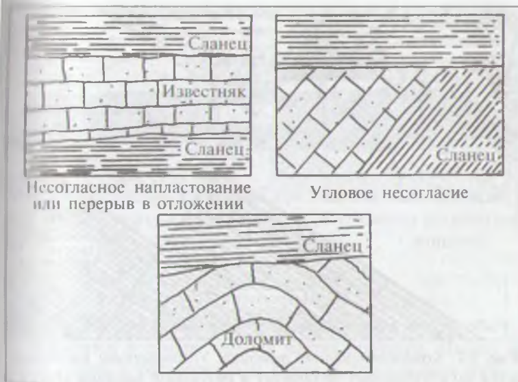
Рис. 3.6. Несогласное напластование
