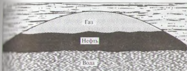
Рис. 3.8. Газ, нефть и вода в коллекторе стремятся разделиться в соответствии с величиной их плотности
