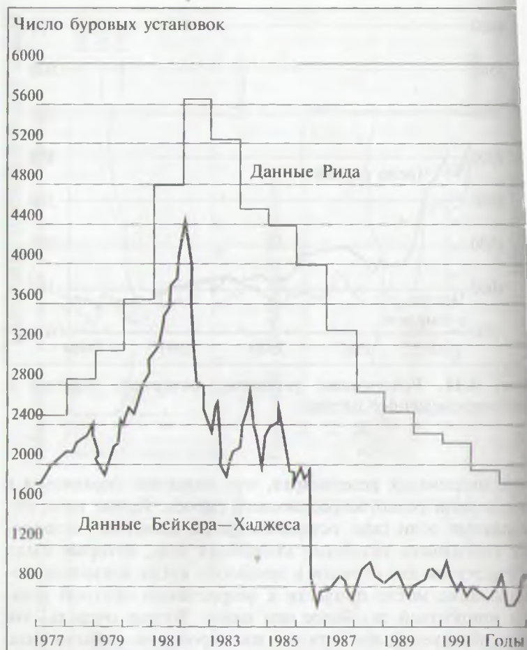
Рис. 1.12. Число буровых установок в США
