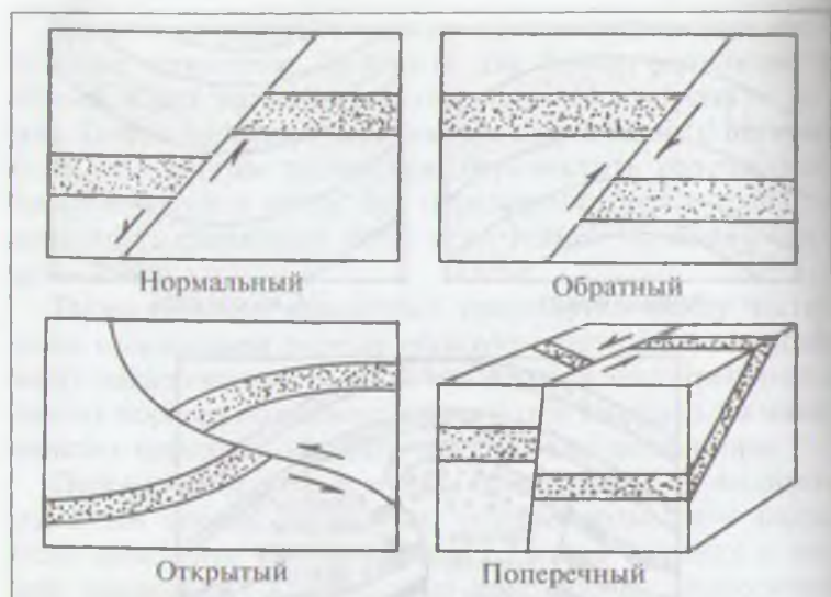
Рис. 3.5. Другой вид деформаций — сброс
