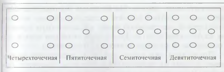
Рис. 4.4. Некоторые типовые схемы размещения скважин
