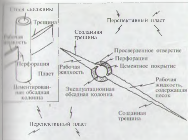
Рис. 13.4. Принцип гидро разрыва
