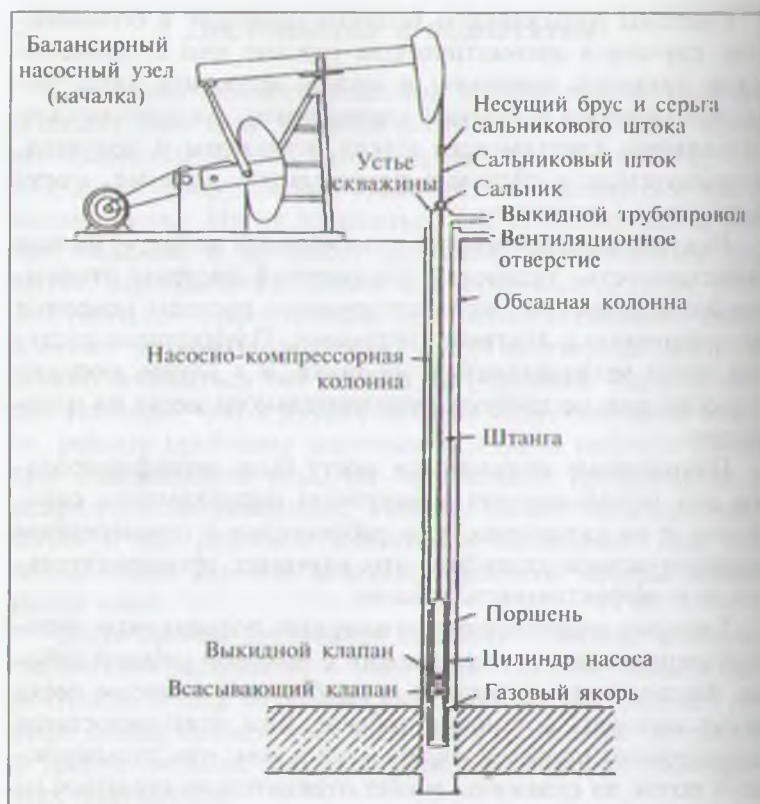
Рис. 10.11. Основные части штанговой насосной системы
