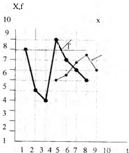
2.7 - rasm. O'rtacha harakatlanuvchi usul bo'yicha vaqt qatorlari va bashorat grafigi
