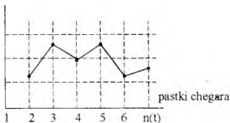
3.8-rasm. Tarqoqlik grafigi
