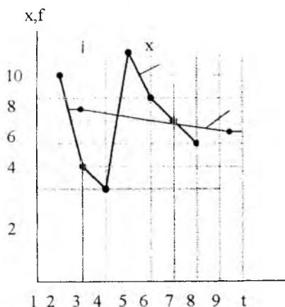
2.11 - rasm. Trendlarni namoyish qilish usuli bo'yicha vaqt qatorlari ( x ) va bashorat ( f )
