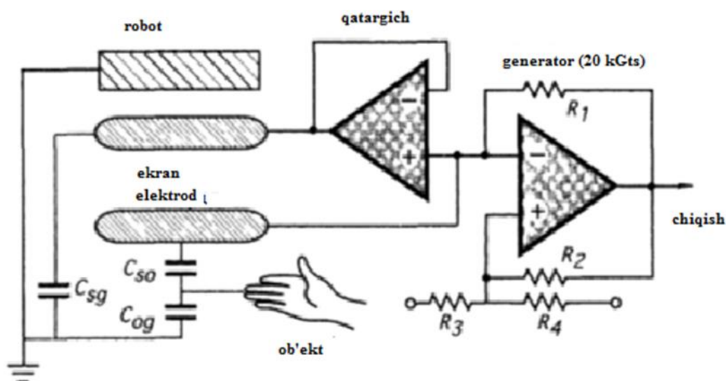
5.7 -rasm. Kirish sig'imlari bilan boshqariladigan chastota modulyatorining soddalashtirilgan sxemasi
