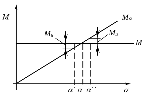
1.7- rasm. Asbob qo'zg'aluvchan qismining turg'un burilish holati
