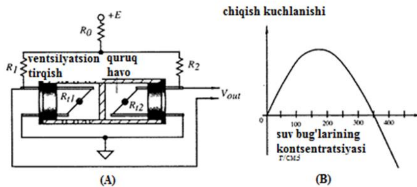
5.31- rasm. O‘z-o‘zidan qiziydigan termistorlarga ega bo‘lgan absolyut namlik datchigi. A – sxemasi va ulanishi. B – chiqish kuchlanishining namlikka bog‘lanishi
