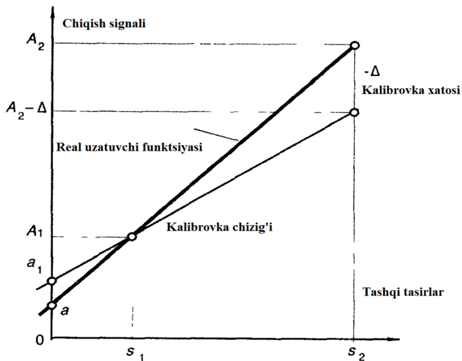
3.3.-rasm. Kalibrlash xatoligi
