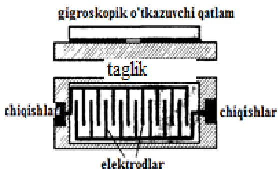
5.30- rasm. Gigristorning sxemasi
