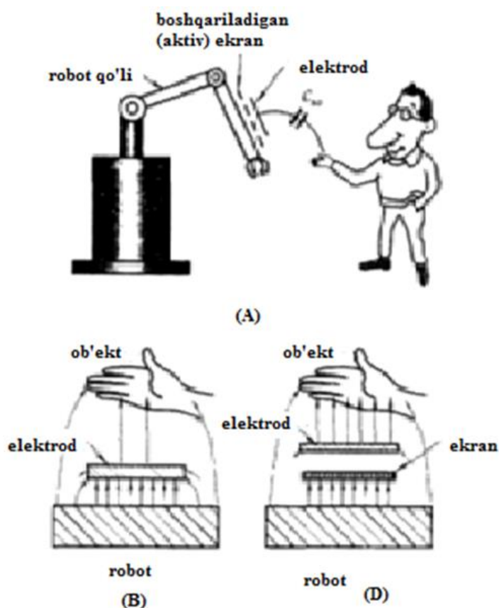
5.6- rasm. Sig'imli yaqinlashish datchigi: (A)-boshqariladigan ekran erga ulangan robotning metall qo'lida joylashgan; (B)- ekran bo'lmaganda elektr maydoni asosan elektrod bilan robot o'rtasida; (D)-ekran maydonni elektrod bilan obyekt o'rtasidagi sohaga yo'naltirilgan
