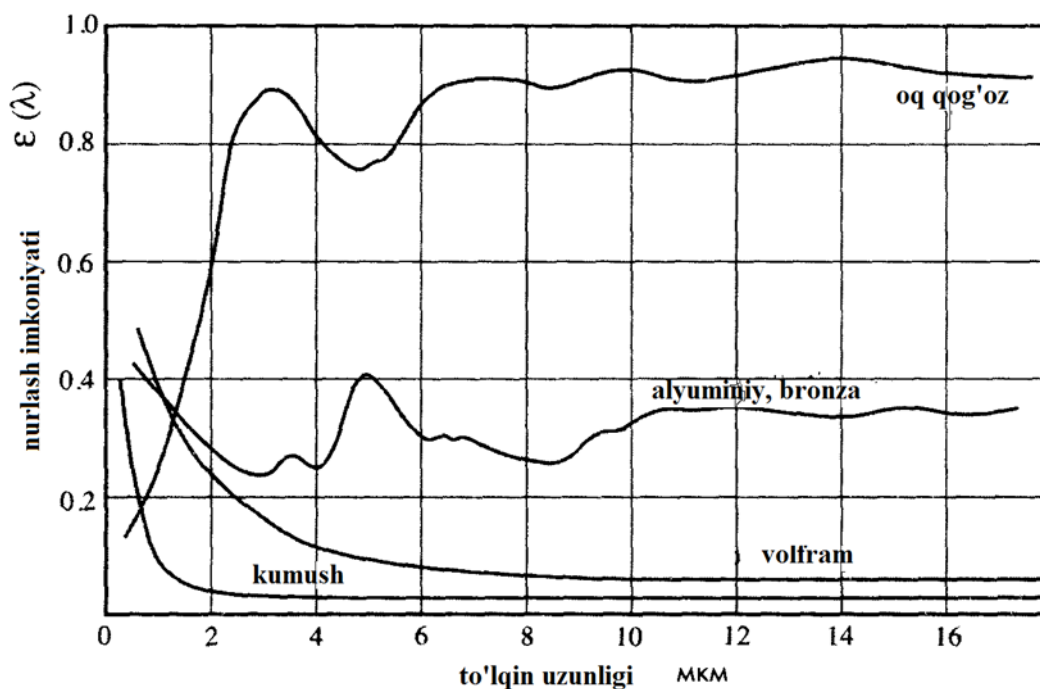
4.30- rasm. Nurlatish qobiliyatining to'lqin uzunligiga bog'lanishi
