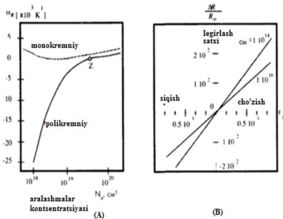
4.37- rasm. Harorat koeffitsiyentining legiraydigan aralashmalarning konsentratsiyasiga bog'liqligi (A), kremniyning pyezorezistiv sezgirligi (B)
