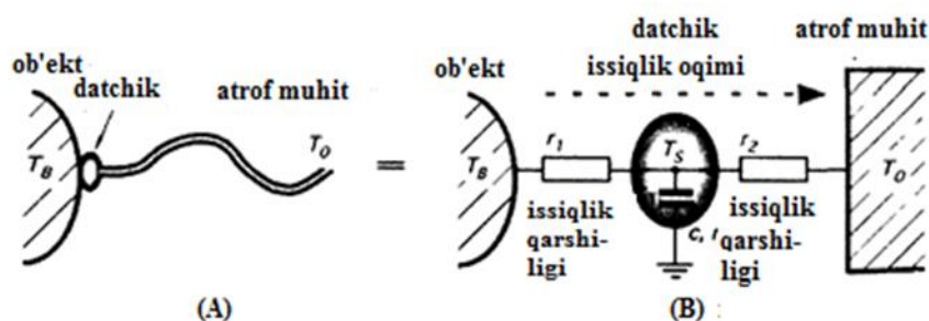
5.13- rasm. Harorat datchigi; (A)- obyekt, tutashtiruvchi kabel bilan issiqlik kontaktida; (B)-ekvivalent issiqlik sxemasi
