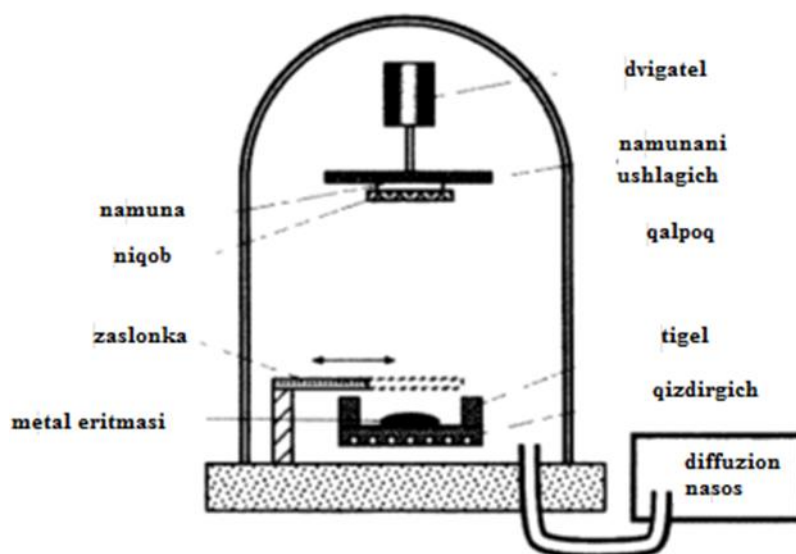
4.39- rasm. Vakuum kamerada yupqa metall plenkani qoplash
