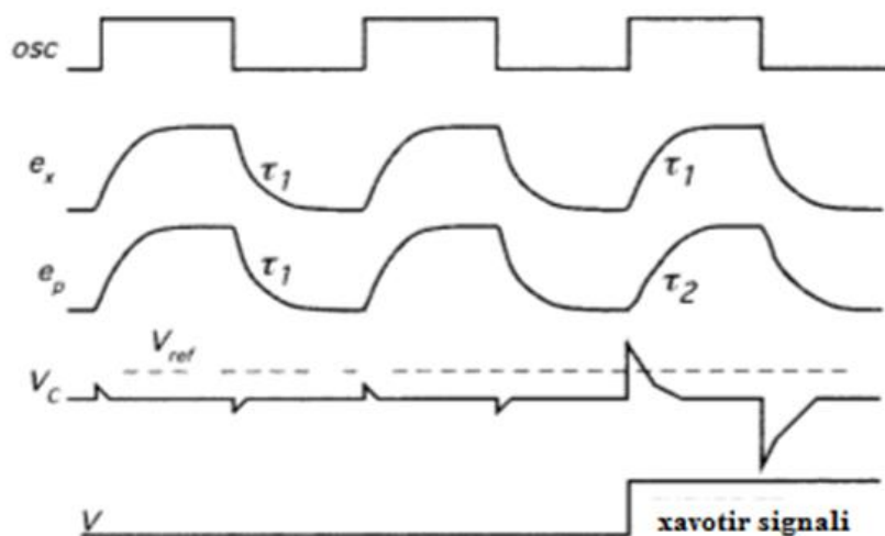
5.4 -rasm. Avtomobilni qo'riqlash uchun sig'imli detektor
