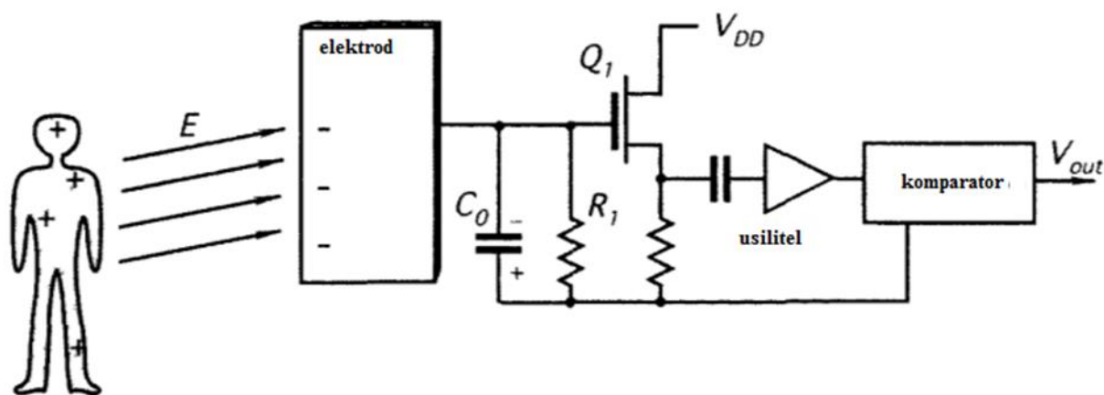
5.8- rasm. Bir qutbli elektrostatik harakat detektori
