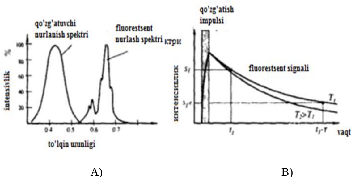
5.15- rasm. Haroratni fluorescent o'lchash uslubi: A – qo'zg'atuvchi va fluorescent nurlatishlarning spektral tavsiflari; B – T_1 va T_2 haroratlar uchun shu'laning eksponensial qonun bo'yicha pasayishi; e – natural logarifmning asosi; t – pasayish tavsifining vaqt doimiysi
