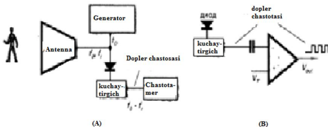
5.1- rasm. O'YuCh mavjud bo'lish detektor: A – Dopler chastotasini o'lchash uchun sxema; B – ostona detektoriga ega bo'lgan sxema
