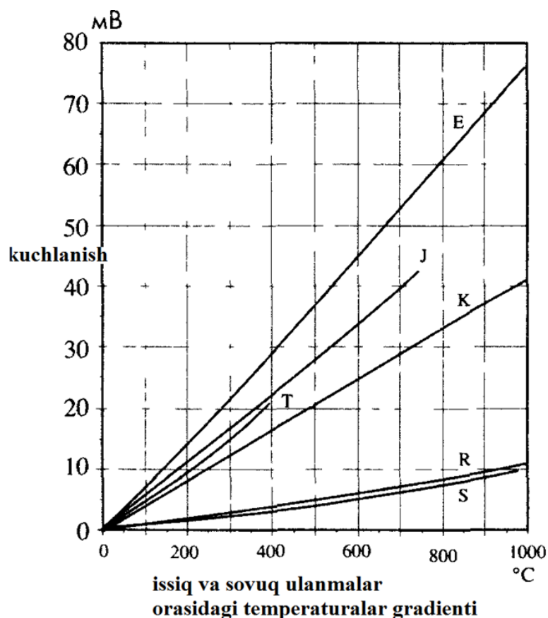
4.21- rasm. Standart termojuftliklarda chiqish kuchlanishining sovuqlik va issiqlik kavsharlar o'rtasidagi haroratlar gradientiga bog'lanishi
