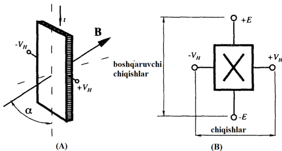
4.17- rasm. A – Xoll datchigining chiqish signali magnit maydonining vektori bilan plastinka tekisligi o‘rtasidagi burchakka bog‘liqligi, B – Xoll datchigining to‘rtta chiqishi
