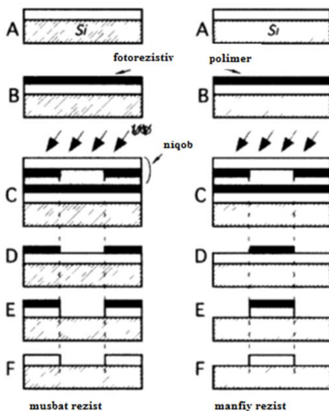
4.42- rasm. Musbat va manfiy fotolitografiya
