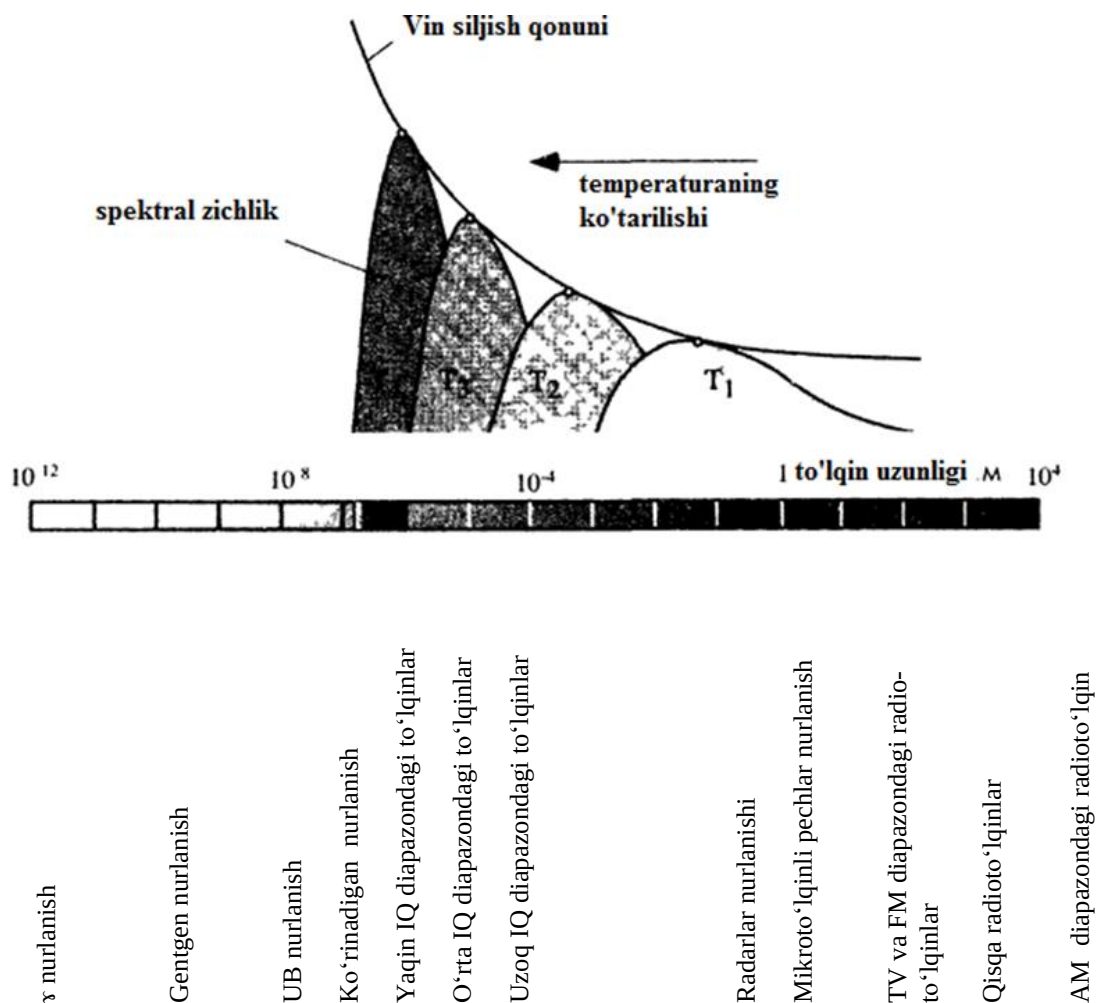
4.27- rasm. Elektromagnitik nurlanish spektri
