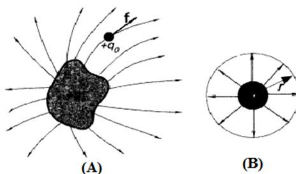
4.1- rasm. A - musbat test zaryadi zaryadlangan obyektning atrofiga kiritilgan; B – sferik obyektning elektr maydoni
