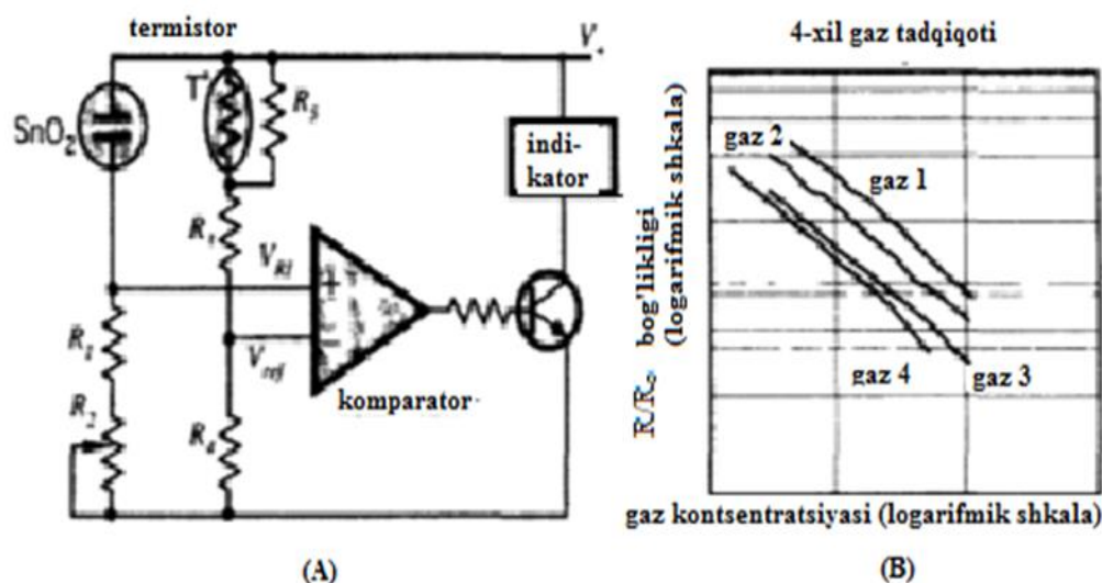
5.37- rasm. Uytston ko'prigiga kiritilgan metall-oksidli kimyoviy detektor (A) va uning turli gazlar uchun qurilgan uzatish tavsiflari (B)
