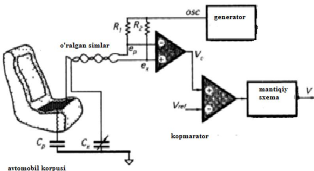
5.4 -rasm. Avtomobilni qo'riqlash uchun sig'imli detektor
