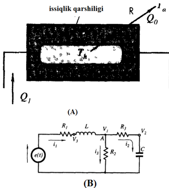
4.35- rasm. A – isitadigan elementning issiqlik modeli, B – rezistiv, sig'imli va induktiv elementlarga ega bo'lgan elektr sxemasi
