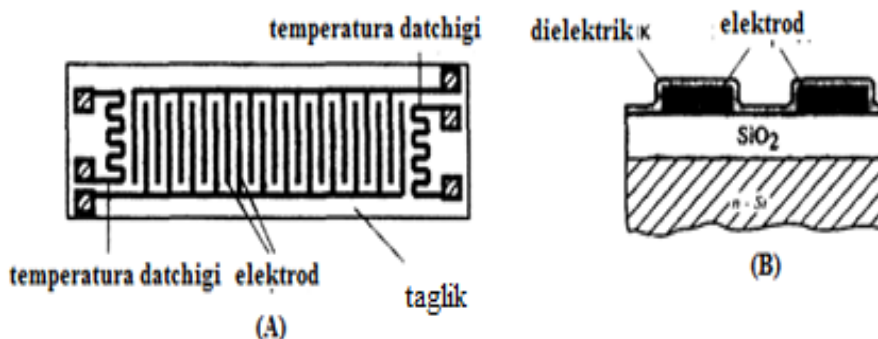
5.28- rasm. Sig'imli yupqa plyonkali namlik datchigi. A – kondensatorning plastinkalarini shakllantiradigan taroqsimon elektrodlar; B – datchikning ko'ndalang kesimi
