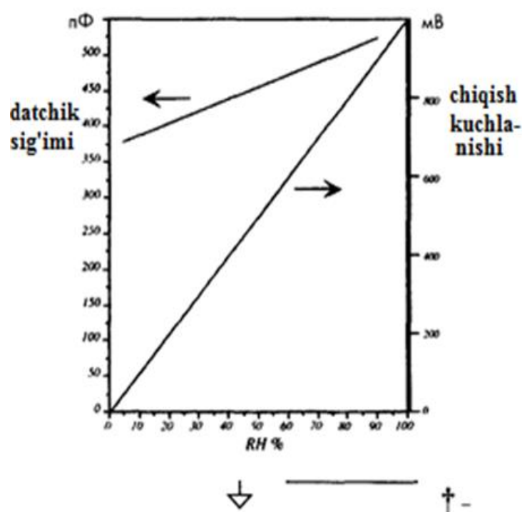
5.26- rasm. Sig'imli datchik va tizimning uzatish funksiyasi
