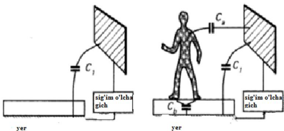
5.3-rasm. Odam detektorning sxemasiga qoʻshimcha sigʻimni olib kirishi
