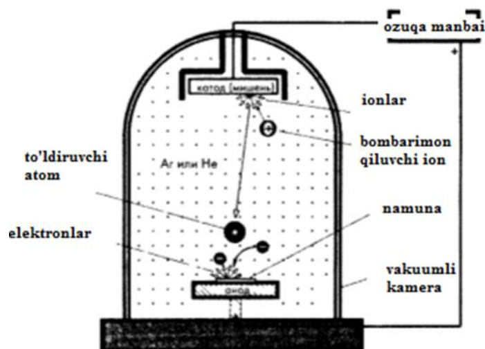
4.10- rasm. Vakuum kamerada ionli changlash
