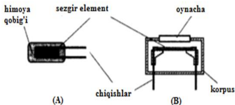
5.14- rasm. Harorat datchiklarining asosiy strukturalari: A – kontaktli datchik; B- kontaktsiz datchik (issiqlik nurlanishi detektor)
