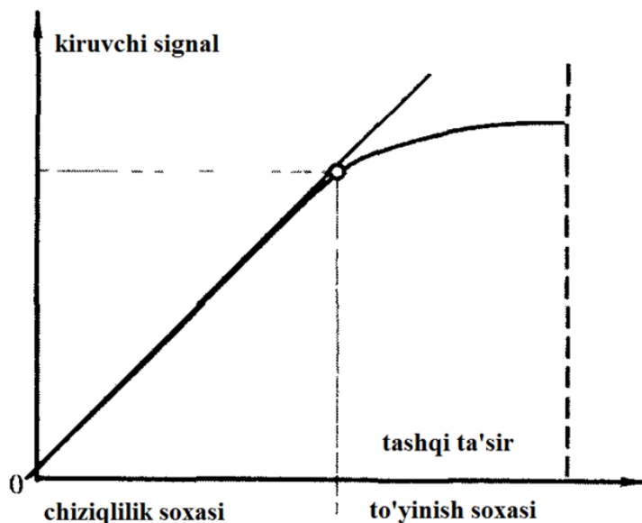
3.6.- rasm. To‘yinishga ega bo‘lgan uzatish funksiyasi
