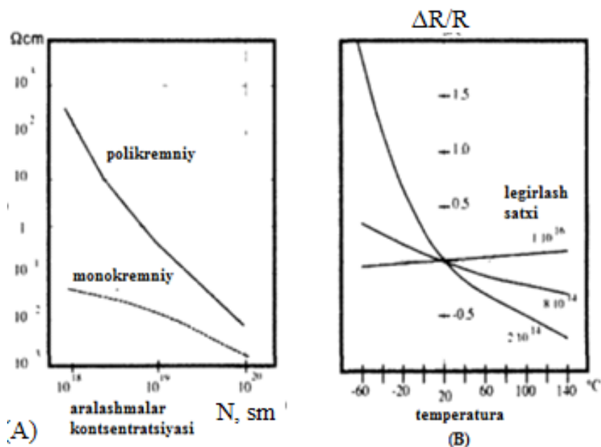
4.36- rasm. Bor bilan legirlangan kremniyning solishtirma qarshiligi (A); legiraydigan aralashmalarning turli konsentratsiyalari uchun kremniy qarshiligining harorat koeffitsiyenti (B)
