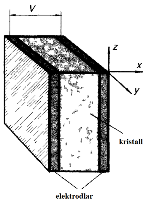
4.8 -rasm. Qutblangan kristallga kiritilgan elektrodlar yordamida shallantirilgan pyezoelektrik datchik
