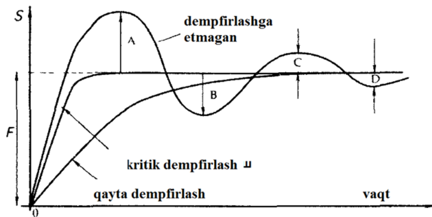
3.10-rasm. Turlicha dempirlash koeffitsiyentlariga ega bo‘lgan datchiklarda chiqish signallarining turlari
