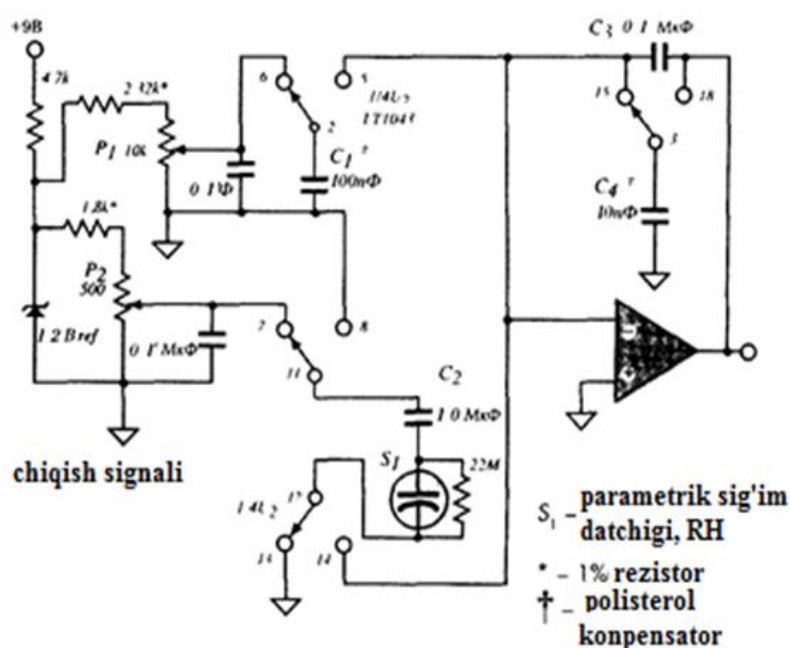
5.25- rasm. Sig'imli datchik yordamida namlikni o'lchashning soddalashtirilgan sxemasi
