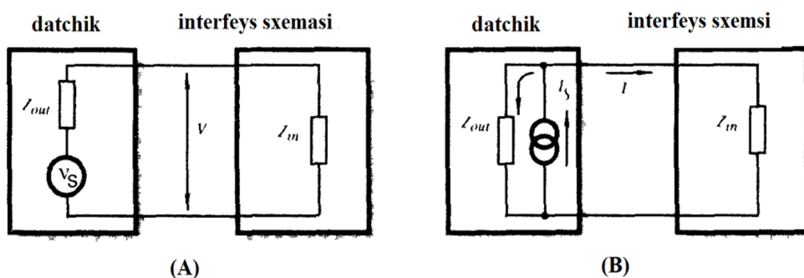
3.8-rasm. Datchikning interfeys sxemasi bilan ulanishi. A – kuchlanish ko'rinishidagi chiqish signaliga ega bo'lgan datchik, B – tokli chiqish signaliga ega bo'lgan datchik
