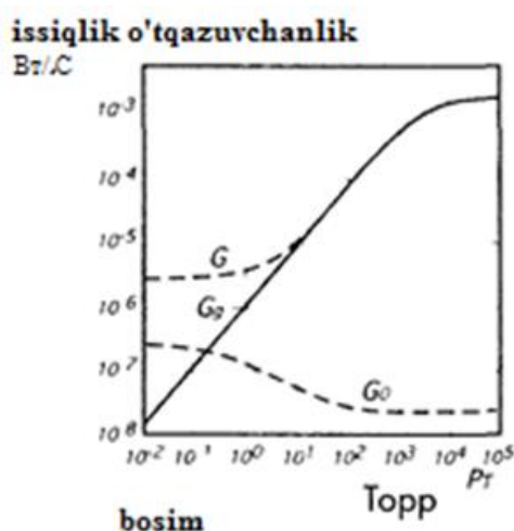
5.19- rasm. Qizdiriladigan plastinkaning issiqlik yo'qotishlari
