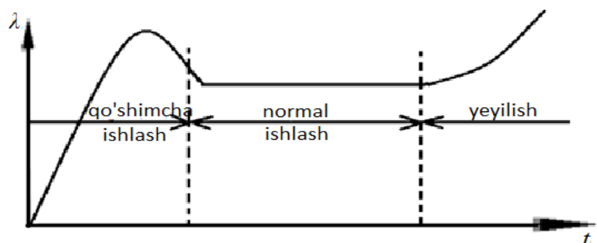
6.8-rasm. Buzilishlar intensivligi bilan ish vaqti orasidagi bogʻlanish
