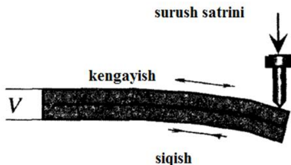
4.10- rasm. Ikki qatlamli pyezoelektrik datchik
