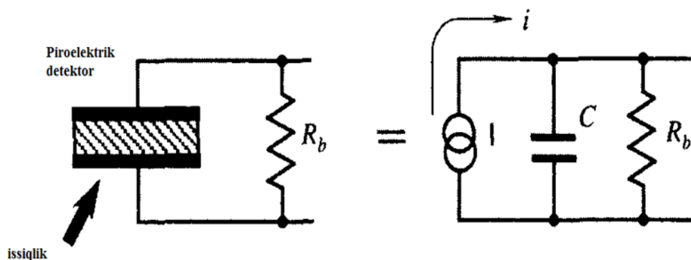
4.13- rasm. Piroelektrik detektor va uning ekvivalent sxemasi
