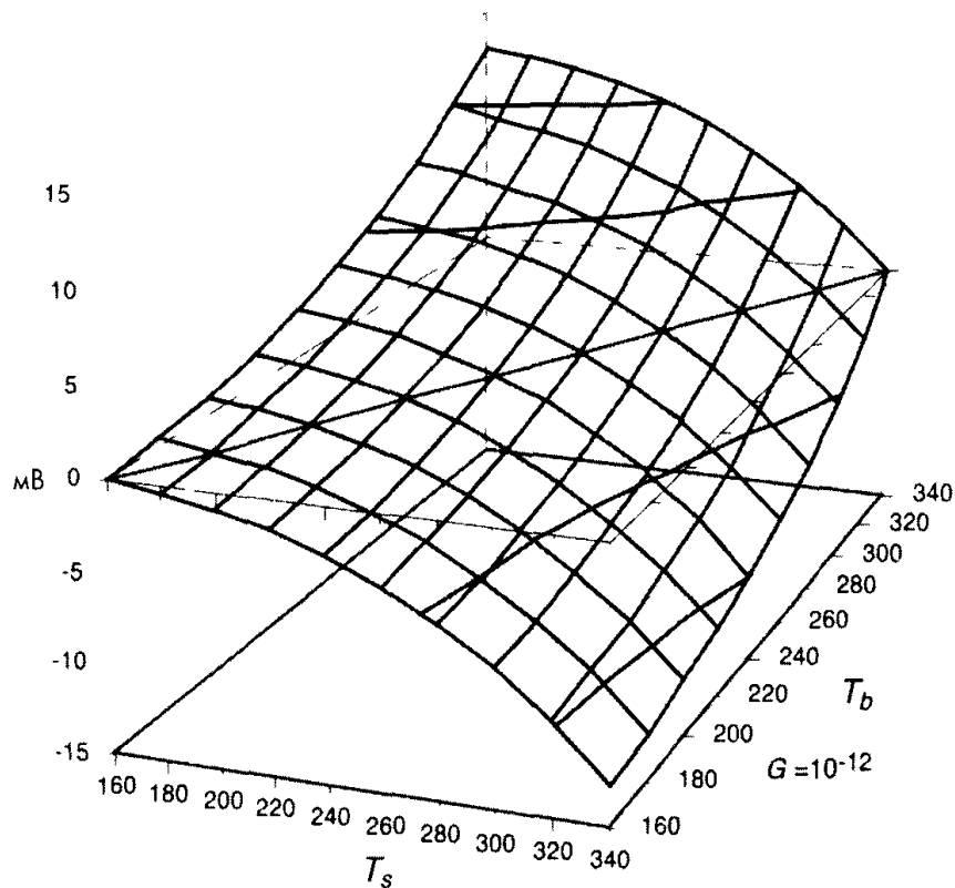
3.1. rasm. Infraqizil harorat datchigining ikki o'lchamli uzatish funksiyasi
