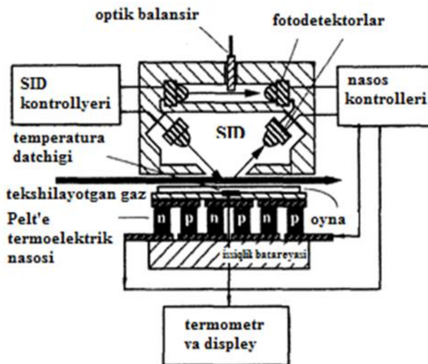
5.32- rasm. Sovutiladigan oynali shudring nuqtasi datchigi
