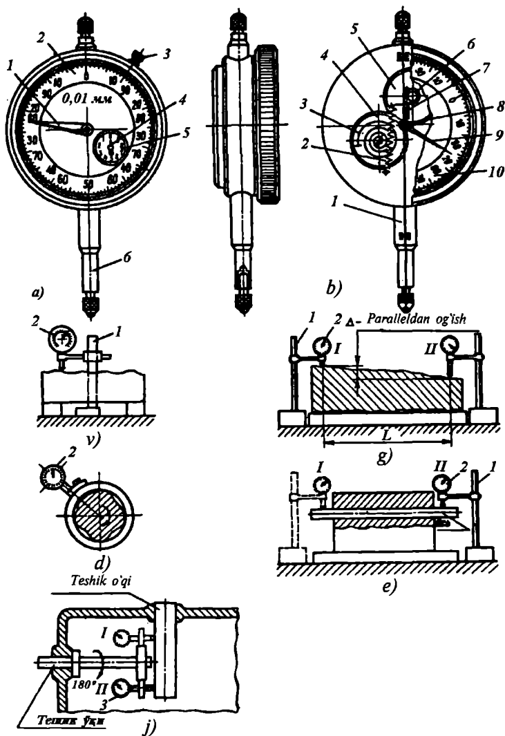
68-rasm. Soat tipidagi indikator (a) va uning tuzilishi (b), chiziqlikdan (v), parallellikdan (g), dumaloqlikdan (d), tekislikka nisbatan o'qning parallelligidan (e), o'qlarning perpendikulyarligidan (j) og'ishlarni o'lchashga doir misollar.
