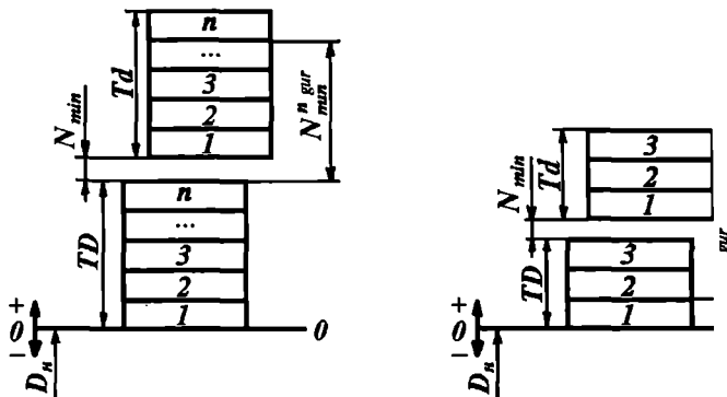
22-rasm. Selektiv yig'ishda tarangli o'tqazishlar uchun saralash guruhleri sonini aniqlash sxemasi ( N_{\min}^{gur} berilgan holat uchun).
