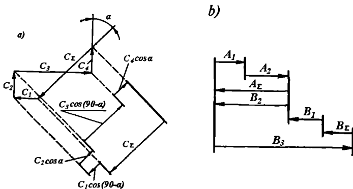
58-rasm. O'lchamlar zanjiri. a) fazoviy; b) chiziqli.
