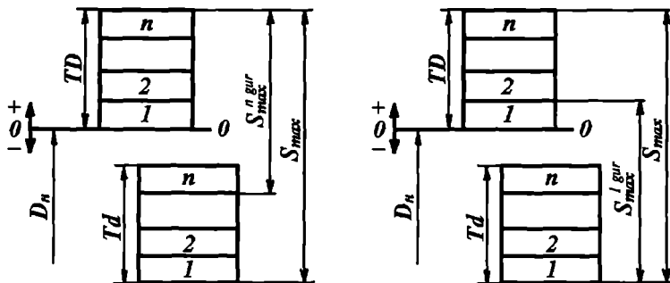
21-rasm. Selektiv yig'ishda tirqishli o'tqazishlar uchun sara-lash guruhlarini aniqlash sxemasi ( S_{\max}^{gur} berilgan holat uchun).
