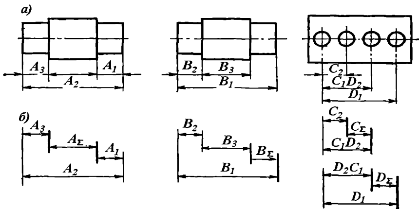
52- rasm. Detal bo'yicha chiziqli o'lchamlar zanjirlari.
