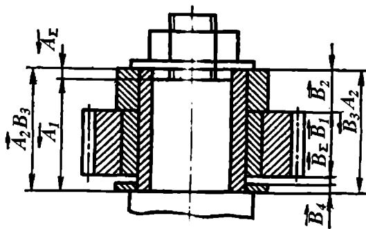
57 – rasm. Ko'payuvchi o'lchamlar zanjiri.
