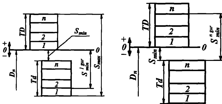
20-rasm. Selektiv yig'ishda tirqishli o'tqazishlar uchun sara-lash guruhlarini aniqlash sxemasi ( S_{\min}^{gur} berilgan holat uchun).
