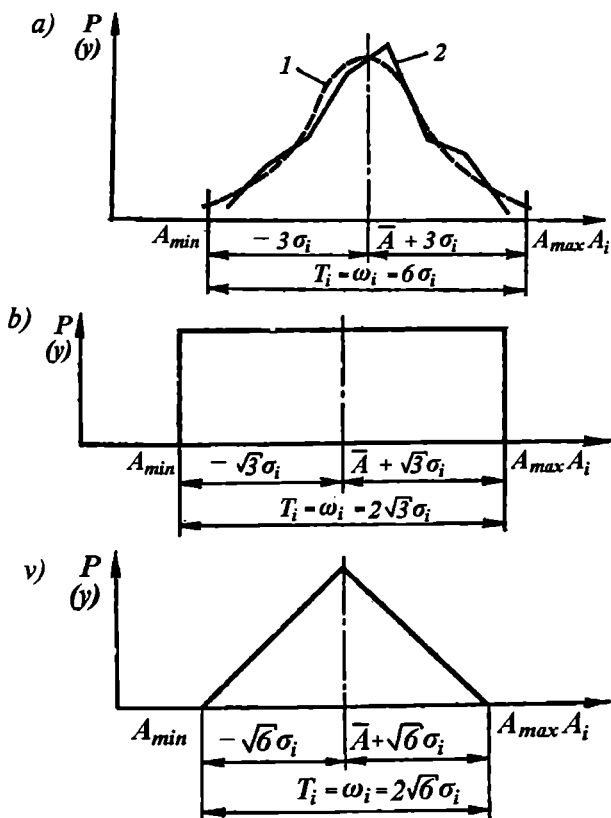
60 – rasmi. Detallar o'lchamlarining taqsimlanish asosiy qonunlari. a-me'yoriy; b-teng ehtimollar; v-uchburchak (Simpson) qonunlari.
