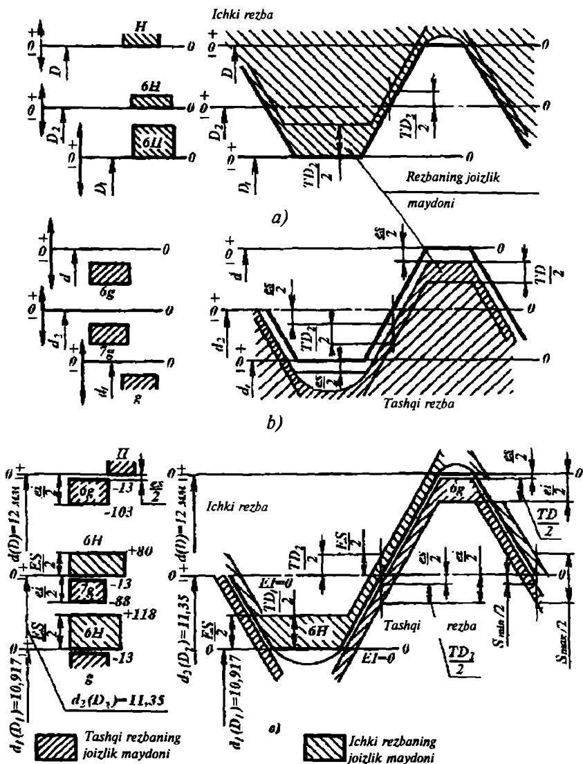
37-rasm. Metrik rezba joizlik maydonlarining joylashish sxemasi, a-ichki, b-tashqi rezbalar uchun, v-tirqishli o'tqazishlar bo'yicha birikkan rezballi detallar.
