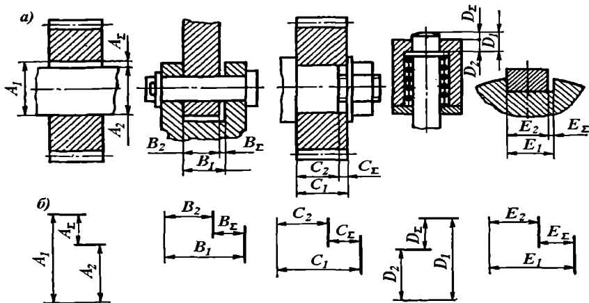
53 - rasm. Yig'ma chiziqli o'lchamlar zanjirlari.
