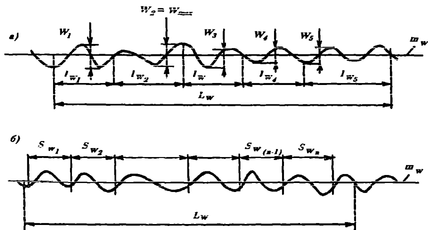
9-rasm. Sirtning to'qlinligi.
