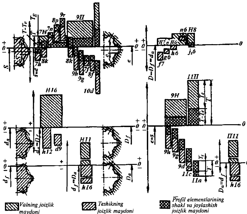
32-rasm. Evolventali shliitsali val va vtulkalarning asosiy parametrlari, joizlik maydonlarining joylashish sxemasi.
