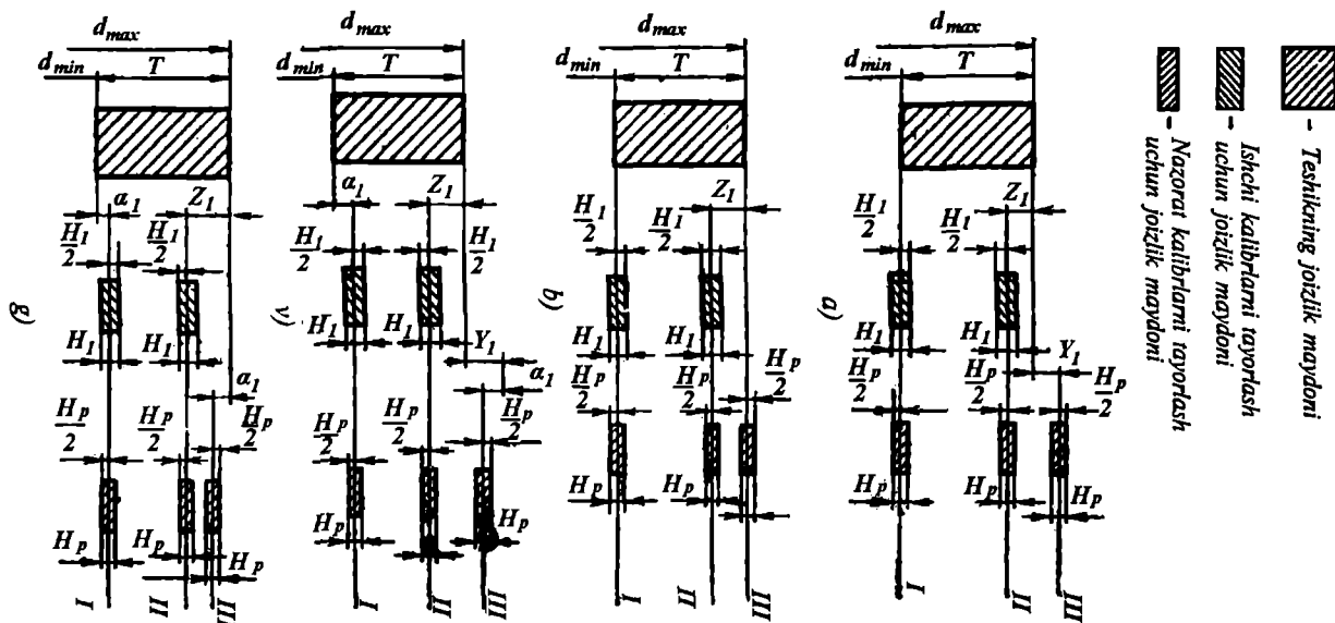
77-rasm. Vallar uchun kalibrar joizlik maydonlarining joylashish sxemasi (I-o'tmaydigan tomoni; II-o'tadigan tomoni; III-eyilish chegarasi).
