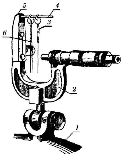
52-rasm. Uch sim usulida o'lchashga moslashtirilgan mikrometr:
