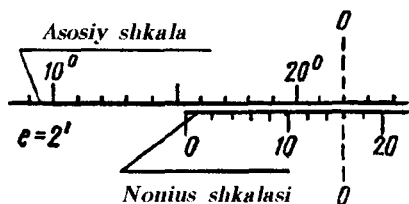
33-rasm. O'lanayotgan burchak qiymatini aniqlash sxemasi.
