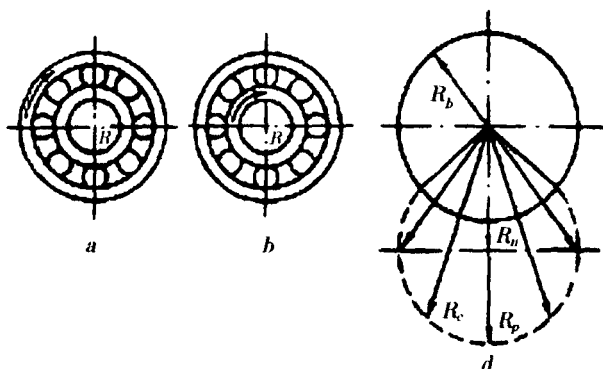
8-rasm. Podshipnik halqalarining yuklanish turlari: a) tashqi halqa aylanma, ichki halqa mahalliy yuklangan; b) tashqi halqa mahalliy, ichki halqa aylanma yuklangan; d) tebranma yuklanish sxemasi.
