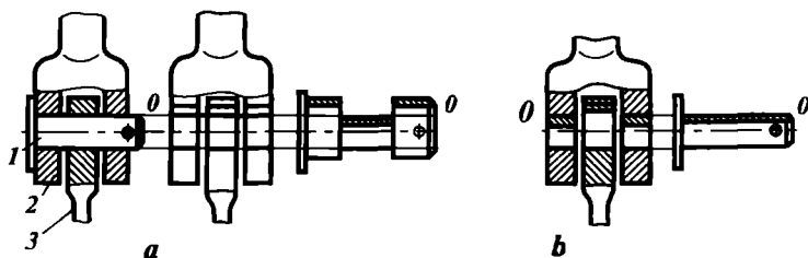
2.5-rasm. Vilka bilan tortkichning shamirli birikmasi (valikning shakli va joizlik maydonlari ko'rgazmali bo'lishi uchun bo'rttirib ko'rsatilgan):
