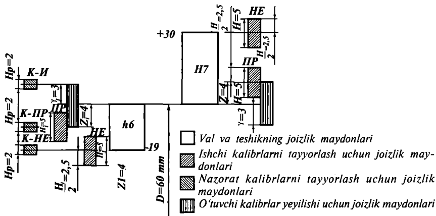
3.22-rasm. Ø60H7/h8 o'lchamli birikma detallarini nazorat qiluvchi kalibr lar joizlik maydonlarining joylashishi sxemasi.
