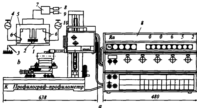
5.37-rasm. Profilograf-profilometr:
