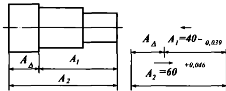
9.11-rasm. Pog'onali detalning o'lchamlar zanjiri.
