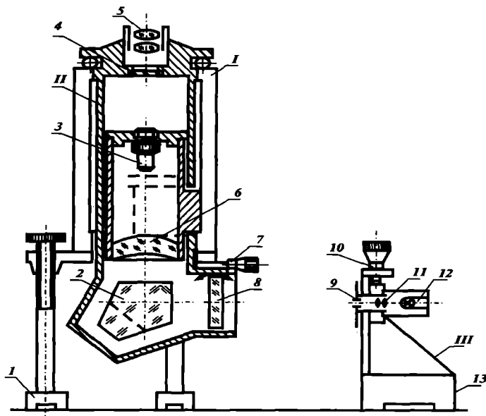
5.17-rasm. Optik-mexanikaviy yassilik o'lachagichi.
