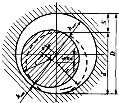
3.6-rasm. Val sapfasining tinch holda (shtrix chiziq) va podshipnik o'mashgan rejimda ishlaganda joylashishi sxemasi.
