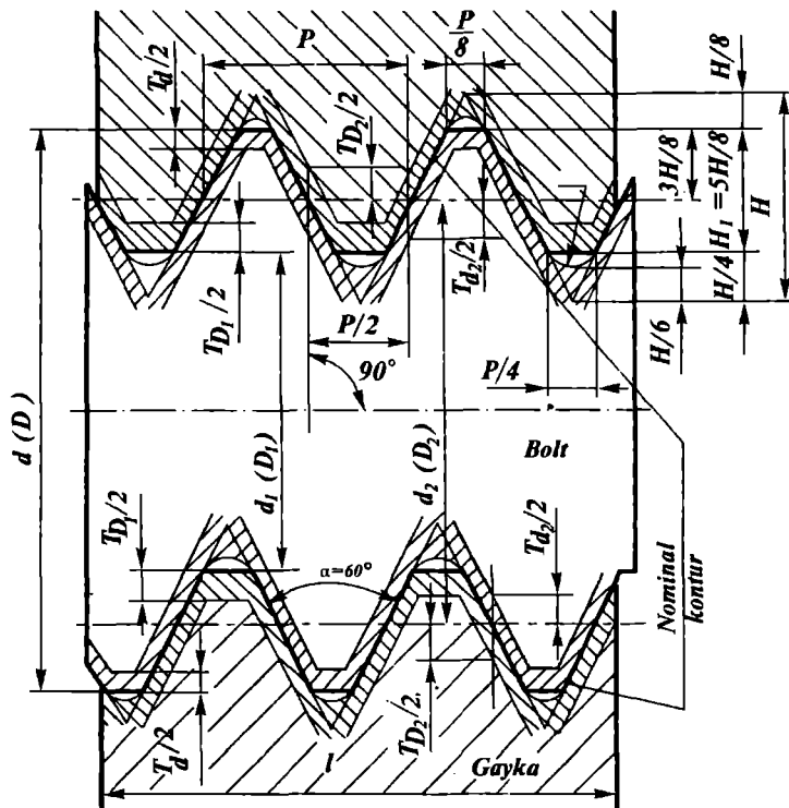
6.2-rasm. H/h o'tqizilmali metrik pezbali birikmaning profili va chekka konturlari.
