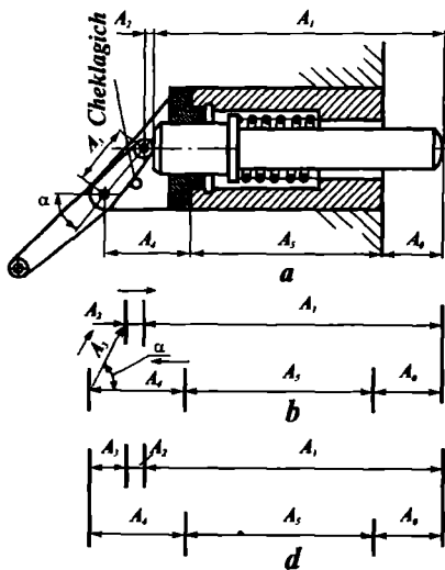
9.15-rasm. Uzelning eskizi (a); ясси o'lichamlar zanjiri (b); to'g'ri chiziqli o'lichamlar zanjiri (d).
