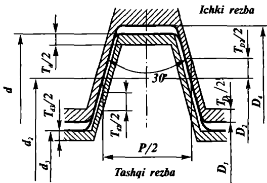
6.10-rasm. Bir kirimli trapetsiyasimon rezba joizlik maydonlarining joylashishi.
