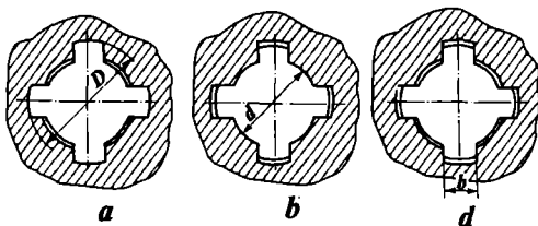
8.4-rasm. To'g'ri yonli shlisli birikmalar:
