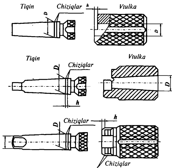
4.6-rasm. Konus va kalibrblar:
