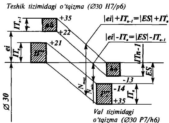
3.2-rasm. Teshiklarning asosiy og'ishlari-ni maxsus qoida bo'yicha aniqlash sxemasi.
