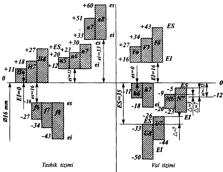
3.3-rasm. ISO va JO'YaTdA tizimida o'tqizmalarining hosil qilinishini tasvirlovchi joizlik maydonlari joylashishining sxemasi.
