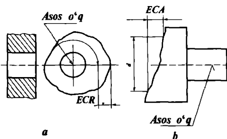
5.23-rasm. Radial va yonlama tepish.
