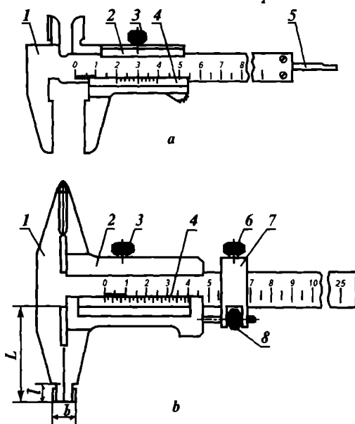
1.6-rasm. Shtangensirkullar:
