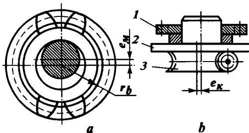
7.6-rasm. Eksentrisitetlarning turi.
