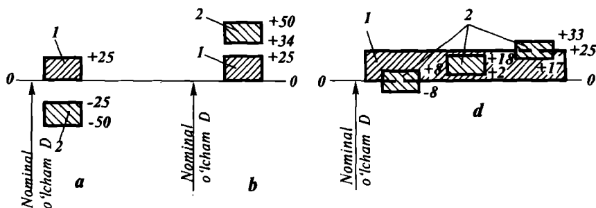
2.2-rasm. Joizlik maydonlarining joylashishi:
