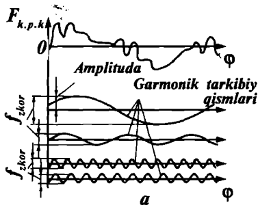
7.8-rasm. Kinematik xatolik va uning garmonik tarkibiy qismlari o'zgarishining tavsifi:
