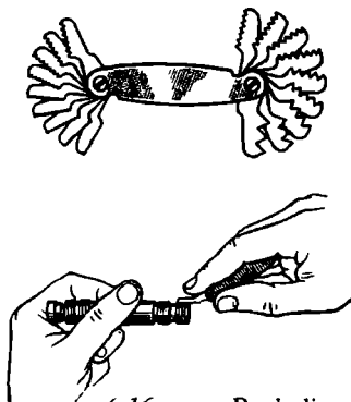
6.16-rasm. Rezbali shablonlar.
