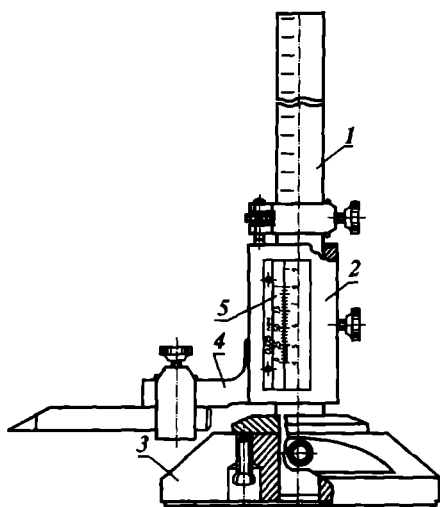
1.8- rasm. Shtangenreysmas.
