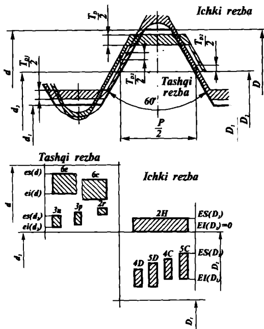
6.8-rasm. Taranglikli rezba joizlik maydonlarining joylashishi: es , ES — tegishli ravishda tashqi va ichki rezbalar diametrlarining yuqori og'ishlari; ei , EI — tegishli ravishda tashqi va ichki rezbalar diametrlarining quyi og'ishlari.
