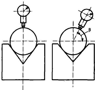
5.6-rasm. Toq sonli qirralikni o'lchash.
