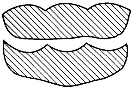
5.30-rasm. Har xil shaklli, lekin Ra ning bir qiymatiga ega bo'lgan yuza notekisliklari profillarining misollari.
