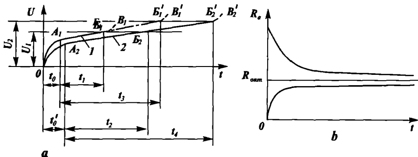
5.40-rasm. Aylanuvchi detallar yeyilishini tavsiflovchi egri chiziqlar:
