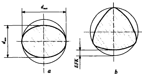
5.4-rasm. Yumaloqlik o'lganagichlari.
