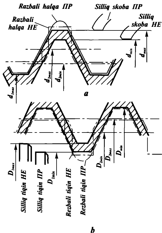
6.12-rasm. Rezba kalibrlar yordamida tekshirish sxemalari:
