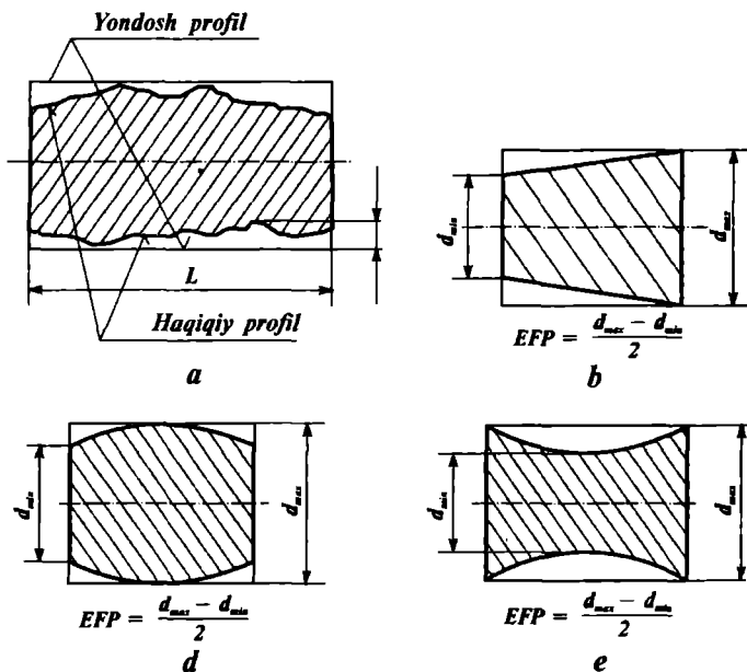
5.7-rasm. Silindrik detal bo'ylama kesimining og'ishlari:
