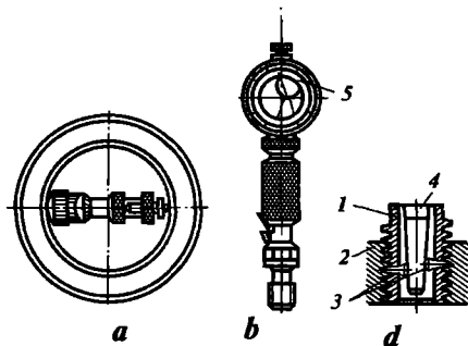
6.18-rasm. Ichki rezba o'rta diametринi o'lchovchi asboblار.
