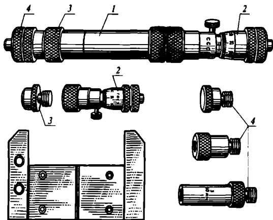
1.22-rasm. Mikrometrik ich o'lchagichi.
