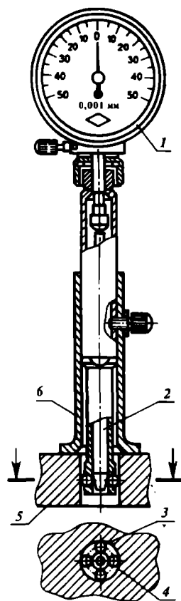
1.24-rasm. Soqqali ich o'Ichagichi.
