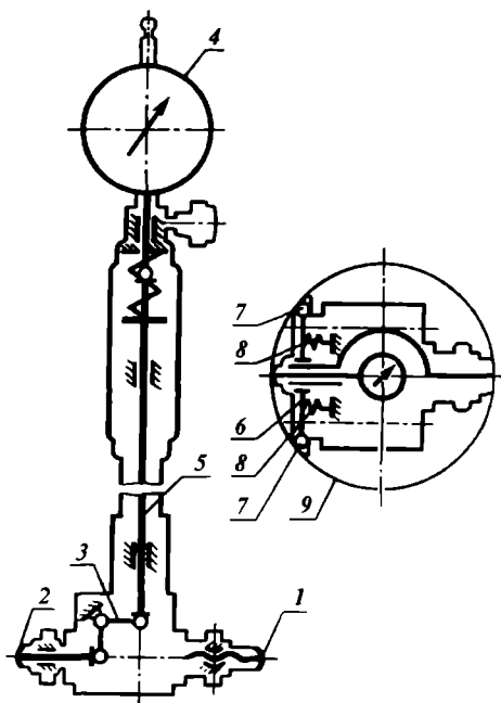
1.23-rasm. Milli sanash kallakli ich o'lchagichi.
