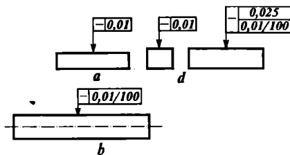
5.10-rasm. Chizmalarda to'g'ri chiziqlikka bo'lgan talablarni belgilash.
