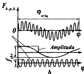
7.8-rasm. Kinematik xatolik va uning garmonik tarkibiy qismlari o'zgarishining tavsifi:
