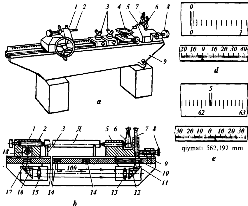
1.28-rasm. ИЗМ o'lash mashinasi:
