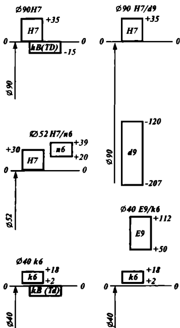
3.14-rasm. 3.13-rasmda ko'rsatilgan detallar joylik maydonlarining joylashish sxemasi.
