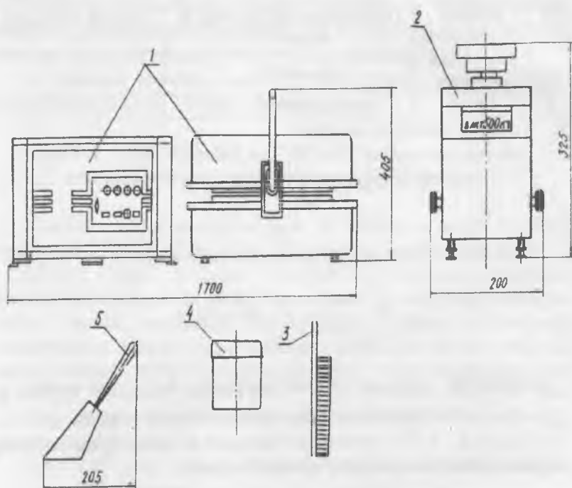
3-rasm. VXS namlikni tezkor o'lchash uskunasi:
