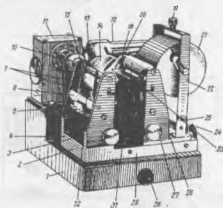
17-rasm. PPL- pilik tayyorlash uskunasi chizmasi:
