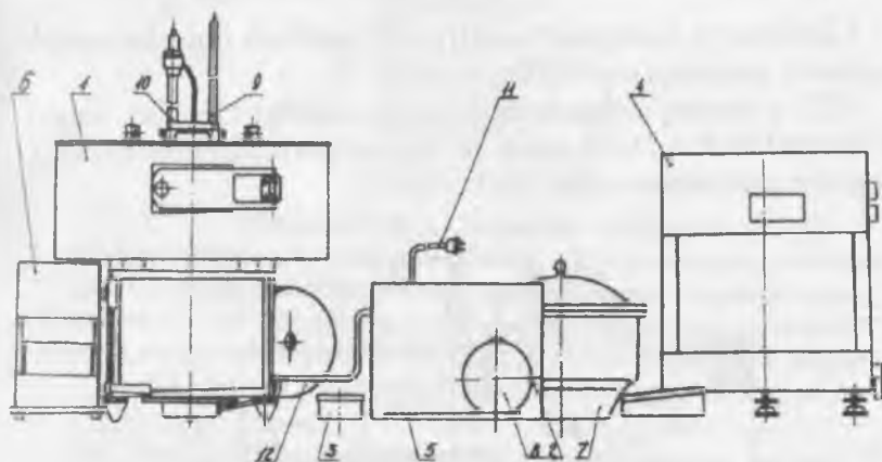
8-rasm. Uz-8 qurilmasi:
