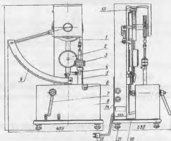
19-rasm. Tola pishiqligini aniqlash uchun DSH-3M-2 dinamometrning chizmasi:
