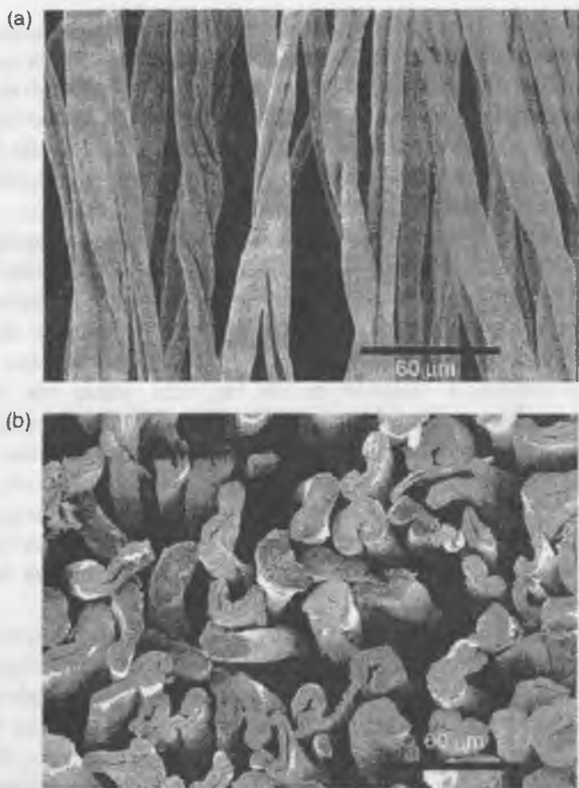
2-rasm. Paxta tolalarining elektron mikrofotografiyasi: (a) bo'ylama va (b) ko'ndalang qirgimi.
