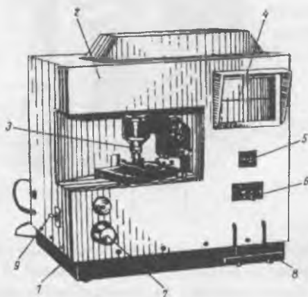
18- rasm. PSV-1 proyeksion tola sanagichining umumiy ko'rinishi: 1 - asosi; 2 - qobig'i; 3 - mikroskop; 4 - ekran; 5 - sanagich; 6 - tasvirni surish uch pozitsiyali tumbleri; 7 - ekran (4) da tola tasvirini surish tezligini o'zgartirish potentsiometri dastasi; 8 - kontakt kalitining klavishi; 9 - yoritgich va sanagichlarni ulashni ta'minlash tumbleri.
