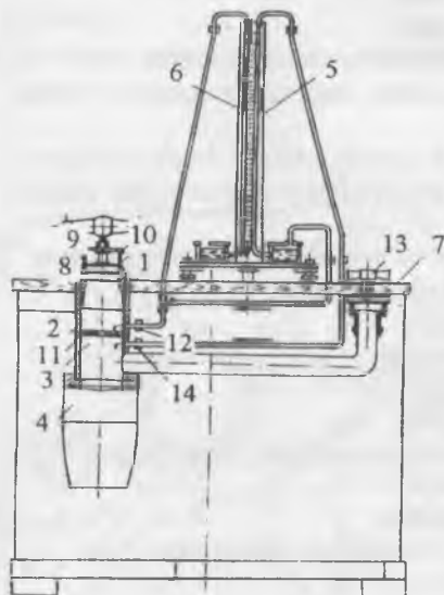
14-rasm. LPS-4 uskunasi chizmasi:
