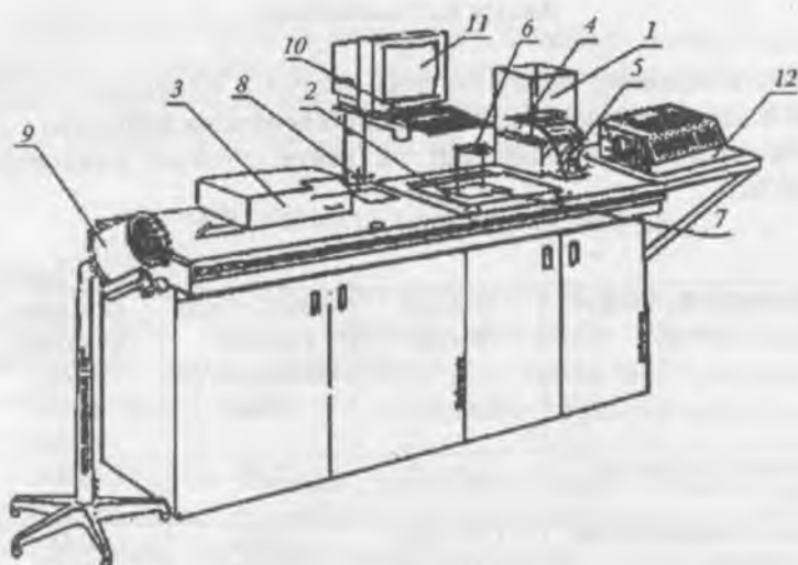
32-rasm. USTER HVI 900 SA o'lchov tizimining chizmasi:
