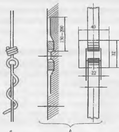
39-rasm. Toylarni bog'laydigan belbog'larni bog'lash chizmasi: a - sim bilan bog'langanda; b - tasma bilan bog'langanda.
