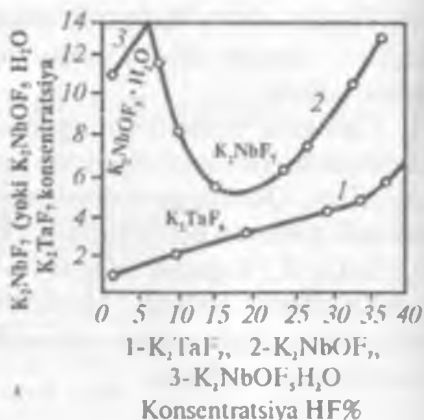
2- grafik. Turli konsentratsiyali plavik kislotalarda tantal va niobiyning fiorti komplekslarining (25°C da) erishi.
