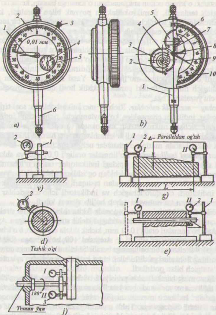
68-rasm. Soat tipidagi indikator (a) va uning tuzilishi (b), chiziqlikdan (v), parallellikdan (g), dumaloqlikdan (d), tekislikka nisbatan o'qning parallelligidan (e), o'qlarning perpendikulyarligidan (j) og'ishlarni o'lchashga doir misollar.
