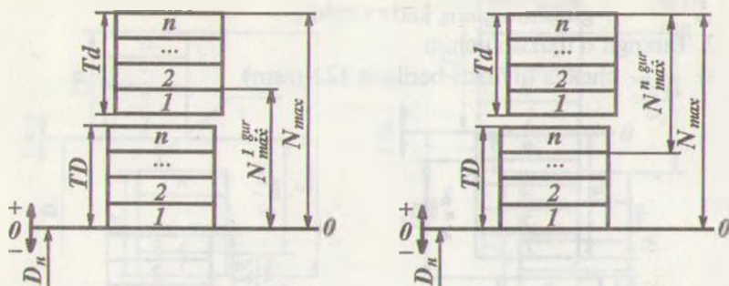
23-rasm. Selektiv yig'ishda tarangli o'tqazishlar uchun saralash guruhlari sonini aniqlash sxemasi ( N_{\max}^{gur} berilgan holat uchun).
