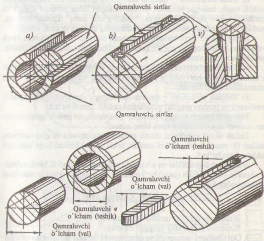
1-rasm. Qamrovchi va qamraluvchi detal va o'lchamlar.
