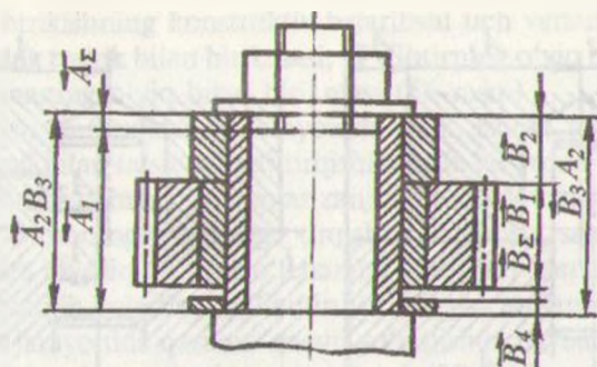
57 — rasm. Ko'paytma o'lchamlar zanjiri.
