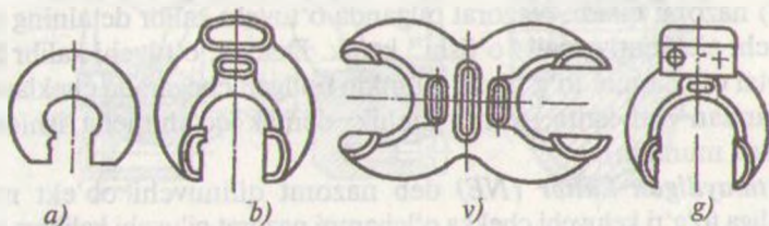
73-rasm. Vallar uchun asosiy kalibrlarning turlari. a—bir tomonli changak 1...180 mm uchun; b—shtamplangan bir tomonlama changak 3...50mm uchun; v—shtamplangan ikki tomonlama changak 3...100 mm uchun; g—dastali bir tomonlama shtamplangan changak 50...170 mm uchun.
