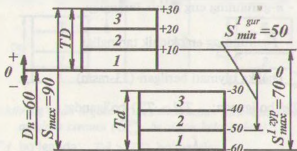
24-rasm. Selektiv tanlash usulida yig'ishga doir misol.
