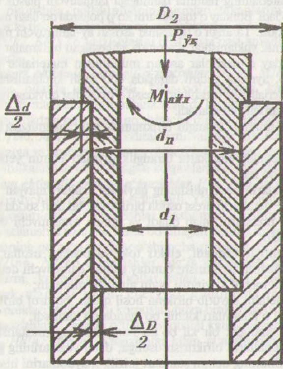
17-rasm. Tarang o'tqazishdagi val va teshik o'lchamlarining munosabati.
