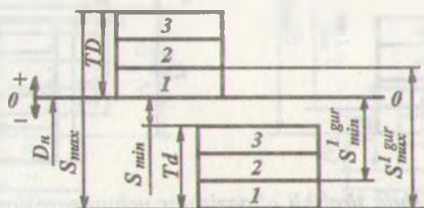
18-rasm. Selektiv yig'ishda tirqishli o'tqazish uchun saralash guruhlar sonini aniqlash sxemasi ( TDQTD ).
