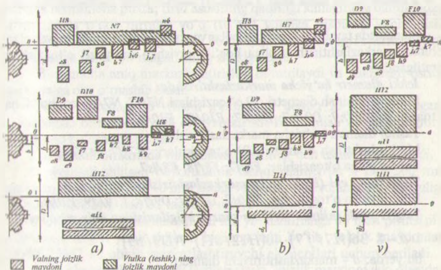
31-rasm. Shlitsali vallar va vtulkalar joizlik maydonlarining joylashish sxemasi.
