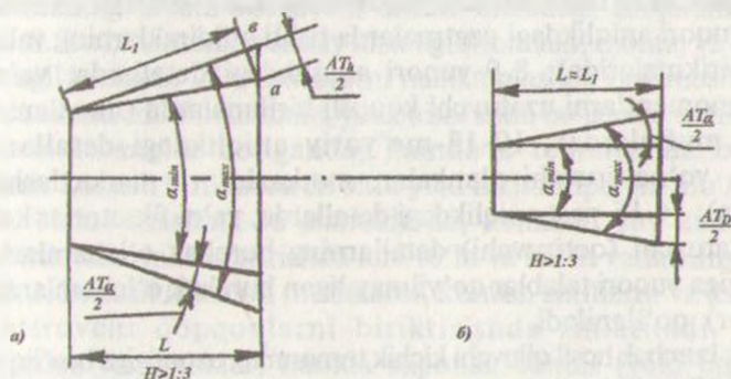
25-rasm. Burchak o'lchamlari joizligi va ularning belgilanishi.
