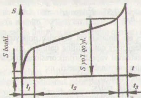
14-rasm. Tirqishning vaqt bo'yicha o'sish jarayoni.
