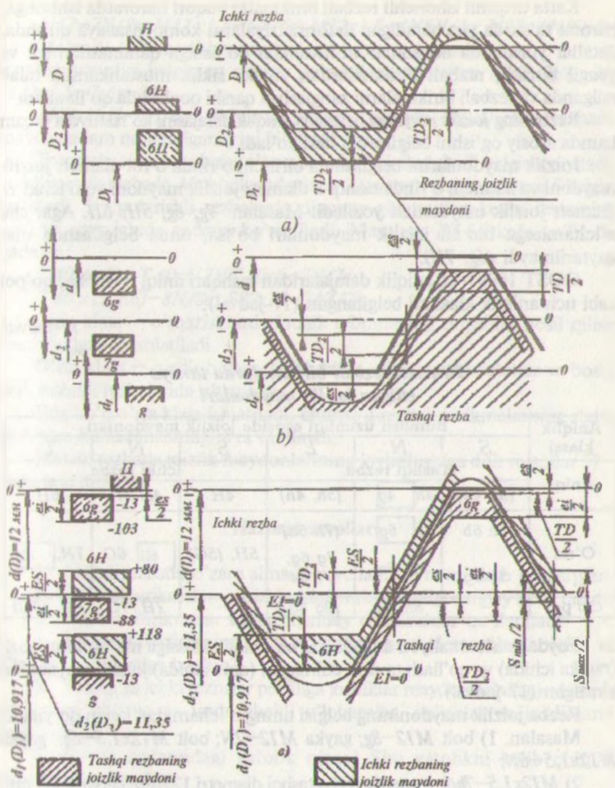
37-rasm. Metrik rezba joizlik maydonlarining joylashish sxemasi, a-ichki, b-tashqi rezbalar uchun, v-tirqishli o'iqazishlar bo'yicha birikkan rezbali detallar.
