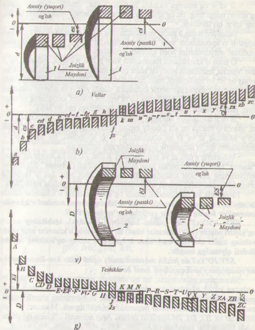
10-rasm. SEV JO'YaT bo'yicha asosiy og'ishlar.
