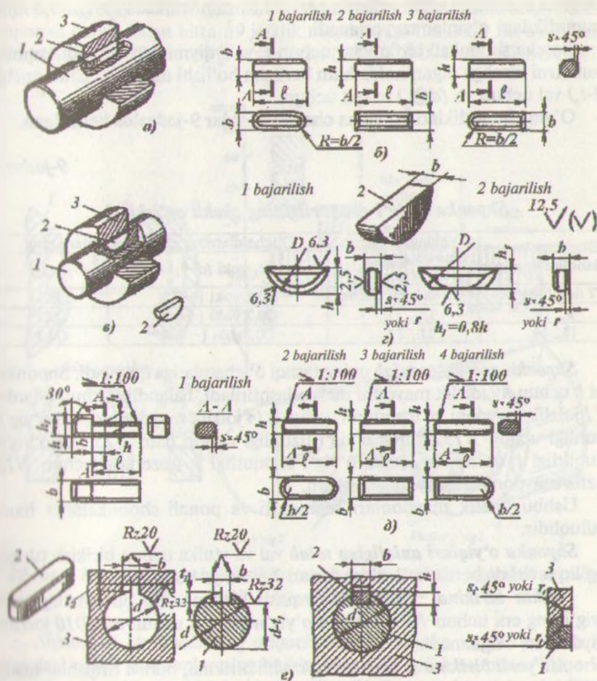
28-rasm. Shponkali birikma va uning turlari. 1-val; 2-shponka; 3-vtulka.
