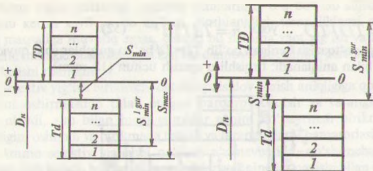
20-rasm. Selektiv yig'ishda tirqishli o'tqazishlar uchun sara-lash guruhlari sonini aniqlash sxemasi ( S_{\min}^{gur} be-rilgan holat uchun).
