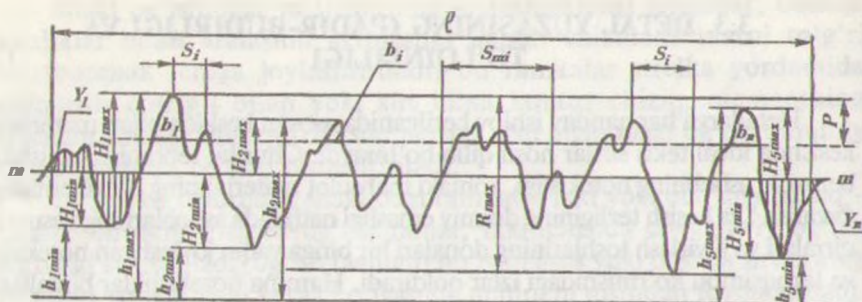
8-rasm. Ishlangan sirtning g'adir-budirligi.
