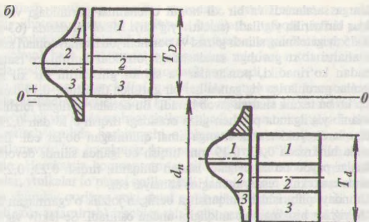
63 — rasm. Selektiv yig'ish:
