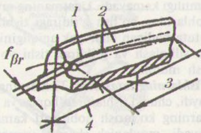
47-rasm. Tishning yo'nalish xatoligi. 1- tishning haqiqiy bo'lish chizig'i;
