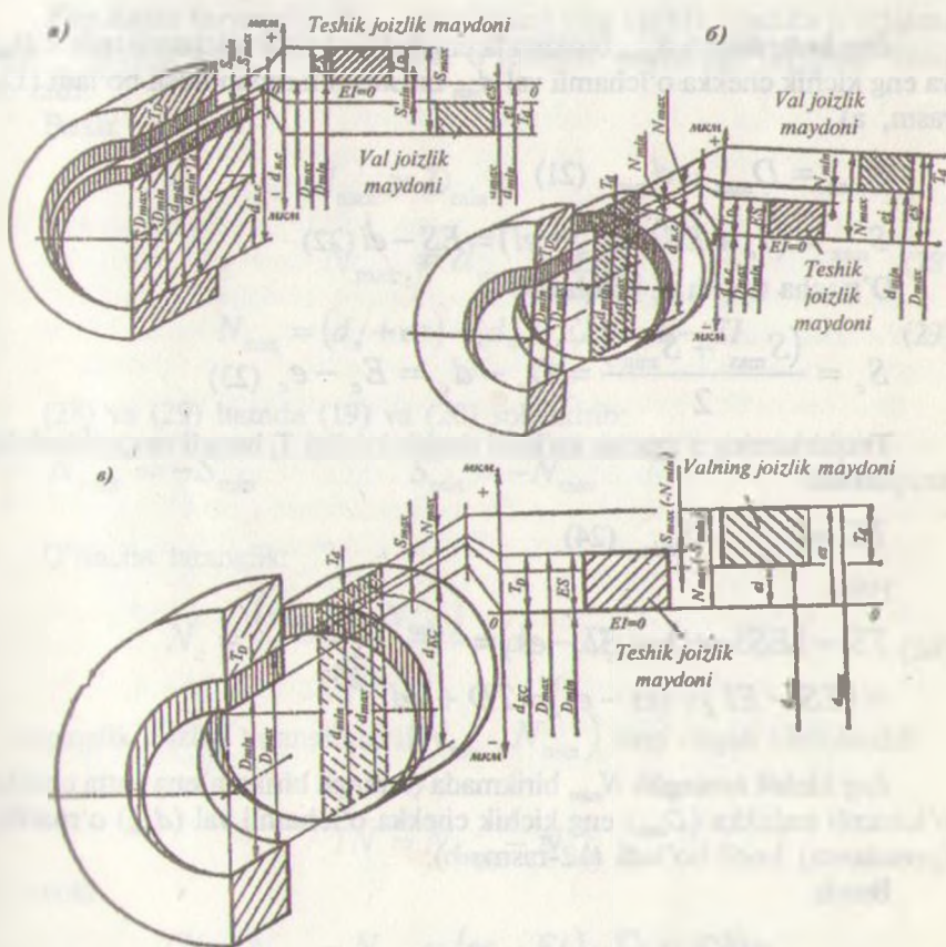
12-rasm. Birikmalardagi a) chekka tirqishlar, b) tarangliklar va v) chekka tirqish va tarangliklar.
