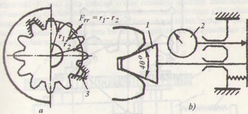
40-rasm. Qadam xatoligi.
