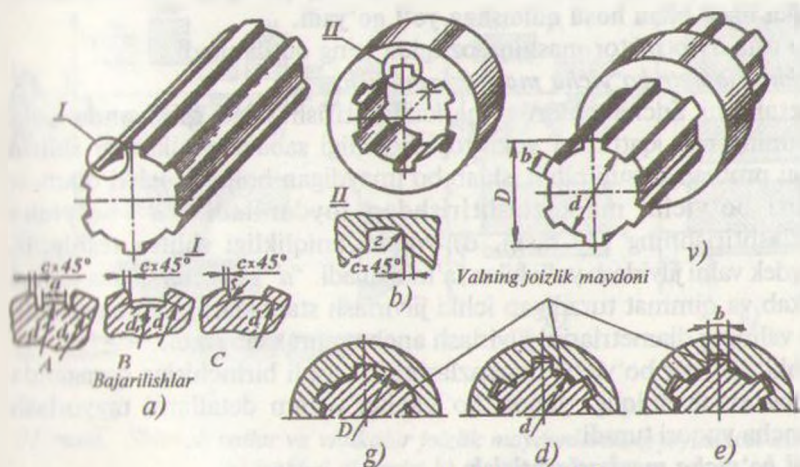
30-rasm. To'g'ri yonli shlitsali birikma.
