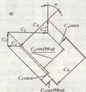
58-rasm. O'lchamlar zanjiri. a) fazoviy; b) chiziqli.
