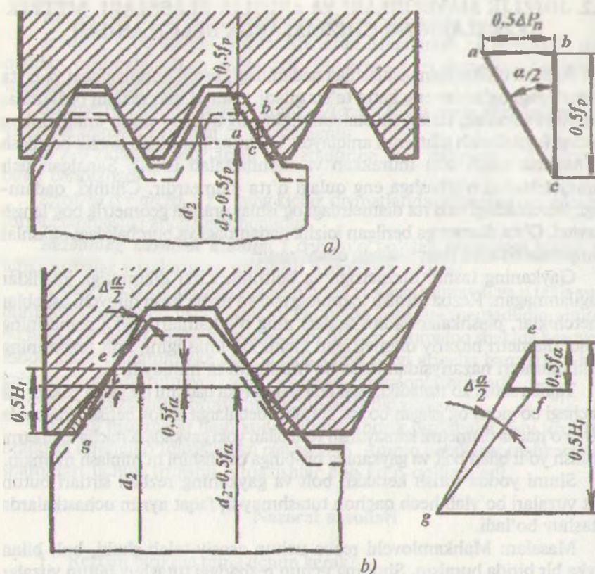
35-rasm. Metrik rezba parametrlari orasidagi bog'liqlik.
