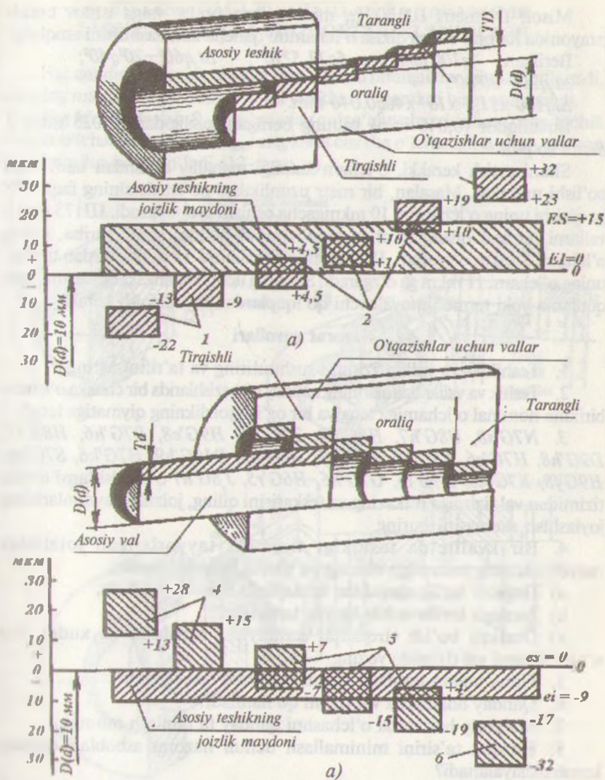
11-rasm. Teshiklar va vallar tizimida o'tqazishlarning joylashishi. a) - teshiklar tizimi. b) - vallar tizimi.
