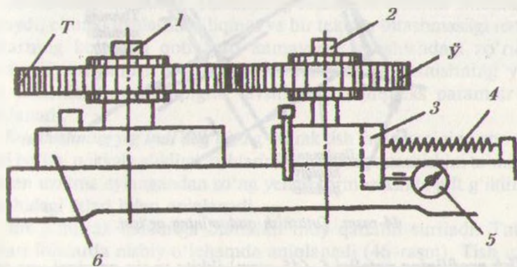
43-rasm. O'qlar oralig'ini o'lchagich.
