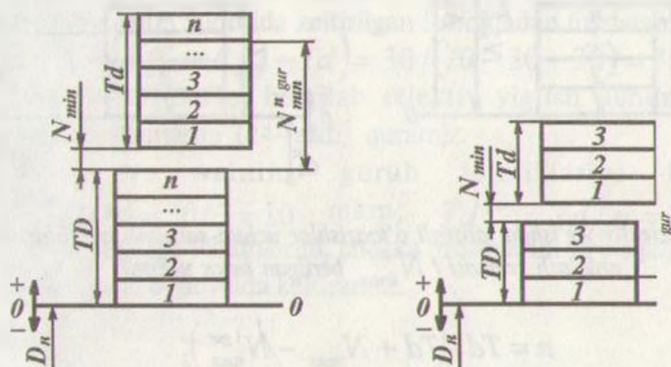
22-rasm. Selektiv yig'ishda tarangli o'tqazishlar uchun saralash guruhleri sonini aniqlash sxemasi ( N_{\min}^{\text{gur}} berilgan holat uchun).
