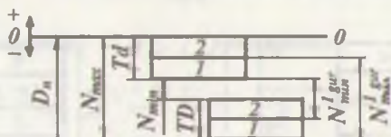
19-rasm. Selektiv yig'ishda tarangli o'tqazish uchun saralash guruhlar sonini aniqlash sxemasi ( TDQTD ).
