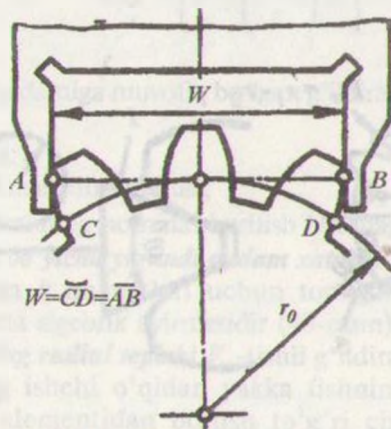
42-rasm. Umumiy me'yor uzunligini aniqlash.
