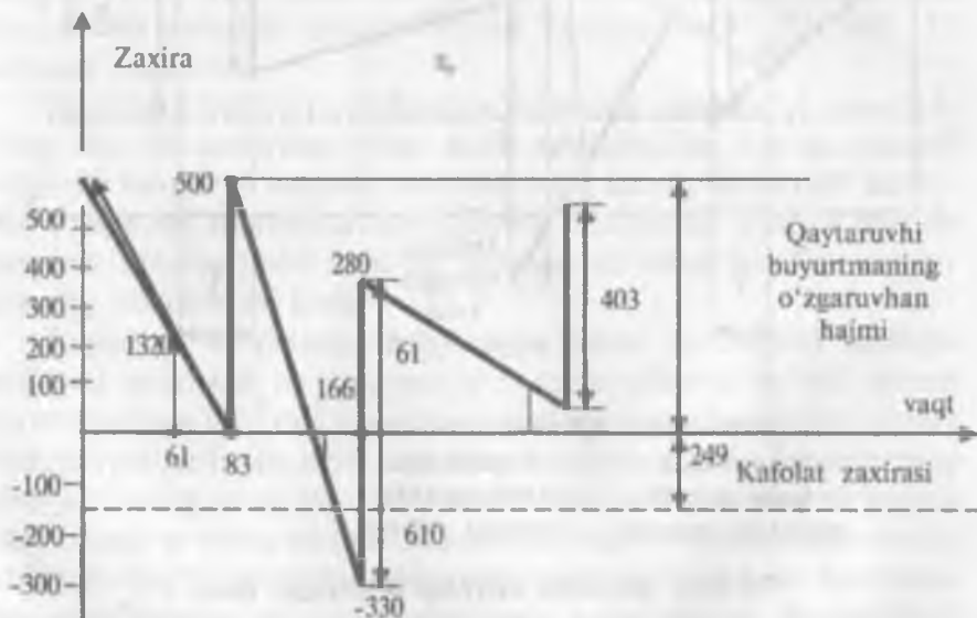
7.3-rasm. Buyurtma davriyligi belgilangan tizimda va materiallarning iste'mol qilinish intensivligi har xil bo'lganda joriy zaxiralar harakatining grafisi.
