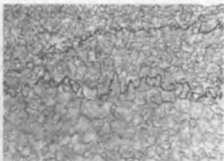
16-rasm. Ohaktoshlardagi stilolitli choklarning mikrofotosurati
