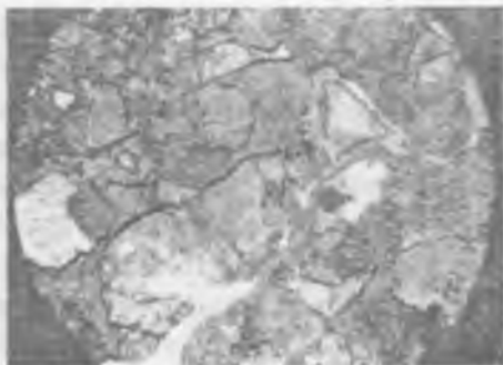
10-rasm. Graviyli polimikt tarkibli qumtoshlarda poykilit tipidagi kalsitli sement mikrofotosurati
