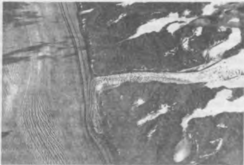
4-rasm. Tog'larda rivojlangan muz oqimlarining fotosurati
