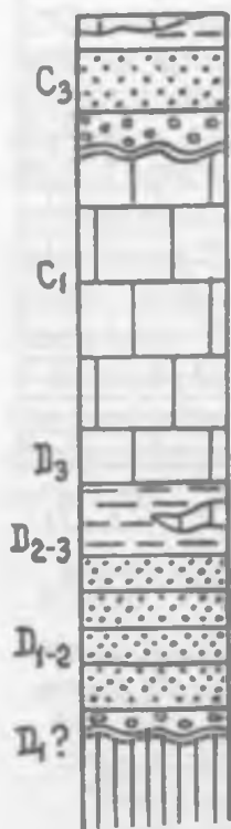
71-rasm. Ikkinchi fatsial zonallik qonunini tushuntiruvchi stratigrafik ustun. Qo'shaloq to'liqlik chiziqli cho'kindi hosil bo'lishdagi uzilishni bildiradi. Boshqa shartli belgilar 70-rasmga berilgan
