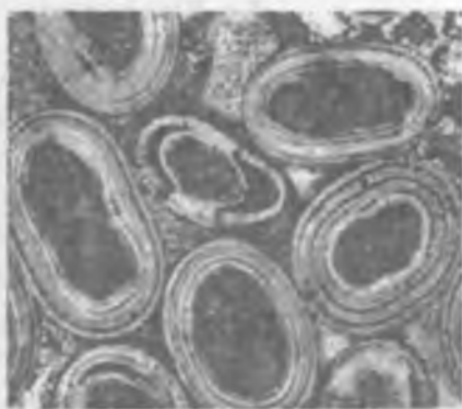
22-rasm. Yadrosiz ohakli pizolitning kesmada ko'rinishi
