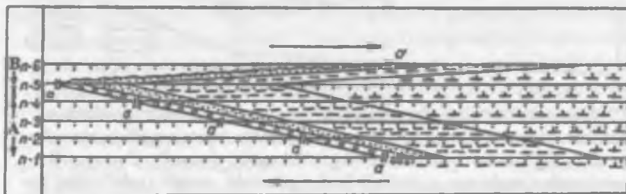
74-rasm. To'rtinchi fatsial zonallik qonunini tushuntiruvchi chizma. To'liqinli chiziqlar – yuvilish yuzasi. Shartli belgilar 72-rasmda berilgan
