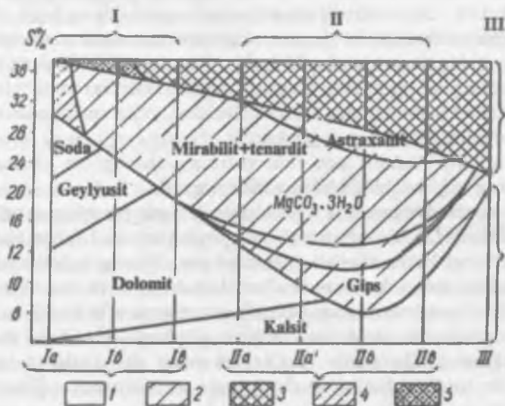
68-rasm. Qurg'oqchil zonalaridagi hozirgi ko'llarda galogenezning umumiy chizmasi (N.M.Straxov bo'yicha). I-sodali ko'llar; Ia-kuchli sodali (Shk>30%); Ib-mo'tadil sodali (Shk 30-3%); kuchsiz sodali (Shk <3%); II-sulfatli ko'llar; IIa-natriy-magniyli; IIa"-magniy-natriyli; IIb-natriy-magniy-kalsiyli; IIv-magniy-kalsiyli; III-NaCl, MgCl, CaCl 2 ga ega bo'lgan xloridli ko'llar. 1-karbonatli bosqich; 2-sulfatli bosqich; 3-xloridli bosqich; 4-soda qo'shimchasi ko'p bo'lgan sulfatli cho'kindilar; 5-natriy sulfatlari qo'shimchalari ko'p bo'lgan galit
