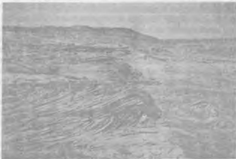
30-rasm. Qatlam ichidagi bir tomonga qiyalangan qiyshiq qat-qatliklarning fotosurati. Yuqori bo'r. Markaziy Qizilqum
