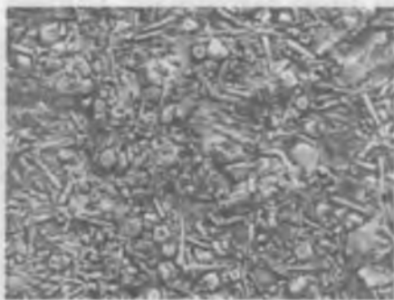
57-rasm. Organogen ohaktoshlarda dengiz nilufarlari qoldiqlarining mikrofotosurati
