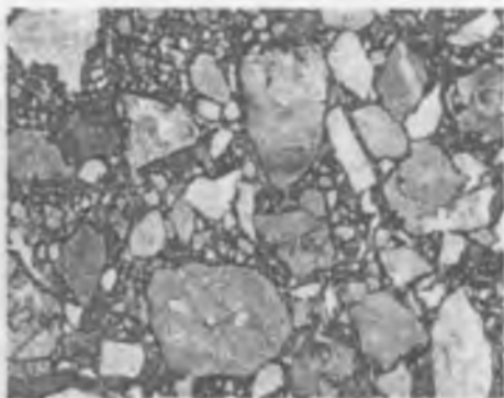
37-rasm. Polimikt tarkibli konglomeratning fotosurati.
