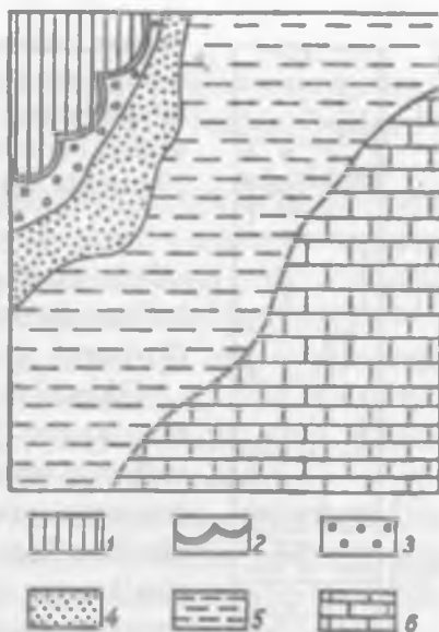
70-rasm. Birinchi fatsial zonallik qonunini tushuntiruvchi chizma.
