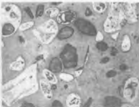
67-rasm. Donali fosforitlar organogen strukturasiining fotosurati. Paleogen. Qizilqum
