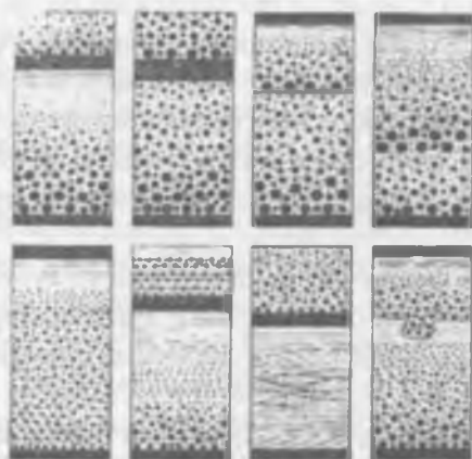
32-rasm. Gradatsion qat-qatlik turlari (Kyunen bo'yicha)
