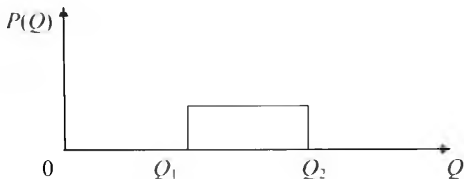
1.25-расм. Эҳтимоллиги текис тақсимланиш қонуниятининг курилишидаги ҳолатий модел
