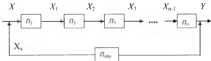
1.11-расм. Таққословчи ўлчаш асбобининг таркибий схемаси
