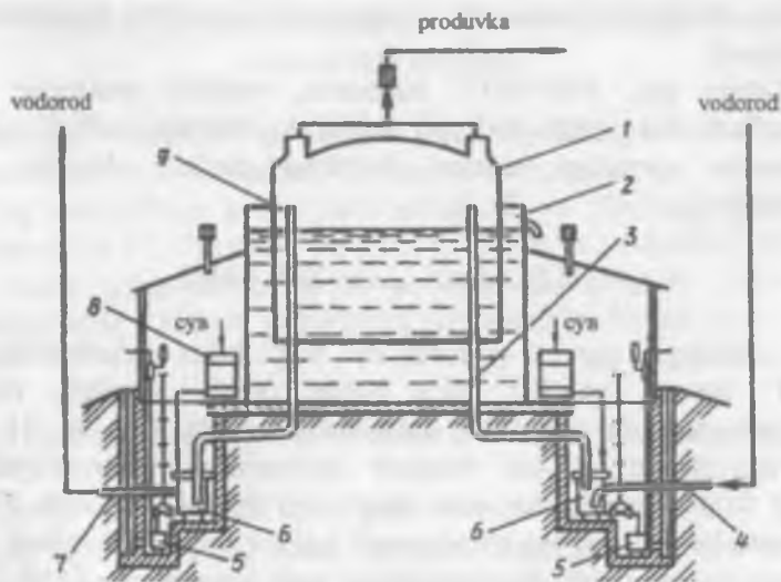
2.5-rasm. Vodorod gazgolderining sxemasi.
