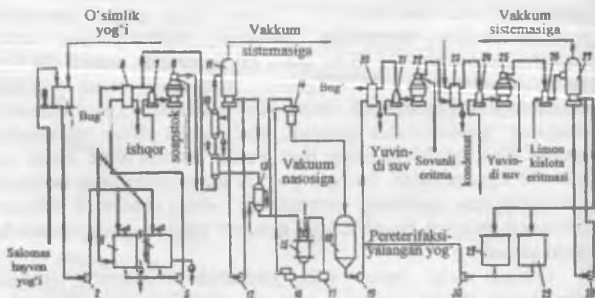
3.20-rasm. Uzlüksiz usulda pereeterifikatsiyalangan yog'lar olish texnologiyasi.
