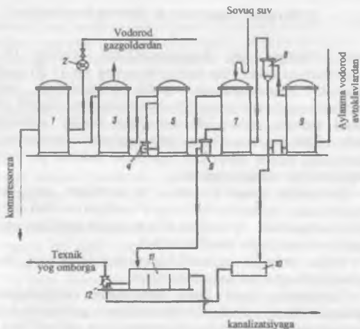
2.9-rasm. Aylanma (aylanma) vodorodni tozalash texnologiyasi.
