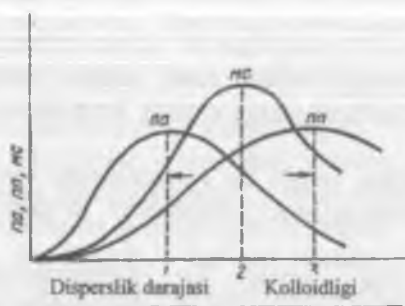
5.4-rasm. Sovun eritmasi (SE)ning yuvish qobiliyatini sirt aktivlik (SA) va sirt mustahkamligi (SM)ni eritmadagi yuvuvchi modda dispersligi (kolloidlik)ga bog'liqligi.
