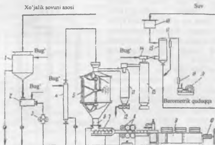
5.13- rasm. Xo'jalik sovuni asosiga ishlov berish texnologiyasi.
