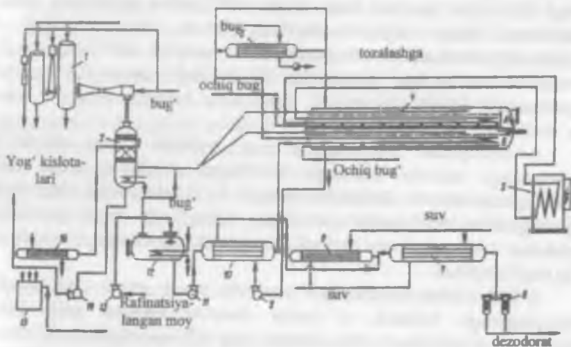
1.19-rasm. «Kixfeld» firmasining unumdorligi 100 t/kun bo'lgan qurilmasida yog'larni hidsizlantirishning texnologik sxemasi.
