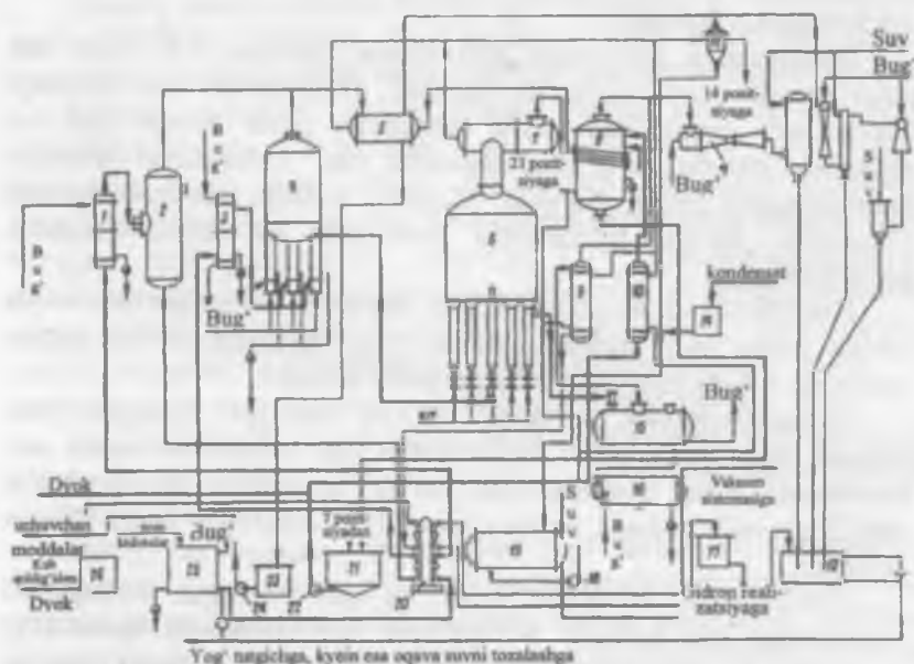
4.11-rasm. Yog' kislotalarini uzluksiz distillyatsiyalashning texnologik sxemasi.
