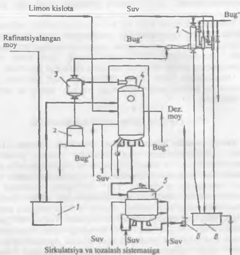
1.15-rasm. Davriy usulda hidsizlantirishni texnologik sxemasi.
