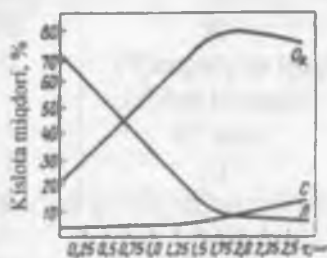
2.1-rasm. Selektiv gidrogenlashda kungaboqar yog'ining yog' kislota tarkibini o'zgarishi.
