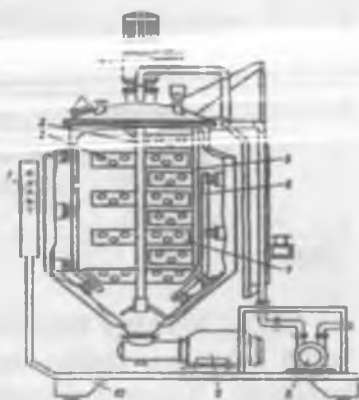
3.7-rasm. «Korum» qurilmasining sarf bak-aralashtirgichining sxemasi.
