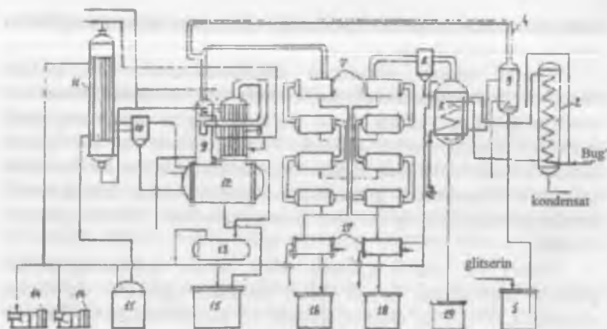
4.9-rasm. Glitserinni distillyatsiya qilish qurilmasining texnologik sxemasi.
