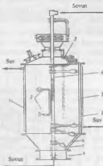
5.12-rasm. Vakuum-quritish kamerasi.
