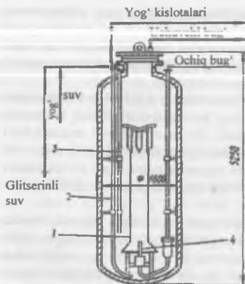
4.4-rasm. Yog'larni gidrolizlash avtoklavi.
