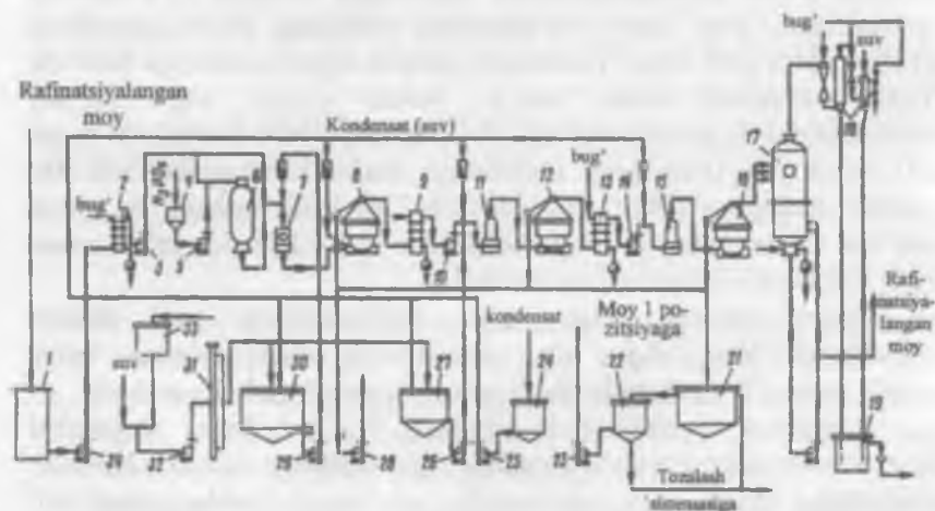
1.8- rasmi. «Alfa-Laval» firmasining unumdorligi 150 t/kun bo'lgan qurilmasida yog'larni rafinatsiyalashning texnologik sxemasi.
