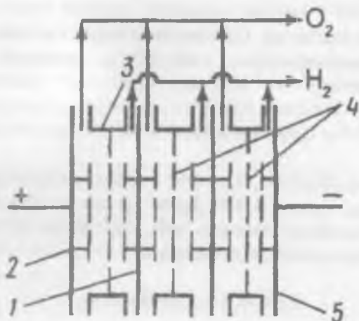
2.3-rasm. Bipolyar elektrodarni ulash sxemasi.
