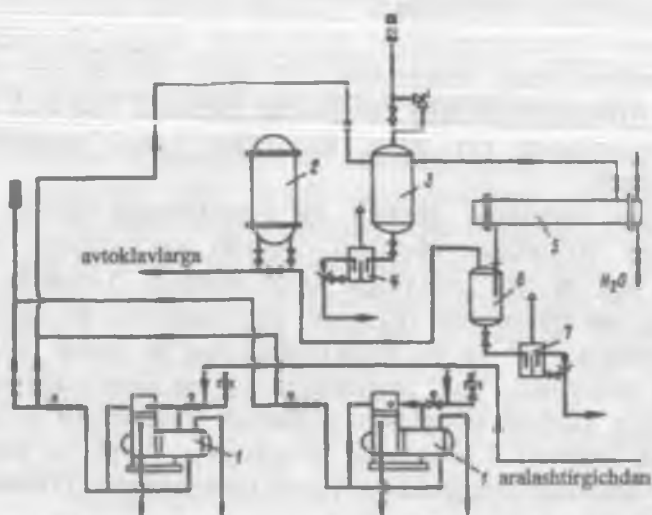
2.10-rasm. Kompressor bo'limining texnologiyasi.
