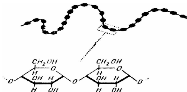
20-rasm. Kraxmal amiloza fraksiyasining tuzilishi.
