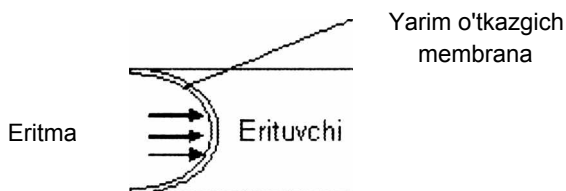
53-rasm. Eritmadagi moddalar urilishi natijasida yarim o'tkazgich membrananing egilishi.
