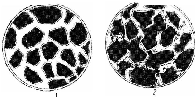
35-rasm. Issiq (1) va sovugan (2) qaynatilib, ezilgan kartoshkani yod bilan bo'yalgan preparatlari
