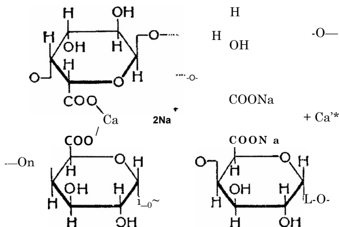
38-rasm. Ikki valentli metall ionlarining bir valentli metall ionlari bilan o'rinlarining almashinishi.
