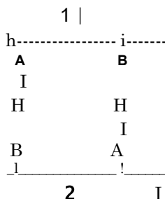
47-rasm. Retseptorlar bilan ta'm yoki hid beruvchi moddalar maxsus halqalari o'rtasida vodorod bog'larining hosil bo'lishi. 1 - ta'm yoki hid beruvchi modda; 2 - retseptor.
