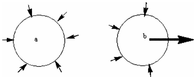
51-rasm. Moddalarning yuqori konsentratsiyali eritmada past konsentratsiyali eritmaga diffuziyasi
