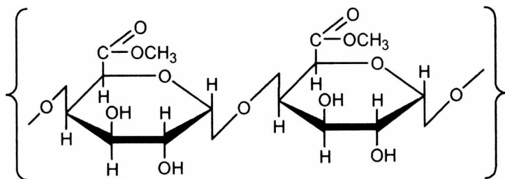
22-rasm. Pektin molekulasining tuzilishi.
