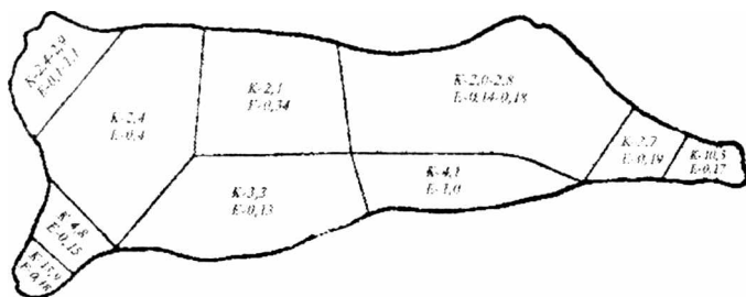
2-rasm. Mol go'shtining kulinar qismlarida kollagen (K) va elastin (E) oqsillarining miqdorlari (%)larda.
