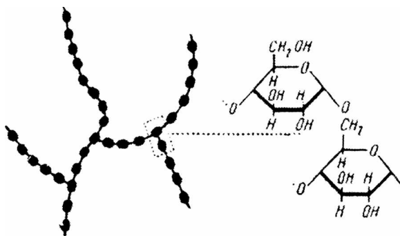
21-rasm. Kraxmal amilopektin fraksiyasining tuzilishi.
