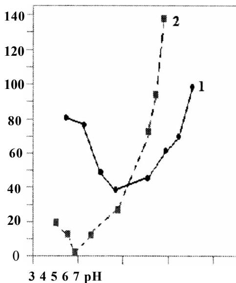
10-rasm. Osh tuzining mol go'shtini suvni adsorbsiya qilish xususiyatiga ta'siri: 1 - tuzlanmagan go'sht; 2 - tuzlangan (2 %) go'sht.
