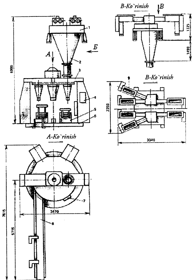
19.4-rasm. 6.055 ADK-50-3VM karuselli o'ltab qadoqlash qurilmasi.
