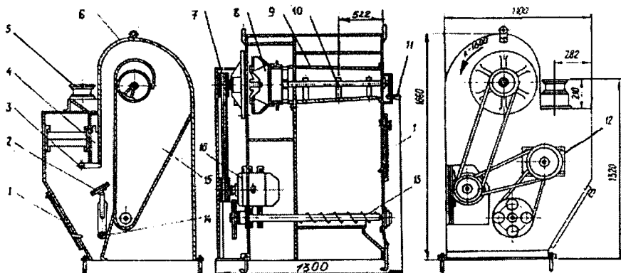
4.5-rasm. A1-BDA aspiratori.
