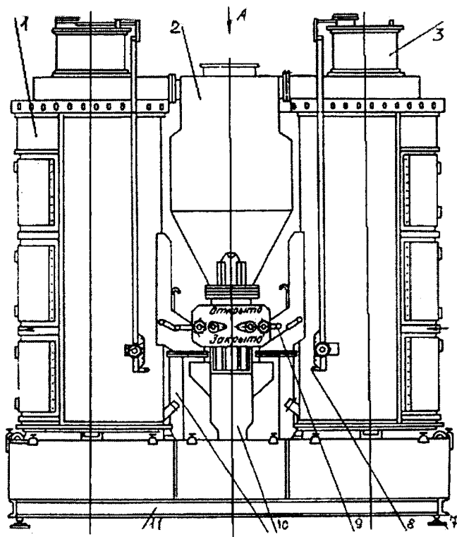
5.4-rasm. R8-USS-2 ajratgichining umumiy koʻrinishi.
