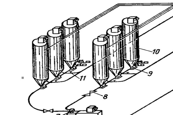
Rasm 26. Unni qopsiz usulda ochiq turdagi omborxonada saqlash sxemasi. 1 - ishlab chiqarish silosi; 2 - havo filtri; 3 - un o'tkazgich kaliti; 4 - oraliq sig'im; 5 - DM-100-2 avtomatik tarozi; 6 - elaklovchi mashina; 7 - matoli filtri; 8 - jumrak; 9 - rotorli ta'minlagich; 10 - bunker; 11 - jumrak; 12 - olti yo'elli kalit; 13 - bunkerlarni aeratsiyalash shuvuri; 14 - kompressor; 15 - unni
