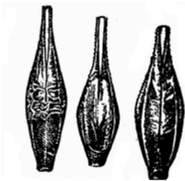
Rasm 8. Arpa donlarining shakllari. 1 - cho'zinchoq; 2 - rombsimon; 3 - ellipissimon.
