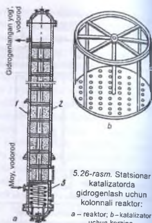
Moyni statsionar katalizatorlar ishtirokida gidrogenlash uchun kolonnali reaktorlar (5.26-rasm)
