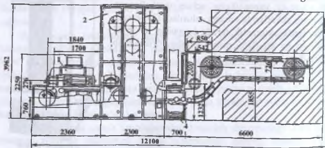
2.7-rasm. Qoliqli non ishlab chiqarish uchun P6-XRM tindirish-pishirish agregati:
