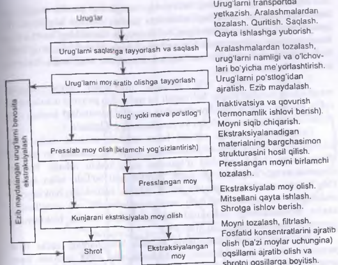
5.1-rasm. O'simlik moylari ishlab chiqarishning asosiy jarayonlari.
