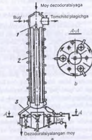
5.23-rasm. Uzlüksiz ishlaydigan dezodorator: a–vertikal qirgim; b–A–A bo'yicha qirgim.
