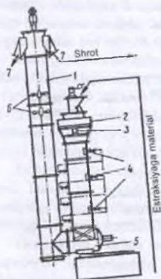
5.10-rasm. ND-1250 rusumli modernizatsiyalangan ekstraktor.
