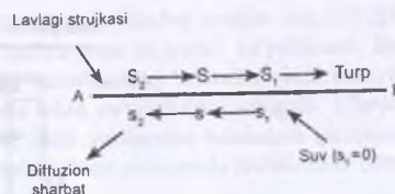
6.3-rasm. Lavlagi strujkasini qarama-qarshi oqimda qandsizlantirish sxemasi: S, S 1 , S 2 – saxarozaning strujkasidagi konsentratsiyasi; s, s 1 , s 2 – saxarozaning diffuzion sharbatdagi konsentratsiyasi.
