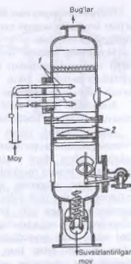
5.19-rasm. Vakuum-quritish apparati.
