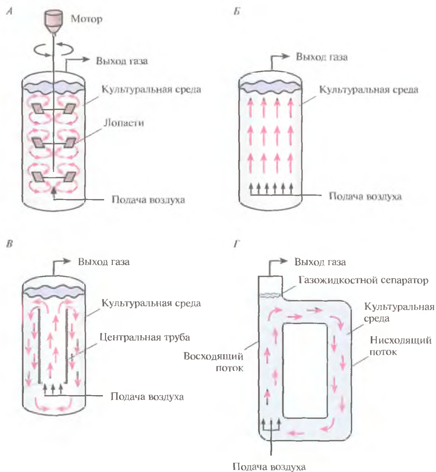
Рис. 16.4. Разные типы биореакторов (упрощенная схема). А. Реактор с механическим перемешиванием. Б. Барботажная колонна. В. Эрлифтный реактор с внутренней рециркуляцией. Г. Эрлифтный реактор с внешней системой рециркуляции. Стрелки — направление потока культуральной среды.
