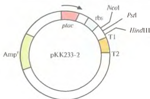
Рис. 6.14. Экспрессирующий вектор на основе плазмиды pKK233-2 (без соблюдения масштаба). Он содержит ген устойчивости к ампициллину ( Amp^r ), являющийся селективным маркером, lac -промотор ( ptac ), lacZ -участок связывания рибосомы ( rbs ), три сайта для рестрицирующих эндонуклеаз ( NcoI , PstI и HindIII ) и два сайта терминации транскрипции (T1 и T2). Стрелка — направление транскрипции.
