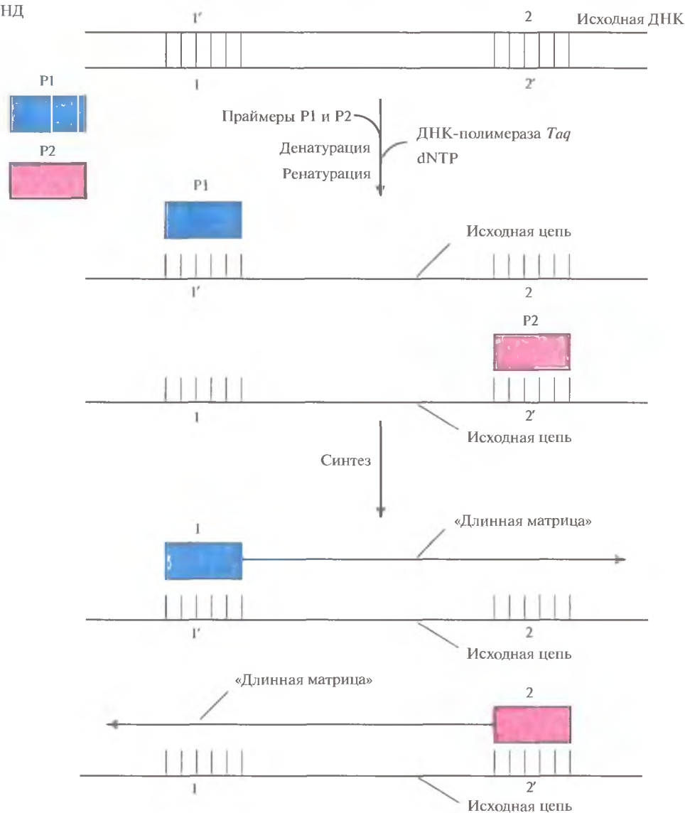
Рис. 5.18. Первый раунд ПЦР. ДНК-мишень фланкирована последовательностями 1'–2' в одной цепи и последовательностями 1–2' — в другой. К образцу ДНК добавляют праймеры (P1 и P2), ДНК-полимеразу Taq и четыре дезоксирибонуклеозидтрифосфата (dNTP). Смесь нагревают до 95 °С, инкубируют в течение 1 мин и медленно охлаждают до 55 °С. При этой температуре праймеры, добавленные в избытке, спариваются с разделенными цепями. Повышают температуру до 75 °С. В этих условиях происходит синтез обеих цепей ДНК, начинающийся с 3'-гидроксильных концов праймеров. Каждая из синтезированных цепей имеет гораздо большую длину, чем расстояние от 3'-гидроксильной группы «ее» праймера до конечного нуклеотида последовательности, комплементарной второму праймеру. Эти цепи служат матрицами во втором раунде ПЦР.
