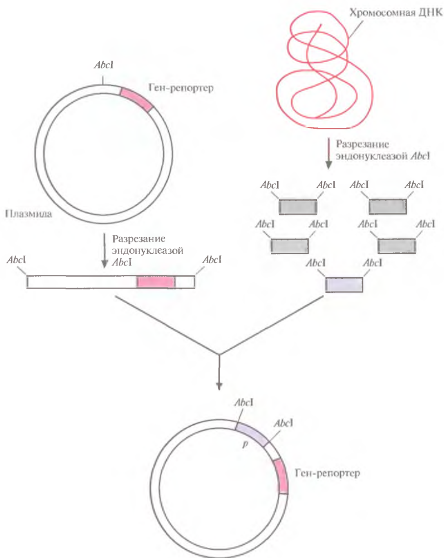
Рис. 6.1. Идентификация сильных регулируемых промоторов. В плазмиду встраивают ген-репортер без промотора. Хромосомную ДНК разрезают рестрицирующей эндонуклеазой AbcI и встраивают фрагменты в плазмиду. Если ген-репортер эффективно экспрессируется, значит, клонированный фрагмент содержит функциональный промотор.
