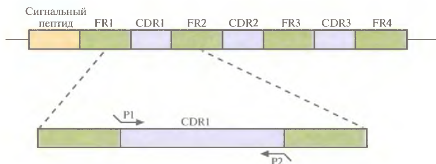
Рис. 10.11. ПЦР-амплификация CDR1-участка, входящего в состав кДНК L-цепи моноклонального антитела грызуна. Олигонуклеотидные праймеры P1 и P2 комплементарны последовательностям ДНК CDR1-участка антитела грызуна. Кроме того, каждый праймер содержит на 5'-конце 12 нуклеотидов, комплементарных каркасным участкам (framework region, FR) кДНК L-цепи антитела человека. Используя шесть пар олигонуклеотидных праймеров — три для V_L - и три для V_H -областей, — с помощью ПЦР амплифицировали отдельно каждый из ДНК-сегментов, кодирующих CDR-участки антитела грызуна. Затем, используя олигонуклеотид-направленный мутагенез, заменили ими соответствующие сегменты генов антитела человека. Такая замена оказалась возможной благодаря тому, что амплифицированные фрагменты содержали участки, комплементарные каркасным областям гена антитела человека.
