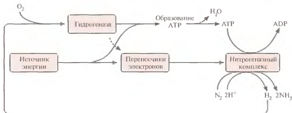
Рис. 14.5. Рециркуляция газообразного водорода — побочного продукта фиксации азота. Нитрогеназа катализирует образование водорода, используя энергию гидролиза ATP, а гидрогеназа катализирует его утилизацию.
