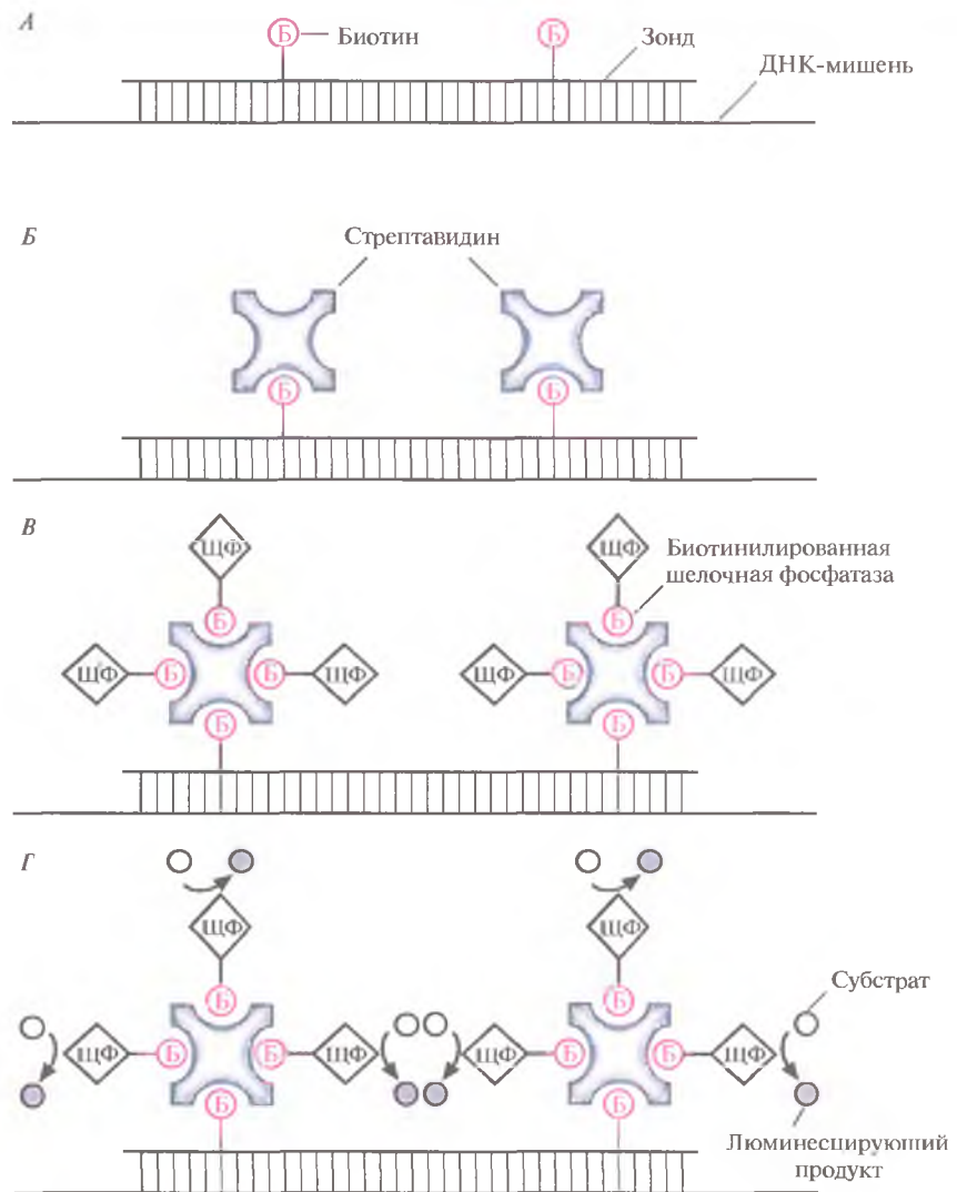
Рис. 9.4. Хемилуминесцентный метод обнаружения ДНК-мишени. Б – биотин, ЩФ – щелочная фосфатаза. А. Связывание биотинилированного зонда с ДНК-мишенью. Б. Связывание стрептавидаина с биотином. В. Связывание биотинилированной щелочной фосфатазы со стрептавидином. Г. Образование люминесцирующего продукта под действием щелочной фосфатазы.
