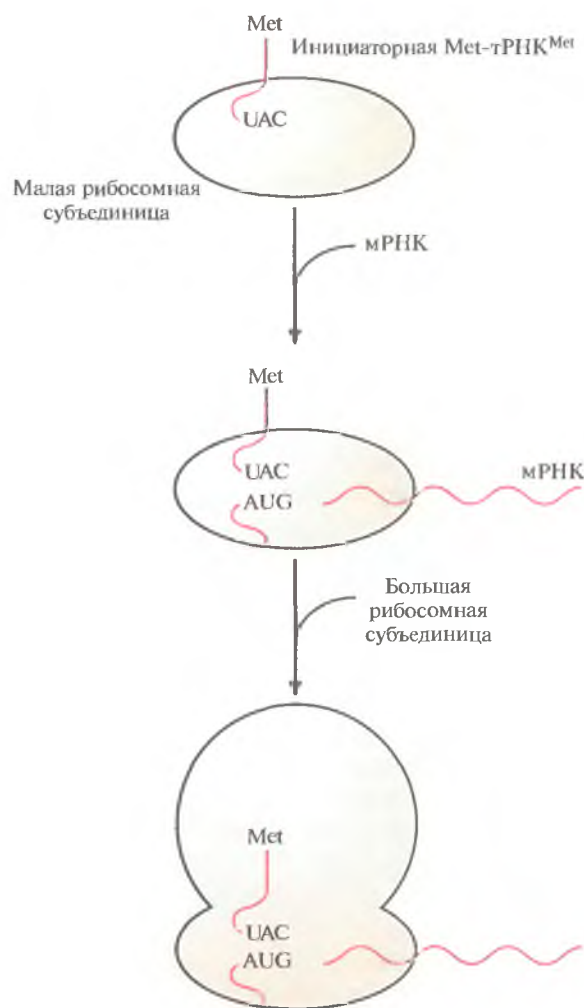
Рис. 3.16. Инициация трансляции в эукариотической клетке. Малая рибосомная субъединица связывается с инициаторной тРНК, «нагруженной» метионином ( \text{Met-tRNA}^{\text{Met}} ), комплекс продвигается по мРНК, пока антикодон UAC инициаторной тРНК не спарится со старт-кодоном AUG мРНК. Далее к комплексу мРНК—тРНК—малая субъединица присоединяется большая субъединица и образуется комплекс инициации.
