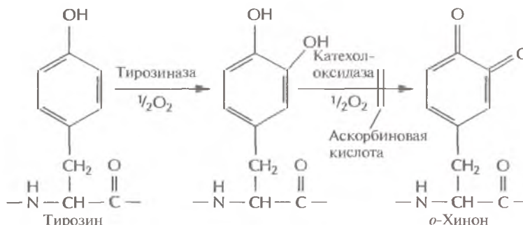
Рис. 12.21. Посттрансляционное гидроксилирование in vitro некоторых тирозиновых остатков адгезивного белка M. edulis . При участии тирозиназы тирозин превращается в DOPA, после чего он может быть окислен до o -хинона катехолоксидазой или тирозиназой. Окисление можно предотвратить добавлением аскорбиновой кислоты.
