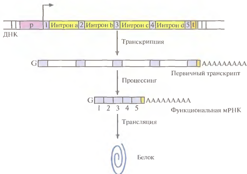
Рис. 3.11. Схематическое изображение эукариотического структурного гена. Указаны промотор (р), сайт инициации транскрипции и ее направление (горизонтальная стрелка), область терминирования транскрипции, узнаваемая РНК-полимеразой (t). 1–5 – экзоны, а–d – интроны. Первичный транскрипт содержит poly(A)-«хвост» на 3'-конце и метилированный нуклеотид G («кэп») на 5'-конце. После транскрипции интроны из первичного транскрипта вырезаются (процессинг), и на образовавшейся функциональной РНК синтезируется белковая молекула (трансляция).
