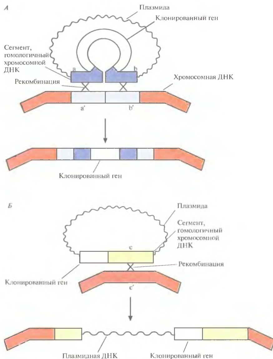
Рис. 6.15. Два способа интеграции клонированного в плазмиде гена в хромосому. А. Ген встроен в середину клонированного в плазмиде сегмента ab , гомологичного сегменту a'b' в хромосомной ДНК. В результате двойного кроссинговера (X-X) клонированный ген оказывается в составе хромосомы. Б. Ген встроен вблизи клонированного в плазмиде сегмента c , гомологичного сегменту c' в хромосомной ДНК. В результате одиночного кроссинговера (X) происходит интеграция в хромосому всей плазмиды вместе с включенным в нее геном.
