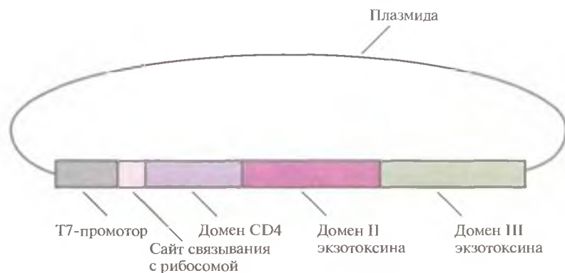
Рис. 10.17. Генетически сконструированный химерный комплекс CD4-экзотоксин А Pseudomonas . Использован промотор бактериофага T7 E. coli .
