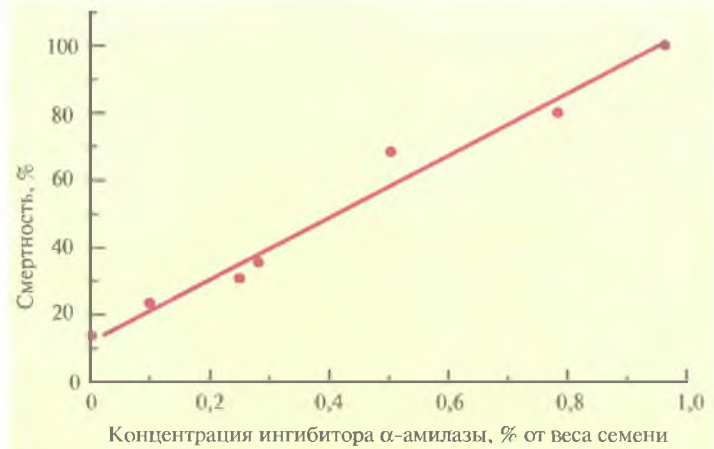
Рис. 18.4. Зависимость смертности личинок зерновки, развивающихся на трансгенных растениях гороха, от количества ингибитора α-амилазы, синтезируемого растениями.
