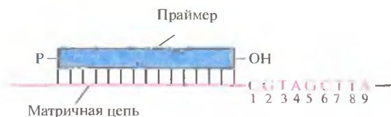
Рис. 5.13. Остановка синтеза ДНК после присоединения дидеозинуклеотида к концу растущей цепи. Фосфодиэфирная связь между концевым дидеозинуклеотидом и следующим нуклеотидом не может образоваться из-за отсутствия 3'-гидроксильной группы.
