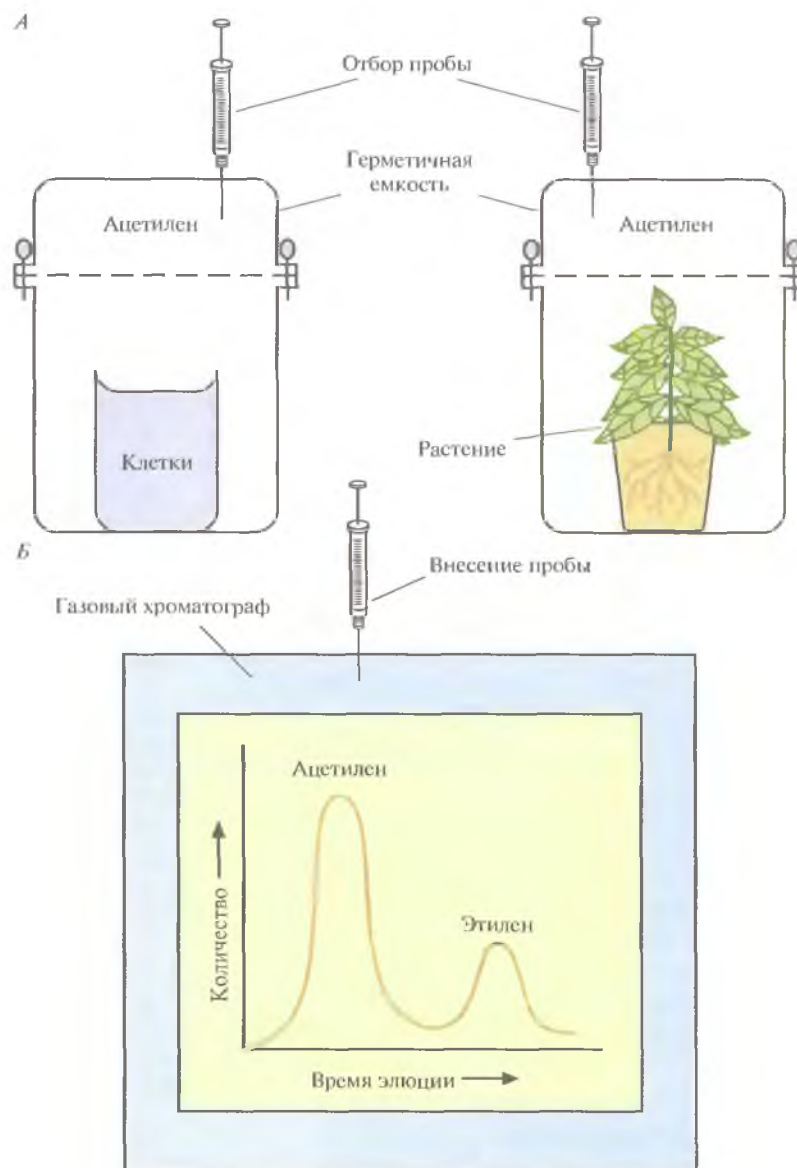
Рис. 14.2. Определение активности нитрогеназы по восстановлению ацетилена до этилена. А. Бактерии (в культуре или ассоциированные с корнями растения), синтезирующие нитрогеназу, либо препарат очищенного фермента (не показано) помещают в герметичную емкость в атмосферу ацетилена. Б. Из емкости периодически отбирают пробы и методом газовой хроматографии измеряют количество ацетилена и этилена. Активность нитрогеназы пропорциональна количеству образовавшегося этилена.
