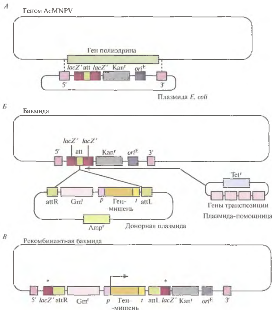
Рис. 7.12. Получение рекомбинантной бакмиды. А. Плазмиду E. coli встраивают в геном АсМNPV с помощью двойного кроссингвера (пунктирные линии) между сегментами ДНК (5' и 3'), фланкирующими ген полиэдрина, с образованием челночного вектора, способного к репликации как в E. coli , так и в клетках насекомых. Встраиваемая плазмидная ДНК содержит ген устойчивости к канамицину ( Kan r ), сайт интеграции ( att ), клонированный без нарушения рамки считывания в последовательности lacZ' , и сайт инициации репликации E. coli ( ori E ). Б. Фрагмент донорной плазмиды, ограниченный двумя сайтами интеграции ( attR и attL ) и несущий ген устойчивости к гентамицину ( Gm r ) и ген-мишень под контролем промотора ( p ) и сайта терминации транскрипции ( t ) гена полиэдрина, встраивают в сайт интеграции ( att ) бакмиды с помощью белков транспозиции, кодируемых плазмидой-помощницей. Плазмида-помощница и донорная плазмида несут гены устойчивости к тетрациклину ( Tet r ) и ампициллину ( Amp r ) соответственно. В. Рекombинантная бакмида содержит дефектный ген lacZ' (*). Угловой стрелкой обозначен сайт инициации транскрипции клонированного гена после трансфекции клеток насекомого рекомбинантной бакмидой.
