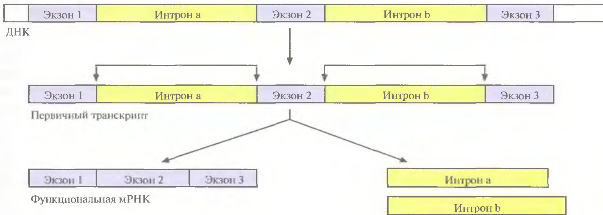
Рис. 3.12. Сплайсинг первичного транскрипта у эукариот. Угловыми стрелками указаны места соединения экзонов 1, 2 и 3 после удаления интронов а и б.
