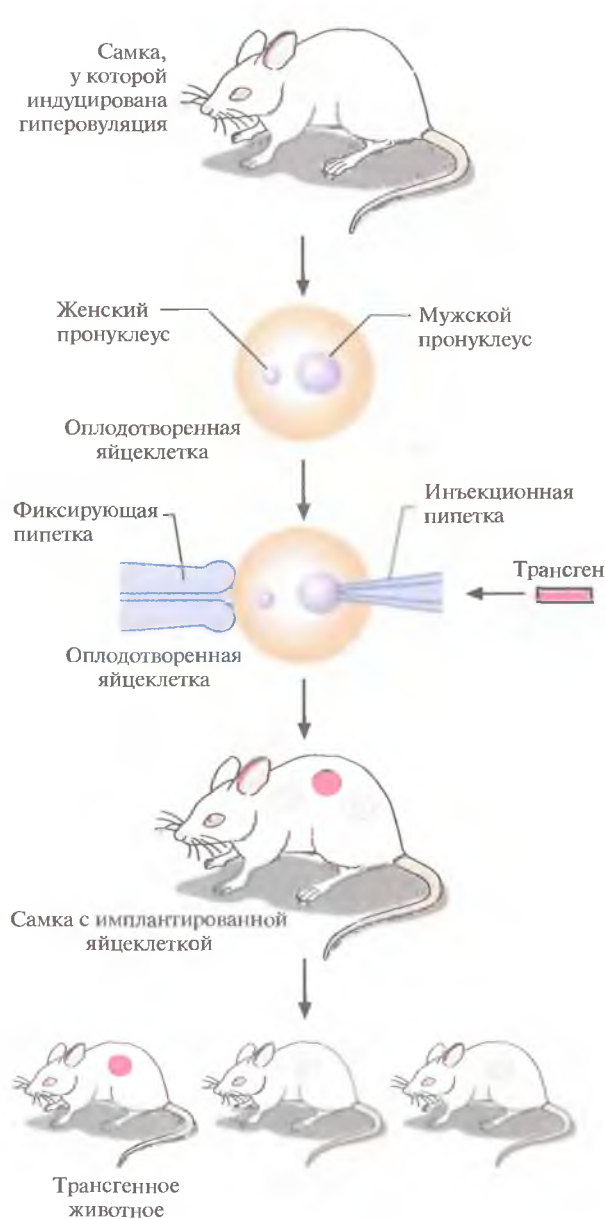
Рис. 19.2. Получение линий трансгенных мышей методом микроинъекций. Яйцеклетки выделяют из самок-доноров, у которых была индуцирована гипероуляция и проведено спаривание с самцами. Трансгенную конструкцию инъецируют в мужской пронуклеус оплодотворенной яйцеклетки. Яйцеклетки имплантируют в «суррогатную» мать, которая производит на свет трансгенных мышат — основателей трансгенных линий.
