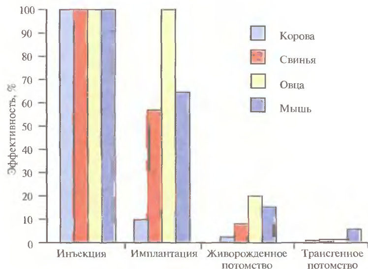
Рис. 19.3. Суммарная эффективность трансгеноза после микроинъекций. Все оплодотворенные яйцеклетки (100%) коровы, свиньи, овцы и мыши инокулировали трансгеном, однако успешная имплантация и появление потомства были редкими событиями: трансгенное потомство давали менее 5% обработанных яйцеклеток.
