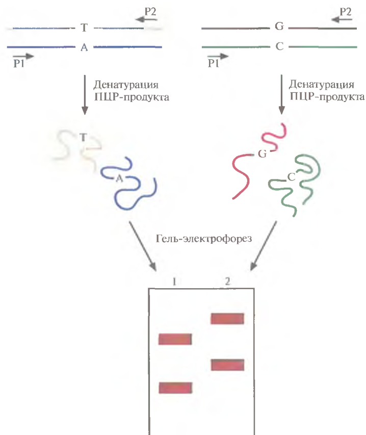
Рис. 20.22. Анализ конформационного полиморфизма одноцепочечной ДНК (SSCP). Препараты ДНК, различающихся одной парой нуклеотидов ( A:T \leftrightarrow G:C ), амплифицируют ПЦР-методом с использованием одинаковых праймеров (P1, P2). ПЦР-продукты денатурируют и разделяют с помощью гель-электрофореза на двух дорожках (1, 2). Расстояние, на которое перемещается одноцепочечная молекула ДНК, зависит от ее конформации, а последняя, в свою очередь, — от нуклеотидной последовательности. Даже если ДНК различаются лишь одним нуклеотидным сайтом, одиночные цепи могут иметь разную конформацию, а следовательно, ПЦР-продукты образуют в геле не две, а четыре полосы.
