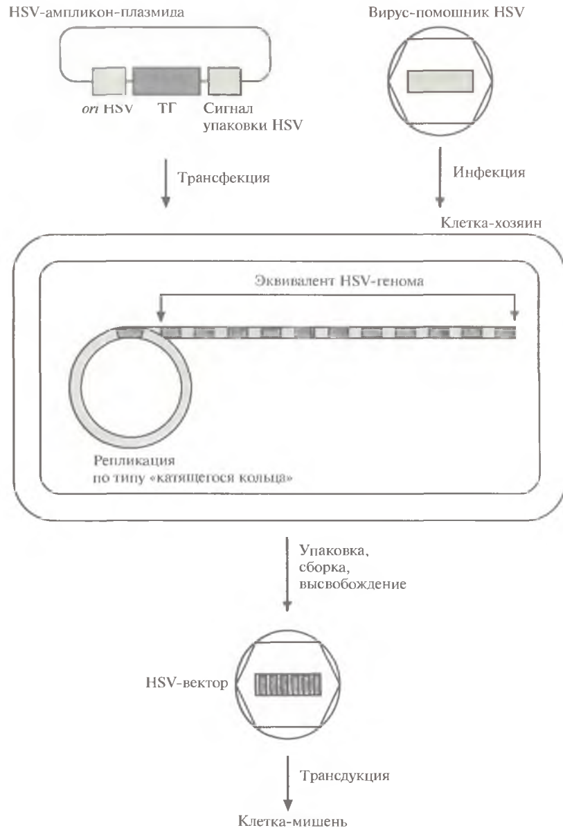
Рис. 21.9. Вектор на основе HSV-ампликон-плазмиды. Точка инициации репликации HSV ( ori HSV), сигнал упаковки HSV и «терапевтический» ген (ТГ) встраивают в плазмиду E. coli (HSV-ампликон-плазмиду). Проводят трансфекцию клетки-хозяина, инфицированной вирусом-помощником HSV, полученной плазмидой. ДНК ампликон-плазмиды реплицируется по типу «катящегося кольца». 10 ампликонов, соответствующих полно-размерному геному HSV, упаковываются в HSV-капсид, который предоставляет вирус-помощник HSV. Геном этого вируса не упаковывается. HSV-частицы, несущие множество копий «терапевтического» гена, высвобождаются при лизисе клетки и используются для трансдукции нейронов.
