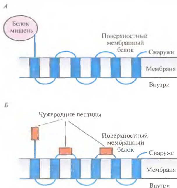
Рис. 6.10. Химерные белки, состоящие из поверхностного бактериального белка и чужеродного белка-мишени, присоединенного к его N- или С-концу (А) либо включенного в экспонируемые участки молекулы (Б). В обоих случаях чужеродные пептиды или белок оказываются на поверхности бактериальной клетки.
