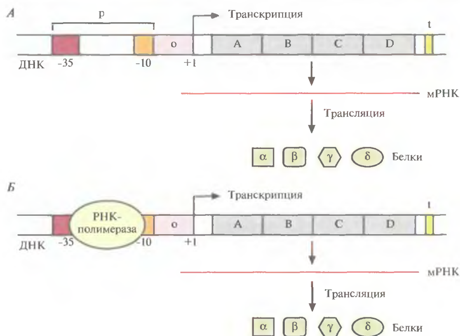
Рис. 3.19. Транскрипция в бактериальной клетке. А. Структурные гены (A, B, C и D) оперона находятся под транскрипционным контролем оператора (o) и промотора (p). РНК-полимераза связывается с участками, находящимися на расстоянии 10 (–10) и 35 (–35) пар оснований от сайта инициации транскрипции (+1). t – Стоп-сигнал, ответственный за остановку транскрипции. \alpha , \beta , \gamma и \delta – белки, продукты генов A, B, C, D. Б. То же, что и на рис. А, но показано связывание РНК-полимеразы с промоторной областью.
