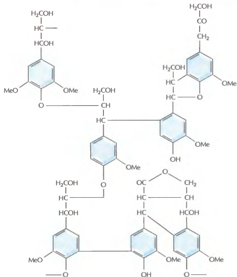
Рис. 13.13. Структура лигнина. Представлены лишь некоторые из возможных способов соединения остатков фенилпропана (шестиуглеродного ароматического соединения, содержащего алькильную группу).
