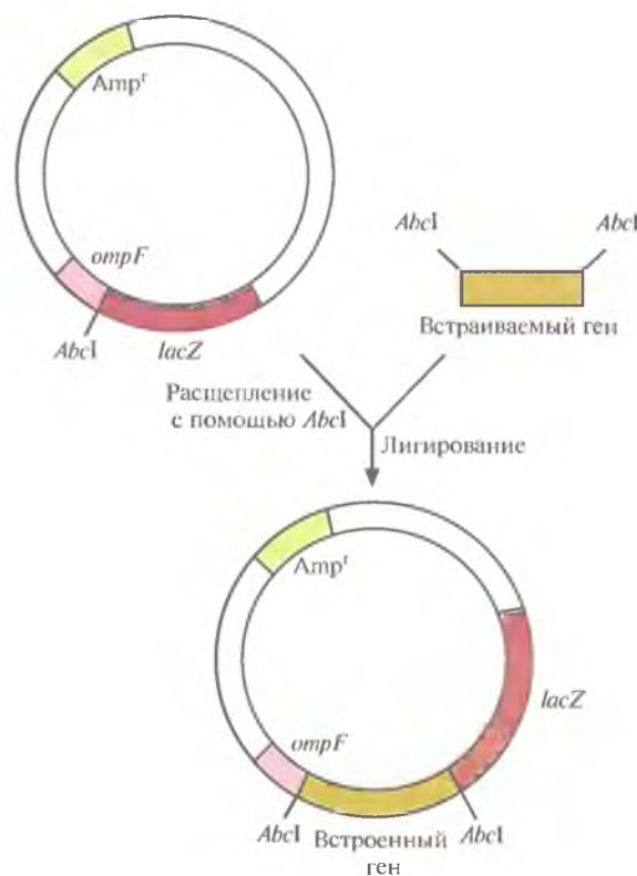
Рис. 6.7. Клонировующий вектор системы слияния. Он содержит ген устойчивости к ампициллину ( Amp^r ) в качестве селективного маркера, 5'-концевой сегмент гена ompF , кодирующий N-конец наружного мембранного белка, сайт для рестрицирующей эндонуклеазы AbcI и укороченный ген \beta -галактозидазы ( lacZ ). Ген, который хотят клонировать, встраивают в AbcI -сайт. После транскрипции и трансляции этой генетической конструкции образуется трехкомпонентный химерный белок.
