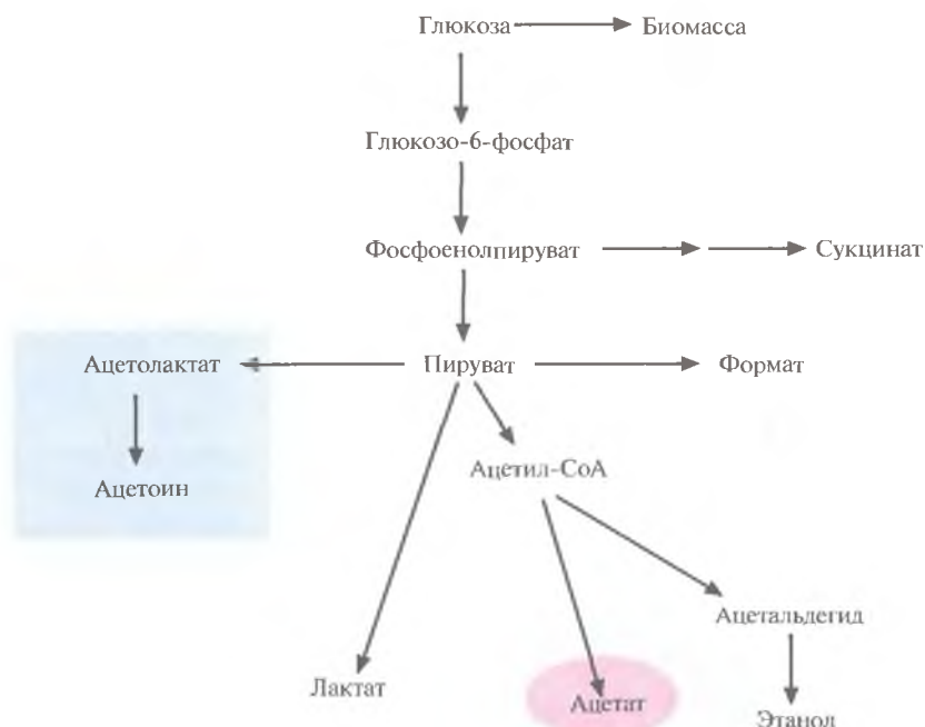
Рис. 6.17. Схематическое представление метаболизма глюкозы в клетках E. coli , трансформированных плазмидой, несущей ген ацетолактатсинтазы.
