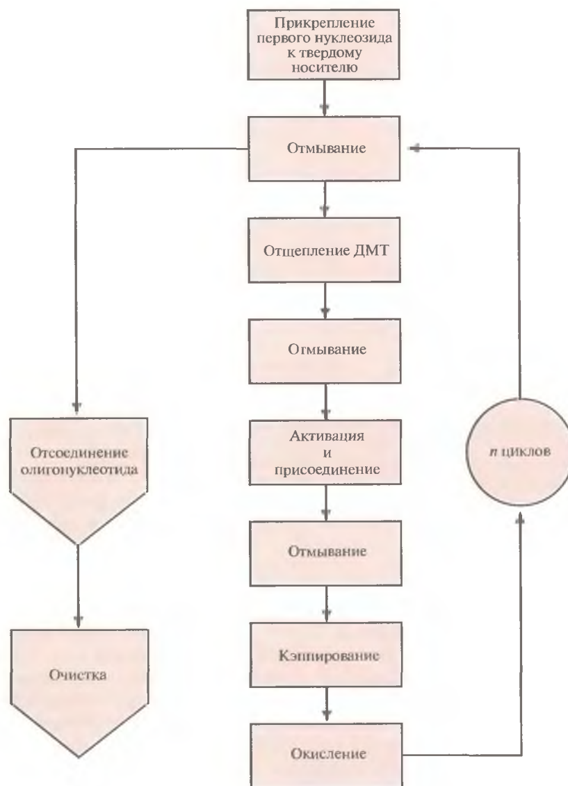
Рис. 5.1. Химический синтез олигонуклеотида. После n циклов образуется одноцепочечный фрагмент ДНК из n + 1 нуклеотида.
