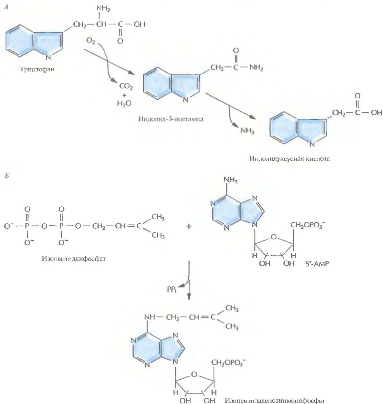
Рис. 17.4. Биосинтез ауксина и цитокинина при участии ферментов, кодируемых генами Т-ДНК Ti -плазмиды A. tumefaciens . А. Синтез ауксина начинается с превращения триптофана в индол-3-ацетамид, катализируемого триптофанмонооксигеназой. Затем происходит превращение индолил-3-ацетамида в индолилуксусную кислоту ферментом индолил-3-ацетамидгидролазой. Б. Синтез цитокинина включает присоединение изопентенильной группы изопентенилдифосфата к 5'-АМР при участии фермента изопентенилтрансферазы с образованием изопентениладенозинмонофосфата.
