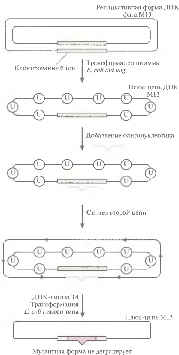
Рис. 8.2. Повышение выхода мутантного фага M13 путем трансформации штамма E. coli dut ung . Ген-мишень встраивают в двухцепочечную репликативную форму ДНК фага M13 и полученными молекулами трансформируют штамм E. coli dut ung . Мутация dut вызывает повышение содержания dUTP в клетке, что приводит к включению в ДНК нескольких остатков dUTP (U), а мутация ung блокирует их удаление. Двухцепочечной ДНК M13, содержащей ген-мишень, трансформируют клетки E. coli дикого типа. Продукт гена ung дикого типа (урацил-N-гликозилаза) удаляет все остатки урацила из исходной цепи, и она деградирует. Мутантная цепь остается интактной, поскольку она не содержит остатков урацила. Эта цепь служит матрицей для репликации ДНК, и в результате доля фаговых частиц, несущих мутантный ген, увеличивается.
