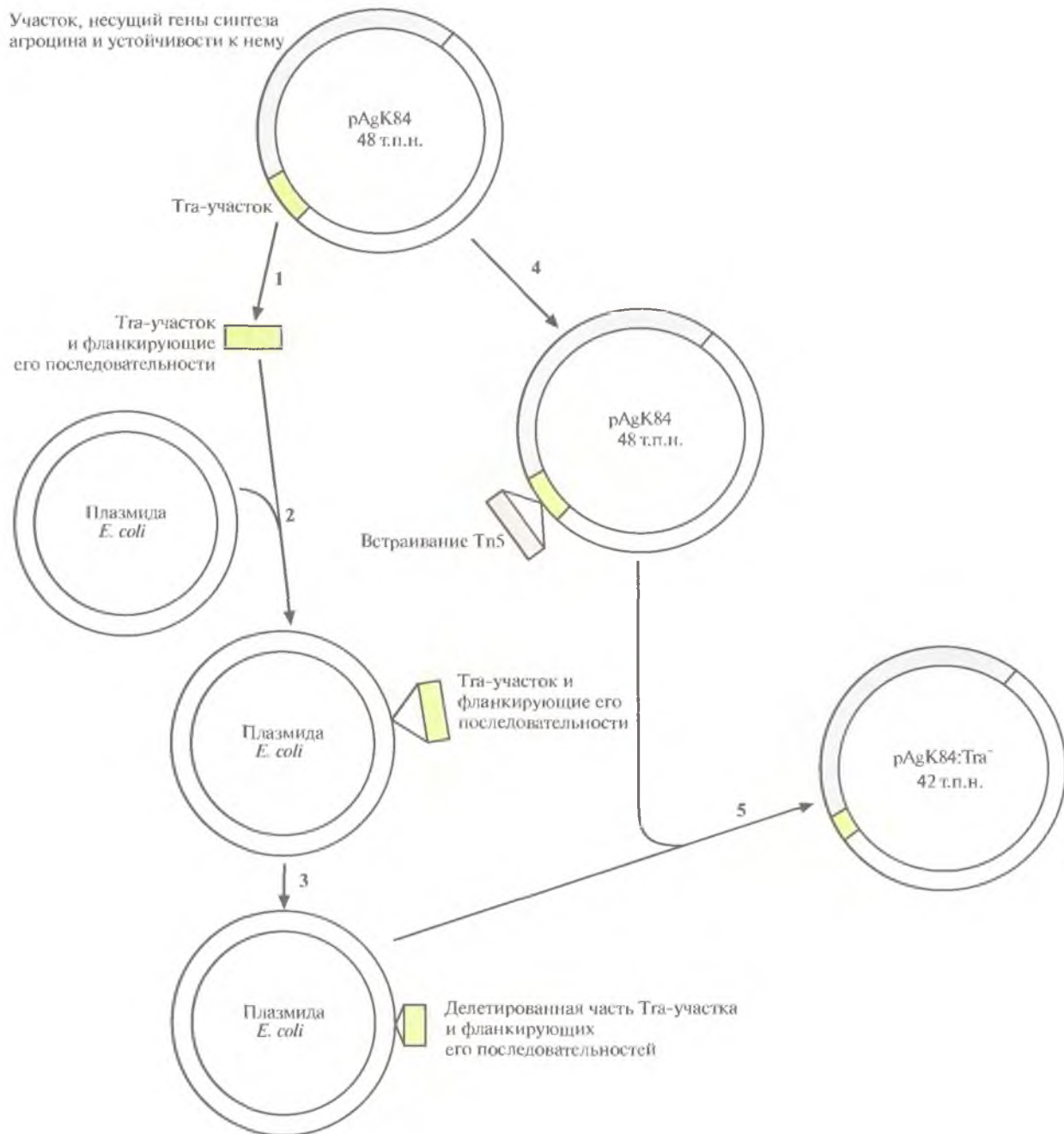
Рис. 14.9. Конструирование неспособной к переносу (Tra - ) модификации плазмиды pAgK84 A. radiobacter , кодирующей гены биосинтеза агроцина 84 и гены устойчивости к нему. Используя рестрикционную карту pAgK84, из плазмиды вырезали (1) фрагмент, который содержал участок Tга, ответственный за перенос, вместе с фланкирующими его последовательностями, и встроили его в плазмиду E. coli (2). С помощью рестриктазной обработки из клонированного фрагмента удалили примерно 80% Tга-участка и часть фланкирующих его последовательностей (в сумме примерно 6 т.п.н.) (3). Осуществили гомологичную рекомбинацию между плазмидой E. coli , содержащей «урезанный» Tга-участок, и плазмидой pAgK84, которая содержала встроенный в Tга-участок транспозон Tn5 с геном устойчивости к канамицину (4). Получили несколько производных плазмиды pAgK84 с частично удаленным Tга-участком (5). Tга - -плазмида pAgK84 больше не могла передаваться другой агробактерии в ходе конъюгации, но все еще была способна детерминировать синтез агроцина 84 и обеспечивать устойчивость к нему. Рисунок выполнен без соблюдения масштаба.
