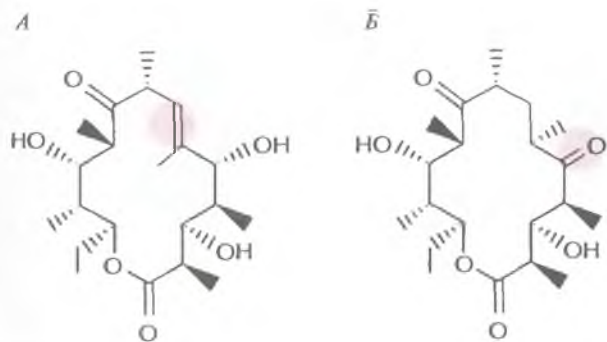
Рис. 12.14. Производные эритромицина, полученные генноинженерными методами. А. В результате мутации в гене еноилредуктазы образуется продукт с двойной связью между атомами С-6 и С-7 (цветной кружок). Б. Делеция гена β-кеторедуктазы сопровождается образованием производного с С-5-карбонильной, а не гидроксильной группой (цветной кружок). (По данным работы Kutz, Donadio, Annu. Rev. Microbiol. 47: 875–912, 1993.)
