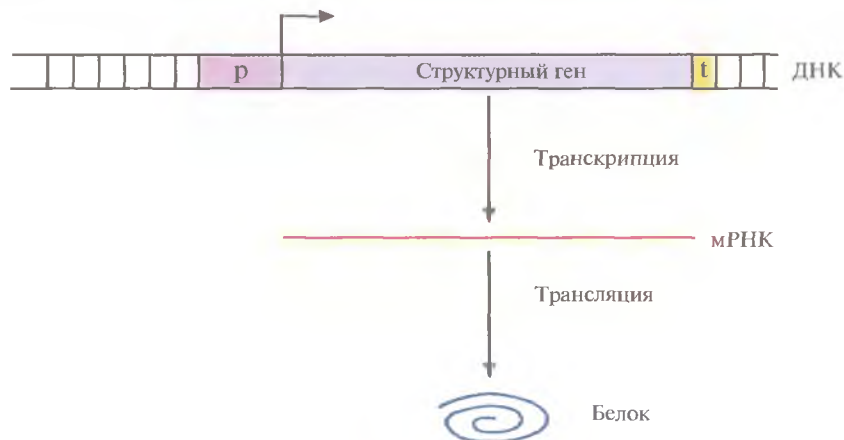
Рис. 3.10. Схематическое изображение прокариотического структурного гена. Указаны промотор (р), сайт инициации транскрипции и ее направление (горизонтальная стрелка), область терминирования транскрипции, узнаваемая РНК-полимеразой (t). Сначала на ДНК как на матрице синтезируется мРНК (транскрипция), а затем осуществляется синтез белковой цепи (трансляция).
