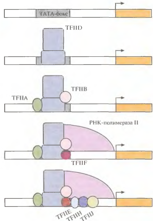
Рис. 3.24. Инициация транскрипции структурного гена эукариот. Сначала фактор транскрипции TFIID связывается с ТАТА-боксом, затем происходит присоединение других факторов транскрипции и РНК-полимеразы II и, наконец, вспомогательных факторов, запускающих транскрипцию. Стрелка — направление транскрипции.
