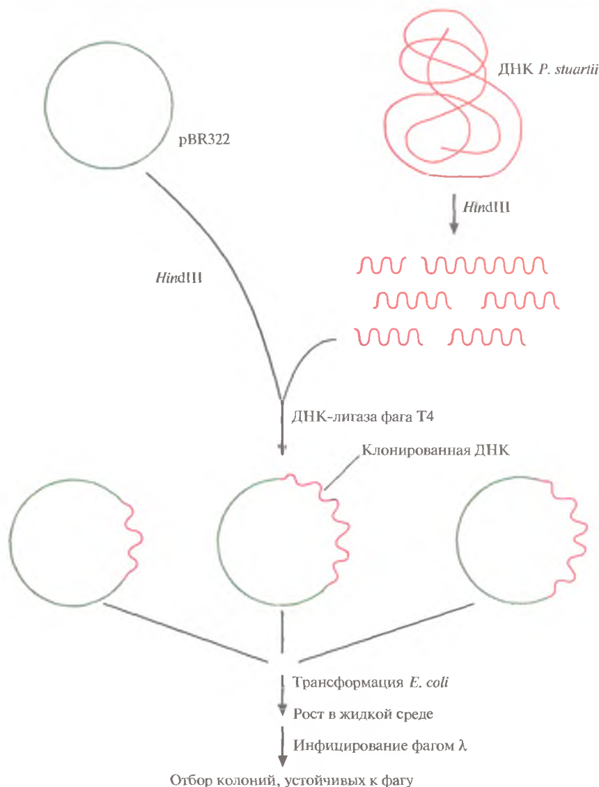
Рис. 12.1. Клонирование гена рестриктазы PstI и отбор несущих его трансформированных бактериальных клеток. Хромосомную ДНК P. stuartii расщепляют HindIII и встраивают фрагменты в плазмиду pBR322. Трансформируют рекомбинантной плазмидой E. coli , выращивают клетки в жидкой среде и инфицируют фагом \lambda . Отбирают трансформанты, устойчивые к фагу; именно они несут и экспрессируют клонированный ген PstI .
