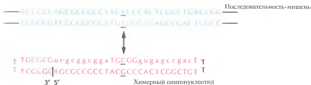
Рис. 21.16. Исправление генетического дефекта, состоящего в замене одной пары нуклеотидов, с помощью химерного олигонуклеотида. Стрелкой указаны мутантный сайт в последовательности-мишени и нормальная пара оснований в химерном олигонуклеотиде. Соответствующие нуклеотиды подчеркнуты. Прописными буквами обозначены дезоксирибонуклеотиды, а строчными — рибонуклеотиды. Жирным шрифтом выделены нуклеотиды, образующие головки шпильки. Вертикальная черта указывает 3'- и 5'-концы химерного олигонуклеотида. (Из работы Yoon et al., Proc. Natl. Acad. Sci. USA 93: 2071–2076, 1996, с изменениями.)
