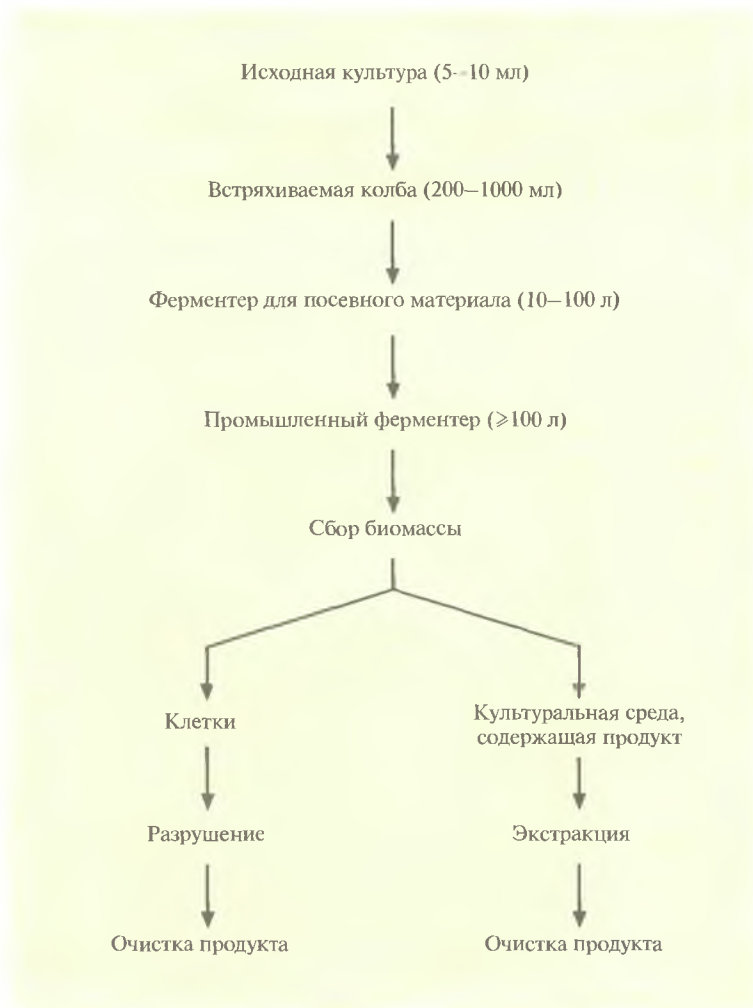
Рис. 16.1. Обобщенная схема процесса промышленной ферментации. Выделяемый продукт находится либо в клетках, либо в культуральной среде, но не в обеих фракциях одновременно, так что дальнейшие манипуляции проводят с одной из этих фракций.
