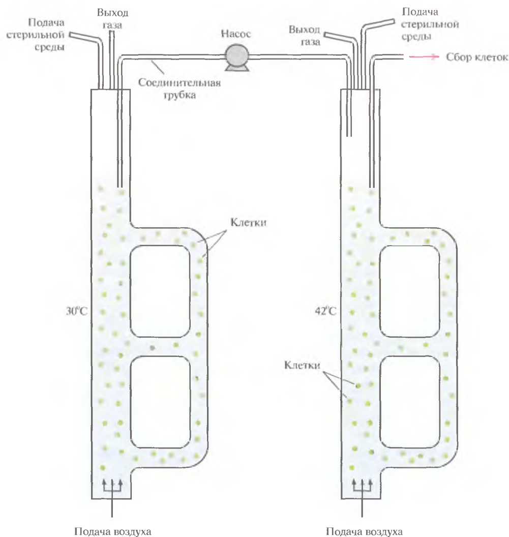
Рис. 16.5. Система из двух эрлифтных биореакторов, использующаяся для температурной индукции синтеза белкового продукта. Из ферментера, в котором осуществляется культивирование при 30 °С (слева), клетки поступают в ферментер с температурой 42 °С (справа), где происходит индукция. У обоих биореакторов имеется двойное внешнее рециркуляционное устройство, оснащенное задвижками. Изменяя положение задвижек, можно создавать рабочий объем, оптимальный для данных условий.
