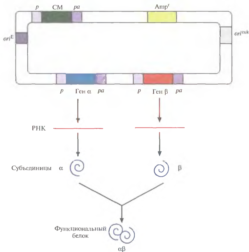
Рис. 7.16. Экспрессирующий вектор с двумя независимо транскрибируемыми генами. Клонированные гены ( \alpha и \beta ) кодируют субъединицы димерного белка ( \alpha\beta ). Каждый ген встроен в вектор как часть отдельной единицы транскрипции и находится под контролем эукариотического промотора ( p ) и сигнала полиаденилирования ( pa ). Каждая субъединица транслируется со своей мРНК; объединяясь, субъединицы образуют функциональный димерный белок ( \alpha\beta ). Векторы содержат сайты инициации репликации, функционирующие в E. coli ( ori^E ) и в клетках млекопитающих ( ori^{euk} ); маркерный ген ( Amp^r ) для отбора трансформированных клеток E. coli ; селективный маркерный ген (CM), находящийся под контролем эукариотических промотора ( p ) и сигнала полиаденилирования ( pa ).
