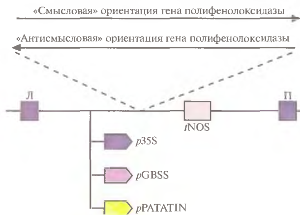
Рис. 18.18. Конструкции со «смысловой» и «антисмысловой» ориентациями гена полифенолоксидазы. Транскрипция в обоих случаях осуществлялась под контролем одного из промоторов: 35S-промотора вируса мозаики цветной капусты ( p35S ), промотора гена синтазы гранулосвязанного крахмала ( pGBSS ) или промотора гена пататина I ( pPATATIN ), а также сигнала терминации транскрипции гена нопалинсинтазы ( iNOS ). Л и П — левая и правая фланкирующие последовательности Т-ДНК соответственно. (По данным работы Bachem et al., Bio/Technology 12: 1101–1105, 1994.)
