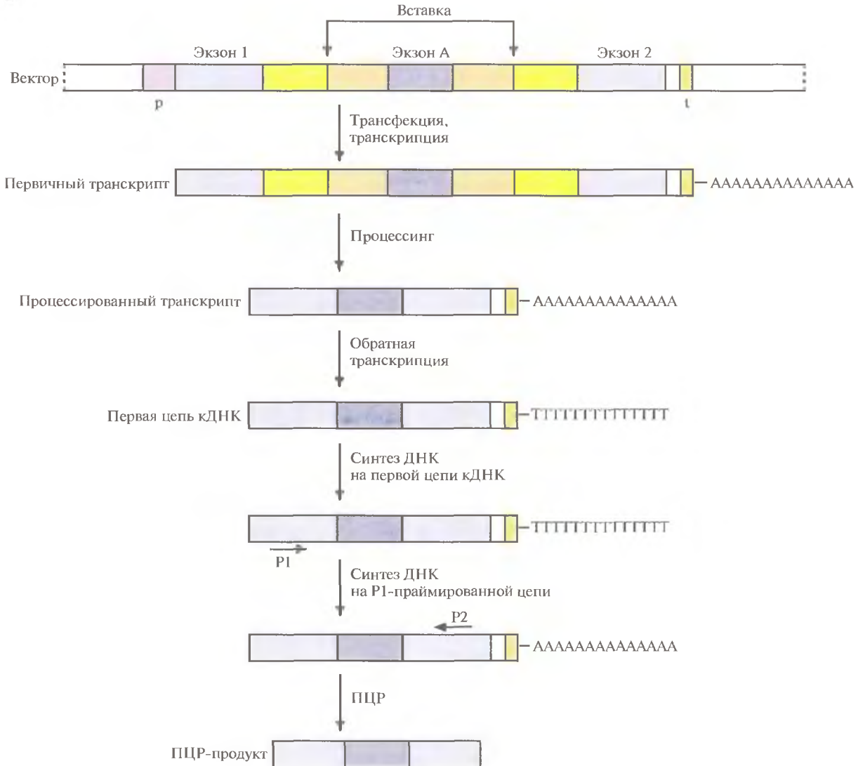
Рис. 20.29. (Продолжение) Б. В полилинкер вектора для улавливания экзонов встроен фрагмент ДНК человека, и эта конструкция введена в эукариотическую клетку (трансфекция). В данном случае экзон содержит функциональные акцепторный и донорный сайты сплайсинга. При процессинге первичного транскрипта удаляются интроны, фланкирующие экзон А, и он оказывается между экзонами 1 и 2. Длина ПЦР-продукта обратного транскрипта показывает, «пойман» ли искомым экзон между экзонами 1 и 2 и, следовательно, содержит ли его данная вставка.
