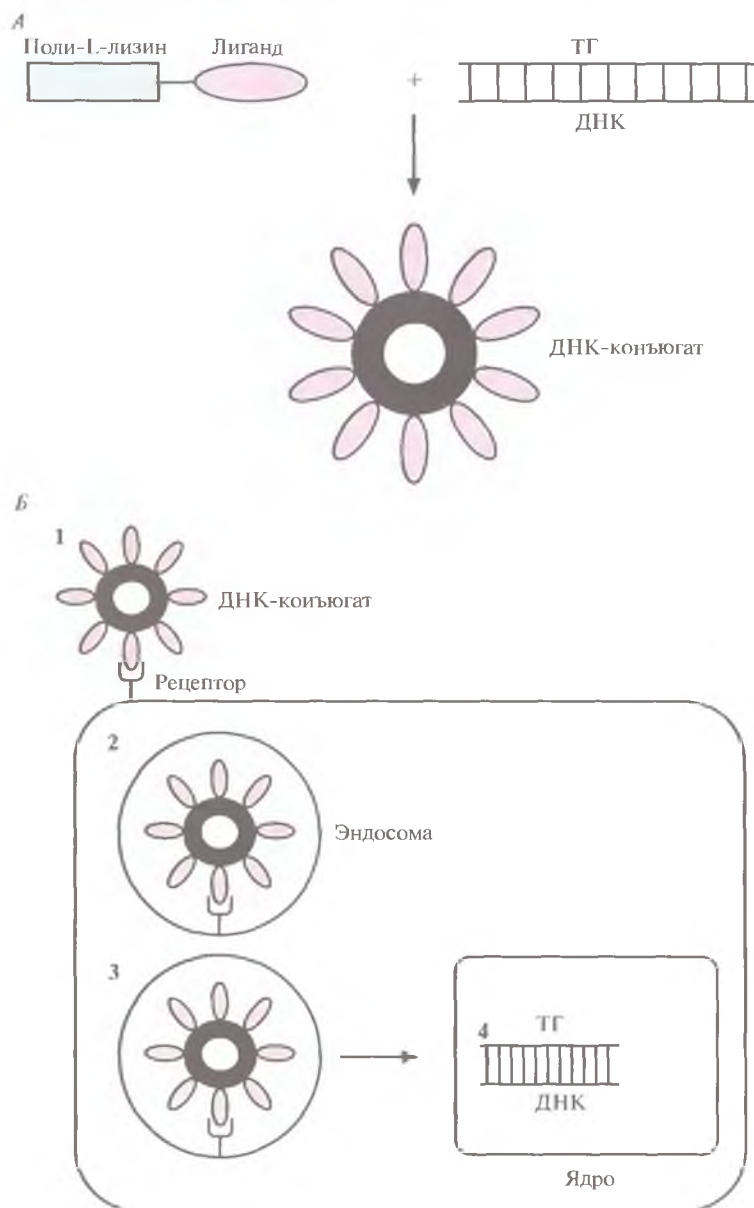
Рис. 21.11. Система доставки «терапевтических» генов с использованием ДНК-конъюгата. А. К поли-L-лизину пришивают лиганд, соединяющийся с поверхностным клеточным рецептором, и добавляют ДНК, содержащую «терапевтический» ген. В результате образуется конденсированная структура, на поверхности которой располагаются лиганды. Б. ДНК-конъюгат связывается со специфическим клеточным рецептором (1) и обволакивается клеточной мембраной (2) с образованием эндосомы (3), которая защищает его от лизосом. В эндосоме часть молекул ДНК высвобождается из конъюгата и проникает в ядро клетки (4), где и происходит экспрессия «терапевтического» гена.
