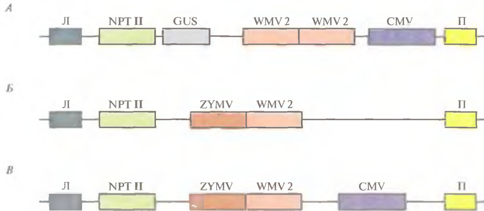
Рис. 18.8. А. Т-ДНК, несущая ген неомифосфотрансферазы (NPT II) в качестве селективного маркера, ген \beta -глюкуронидазы (GUS) в качестве репортерного гена, две копии гена белка оболочки вируса 2 мозаики арбуза (WMV2) и ген белка оболочки вируса мозаики огурца (CMV). Левая и правая фланкирующие последовательности Т-ДНК обозначены Л и П соответственно. Б. Конструкция, аналогичная конструкции А, но без CMV и NPT II, содержащая одну копию WMV2 и ген белка оболочки вируса желтой мозаики кабачков (ZYMV). В. Конструкция, аналогичная конструкции Б, но содержащая CMV. Во всех трех конструкциях присутствуют соответствующие промоторы и сигналы термации транскрипции.
