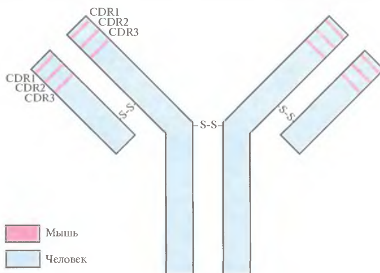
Рис. 10.10. Полученное методом генной инженерии антитело, сходное по своей структуре с антителом человека. Сегменты ДНК, кодирующие CDR-участки (CDR1, CDR2 и CDR3) антитела человека, заменены на последовательности, кодирующие CDR-участки H- и L-цепей иммуноглобулина мыши. Продуктом этого рекомбинантного гена является иммуноглобулин с антигенсвязывающей специфичностью моноклонального антитела мыши (участки, выделенные розовым цветом) и остальными свойствами антитела человека (участки, выделенные голубым цветом).
