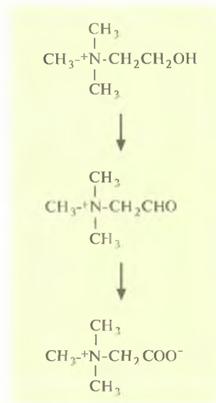
Рис. 18.13. Превращение холина в бетаин.
