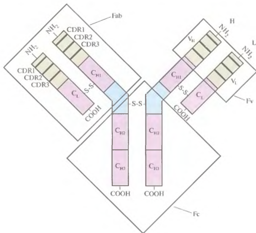
Рис. 10.5. Строение молекулы антитела. Н- и L-цепи состоят из переменных ( V_H и V_L ) и константных ( C_L , C_{H1} , C_{H2} и C_{H3} ) доменов. Переменные домены содержат CDR-участки (CDR1, CDR2 и CDR3).
