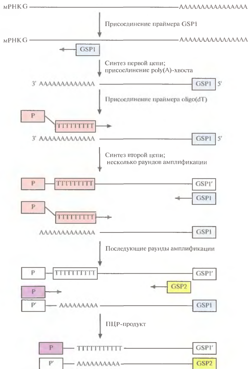
Рис. 5.23. ПЦР-амплификация кДНК, комплементарной 5'-концевой части мРНК первой цепи, осуществляемая обратной транскриптазой, иницируется праймером GSP. Затем к этой цепи с помощью концевой дезоксирибонуклеотидилтрансферазы присоединяется poly(A)-хвост. Для синтеза второй цепи в качестве праймера используется oligo(dT). Проводят несколько раундов амплификации при участии указанных праймеров, добавляют вторые праймеры (GSP2 и P) и получают кДНК, отвечающую 5'-концу мРНК.
