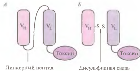
Рис. 10.15. Схематическое изображение одноцепочечного Fv-иммунотоксина (А) и Fv-иммунотоксина, стабилизированного дисульфидной связью (Б).
