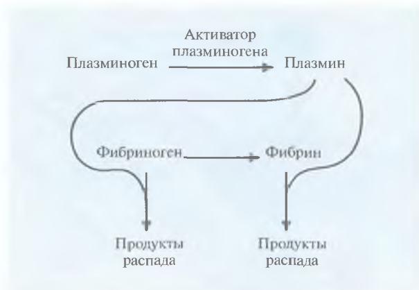
Рис. 10.7. Активация плазминогена с превращением его в плазмин и разрушение плазмином двух субстратов (фибриногена и фибрина) в крови.
