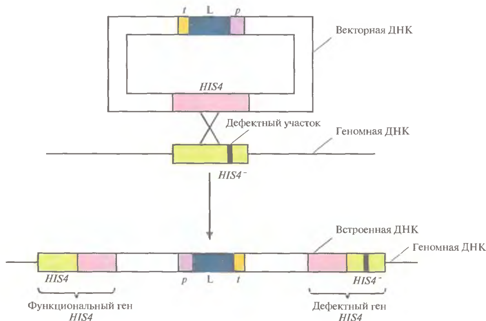
Рис. 7.7. Интеграция экспрессирующего плазмидного вектора в дефектный хромосомный ген HIS4 - P. pastoris . В результате кроссинговера между плазмидным геном HIS4 и геном HIS4 - клетки-хозяина происходит интеграция в геном всей плазмиды, которая оказывается фланкированной функциональным и дефектным генами HIS4 . p , L и t – промотор AOX1 , кДНК бычьего лизоцима C2 и сигнал терминации транскрипции-полиаденирования соответственно. Черная полоска – дефектный участок в HIS4 - -гене.
