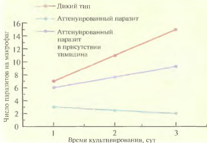
Рис. 11.7. Пролиферация L. major дикого типа и аттенуированного паразита в мышиных макрофагах. Для инвазии в обоих случаях использовали одинаковое количество L. major , находящихся в стационарной фазе. (Из работы Titus et al., Proc. Natl. Acad. Sci. USA 92: 10267–10268, 1995, с изменениями.)
