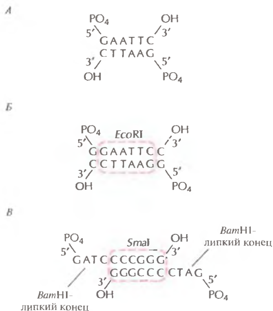
Рис. 5.8. Типичные линкеры и адаптор. А. EcoRI -линкер, состоящий из 6 пар нуклеотидов. Б. EcoRI -линкер из 8 пар нуклеотидов. В. BamHI - SmaI -адаптор с BamHI -липкими концами и сайтом узнавания для SmaI .
