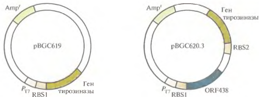
Рис. 12.19. Экспрессирующие плазмиды E. coli , несущие гены биосинтеза меланина. pBGC619 содержит ген тирозиназы, а pBGC620.3 — открытую рамку считывания (ORF438) для синтеза меланина и ген тирозиназы. Транскрипция клонированных генов осуществляется под контролем промотора P_{T7} бактериофага T7. RBS1 и RBS2 — два разных сайта связывания рибосом. Обе плазмиды несут гены устойчивости к ампициллину ( Amp^r ).
