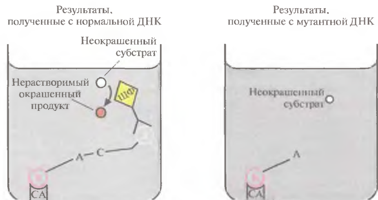
Рис. 9.10. Метод ПЦР/ЛОЗ. Б – биотин; Д – дигоксигенин; ЩФ – щелочная фосфатаза; СА – стрептавидин.
