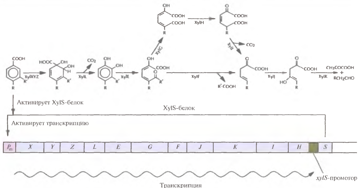
Рис. 13.6. Путь мета -расщепления толуола и ксилола и xyl -оперон плазмиды pWWO. xyl -Оперон находится под контролем P_m -промотора, который регулируется с помощью продукта гена xylS , в свою очередь активируемого одним из исходных субстратов. Гены xylX – xylH находятся под контролем P_m -промотора. Ген xylS не входит в состав оперона и экспрессируется конститутивно. Исходным субстратом может быть бензоат (R и R' – это H), 3-метилбензоат (R – это H, R' – это CH 3 ), 3-этилбензоат (R – это H, R' – это CH 2 CH 3 ) и 4-метилбензоат (R – это CH 3 , R' – это H). Гены xylXYZ кодируют толуолдиоксигеназу, xylL – дигидроксициклогексадиенкарбоксилатдегидрогеназу, xylE – катехол-2,3-диоксигеназу, xylF – гидролазу полуальдегида гидроксимуконной кислоты, xylG – дигидрогеназу полуальдегида гидроксимуконной кислоты, xylH – 4-оксало-кродонат-таутомеразу, xylI – 4-оксало-кродонатдекарбоксилазу, xylJ – 2-оксопента-4-еноатгидратазу, xylK – 2-оксо-4-гидроксипентонатальдолазу.
