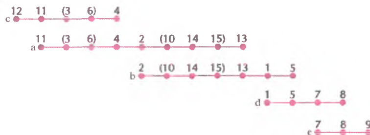
Рис. 20.18. STS-картирование. А. STS (с 1 по 15), обнаруженные с помощью ПЦР-скрининга в клонах а–е, обозначены знаком плюс (+). Буквами L и R указаны STS, находящиеся на 5'- и 3'-концах вставки (на ее левом и правом концах соответственно). Б. Идентифицировав перекрывающиеся участки, можно построить контиг из пяти клонов и карту расположения STS. Полученные данные не позволяют установить порядок некоторых из них (номера в скобках). Интервалы между STS представлены одинаковыми; в действительности они неизвестны.
