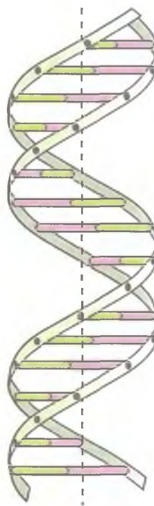
Рис. 3.3. Модель двойной спирали ДНК. Поперечные перекладины — комплементарные пары оснований, «боковины» — сахарофосфатный остов.
