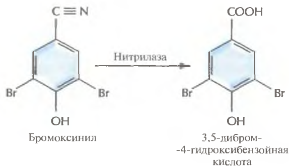
Рис. 18.10. Инактивация гербицида бромоксинила при помощи нитрилазы K. ozaenae .
