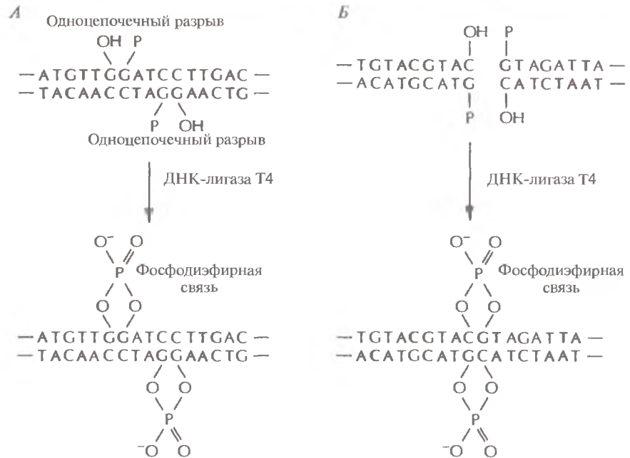
Рис. 4.6. ДНК-лигаза Т4 образует фосфодиэфирные связи между 5'-фосфатными и 3'-гидроксильными группами в месте разрыва в остове двухцепочечной ДНК. А. Лигирование липких концов. Б. Лигирование тупых концов.
