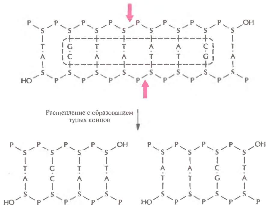
Рис. 4.3. Расщепление короткого фрагмента ДНК рестриктазой типа II HindII с образованием тупых концов. Стрелки — связи, по которым происходит расщепление в сахарофосфатном остове. Буквенные обозначения — те же, что и на рис. 4.2. Последовательность, распознаваемая рестриктазой HindII , выделена штриховой линией.
