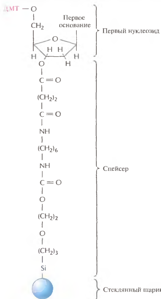
Рис. 5.2. Комплекс, с которого начинается химический синтез цепи ДНК. К 5'-гидроксильной группе дезоксирибозы первого нуклеозида присоединена диметокситритильная (ДМТ) группа, а к 3'-гидроксильной группе — спейсерная молекула. Последняя в свою очередь связана с твердым носителем (пористым стеклянным шариком).
