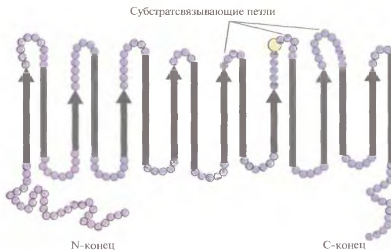
Рис. 12.5. Структура 2,5-DKG-редуктазы, воссозданная исходя из ее аминокислотной последовательности. Стрелки — \beta -слои, полосы — \alpha -спиральные участки, кружки — аминокислотные остатки, находящиеся на N- и С-концах молекулы или соединяющие \beta -слои и \alpha -спирали. Показаны три петли, возможно, участвующие в связывании субстрата. Желтый кружок — 192-й аминокислотный остаток.
