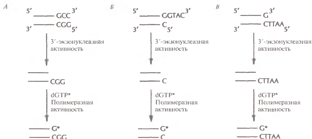
Рис. 20.20. Концевое мечение двухцепочечных ДНК с помощью ДНК-полимеразы Т4. 3'-экзонуклеазная активность ДНК-полимеразы катализирует отщепление 3'-концевых нуклеотидов фрагментов ДНК с тупыми концами (А), с выступающими 3'-концами (Б) или с выступающими 5'-концами (В). Отщепление происходит до тех пор, пока на противоположной цепи не экспонируется основание, комплементарное меченому дезоксирибонуклеотиду, введенному в реакционную смесь (dGTP*); затем «включается» полимеразная активность ДНК-полимеразы Е4, и к 3'-концу присоединяется свободный меченый дезоксирибонуклеотид. Метка включается в оба конца фрагментов ДНК (на рисунке это не показано). Для мечения можно использовать любой дезоксирибонуклеотид.
