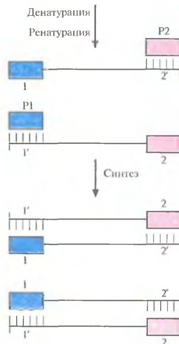
Рис. 5.21. Тридцатый раунд ПЦР. На этом этапе в реакционной смеси содержатся практически одни «короткие матрицы».
