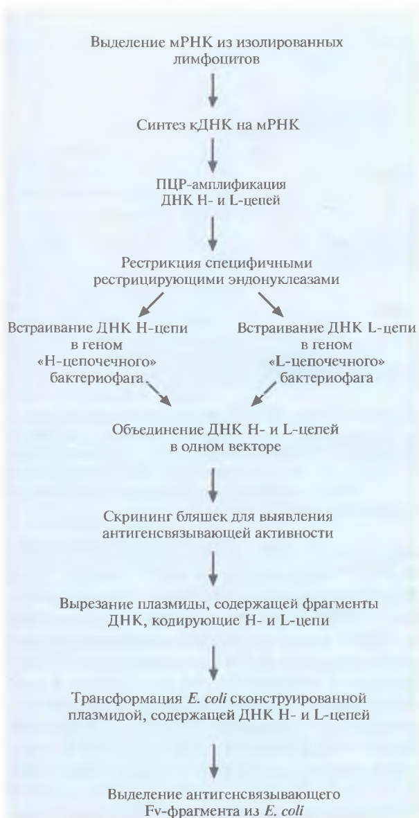
Рис. 10.12. Создание с помощью E. coli комбинаторной библиотеки кДНК V_L - и V_H -областей антитела.
