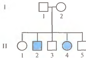
Рис. 20.2. Аутосомно-рецессивный тип наследования. Характерные признаки: 1) у здоровых родителей могут появляться больные дети; 2) лица мужского и женского пола поражаются с одинаковой частотой; 3) если больны оба родителя, то больны и все их дети (эта ситуация на рисунке не отражена).
