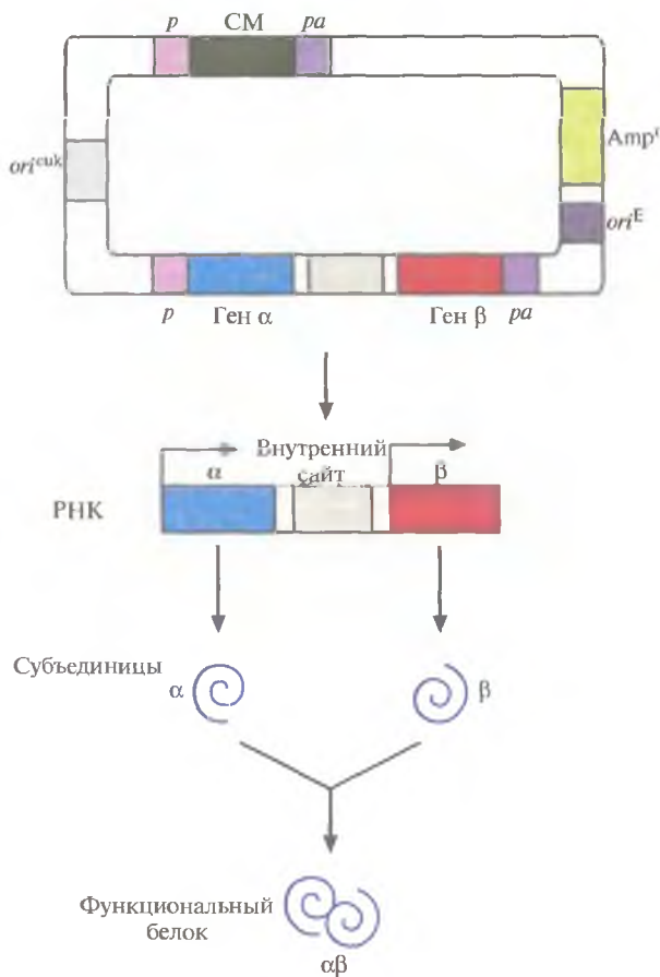
Рис. 7.17. Двухсторонний экспрессирующий вектор. Клонированные гены ( \alpha и \beta ) кодируют субъединицы димерного белка ( \alpha\beta ). Они разделены сегментом ДНК, который после транскрипции, на уровне мРНК, играет роль внутреннего сайта связывания рибосом. Каждый ген находится под контролем эукариотических промотора ( p ) и сигнала полиаденилирования ( pa ). Трансляция мРНК начинается с 5'-конца и с внутреннего сайта (угловые стрелки). Синтезированные субъединицы объединяются с образованием функционального димерного белка. Вектор содержит сайты инициации репликации, функционирующие в E. coli ( ori^E ) и в клетках млекопитающих ( ori^{euk} ); селективный маркерный ген ( Amp^r ) для отбора трансформированных клеток E. coli ; селективный маркерный ген ( CM ), находящийся под контролем эукариотического промотора ( p ) и сигнала полиаденилирования ( pa ).
