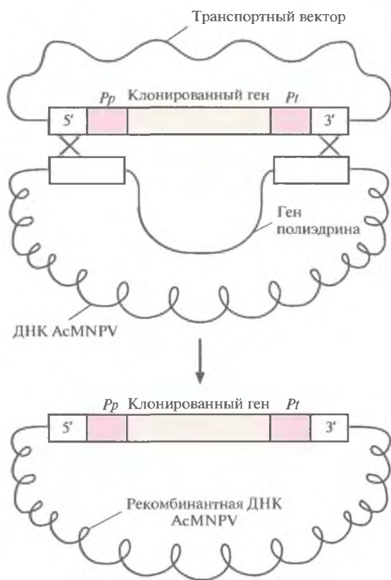
Рис. 7.9. Замещение гена полиэдрина AcMNPV единицей экспрессии транспортного вектора в результате двойного кроссинговера в 5'- и 3'-фрагментах.
