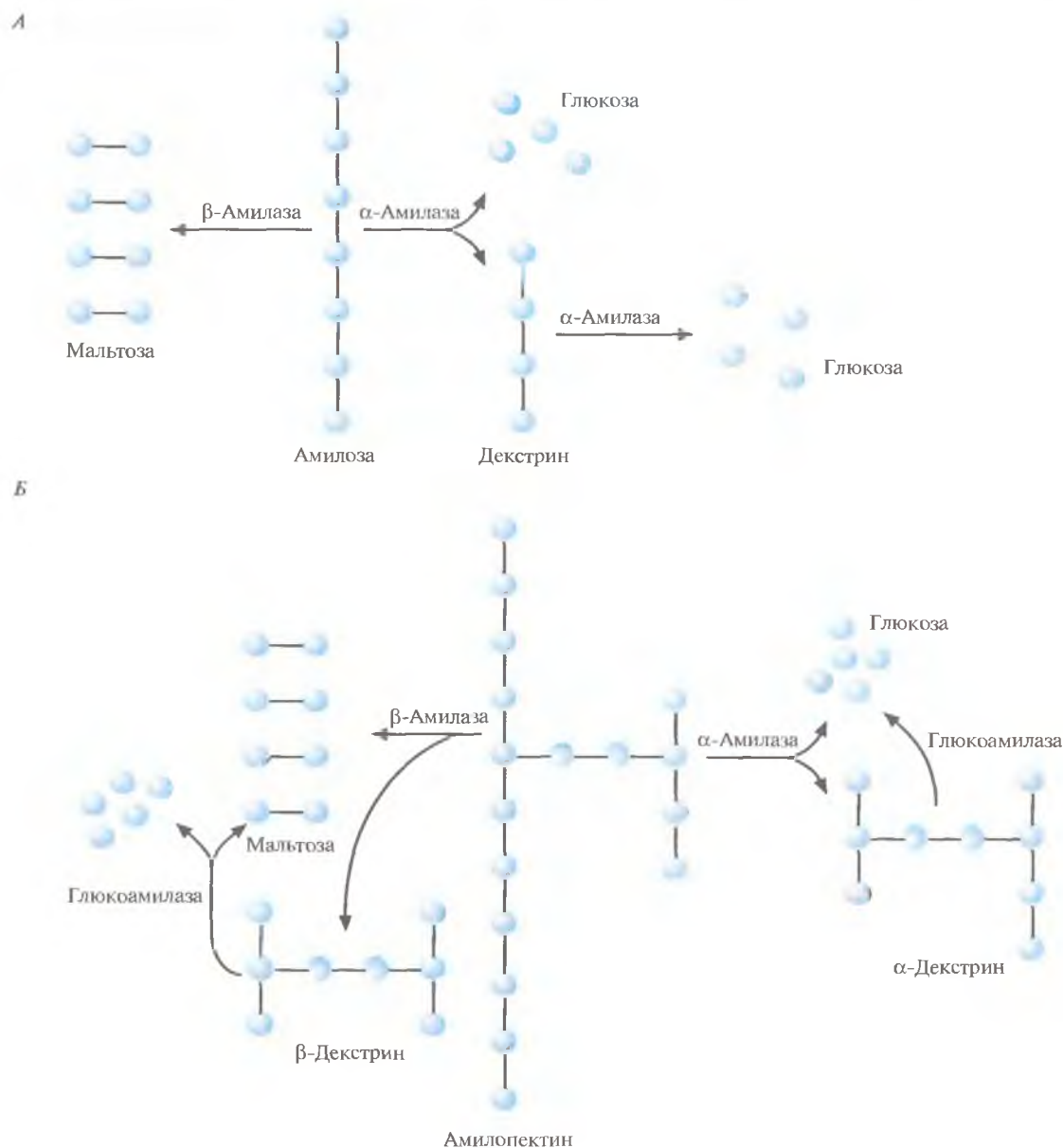
Рис. 13.9. А. Ферментативный гидролиз амилозы. Б. Ферментативный гидролиз амилопектина. Голубые кружки — остатки D-глюкозы.
