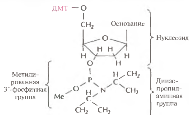
Рис. 5.3. Структурная формула фосфорамидита. Такие производные всех четырех оснований — А, Т, Г и С — используются для химического синтеза ДНК. ДМТ — диметокситритил, Me — метильная группа.
