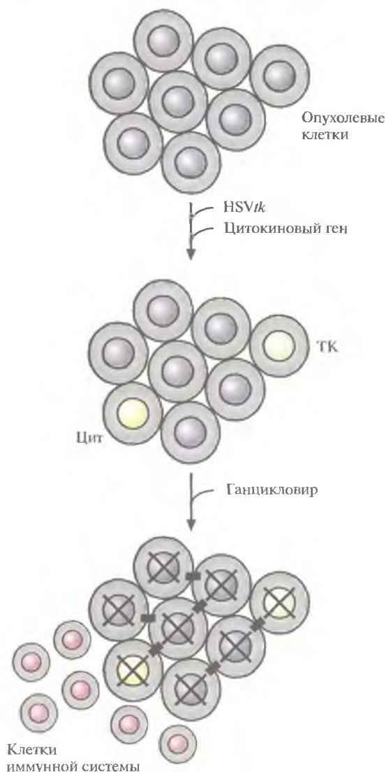
Рис. 21.12. Комбинированный подход с использованием GCV–HSVtk-терапии и генной иммунотерапии. Опухолевые клетки трансдуцировали in vivo геном тимидинкиназы вируса простого герпеса (HSVtk) и цитокинным геном. Трансдуцированные клетки опухоли, которые синтезируют цитокин (Цит), привлекают иммунные клетки, а те, которые синтезируют тимидинкиназу (ТК), фосфорилируют ганцикловир. Фосфорилированный ганцикловир проникает через межклеточные контакты (черные прямоугольники) в соседние клетки и, связываясь с ДНК, уничтожает их (X).
