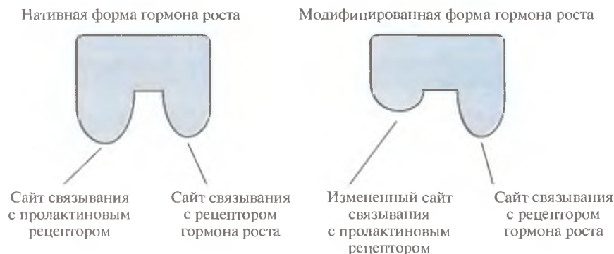
Рис. 10.2. Схематическое изображение нативной и модифицированной форм гормона роста человека (ГРЧ). С помощью олигонуклеотид-направленного мутагенеза получена форма ГРЧ, утратившая способность связываться с пролактиновым рецептором, но сохранившая специфичность к рецептору гормона роста.
