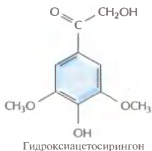
Рис. 17.2. Структурные формулы ацетосирингона и гидроксиацетосирингона. Эти соединения выделяются растением в ответ на повреждение и активируют vir -гены Ti-плазмиды.
