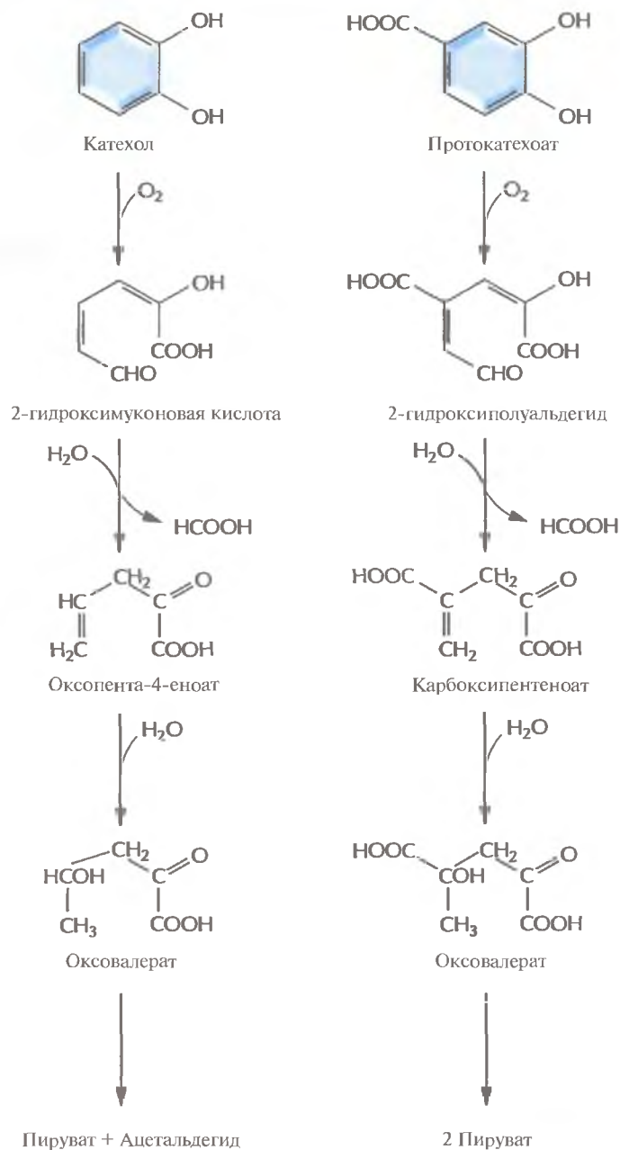
Рис. 13.4. Путь мета -расщепления при ферментативном превращении катехола и протокатехоата в пируват и ацетальдегид.
