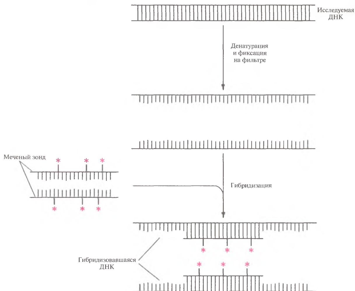
Рис. 4.11. ДНК-гибридизация. Исследуемую ДНК подвергают денатурации и фиксируют на твердой подложке, например на нитроцеллюлозном или нейлоновом фильтре. Меченый ДНК-зонд (обычно длиной от 100 до 1000 п. н.) тоже денатурируют, наносят на фильтр с исследуемой ДНК и проводят их отжиг. Для удаления негибридизовавшегося ДНК-зонда фильтр промывают и визуализируют метку. Если гибридизация между зондом и исследуемой ДНК не произошла, то никакой метки на фильтре не обнаруживается. (Метка на рисунке обозначена цветной звездочкой.)
