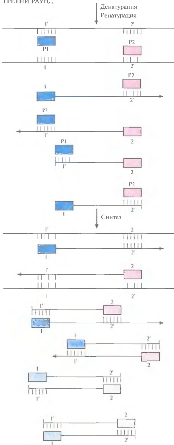
Рис. 5.20. Третий раунд ПЦР. При отжиге праймеры гибридизуются с комплементарными участками исходных цепей, а также «длинных» и «коротких» матриц. При ферментативном синтезе in vitro на исходных цепях синтезируются «длинные» матрицы, а на «длинных» и «коротких» матрицах — только «короткие матрицы».
