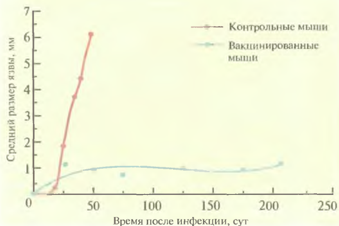
Рис. 11.8. Иммуитет к вирулентному паразиту L. major , вырабатывающийся у мышей BALB/c после инвазии аттенуированного паразита L. major . В момент времени 0 мышей, предварительно вакцинированных аттенуированным паразитом, заражали вирулентным паразитом, а затем определяли средний размер лейшманиозных язв. Контрольных мышей не вакцинировали. (Из работы Titus et al., Proc. Natl. Acad. Sci. USA 92: 10267–10268, 1995, с изменениями.)
