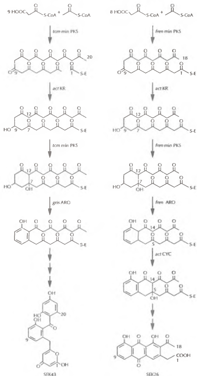
Рис. 12.16. Искусственно созданные пути биосинтеза поликетидных антибиотиков SEK43 и SEK26. Обозначения: act – актинорodin, tcm – тетраценомицин, fren – френолидин, gris – гризеузин, min PKS – минимальная поликетидсинтаза, KR – \beta -кеторедуктаза, ARO – ароматаза, CYC – циклаза.
