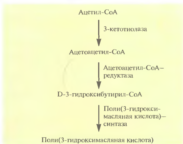
Рис. 12.22. Синтез поли(3-гидроксимасляной кислоты) из ацетил-СоА. Справа от стрелок указаны ферменты, катализирующие соответствующие реакции.
