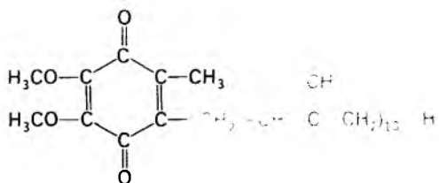
Окисленная форма кофермента Q 10 (окисленный Q 10 )
