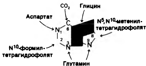
Рис. 22.4. Происхождение атомов пуринового кольца.
