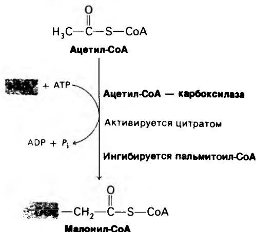
Рис. 23.9. Ацетил-СоА – карбоксилаза – ключевой регуляторный участок синтеза жирных кислот.
