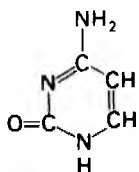
Цитозин (пиримидиновое основание)
