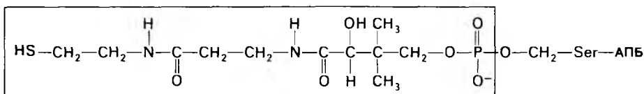
Фосфопантетеиновая простетическая группа АПБ
