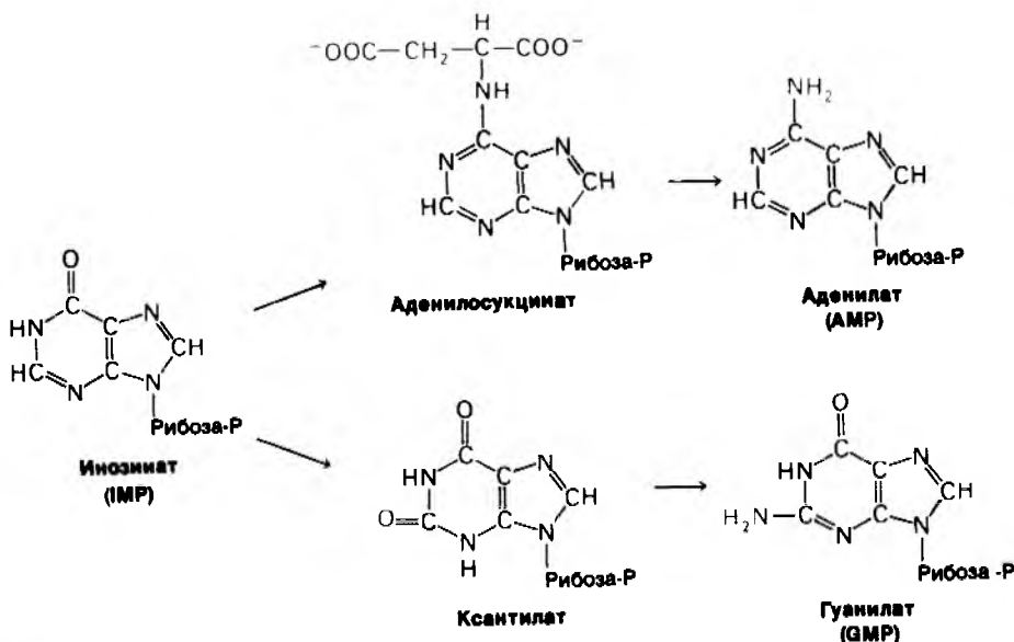
Рис. 22.8. АМР и GMP синтезируются из IMP.
