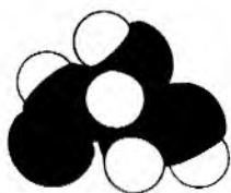
Рис. 12.3. Абсолютная конфигурация D-глицеральдегида.
