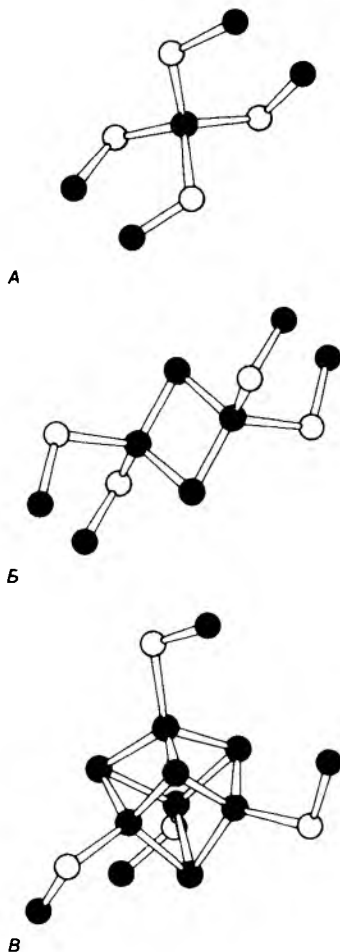
Восстановленная форма кофермента Q 10 (восстановленный Q 10 )
