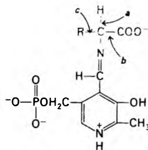
Рис. 18.3. Пиридоксальфосфатные ферменты лабилизируют одну из трех связей при \alpha -углеродном атоме аминокислотного субстрата. Например, связь a лабилизируется трансаминазами, связь b — декарбоксилазами и связь c — альдолазами (такими, как треонин-альдолаза). Пиридоксальфосфатные ферменты катализируют также реакции при \beta - и \gamma -углеродных атомах аминокислот.
