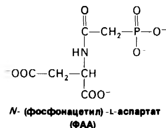
Рис. 22.12. Структура ФАА, эффективно ингибитора АТКазы.
