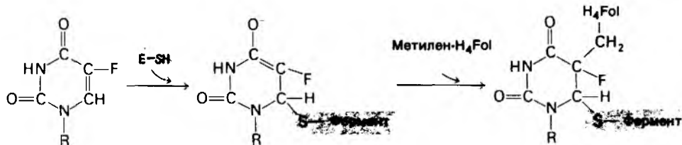
Рис. 22.23. Тимидилат-синтетаза необратимо ингибируется фтордезоксисуридилатом (F-dUMP). Этот аналог образует ковалентный комплекс одновременно с сульфгидрильным остатком фермента (выделен голубым цветом) и с молекулой метилентетрагидрофолата (отмечен желтым цветом).
