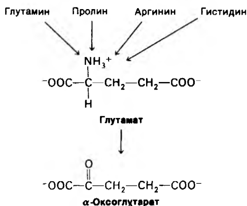
Рис. 18.8. \alpha -Оксоглутарат – «пункт входа» для некоторых \text{C}_5 -аминокислот, которые сначала превращаются в глутамат.
