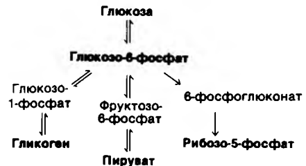
Рис. 23.10. Метаболические превращения глюкозо-6-фосфата.
