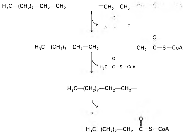
Рис. 17.5. Первые три цикла при расщеплении пальмитата. Двухуглеродные фрагменты последовательно удаляются с карбоксильного конца жирной кислоты.
