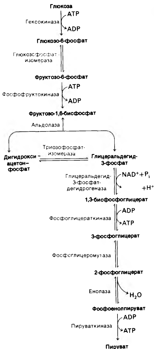
Рис. 12.8. Гликолитический путь.
