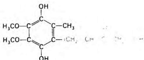
Восстановленная форма кофермента Q 10 (восстановленный Q 10 )
