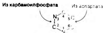
Рис. 22.11. Происхождение атомов пиримидинового кольца. С-2 и N-3 происходят из карбамоилфосфата, остальные атомы кольца — из аспартата.
