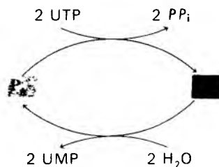
Рис. 21.17. Более высокий уровень каскадной регуляции глутамин-синтетазы. Регуляторные белки P_A и P_D , определяющие специфичность глутамин-синтетазы, способны к взаимопревращению. P_A превращается в P_D путем уридилрования (присоединения остатка UMP). Обратная реакция происходит путем гидролиза. Ферменты, катализирующие эти реакции, «чувствуют» концентрации промежуточных продуктов метаболизма.
