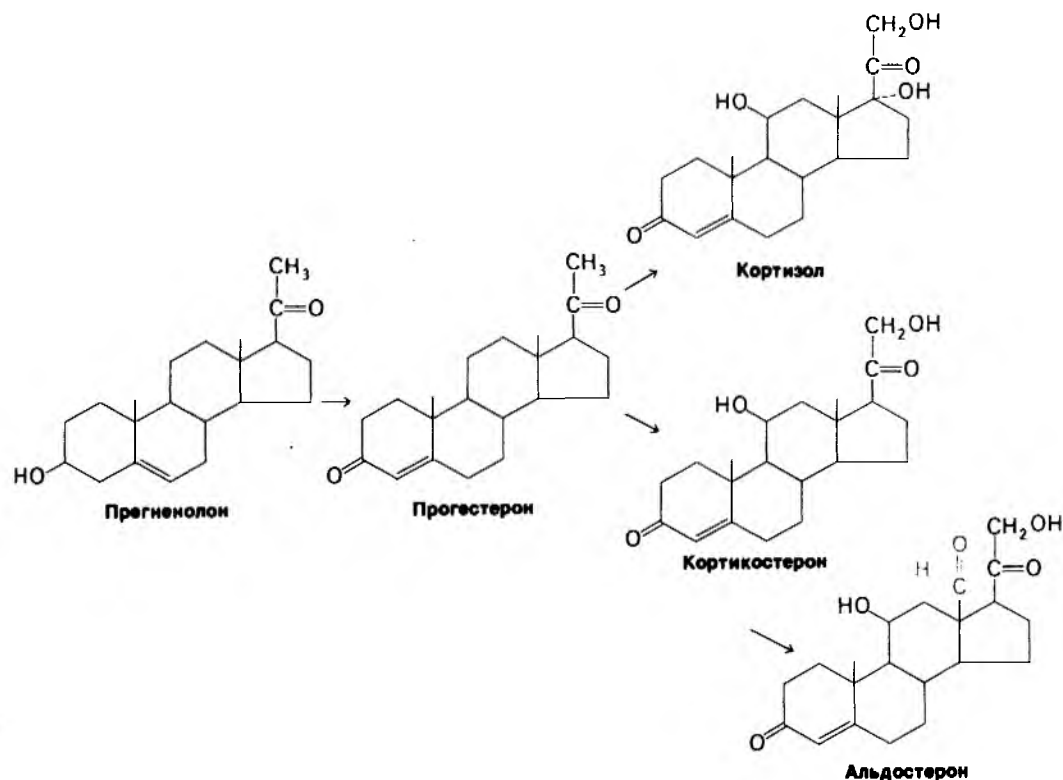
Рис. 20.20. Синтез прогестерона и кортико-стероидов.
