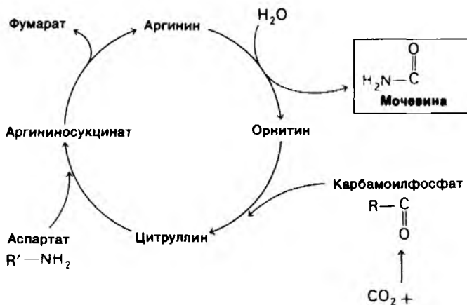
Рис. 18.4. Цикл мочевины.
