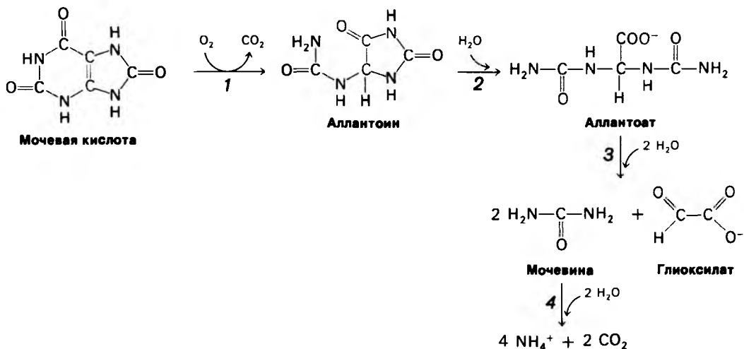
Рис. 22.29. Распад мочевой кислоты до \text{NH}_4^+ и \text{CO}_2 . Эти реакции катализируются ферментами уриказой (1), аллантаиназой (2), аллантаоиказой (3) и уреазой (4).
