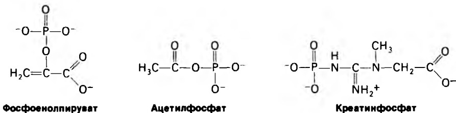
Рис. 11.7. Соединения, имеющие более высокий потенциал переноса фосфатной группы, чем АТФ.
