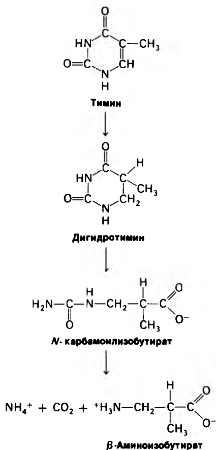
Рис. 22.30. Распад тимина.
