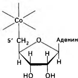
Рис. 18.14. 5'-углеродный атом 5'-дезоксаденозина находится в координационной связи с атомом кобальта 5'-дезоксаденозилкобаламина. Это — единственный известный пример связи углерод — металл в биомолекуле.
