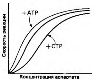
Рис. 22.14. Аллостерические свойства аспарат - транскарбамоилазы. АТФ – активатор, СТР – ингибитор фермента [Gerhart J.C., Curr. Top. Cell Regul., 2, 275 (1970).]
