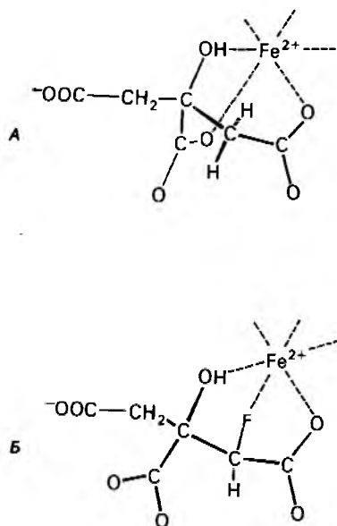
Рис. 13.14. Предполагаемая модель связывания цитрата и фторцитрата с активным центром аконитазы: А – связывание цитрата, приводящее к катализу; Б – связывание фторцитрата, приводящее к ингибированию. Атом фтора фторцитрата образует хелат с ионом железа в активном центре. (Печатается с любезного разрешения д-ра Jenny Glusker.)
