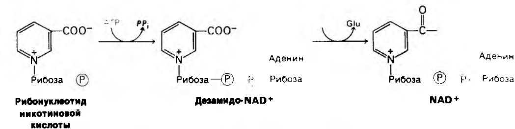
Рис. 22.25. Синтез NAD + из рибонуклеотида никотиновой кислоты.
