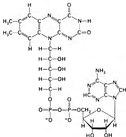
Рис. 11.9. Строение окисленной формы флавинаденидинуклеотида (FAD).
