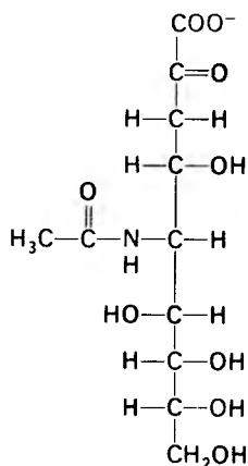
N -ацетилнейраминовая кислота (форма с открытой цепью)
