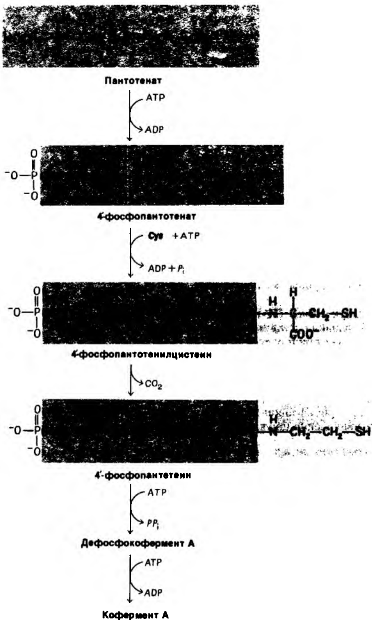
Рис. 22.26. Синтез кофермента А из пантотената.
