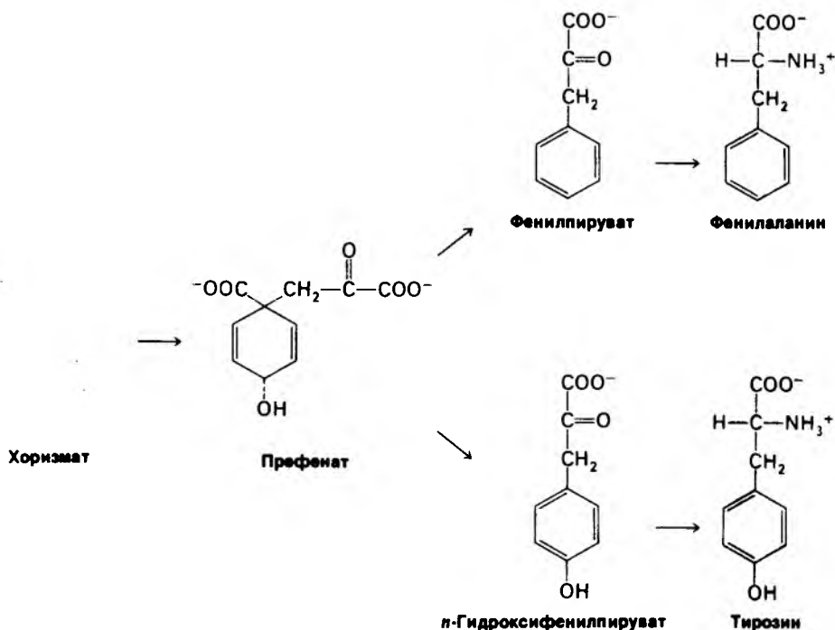
Рис. 21.11. Синтез тирозина и фенилаланина из хоризмата.
