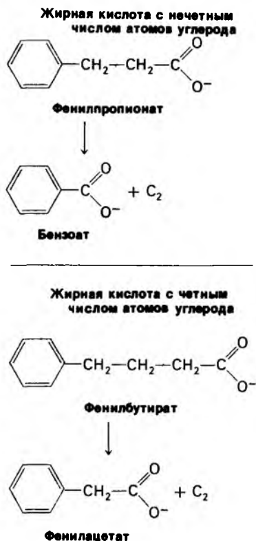
Рис. 17.3. Эксперимент Кнопа (Кноор), показывающий, что жирные кислоты распадаются путем отщепления двухуглеродных фрагментов.
