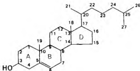
Рис. 20.18. Нумерация атомов углерода в молекуле холестерола.
