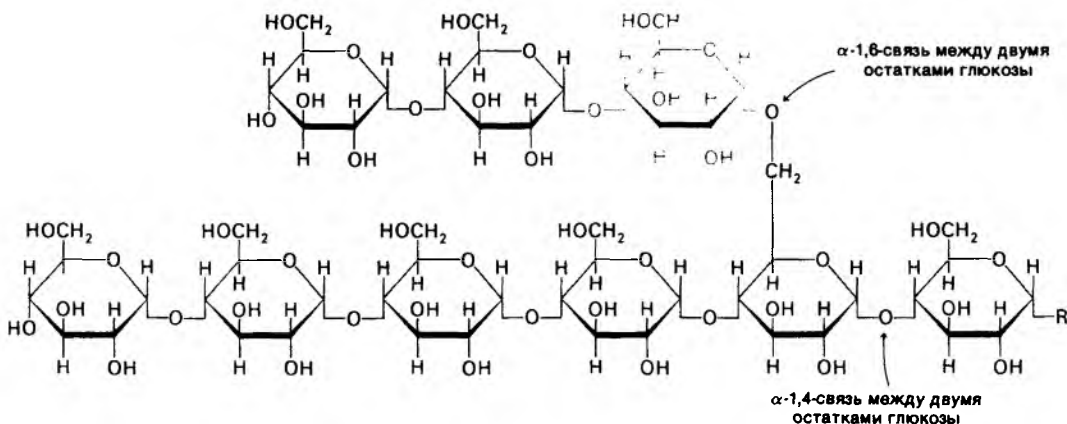
Рис. 16.1. Структура двух наружных ветвей частицы гликогена. Остатки на невосстановленных концах показаны красным цветом, остатки, с которых начинается ветвь, — синим. Остальная часть молекулы гликогена обозначена символом R.
