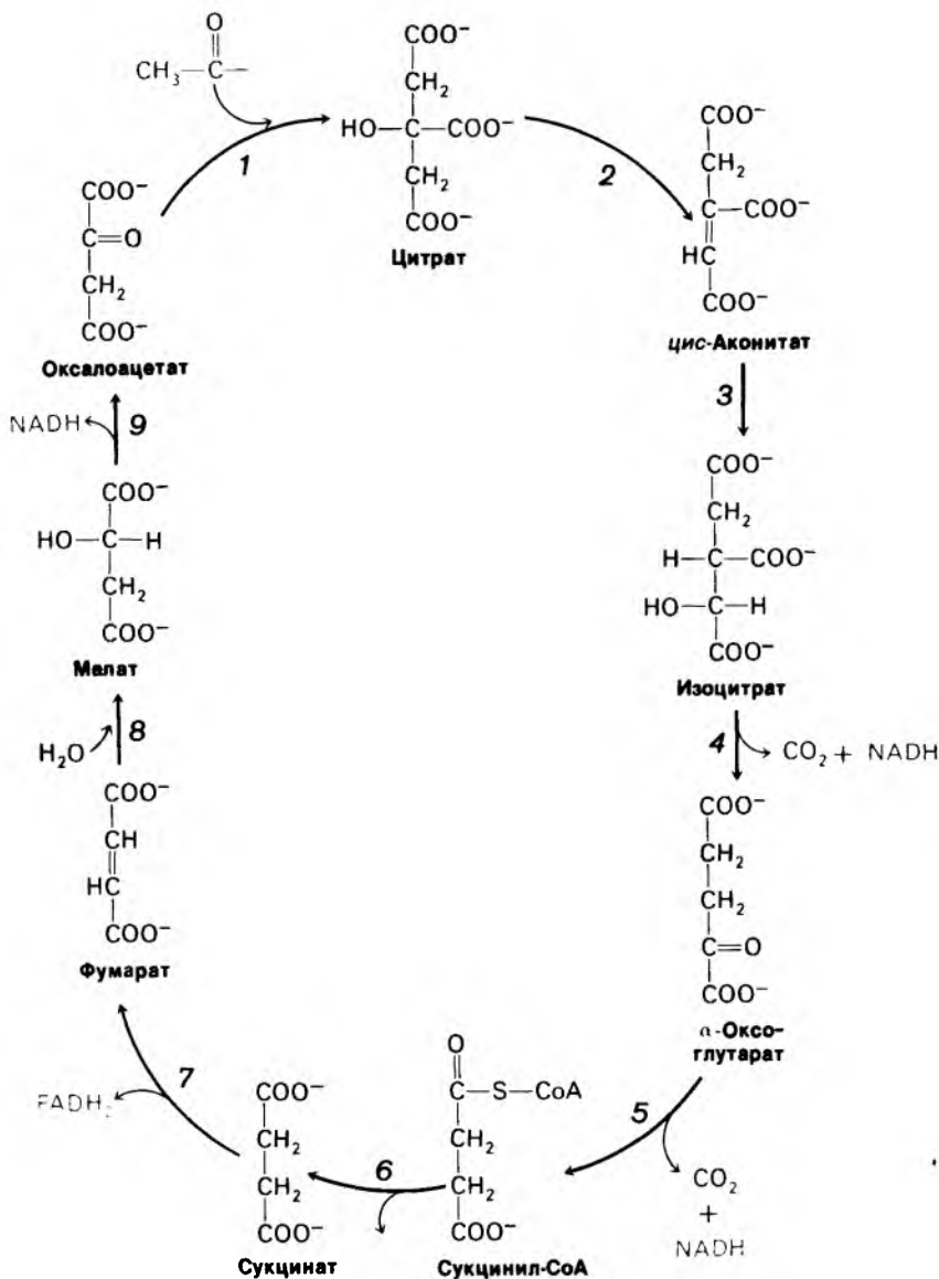
Рис. 13.5. Цикл трикарбоновых кислот.
