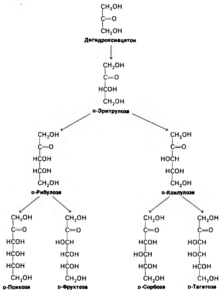
Рис. 12.20. Стереохимические соотношения D-кетоз, содержащих три, четыре, пять и шесть атомов углерода.
