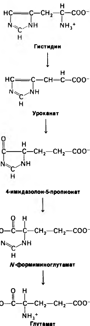
Рис. 18.9. Превращение гистидина в глутамат.
