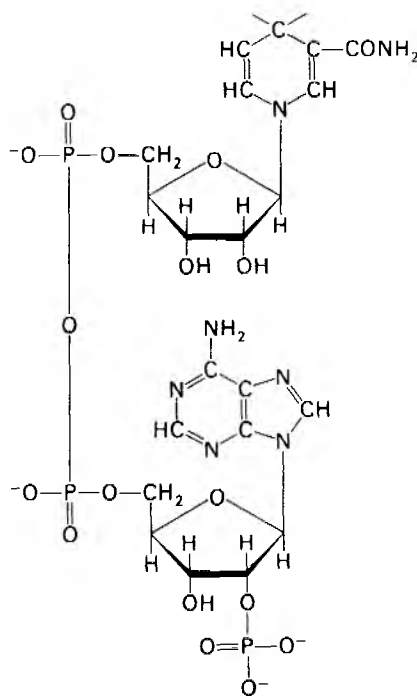
Восстановленный никотинамидденин- динуклеотидфосфат ( NADPH )
