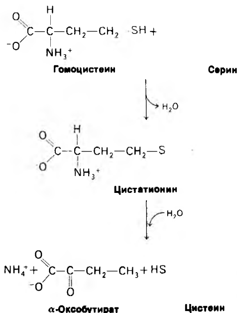
Рис. 21.8. Синтез цистеина.
