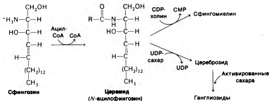
Рис. 20.4. Керамид – предшественник сфингомиелина и ганглиозидов.
