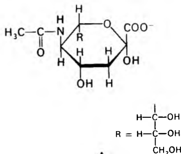
N -ацетилнейраминовая кислота (пиранозная форма)
