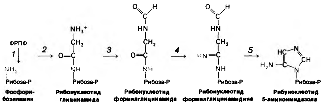
Рис. 22.6. Первый этап биосинтеза пуринов: образование 5-аминоимидазолрибонуклеотида из ФРПФ. Смысл этих реакций заключается в замещении пирофосфатной группы аминок группой боковой цепи глутамин (1), присоединении глицина (2), формилировании с участием метенилтетрагидрофолата (3), переносе атома азота глутамин (4), дегидратировании и замыкании кольца (5).
