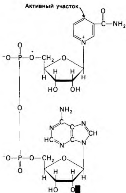
Рис. 11.8. Строение окисленной формы никотинамидадениндинуклеотида ( \text{NAD}^+ ) и никотинамидадениндинуклеотидфосфата ( \text{NADP}^+ ). В \text{NAD}^+ \text{R} = \text{H} ; в \text{NADP}^+ \text{R} = \text{PO}_3^{2-} .
