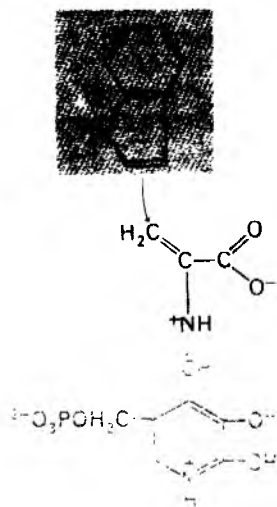
Рис. 21.13. Предполагаемый промежуточный продукт при синтезе триптофана. Серин образует шиффово основание с ПЛФ, связанным с β-цепью белка, которое затем дегидратируется и образует шиффово основание аминокрилата (показано красным цветом). Этот связанный с ферментом промежуточный продукт атакуется индолом, продуктом другой частичной реакции, катализируемой α-субъединицей белка. В результате образуется триптофан.
