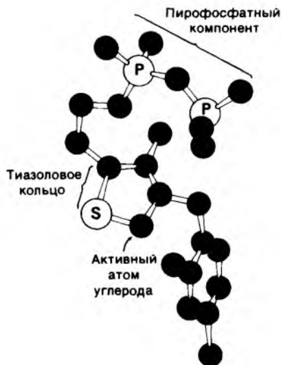
Рис. 13.6. Модель тиаминпирофосфата.
