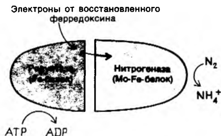
Рис. 21.3. Схематическое изображение нитрогеназного комплекса. Перед тем как \text{N}_2 превращается в \text{NH}_4^+ , комплекс диссоциирует и редуктаза отделяется от нитрогеназного компонента.
