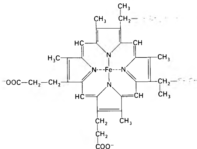
Рис. 14.6. Гем в цитохромах c и c_1 ковалентно присоединен к двум цистеиновым боковым цепям.
