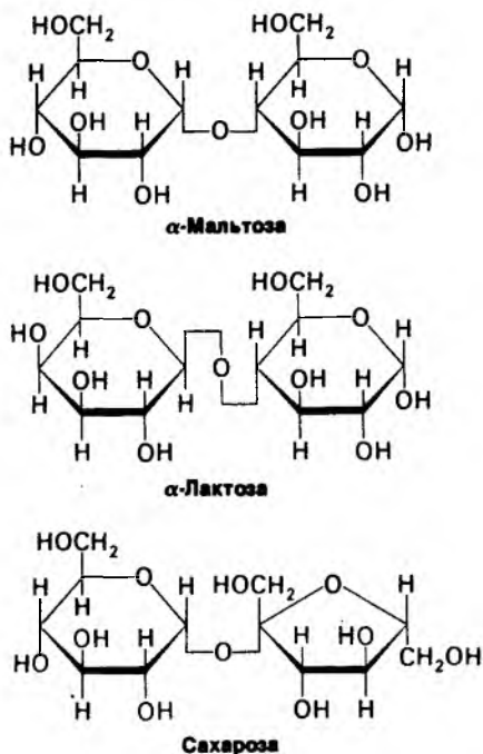
Рис. 16.12. Строение наиболее широко распространенных дисахаридов: α-мальтозы, α-лактозы и сахарозы. Буква α относится к конфигурации аномерного углеродного атома на восстанавливающем конце дисахарида, а не к конфигурации гликозидной связи.
