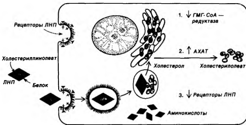
Рис. 20.17. Превращения липопротеинов низкой плотности в культивируемых фибробластах человека. ГМГ-СоА—редуктаза—3-гидрокси-3-метилглутарил-СоА—редуктаза; АХАТ—ацил-СоА:холестерол-ацилтрансфераза. (Печатается с любезного разрешения д-ра Michael Brown и д-ра Joseph Goldstein.)
