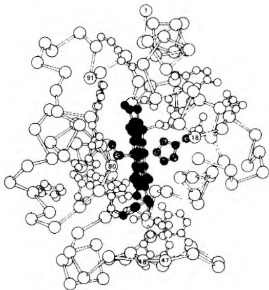
Рис. 14.14. Трехмерная структура восстановленного цитохрома с тунца. Показаны группа гема (окрашено красным), метионин-80 (окрашено синим), гистидин-18 (окрашено синим) и \alpha -углеродные атомы [Takano T., Kallai O. B., Swanson R., Dickerson R. E., J. Biol. chem., 248 , 5244 (1973).]
