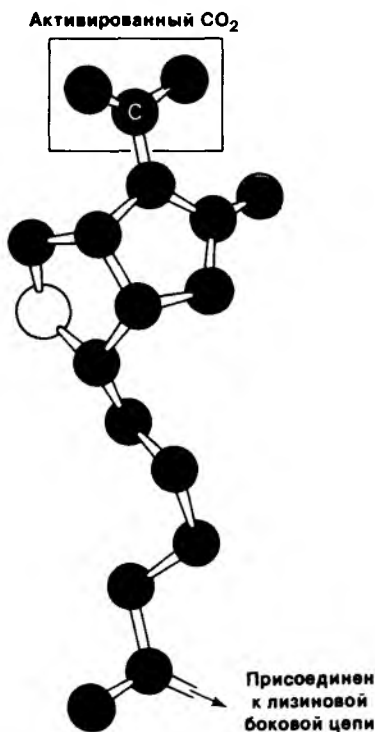
Рис. 15.6. Молекулярная модель карбоксибиотина.
