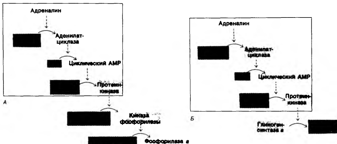
Рис. 16.9. Каскады реакций, регулирующих обмен гликогена: А – распад гликогена; Б – синтез гликогена. Неактивные формы ферментов показаны красным, активные – зеленым цветом. Последовательность реакций, приводящих к активации протеинкиназы, одна и та же для регуляции распада и для регуляции синтеза гликогена.
