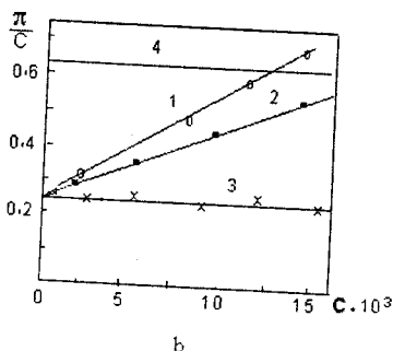
71 – rasm. Har xil eritmalar uchun \pi/c nisbatning c ga bog‘liqligi: a – sellyuloza atsetatining atsetondagi eritmasi har xil fraksiyalari; b – nitrosellyulozaning atseton (1), metanol (2), nitrobenzol (3) dagi eritmasi va Vant-Goff tenglamasiga bo‘ysinadigan ideal eritma (4).
