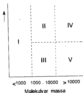
103 – rasm. Polimer fizikaviy xossalarining molekulyar massasi va kristallilik darajasiga bog'liqligi.
