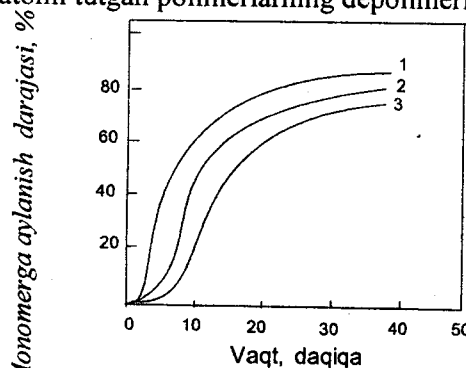
123-rasm. Polimetilmetakrilat depolimerlanishining qizdirish vaqtiga bog'liqligi:
