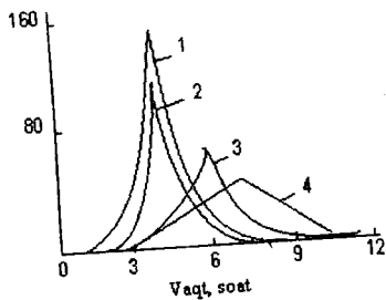
29-rasm. Kaprolaktamning suv ishtirokidagi polimerlanish tezligi 1-1,96%; 2-1,56%; 3-0,76%; 4-0,5% H_2O .
