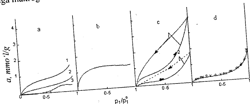
129-rasm. Polimerlarda «inert» suyuqliklar bug'lari sorbsiyasining izotermasi: a – g'ovaksiz (1 – polivinil spirti; 2 – polivinilxlorid; 3 – polistirol); b – mikrog'ovakli; c – tutash g'ovakli sorbentlar (1 – erituvchi muhitida olingan stirol – divinilbenzol sopolimeri; 2 – poliarilat (uzluksiz egrilar – sorbsiya, uzoq egrilar – desorbsiya); d – makrog'ovakli (o – stiروفleks pardasi; x – polistirolning makrog'ovakli pardasi).
