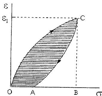
110 – rasm. Amorf polimer deformatsiyasida gisterezis hodisasi (ko‘rsatgichlar deformatsiya jarayoni ning yo‘nalishini ko‘rsatadi).
