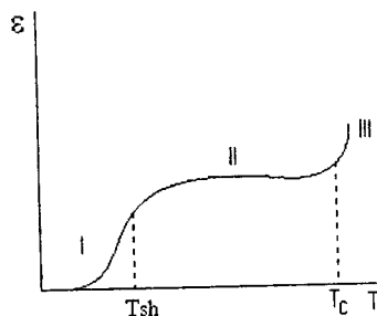
105 – rasm. Amorf polimerning termomexanik egri chizig'i. I-shishasimon holat; 2 – yuqori elastik holat va 3– qovushqoq – oquvchan holat oralig'lari.
