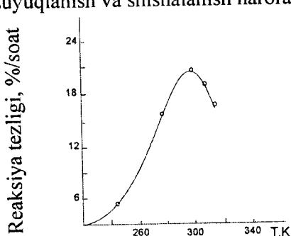
122-rasm. Xlormetil reaksiyasi boshlang'ich tezligining haroratga bog'liqligi.
