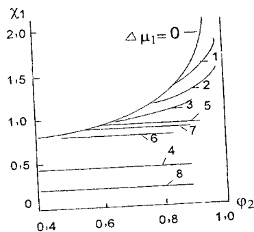
53-rasm. \chi_1 parametrining polimerning eritmadagi hajmiy ulushiga bog'liqligi: 1-tabiiy kauchuk – atseton; 2-tabiiy kauchuk – metiletilketon; 3-tabiiy kauchuk – etilatsetat; 4-tabiiy kauchuk – benzol; 5-polistirol – atseton; 6-polistirol – n-propilatsetat; 7- poliizobutilen – benzol; 8-poliizobutilen – xloroform.
