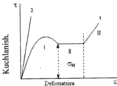
113 – rasm. Shishasimon polimerning moʻrtlik haroratidan yuqori (1) va past (2) haroratlarda choʻzilish egri chizigʻi. \sigma_M – majburiy elastik chegara.
