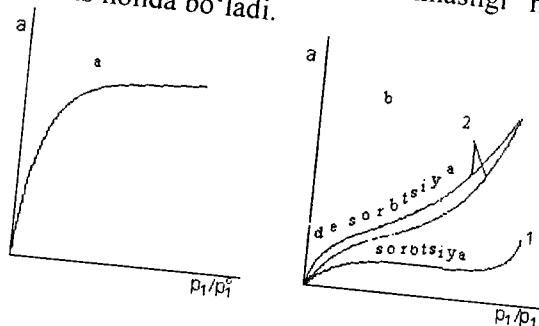
128-rasm. Bir jinsli mayda g'ovakli sorbentlar (a), g'ovaksiz (b, 1 egri chiziq) va ko'chuvchan g'ovakli sorbentlarda (b, 2 egri chiziq) bug'lar sorbsiyasining tipik izotermalari.
