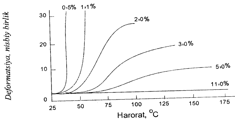
117- rasm. Fenolformaldegid oligomerlarning qotishigaurotropin miqdorining (egri chiziqlardagi raqamlar) ta'siri.
