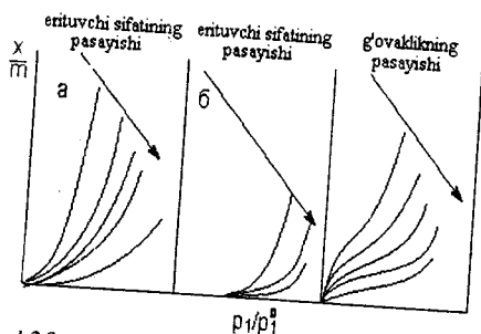
130-rasm. Polimerlarning noinert suyuqliklar bug'ini sorbsiyalash izotermasi:
