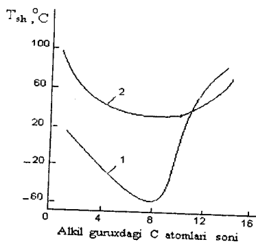
118- rasm. n -alkilakrilatlar (1) va n -alkilmetakrilatlar (2) polimerlari shishalanish haroratining alkil guruhlar soniga bog'liqligi.
