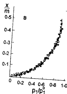
131-rasm. n-geksanning yuqorielastik polimerlarga sorbsiyalanish izotermasi: o – tabiiy kauchuk; x – butadien sintetik kauchugi; • – izopren sintetik kauchugi (SKI); Δ – SKI ning yuqori-molekulyar fraksiyalari; ← sintetik kauchuk SK-1; ○ – CK-2.
