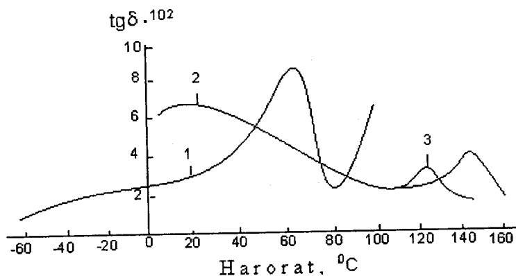
134-rasm. Stereotartibli polimetilmetakrilat namunalarining 20 Gts da tg\delta ning haroratga bog'liqligi: 1 - izotaktik; 2 - sindiotaktik; 3 - ataktik.
