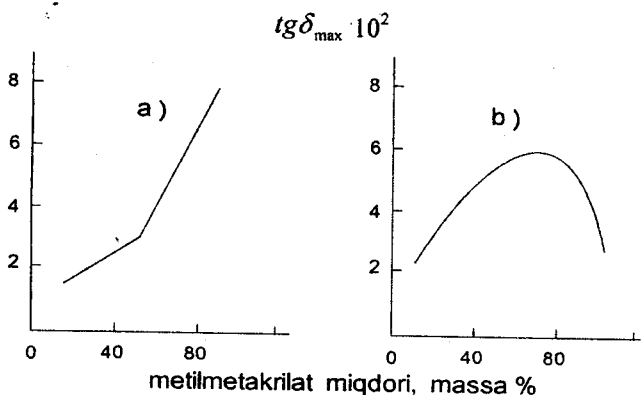
133-rasm. tg\delta_{\max} ning sopolimerdagi stirool-metilmetakrilat nisbatiga bog'liqligi: a – 400 Gts dagi dipol-guruhli yo'qotish; b – 20 Gts dagi dipol-segmental yo'qotish.
