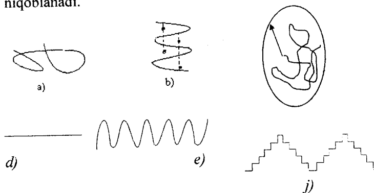
87-rasm. Makromolekulalarning konformatsion turlari:
