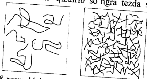
68-rasm. Makromolekulalarning suyultirilgan (a) va konsentrlangan (b) eritmalarida o'zaro joylashish sxemasi.
