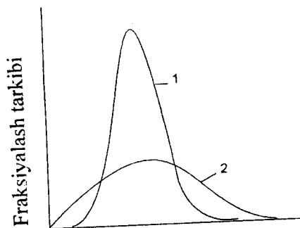
1-rasm. Molekulyar massa bo'yicha taqsimlanish egrilari
