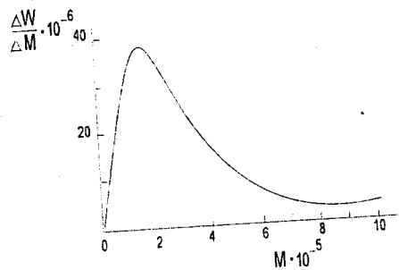
62-rasm. Polimerlarning molekulyar massa bo'yicha taqsimlanish differensial egrisi.
