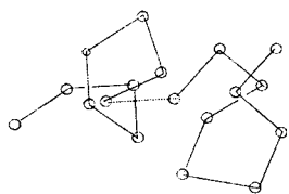
37-rasm. Erkin a'zolanagan zanjir konformatsiyalari.
