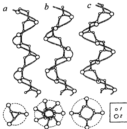
96 - rasm. Izotaktik vinil polimerlarning spiral strukturasi. a - 3_1 - spiral; b - 7_2 - spiral; c - 4_1 - spiral; 1 - asosiy zanjirni hosil qiluvchi uglerod atomlari; 2 - takroriy uglerod atomlariga birikkan R-o'rindosh. Tasvirni soddalashtirish uchun uglerod atomlariga birikkan vodorod atomlari ko'rsatilmagan.
