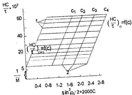
72-rasm. Nur yoyish yordamida olingan natijalarni ekstrapolyatsiya qilish uchun qo'llaniladigan B. Zimm diagrammasi. (Sellyuloza nitrating atsetondagi eritmasi), c ni 2000 marta oshirish chizmani chizishni osonlashtirish uchun qilingan. 1 - o'zgarmas \theta larda C = 0 gacha ekstrapolyatsiya qilish natijalari; 2 - o'zgarmas c larda \theta = 0 gacha ekstrapolyatsiya qilish natijalari.
