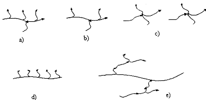
86-rasm. Tarmoqlangan polimerlarning turlari: a, b – qisqa va uzun yon zanjirli; c – yulduzsimon; d ) o‘rkachsimon; e – statistik makromolekulalar.
