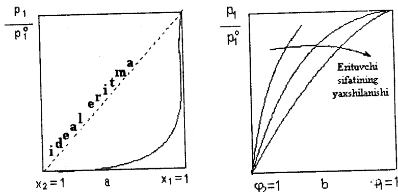
48-rasm. Polimer eritmasi ustidagi erituvchi bug' bosimining komponentlar x mo'l (a) va \phi -hajmiy (b) ulushlariga bog'liqligi.
