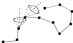
38-rasm. Belgilangan (fiksatsiyalangan) valent burchakli zanjir konformatsiyalari.
