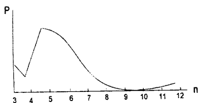
26-rasm. Sikllanish ehtimolligi ( r ) ning halqadagi atomlar soni ( n ) ga bog'liqligi.
