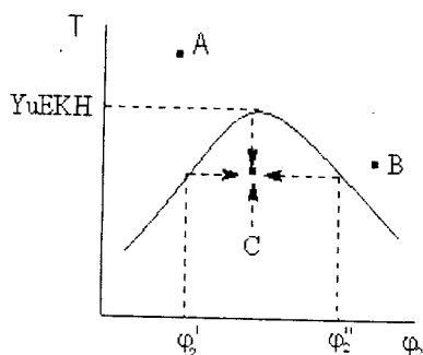
45-rasm. YuEKH li sistema uchun harorat – tarkib egri.
