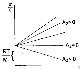
50-rasm. \pi/c ning polimerning turli erituvchilardagi eritmalarining konsentratsiyasiga bog'liqligi.
