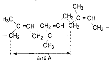
Sis-izomer (kauchuk)
