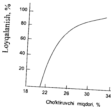
60-rasm. Turbidimetrik titrlashning tipik egrisi
