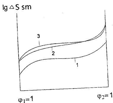
52-rasm. Tabiiy kauchuk-benzol sistemasi uchun aralashish entropiyasining eritma tarkibi-ga bog'liqligi: 1-ideal aralashish entropiyasi; 2- chin aralashish entropiyasi; 3-nazariy hisoblangan aralashish entropiyasi.
