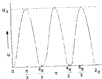
35-rasm. Etan molekulasini potensial energiyasining metil guruhi burilish burchagiga bog'liqligi.
