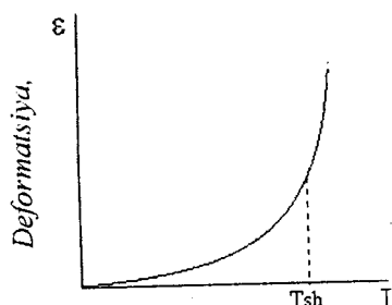
104 – rasm. Quyimolekulyar shishalanuvchi suyuqlikning termomexanik egri chizig'i.
