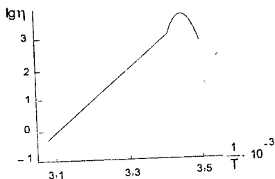
78-rasm. Polimer eritmali qovushqoqligining harorat bilan o'zgarishi.
