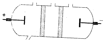
59-rasm. Elektrodializator.
