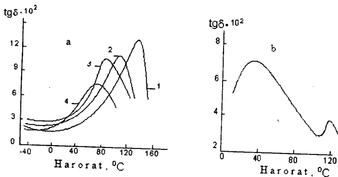
132-rasm. Polivinil spirtining ba'zi atsetallari (a) va polimetilmetakrilat (b) uchun tg\delta ning haroratga bog'liqligi: 1 – etilal; 3 – propilal; 3 – butiral; 4 – oktilal.
