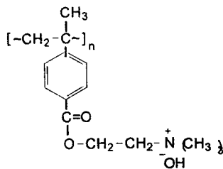
polirimetilammoniy - metakrilat
