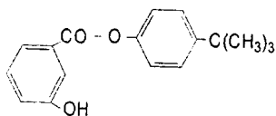
4-tret-butilfenilsalitsilat
