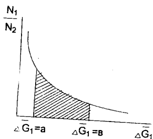
55-rasm. Komponent kimyoviy potentsialining eritma tarkibiga qarab o'zgarishi.
