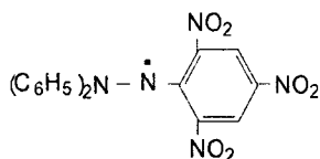
difenilpikrilgidrazin
