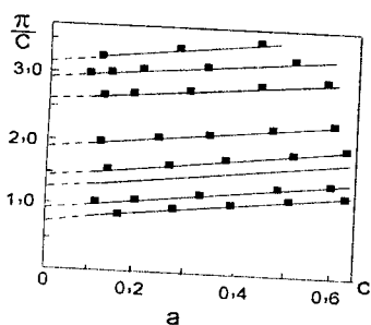
71 – rasm. Har xil eritmalar uchun \pi/c nisbatning c ga bog‘liqligi: a – sellyuloza atsetatining atsetondagi eritmasi har xil fraksiyalari; b – nitrosellyulozaning atseton (1), metanol (2), nitrobenzol (3) dagi eritmasi va Vant-Goff tenglamasiga bo‘ysinadigan ideal eritma (4).
