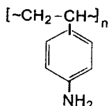
poli-n-aminostirol
