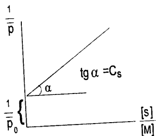
6-rasm. Erituvchiga zanjir uzatilish konstantasini aniqlash.
