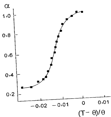
58-rasm. Globula-o'ralma o'tishdagi makromolekula o'lchamining haroratga bog'liqligi (nuqtalar-tajriba natijalari, chiziq-nazariy).
