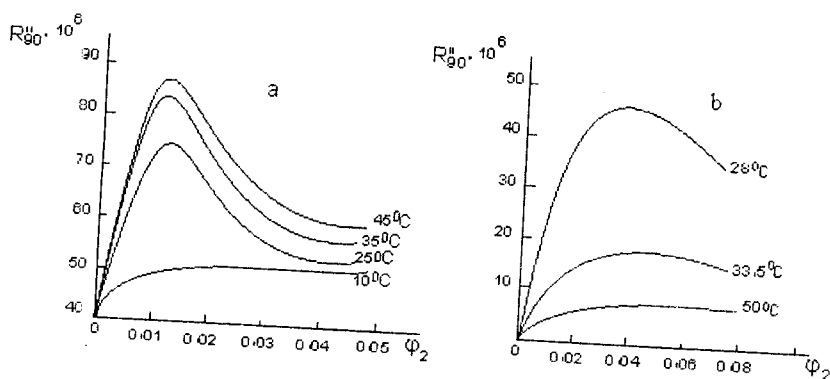
76-rasm. Ortiqcha yorug'lik yoyilishning ( R_{90}'' ) eritmadagi polimerning hajmiy ulushiga bog'liqligi: a – polistirol yaxshi erituvchi – benzolda; b – polistirol yomon erituvchi – siklogeksanda.
