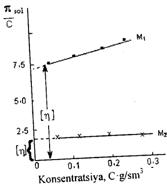
65-rasm. Keltirilgan qovushqoqlikning konsentratsiyaga bog'liqligi ( M_1 \gg M_2 ).
