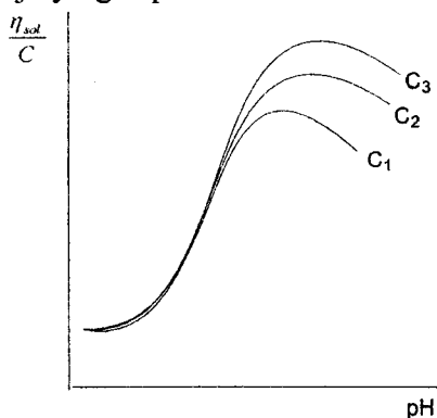
82 – rasm. Har xil konsentrat-siyali polikislota eritmasi keltirilgan qovushqoqligining muhit pH ga bog'liqligi ( C_1 > C_2 > C_3 ).
