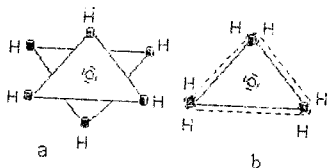
34-rasm. Etan molekulasidagi vodorod atomlarining har xil fazoviy joylanishi (pastda—molekulaning soyasi). a-tsis-holat; b-trans-holat.
