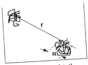
63-rasm. Suyultirilgan eritmada makromolekulalar holati.
