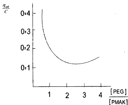
83-rasm. Polimetakril kislota bilan polietilenglikol aralashmasi suvli eritmalari keltirilgan qovushqoqligining tarkib bilan o'zgarishi.
