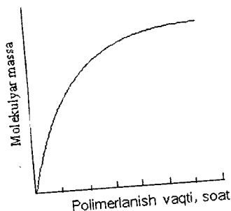
32-rasm. Geksametilendiizotsianat va 1,4-butandiolning bosqichli polimerlanishida poliuretan molekulyar massasining o'sishi.
