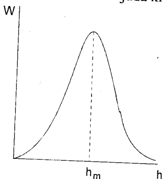
41-rasm. Makromolekulaning ikki uchi orasida molekular taqsimlanish egrisi.
