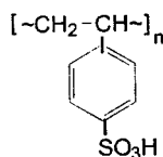
polistirolsulfon kislotali
