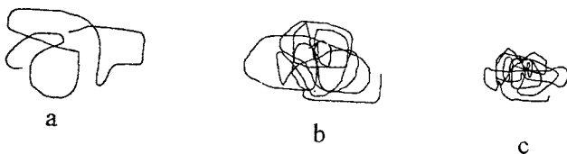
57-rasm. Bo'kkan o'ralma (a), ideal o'ralma (b) va globula (c) shaklidagi shartli ko'rinishlari. Barcha hollarda zanjirning uzunligi bir xil.
