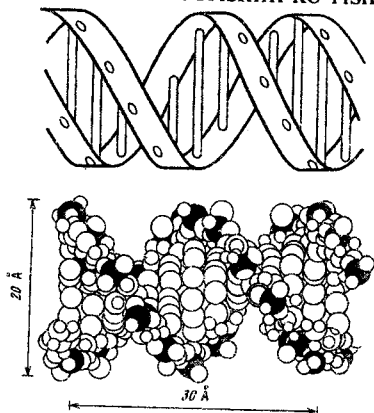
97 – rasm. Uotson – Krikning DNK spiral struktura modeli.
