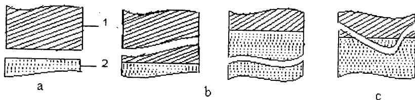
119 – rasm. Adgezion birikmaning emirilish sxemasi: 1 – adgeziv; 2 – substrat; a – adgezion emirilish; b – kogeziyon emirilish; c – aralash emirilish.
