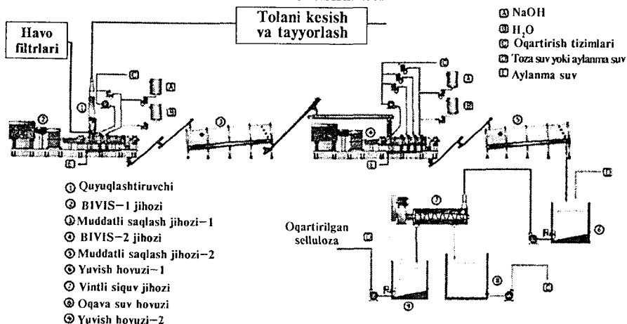
26-rasm. Paxta momig'idan selluloza olish texnologiyasi.
