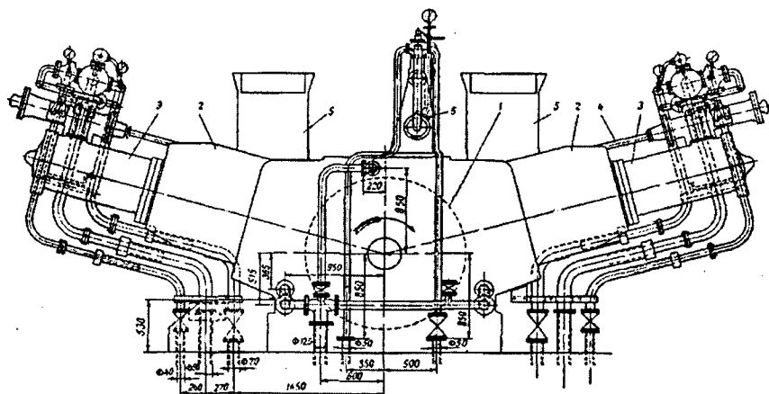
37-rasm. Greyt-Norzen turidagi gidravlik defibrer: 1 — defibrer toshi; 2 — siquv qutilari; 3 — gidravlik silindrlar; 4 — siquv qutisi boshqaruvchisi; 5 — yuklash qutilari; 6 — toshni mahkamlash moslamasi.
