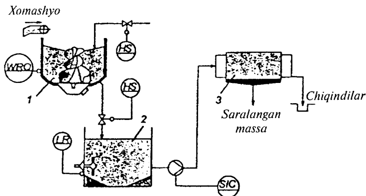
60-rasm. Laminirlangan qog'oz va qalin qog'oz qutilarini (sharbat, sut va boshqalar) davriy usulda maydalash-titish sxemasi:
