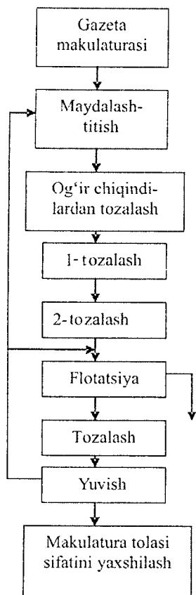
53-rasm. Gazeta qog'ozini uchun flotatsiyadan foydalanib, sifati yaxshilangan makulatura tolasi tayyorlash sxemasi.
