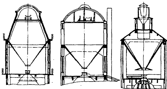
5-rasm. Payraha uchun turli ko'rinishdagi bunkerlar.
