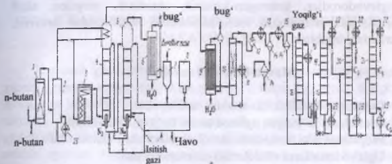
57-rasm. Parafinlarni birinchi bosqichda degidirlash texnologik sxemasi. 1-qurutgich; 2-bug'latgich; trubkasimon pech; 4-reaktor; 5-regenerator; 12-kompressor; 14-separator; 16-absorber; 17-issiqlik almashtirgich; 6,9-utilizator-qozon; 7-elektrofiltr; 8-bunker; 10-srubber; 11,13,15,19-sovutgichlar; 18-bug'latish kolonkasi; 20,21-rektifikatsiya kolonnalari; 22-deflegmatorlar; 23-qaynatgich.
