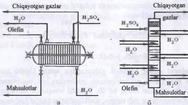
27-rasm. Etilen va propilenni sulfat kislotasi bilan gidratlash qurilmalari: a) diskli aralashtirgichli gorizontaal absorber; b) uzluksiz ravishda ishlaydigan tarekali-kolonnali absorber.
