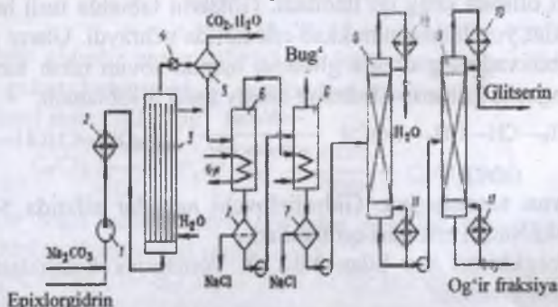
25-rasm. Xlorlash usuli bilan glitserin olish texnologik sxemasi: 1-nasos, 2-isituvchi, 3-reaktor, 4-drossel ventili, 5-separator, 6-bug'latish kublari, 7-filtrlar, 8-suvni haydash kolonnasi; 9-og'ir fraksiyani ajratish kolonnasi, 10-kondensator deflegmator, 11-qaynatgichlar.
