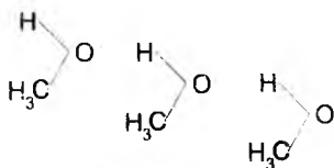
Metil spirti
