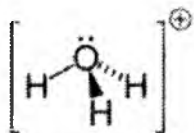
Oksoniy ioni
