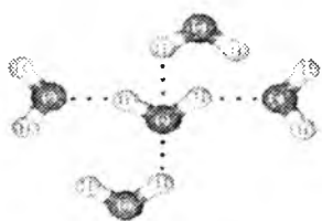
Suvning vodorod bog' hosil qilishi
