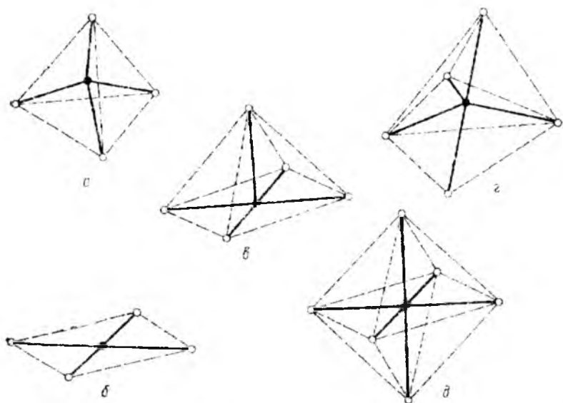
5.5–Rasm. O'zgaruvchan valentli metallarni ligandalar bilan hosil qilgan komplekslarini fazoviy joylashishi:
