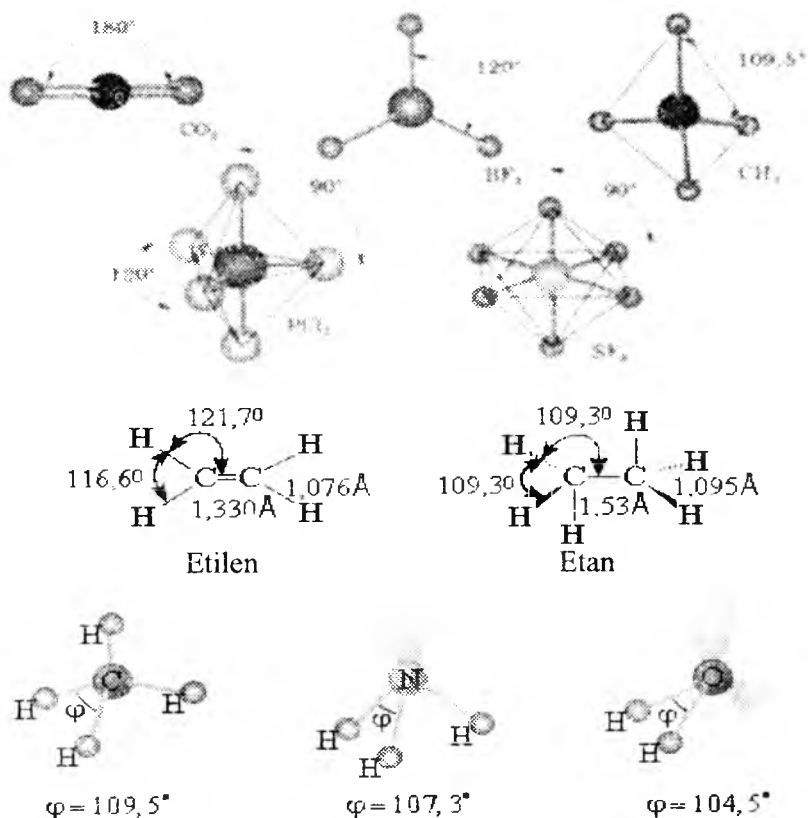
1.1-Rasm. Kimyoviy birikmalarda valent burchaklari
