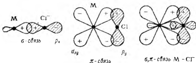
5.7–Rasm. M metallni \pi -donorli \sigma -ligandalar ( \text{Cl} ) bilan bog' hosil qilishi.
