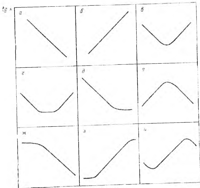
5.3-Rasm. Reaksiya tezlik konstantasini muhit kislotaligiga bog'liq grafiklari
