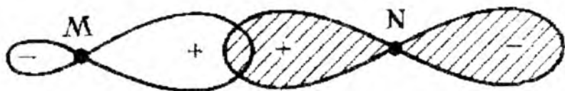
5.6. – Rasm. M metallni \sigma -liganda ( :\text{CH}_3 ) bilan bog' hosil qilishi.
