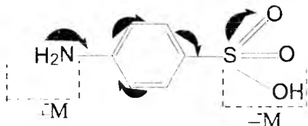
p-aminobenolsulfokislota
