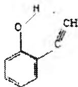
2,6-digidrokisbenzoy kislota
