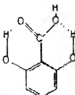
2,6-digidrokisbenzoy kislota
