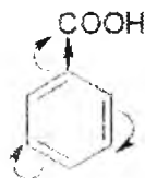
benzoyl kislota benzoyl aldegid
