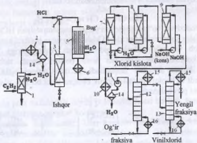
23-rasm. Atsetilenni gidroxlorlash bilan vinilxlorid olish texnologik sxemasi: 1-olovni to'suvchi; 2,6,10-sovutgichlar; 3-quritish kolonnasi; 4-aralashtirgich; 5-reaktor; 7-9-skrubberlar; 11-kompressor; 12,13-rektifikatsiya kolonnalari; 14-separator; 15-deflegmator; 16-qaynatgich.
