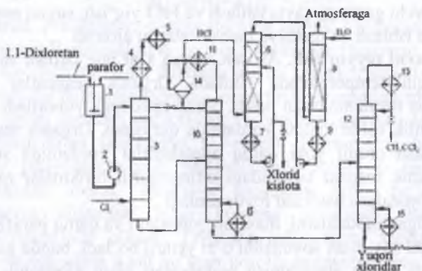
18-rasm. 1,1,1-trixloretnan olish texnologik sxemasi:
