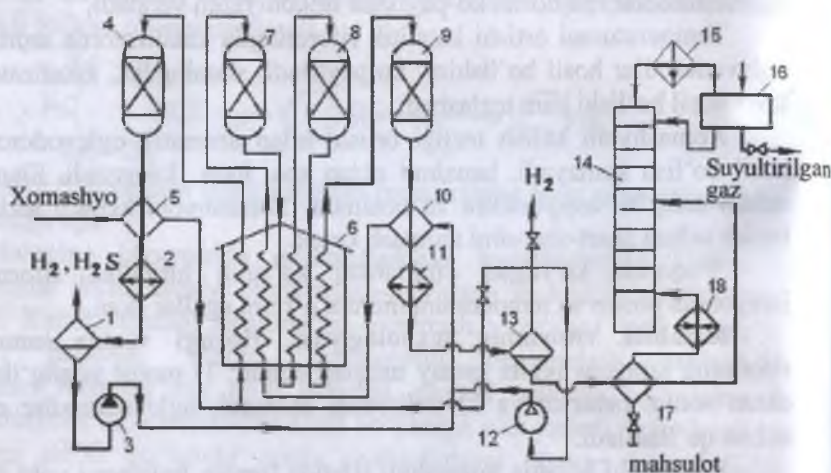
6-rasm Platforming jarayoni texnologik sxemasi:
