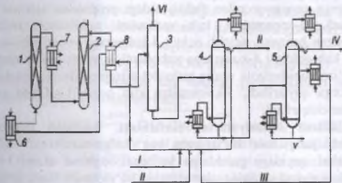
33-rasm. Seolitli katalizatorlar ishtirokida benzolni alkillash bilan izopropilbenzol olish texnologik sxemasi: 1-alkillash reaktori; 2- perealkillash reaktori; 3-depropanizator; 4,5-rektifikatsiya kolonnalari; 6-isitgich; 7-sovutgich; 8-issiqlik almashtirgich; I-propan-propilen fraksiyasi; II-benzol; III-diizopropilbenzol; IV-kumol; V-poliizopropil-benzollar; VI- propan.
