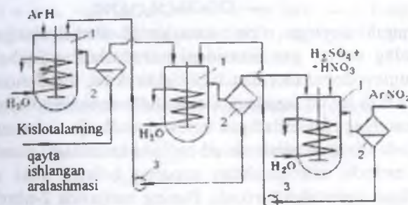
47-rasm. Aromatik birikmalarni nitrollash reaksiya qurilmasi:
