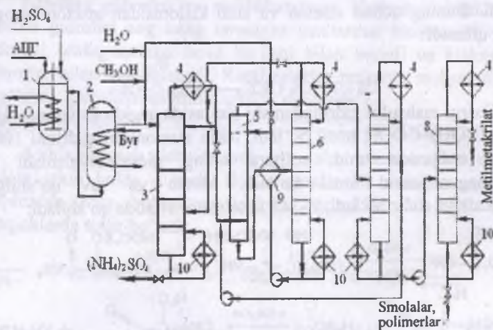
26-rasm. Atsetonsiangidrindan metilmetakrilat olish texnologik sxemasi: 1–aralashtirgich; 2 – reaktor; 3– efirizator; 4– kondensator-deflegmatorlar; 5 – ekstraktor; 6 – bug'latish kolonnasi; 7,8 – rektifikatsiya kolonnalari; 9,10–issiqlik almashtirgich.
