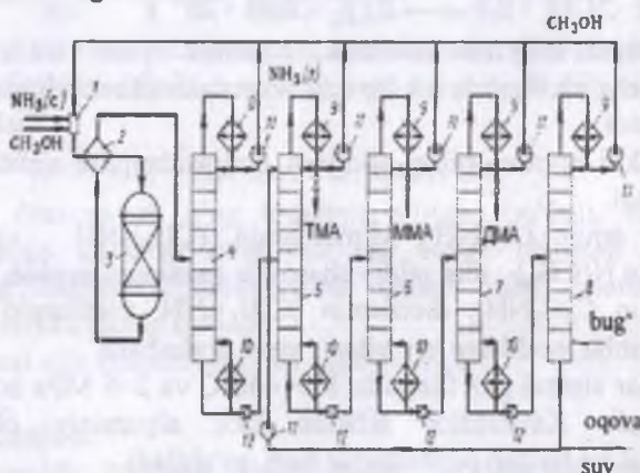
35- rasm. Metilamin ishlab chiqarish texnologiyasi:
