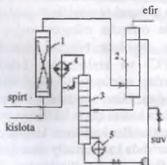
32-rasm. Sulfokationitlar ishtirokida sodir bo'ladigan eterifikatsiya jarayonining texnologik sxemasi: 1-reaktor;
