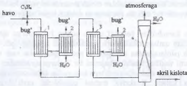
53-rasm. Propilenni ikki bosqichda oksidlash bilan akril kislota olish texnologik sxemasi: 1-birinchi bosqichda oksidlash reaktori; 2-qozon utilizatorlar; 3-ikkinchi bosqichda oksidlash reaktori; 4-absorber.
