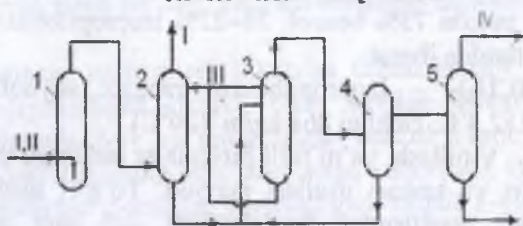
39-rasm. Atsetilen va vodorod sianiddan akrilonitril olish texnologiyasi: 1- reaktor; 2- absorber; 3- bug'latish kolonnasi; 4- separator; 5- akrilonitrilni tozalovchi rektifikatsiya kolonnasi.
