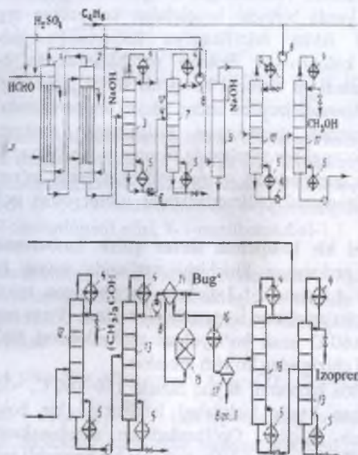
58-rasm. Izobuten va formaldegiddan izopren olish texnologik sxemasi: 1,2- 1- bosqich reaktorlari, 3,7,10,13,18,19- rektifikatsiya kolonnalari; 4-deflegmator, 14-issiqlik almashtirish, 15-2 bosqich reaktori; 16-sovutgich; 5-qaynatgich; 6-drossel ventili; 8-nasoslar; 9-neytralizator; 17-separator.
