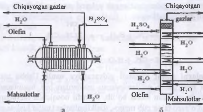
27-rasm. Etilen va propilenni sulfat kislota bilan gidratlash qurilmalari: a) diskli aralashtirgichli gorizontaal absorber; b) uzluksiz ravishda ishlaydigan tarekali-kolonnali absorber.
