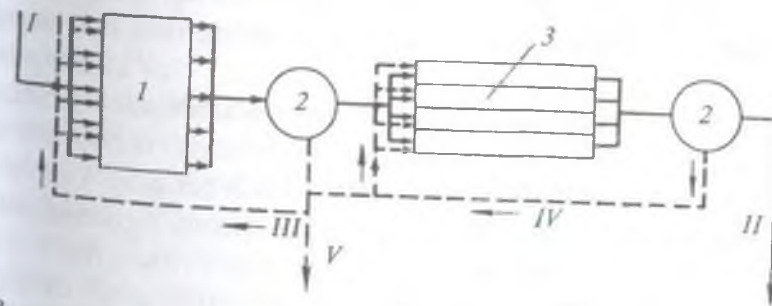
8- rasm. Aerotenklarda oqova suvlarning ikki bosqichli tozalash sxemasi. 1 — aerotank; 2 — ikkilamchi tintirgich; 3 — aerotank reaktorlar; I — oqova suvlari tozalashga; II — oqova suvining tozalangani; III — birinchi bosqich aktiv balchig'i; IV — ikkinchi bosqich aktiv balchig'i; V — ortiqcha aktiv balchiq.
