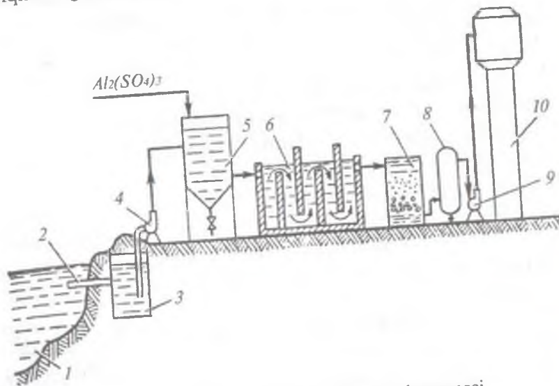
12- rasmda. Ichimlik suvini tayyorlash sxemasi. 1 — suv manbai; 2 — suv olish joyi; 3 — dag'al tindirgich; 4 — birinchi ko'tarib beruvchi nasos; 5 — aralashtirgich; 6 — tindirgich; 7 — filtrlash; 8 — xlorator; 9 — ikkinchi ko'tarib beruvchi nasos; 10 — suv bosimi minorasi.
