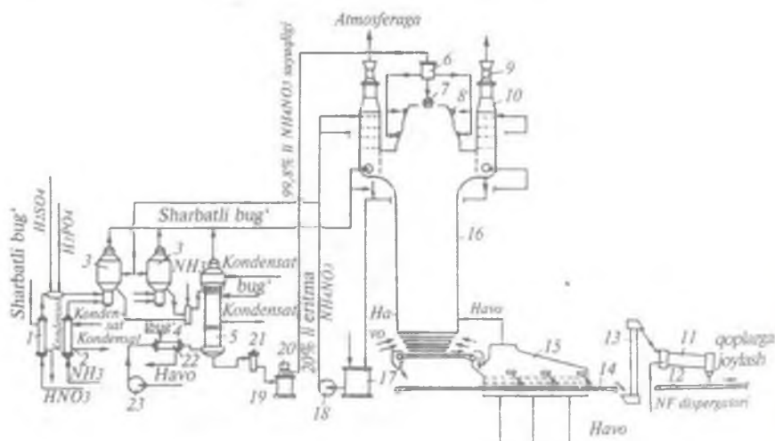
71- rasmda. Ammoniy nitrat ishlab chiqarish agregatining AS-72 sxemasi.
