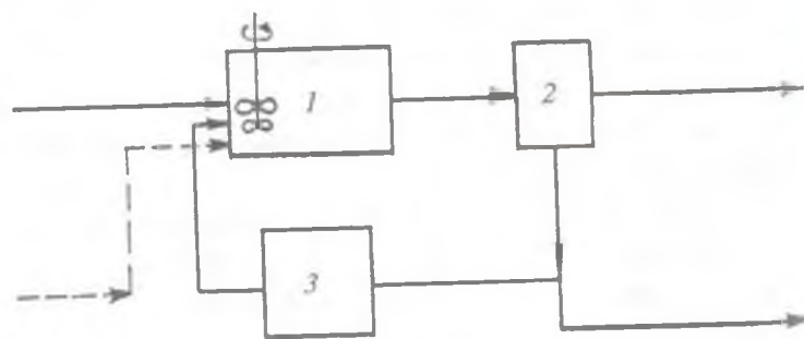
17- rasm. Oqova suvlarni biologik tozalash qurilmasining sxemasi 1 — aerotank; 2 — ikkilamchi tintirgich; 3 — balchiq regeneratori.
