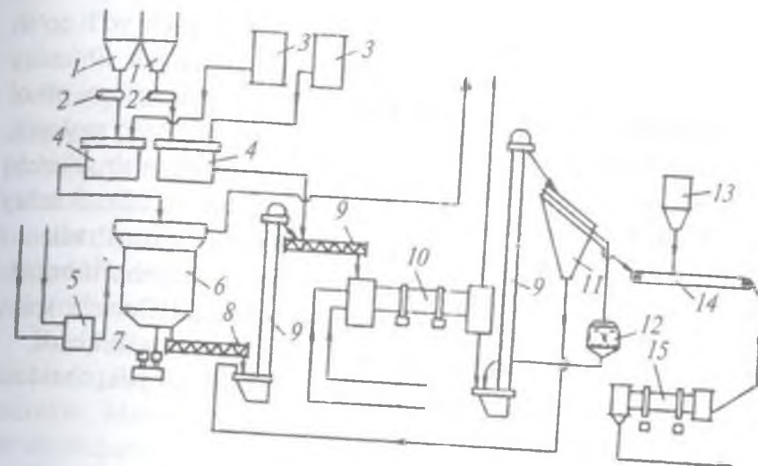
78- rasm. Fosforit uni va ekstraksiyon fosfat kislotasidan donador qo'sh superfosfatni uzluksiz ishlab chiqarish sxemasi.
