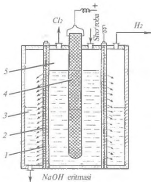
83- rasm. Filtrlovchi diafragma elektroliz vannasining sxemasi.
