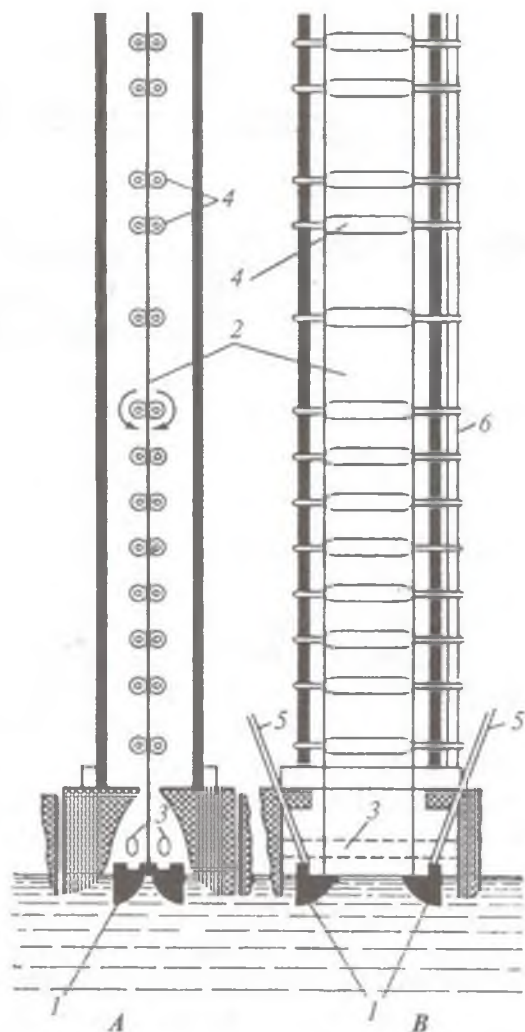
81- rasm. Shisha listini shisha suyuqlanmasidan choʻzib tayyorlash.
