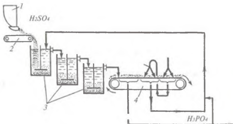
77- rasm. Ekstraksiya usuli bilan fosfat kislota ishlab chiqarish. 1 — bunker; 2 — tasmali dozalogich; 3 — ekstraktorlar; 4 — tasmali vakuum filtr.
