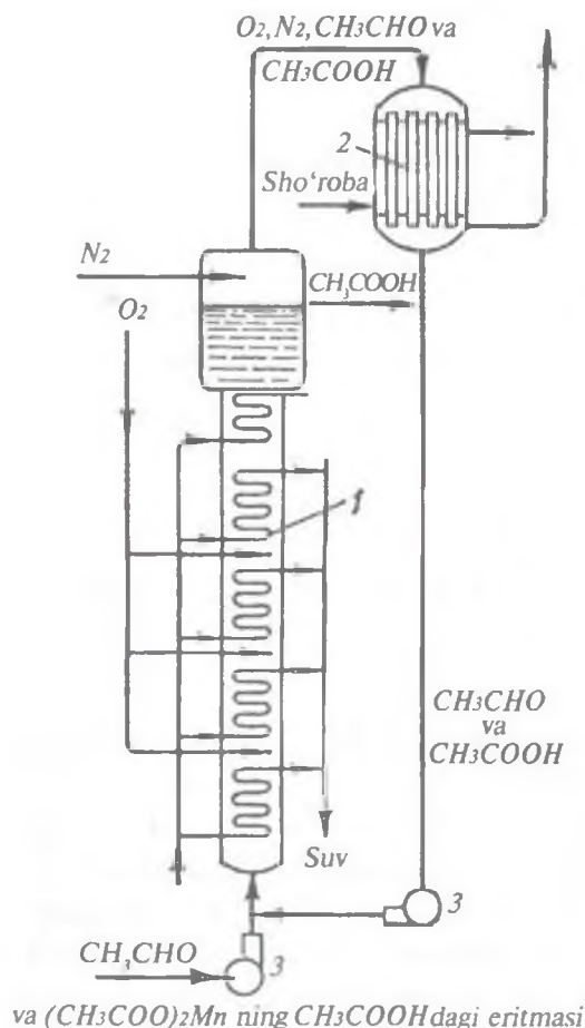
109- rasm. Sirka aldegidni oksidlab sirka kislotasi olish sxemasi. 1 — oksidlash minorasi(kolonna) 2 — kondensator; 3 — nasoslar.
