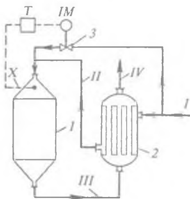
1- rasm. Reaktorning harorat rejimini oddiy avtomatlashtirish sxemasi.
