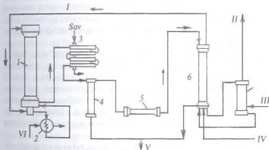
62- rasm. O'rta bosimda ammiak ishlab chiqarish sxemasi.
