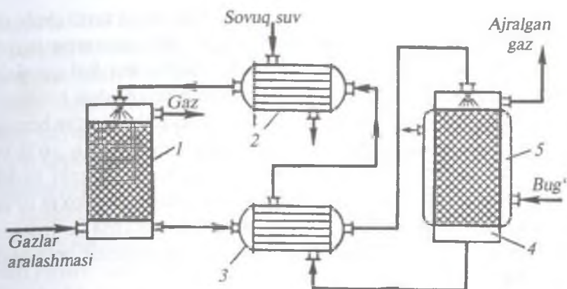
9- rasm. Absorbsiya – desorbsiya usulida gazlarni ajratish qurilmasining sxemasi.
