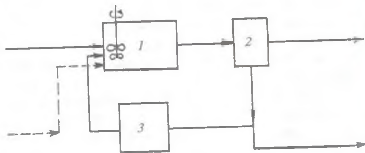
17- rasm. Oqova suvlarni biologik tozalash qurilmasining sxemasi 1 — aerotenk; 2 — ikkilamchi tintirgich; 3 — balchiq regeneratori.
