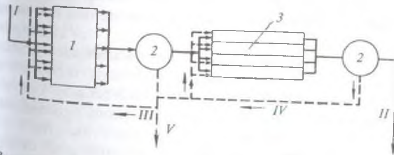
18- rasm. Aerotenklarda oqova suvlarning ikki bosqichli tozalash sxemasi. 1 — aerotenk; 2 — aralashtirgich; 3 — aerotenk reaktorlar; I — oqova suvlari tozalashga; II — oqova suvining tozalangani; III — birinchi bosqich aktiv balchiq'i; IV — ikkinchi bosqich aktiv balchiq'i; V — ortiqcha aktiv balchiq.
