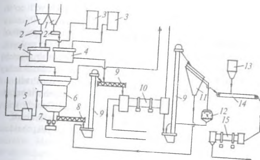
78- rasm. Fosforit uni va ekstraksion fosfat kislotasidan donador qo'sh superfosfatni uzluksiz ishlab chiqarish sxemasi. 1 — Fosforit uni uchun bunker; 2 — massa dozalogich; 3 — fosfat kislotasi uchun bosimli bak(idish); 4 — reaktor; 5 — yoqilg'i; 6 — sachratib qurutuvchi; 7 — taroqsimon uzatma; 8 — shnek; 9 — elevator; 10 — baraban quritgich; 11 — g'alvir; 12 — maydalagich; 13 — maydalangan bo'r bunker; 14 — tasmali transportyor; 15 — baraban neytrallagich.
