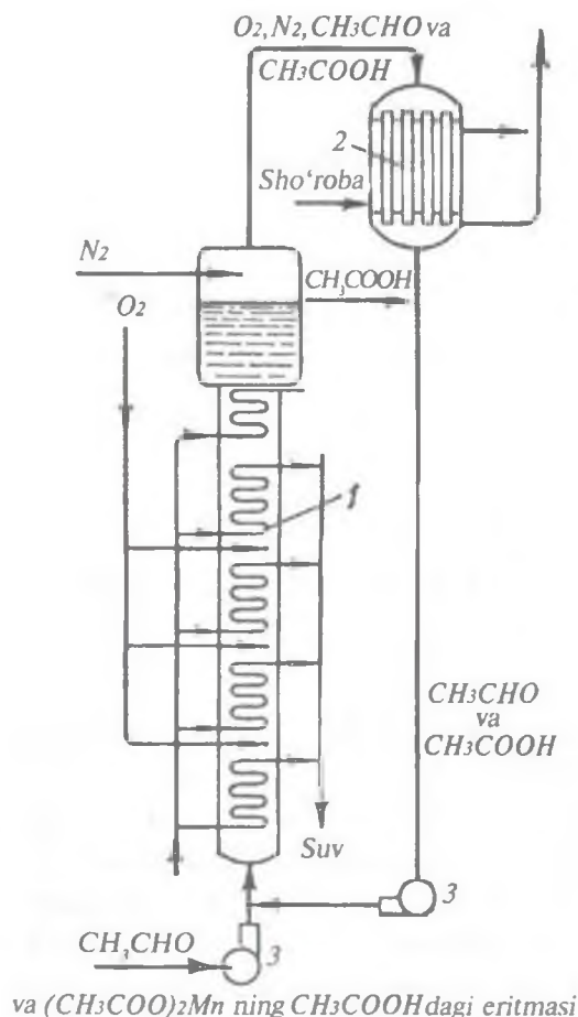
109- rasm. Sirka aldegidni oksidlab sirka kislota olish sxemasi. 1 — oksidlash minorasi(kolonna) 2 — kondensator; 3 — nasoslar.
