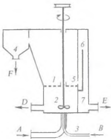
8- rasm. Aralashtirib flotatsiyalash mashinasining bo'lmasi.
