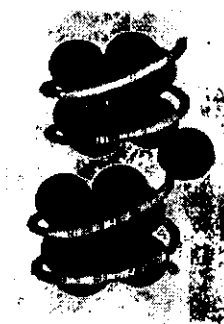
21-rasm. Nukleosoma
