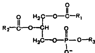
Glitserofosfolipid
