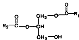
Diglitserid
