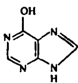
gipoksantin
