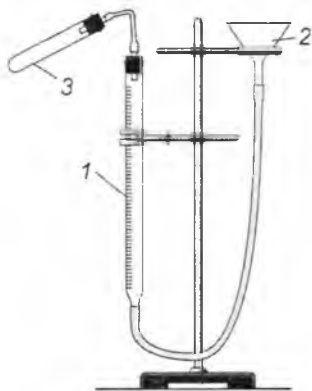
20-rasm. Ekvivalent aniqlanadigan asbob: 1 — 100 ml li byuretka; 2 — voronka; 3 — probirka.
