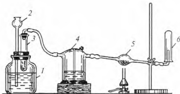
24-rasm. Oksid tarkibini aniqlash asbobi.
