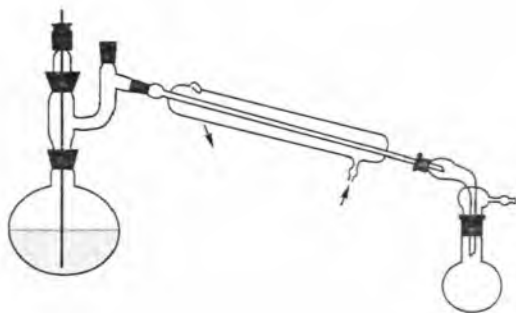
18-rasm. Vakuumda haydash asbobi.
