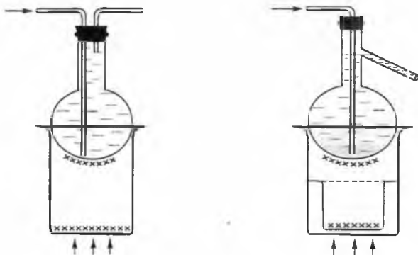
15-rasm. Moddalarni sublimatlash yo'li bilan tozalash.
