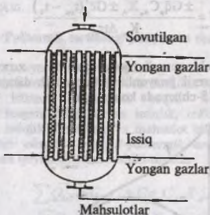
3.16-chizma. Endotermik reaksiyalar uchun katalitik quvurli reaktor.
