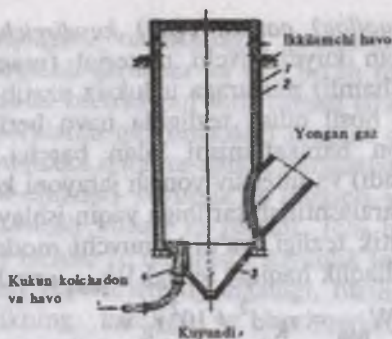
4.7-chizma. Chang holda yondirish kuydirgichi: 1 — tashqi qobiq; 2 — himoya qatlami; 3 — bunker; 4 — forsunka;
