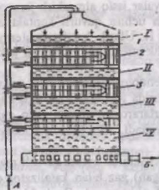
5.13-chizma. Katalizator qatlamlari o'rtasida (oralig'ida) issiq almashtirgichli tokchalı kontakt apparati: 1 — panjara; 2 — issiqlik almashtiruvchi quvurlar; 3 — to'siqlar; 1, 2, 3, 4 — katalizator qatlamlari; A — kirayotgan gaz; B — chiqayotgan mahsulot.
