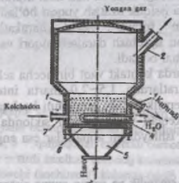
4.8-chizma. «Qaynoq» qatlamda yondirish kuydirgichi:
