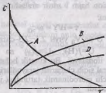
2.3-chizma. Binar parallel qaytmas A \xrightarrow{k_1} B reaksiyada k_1 > k_2 bo'lganda konsentratsiyalar o'zgarishi.
