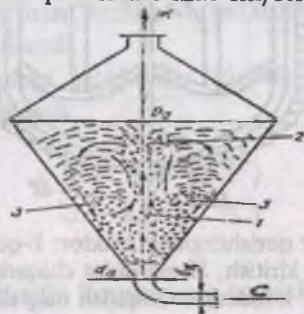
4.13-chizma. Favvora qatlamli reaktor: 1 – favvora yadrosi; 2 – favvora; 3 – zich tushuvchi qatlam; D_a – favvora zonasida reaktor diametri; d_k – reaktorning ostki bo'g'zi diametri; d_k – quvur diametri.
