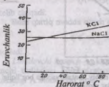
4.18-chizma. Kaliy va natriy xloridlarning harorat ta'sirida eruvchanligi (suyulishi). 4.19-chizma. KCl — NaCl — H 2 O sistemada eruvchanlik diagrammasi (t q 25°C va 100°C).
