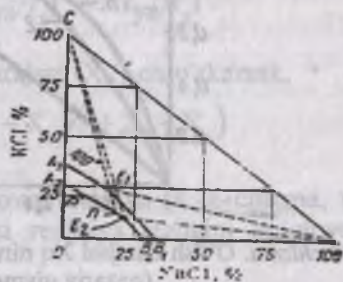
4.18-chizma. Kaliy va natriy xloridlarning harorat ta'sirida eruvchanligi (suyulishi). 4.19-chizma. KCl — NaCl — H 2 O sistemada eruvchanlik diagrammasi (t q 25°C va 100°C).
