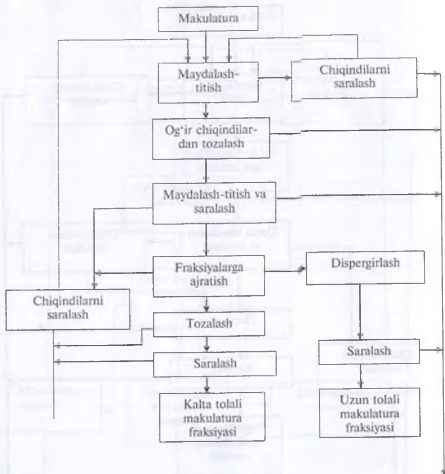
52-rasm. Qadoqlash va qalin qog'oz ishlab chiqarish uchun makulatura massasini tayyorlash sxeması.
