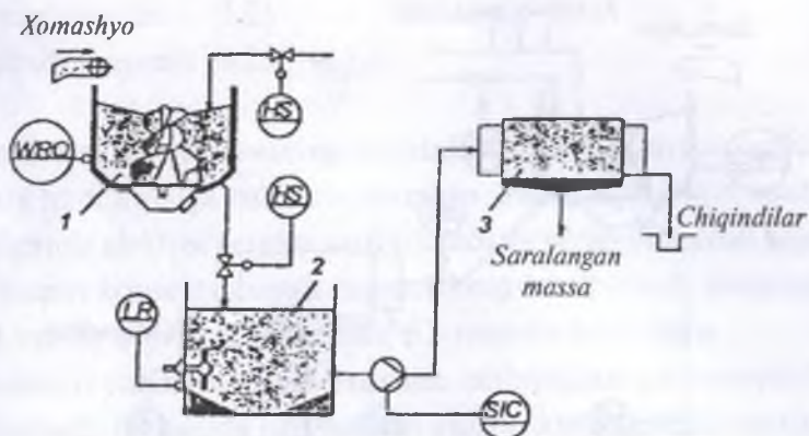
60-rasm. Laminirlangan qog'oz va qalin qog'oz qutilarini (sharbat, sut va boshqalar) davriy usulda maydalash-titish sxemasi: 1—gidromaydalagich; 2—massa basseyini; 3—saralash barabani; WRQ — massa konsentratsiyasi va sarfini belgilab borish; LR — sathni boshqarish; HS — qo'l bilan boshqarish; SIC — aylanish chastotasini boshqarish.
