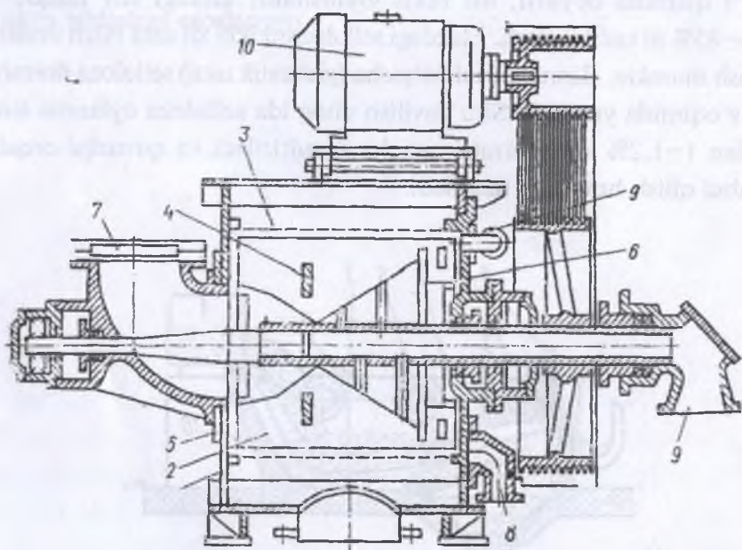
17-rasm. CIIC turdagi markazdan qochma ajratkich: 1–kojux; 2–rotor; 3–silindrik elak; 4–to'siq; 5–old tomon; 6–orqa qopqoq; 7–massaning kirish qismi; 8–chiqindilarni chiqarish joyi; 9–suyultirish suvining tarnovi; 10–elektroharakatlantiruvchi.
