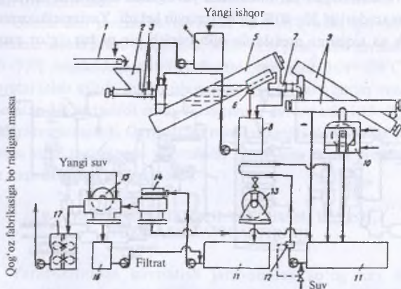
29-rasm. Sovuq-natron usulida yarimselluloza olish texnologik sxemasi: 1—payraha konveyeri; 2—bunker; 3—qabul qiluvchi; 4—o'chovchi; 5—reaksiyaviy quvur; 6—ortiqcha ishqorni suzib oluvchi to'r; 7—ortuvchi; 8—aylanma ishqor baki; 9—vintli konveyer; 10—xemifayner; 11—massa basseyini; 12—konsentratsiya boshqaruvchi; 13—diskli tegirmon; 14—selektifayner; 15—vakuum-filtr; 16—aylanma suv baki; 17—yuqori konsentratsiyadagi massa hasseyini.
