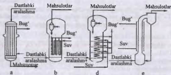
52-rasm. Geterogen-katalitik oksidlash reaktorlari.
