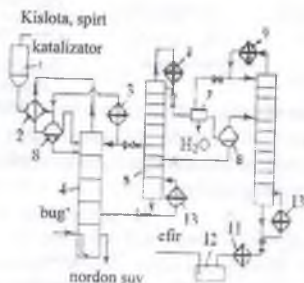
31-rasm. Uzluksiz usul bilan etilatsetat olish texnologiyasi:
