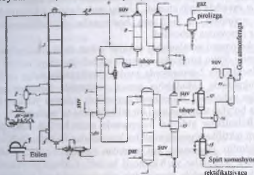
28-rasm. Etanol olish texnologiyasi:
