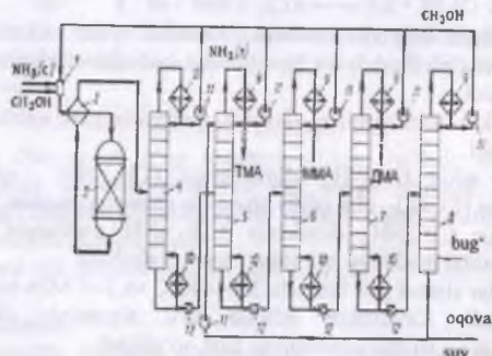
35- rasm. Metilamin ishlab chiqarish texnologiyasi:
