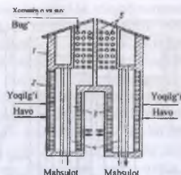
3-rasm. Piroliz pechining sxemasi:
