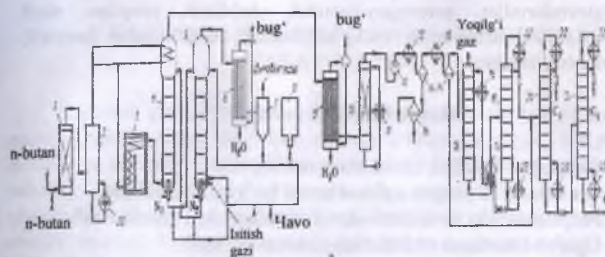
57-rasm. Parafinlarni birinchi bosqichda degidrlash texnologik sxemasi. 1-qurutgich; 2-bug'latgich; trubkasimon pech; 4-reaktor; 5-regenerator; 12-kompressor; 14-separator; 16-absorber; 17-issiqlik almashtirgich; 6,9-utilizator-qozon; 7-elektrofiltr; 8-bunker; 10-srubber; 11,13,15,19-sovutgichlar; 18-bug'latish kolonkasi; 20,21-rektifikatsiya kolonnalari; 22-deflegmatorlar; 23-qaynatgich.
