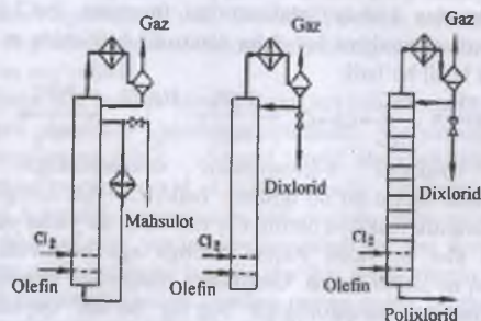
21-rasm. Suyuq fazada ion katalitik xlorlash reaktori:
