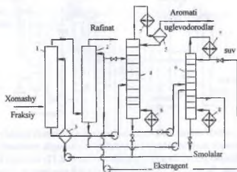
9-rasm. Aromatik uglevodorodlarni ekstraksiya usuli bilan ajratish texnologik sxemasi: 1,4 rektifikatsiya kolonnalari; 2-skrubber; 3- issiq almashtirgich; 5-separator; 6-ekstragentni rekuperatsiyalash kolonnasi; 7- deflegmatorlar; 8-qaynatgichlar.
