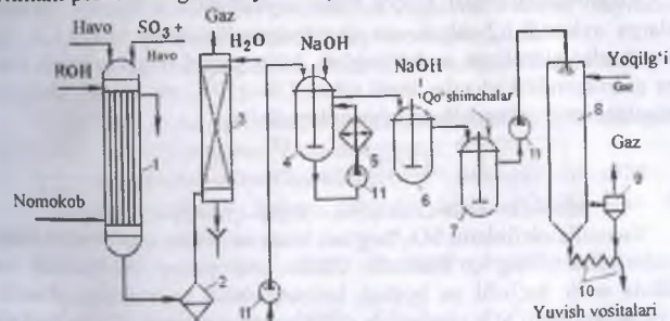
44-rasm. Alkilsulfatlar asosida olinadigan yuvish vosialari ishlab chiqarish texnologiyasi: 1-reaktor; 2- separator; 3- absorber; 4,6-neytralizatorlar; 5- sovitgich; 7-aralashtirgich; 8- quritgich; 9-siklon; 10-shnek; 11-nasoslar.
