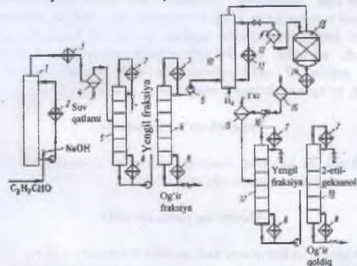
61-rasm. 2-etilgeksanol olish texnologik sxemasi: 1-reaktor; 2,3,11,14- sovutgichlar; 4,15- separatorlar; 5,6,17,18- rektifikatsiya kolonnalari; 7-deflegmatorlar; 8-qaynatgichlar; 9- nasos; 10,13- gidrirlash kolonnalari; 12- filtr; 16-drosselli ventill.
