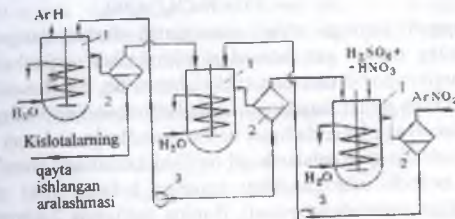
47-rasm. Aromatik birikmalarni nitrollash reaksiya qurilmasi: 1-nitratlar; 2-separatorlar; 3-nasoslar.
