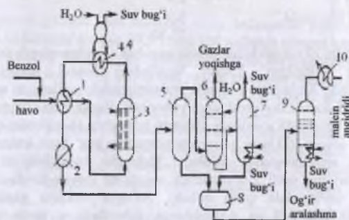
55-rasm. Benzolni gaz fazasida oksidlash bilan malein anhidridi ishlab chiqarish texnologik sxemasi: 1- issiqlik almashtirgich; 2-sovutgich; 3-reaktor; 4-utilizator qozon; 5- separator; 6- skrubber; 7-degidrator; 9- rektifikatsiya kolonnasi; 10- kondensator sovutgich.
