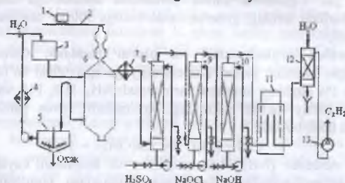
12-rasm. Kalsiy karbiddan atsetilen olish texnologiyasi:
