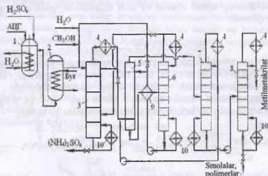
26-rasm. Atsetonsiangidrididan metilmetakrilat olish texnologik sxemasi: 1–aralashtirgich; 2 – reaktor; 3– efrizator; 4– kondensator-deflegmatorlar; 5 – ekstraktor; 6 – bug'latish kolonnasi; 7,8 – rektifikatsiya kolonnalari; 9,10–issiqlik almashtirgich.
