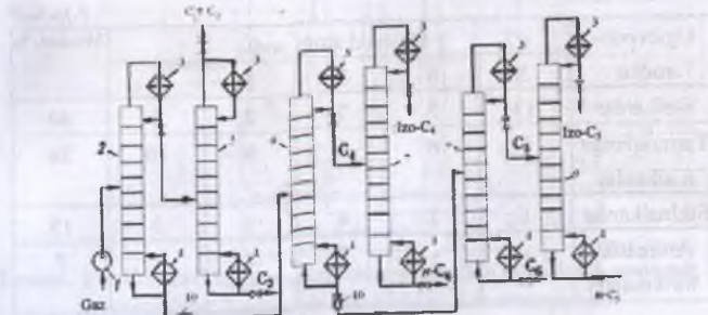
1-rasm. C 1 -C 5 uglevodorodlarini ajratish texnologik sxemasi: 1- kompressor; 2,5,6,7,8,9-rektifikatsiya kolonnalari; 3-deflegmatolar; 4- qaynatgichlar 10-drossel ventili.
