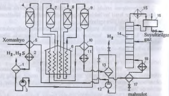
6-rasm Platforming jarayoni texnologik sxemasi:
