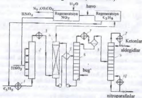
48-rasm. Propanni nitrollash texnologik sxemasi:
