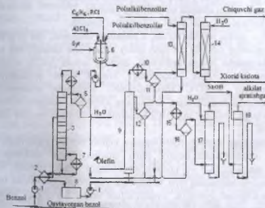
1-nasoslar; 2- issiqlik almashtirgich; 3- benzolni quritish kolonnasi; 4,10- kondensapitorlar; 5- separator; 6- katalitik kompleks hosil qiluvchi apparat; 7- qaynatgich; 8- yig'gich; 9- alkilator; 11- gaz ajratgich; 12,16-separatorlar; 13- absorber; 14- suv skrubber; 15- sovutgich 17,18-yuvish kolonnalari.
