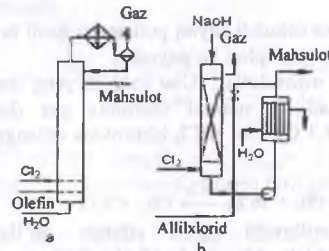
22-rasm. Xlorgidrinlash reaktori: a) qaytar kondensatorli barbotajli kolonna; b-retsirkulyatsiyali trubkasimon reaktorda alohida gipoxlorlash va xlorgidrinlash moslamasi.
