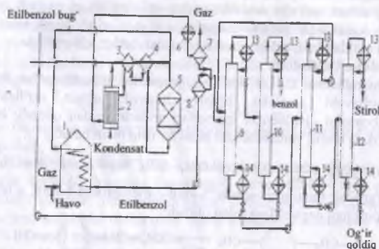
56-rasm. Stirol ishlab chiqarish texnologik sxemasi:
