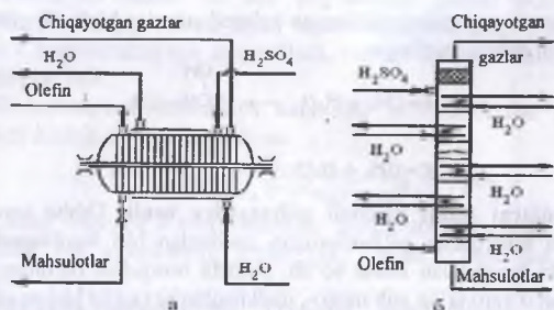
27-rasm. Etilen va propilenni sulfat kislotasi bilan gidratlash qurilmalari: a) diskli aralashtirgichli gorizontal absorber; b) uzluksiz ravishda ishlaydigan tarelkali-kolonnali absorber.
