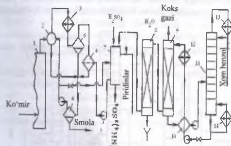
8-rasm. Toshko'mirni kokoslash mahsulotlarini kondensatsiyalash va yengil mahsulotlarini ajratishni texnologik sxemasi:
