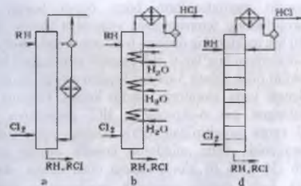
17-rasm. Suyuq fazada radikal-zanjirli xlorlash xloratorlar:
