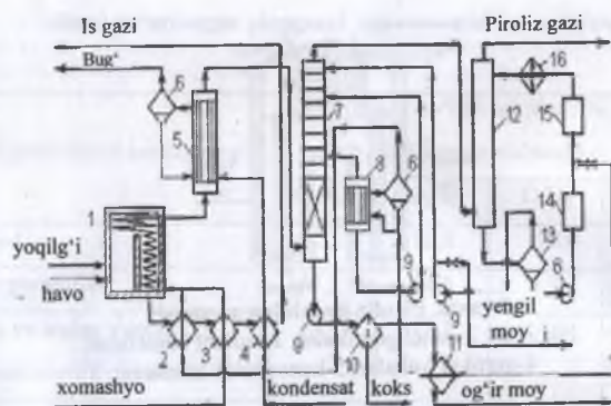
4-rasm. Benzinni piroliz qilish texnologik sxemasi:
