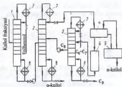
10-rasm. Izomerlanish bilan birgalikda olib boriladigan kisilol fraksiyalarini ajratish texnologik sxemasi: 1-etil benzolni haydash kolonnasi, 2-o-kisilolni ajratish kolonnasi, 3-yengil va og'ir fraksiyalarni ajratish kolonnasi, 4,5-1 va 2 bosqichli kristallash moslamalari, 6-izomerlanish qurilmasi, 7-deflegmatorlar 8-qaynatgichlar.
