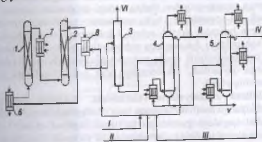
33-rasm. Seolitli katalizatorlar ishtirokida benzolni alkillash bilan izopropilbenzol olish texnologik sxemasi: I-alkillash reaktori;
