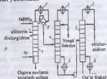
24-rasm. Epixlorgidrin olish texnologiyasi sxemasi:
