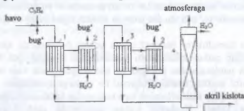
53-rasm. Propilenni ikki bosqichda oksidlash bilan akril kislotasi olish texnologik sxemasi: 1-birinchi bosqichda oksidlash reaktori; 2-qozon utilizatorlar; 3-ikkinchi bosqichda oksidlash reaktori; 4-absorber.
