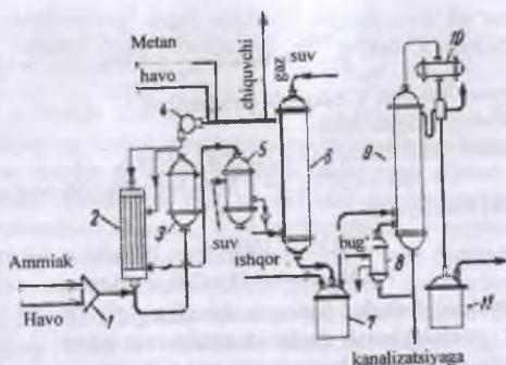
40-rasm Metanni oksidlash usuli bilan formaldegid olish texnologik sxemasi: 1-gorelka; 2-issilik almashtirgich; 3-reaktor; 4-gaz purkagich; 5-suv sovutgich; 6-suv skrubberi; 7-formaldegid eritmasini neytrallovchi idish; 8-qaynatgich; 9-rektifikatsiya kolonnasi; 10-deflegmator; 11-formaldegid yig'gich.
