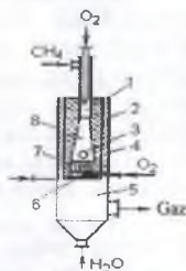
13-rasm. Metandan atsetilen olishda qo'llaniladigan oksidlanish piroliz reaktorining sxemasi: 1-aralashtirish kamerasi; 2-korpus; 3-saqlovchi; 4-yonish kamerasi; 5-pastki kamera; 6-purkagich; 7-yondirish plitasi; 8- diffuzor.
