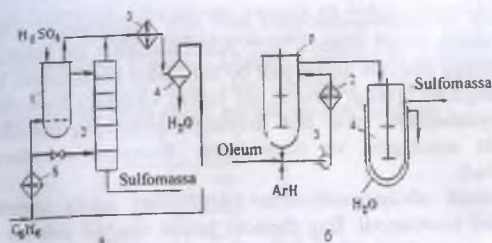
45a-rasm. Benzolni bug'da sulfirlash sxemasi:
