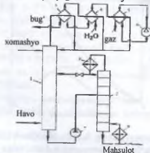
51-rasm. Benzin yengil fraksiyasini oksidlanish sxemasi:
