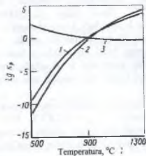
15-rasm. Konversiya reaksiyalarining temperaturaga bog'liqligi:
