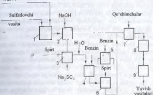
42-rasm. Alkilsulfat turidagi SFM ishlab chiqarishdagi asosiy jarayonlar sxemasi: 1- sulfatlash; 2- neytrallash; 3- natriy sulfatlash ajratish bo'limi; 4- ekstraksiya; 5- benzinni regeneratsiyalash va reaksiyaga kirishmagan organik reagentlarni ajratish; 6- spirt-erituvchini regeneratsiyalash; 7- yuvish vositalarini boshqa komponentlar bilan aralashtirish; 8- quritish; 9- maydalash va qadoqlash.
