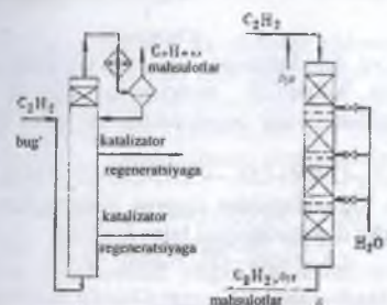
29-rasm. Atsetilen gidratatsiya reaksiya jihozining sxemasi:
