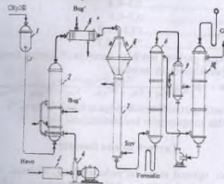
41-rasm. Metil spirtni oksidlash bilan formalin olish texnologik sxemasi: 1-o'lchagich; 2-bug'latgich; 3-filtr; 4-havo purkagich; 5-isitgich; 6-kontakt apparati; 7-sovutgich; 8, 10-absorberlar; 9-oraliq sovutgich.
