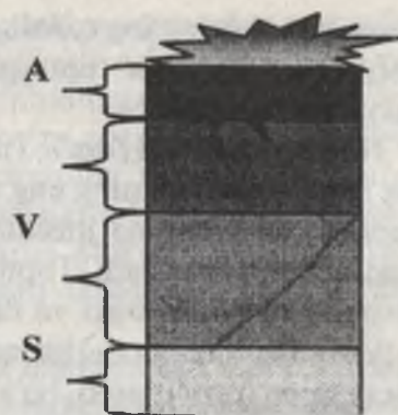
1-rasm. Tuproqning genetik qatlamlari
