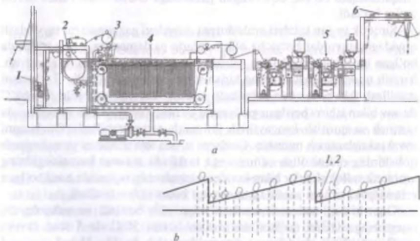
2.21- ras m. «Messera» qaynatish apparatining texnologik chizmasi (a) va apparat ichida gazlamaning harakatlanuvchi roliklar zanjiriga ilish chizmasi (b):
