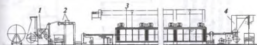
5.10- rasm. «Famateks» firmasining quritish-kengaytirish mashinasining chizmasi:
