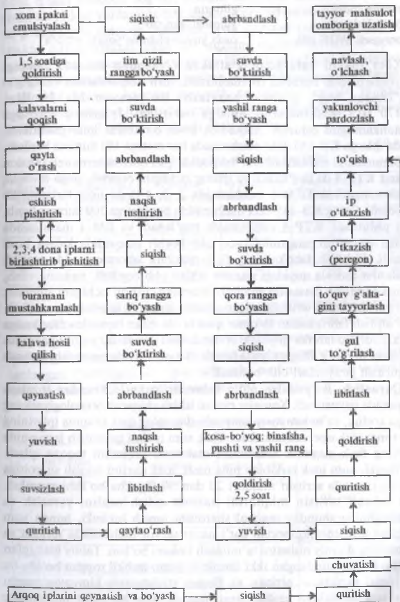
4.17- rasm. Abri matolar ishlab chiqarish texnologik ketma-ketligi.
