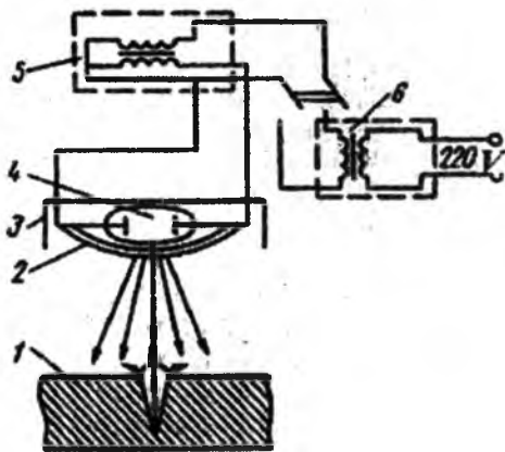
9.8-rasm. Kapillyar usulda detallarni tekshirish sxemasi:
