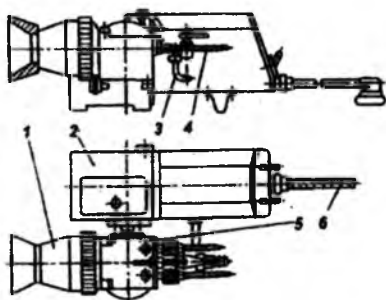
9.13-rasm. EM-12M elektrometallizatorining sxemasi:
