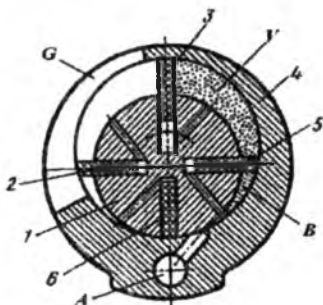
8.6-rasm. Ratatsion pnevmodvigatelning ishlash sxemasi:
