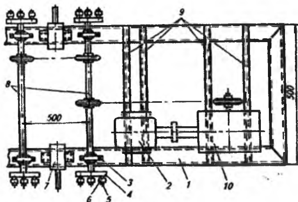
10.11-rasm. Ikkita aravachani obkatkash stendi:
