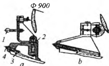
5.5-rasm. Jilvirlash aylanalarini aylana radiusi (a) va chekka aylanasi (b) bo'yicha qattiq qotishmali disklar yordamida to'g'rilash: 1 – dastak; 2 – taqalish tayanchi; 3 – bolt; 4 – gayka.
