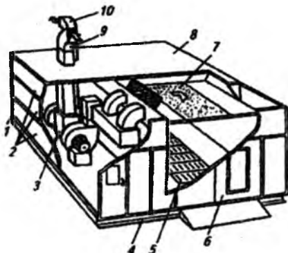
12.2-rasm. Bir ish joyiga mo'ljallangan bo'yash-quritish kamera qurilmasi:
