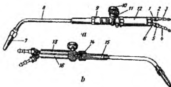
4.6-rasm. "Moskva" gorelkasining umumiy va qirqim ko'rinishi: 1 va 6 – shtutserlar; 2,5 va 9 – gaykalar; 3 va 4 – nipellar; 7 – mundshtuk; 8 – almashtiriluvchan uchlik; 10 va 11 – jo'mrak; 12 – dastak; 13 va 16 – kislorod va atsetelen quvurlari; 14 – injektor; 15 – aralashish kamerasi.
