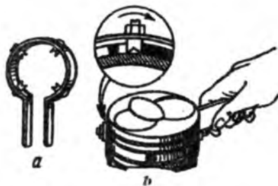
1.7-rasm. Prujinali siqgich yordamida porshen ariqchasidan qurumni tozalash: a —siqish qurilmasi; b —tozalash jarayoni.
