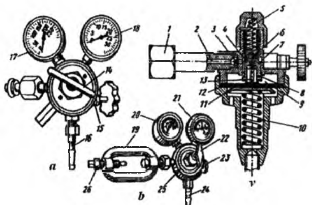
4.5-rasm. Gaz reduktorlari: a va b – kislorod reduktorining umumiy va qirqma ko‘rinishi; v – atsetelen reduktorining umumiy ko‘rinishi; 1 – gayka; 2 – gaz kanali; 3 – issiqlik so‘ndirgich; 4 – yuqori bosimli kamera; 5 – prujina; 6 – klapan; 7 – egarcha; 8 – qo‘yilma; 9 – ishchi kamera; 10 – bosh prujina; 11 – disk; 12 – membrana; 13 – o‘zak; 14 va 15 – jo‘mrak; 16 va 24 – nipellar; 17, 18, 20 va 21 – manometrlar; 19 – xamut; 23 – jo‘mrak; 25 – reduktor korpusi; 26 – saqlash vinti.
