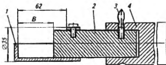
6.5-rasm. Polimer qorishmasini quyish moslamasi:
