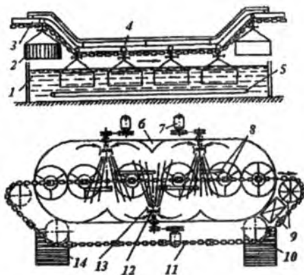
1.3-rasm. OM-5333 konveyerli yuvish mashinasining sxemasi:
