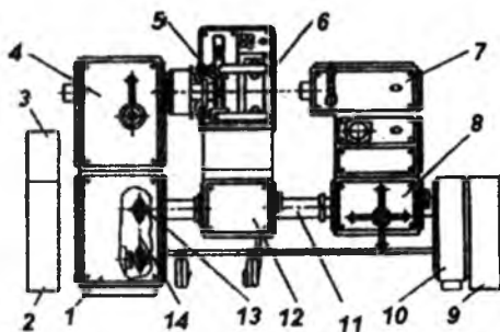
9.10-rasm. 011-1-10-Remdetal qoplama qoplash qurilmasining sxemasi:
