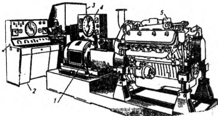
10.8-rasm. KH-136B tormozlab-obkatkalash stendining jihozlari: 1 – harakatga keltirish qurilmasi; 2 – boshqarish pulti; 3 – suyuqlik reostati; 4 – yuklash mexanizmi; 5 – sinalayotgan dvigatel.
