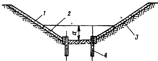
Рис. 44. Крепление откосов каналов:
