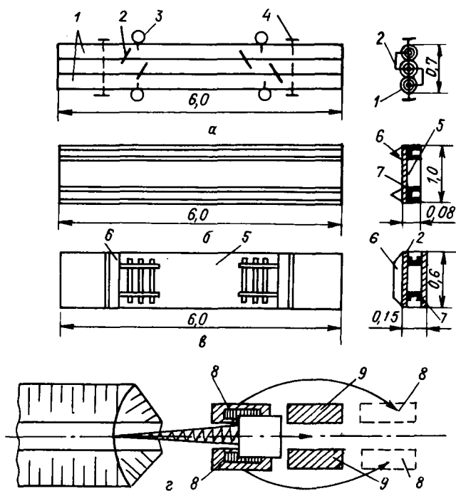
Рис. 30. Разработка грунта одноковшовыми экскаваторами со сланей:
