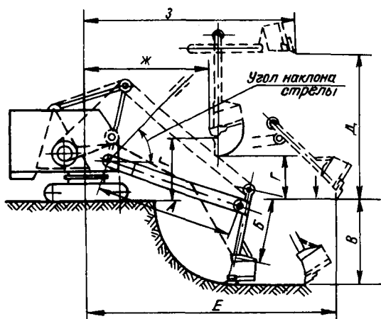
Рис. 41. Схема экскаватора Э-652Б с обратной лопатой:
