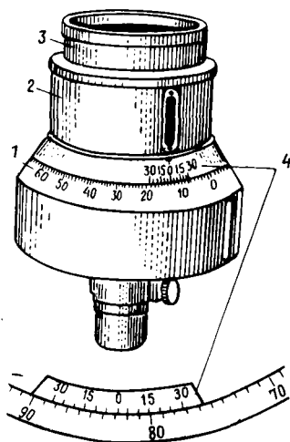
Рис. 6. Гониометр:
