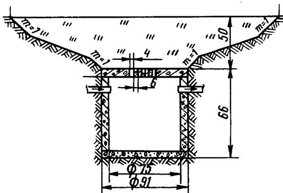
Рис. 21. Поглощающий колодец:
