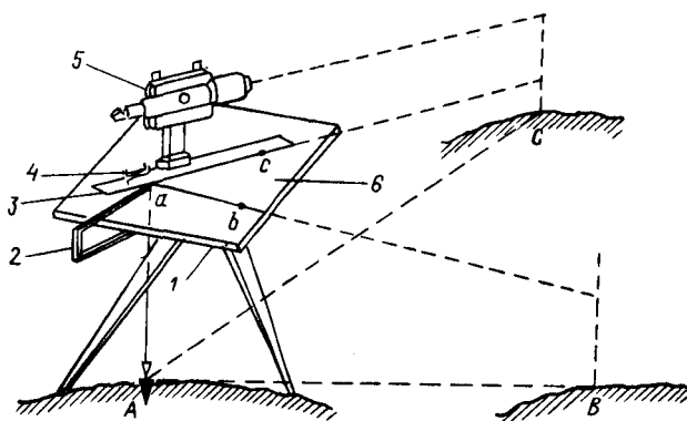
Рис. 7. Мензула:
