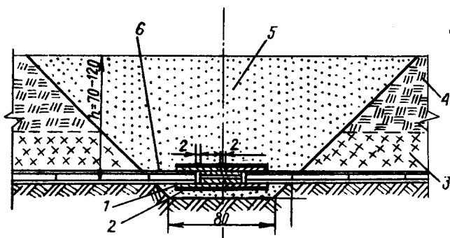
Рис. 22. Поглощительная колонка:
