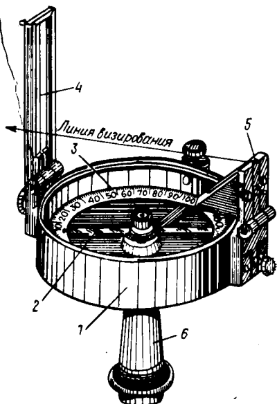
Рис. 5. Буссоль:
