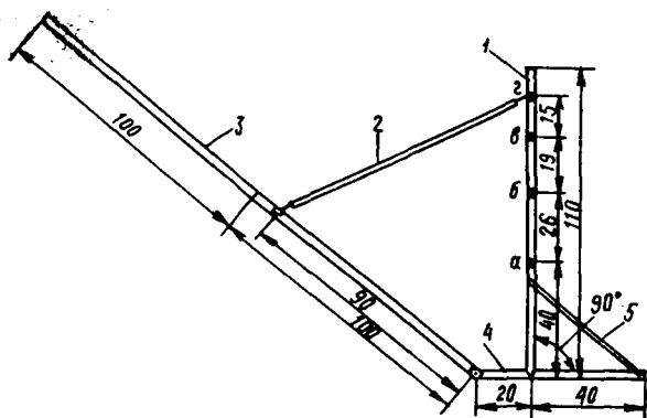
Рис. 63. Шаблон для измерения заложения откосов:
