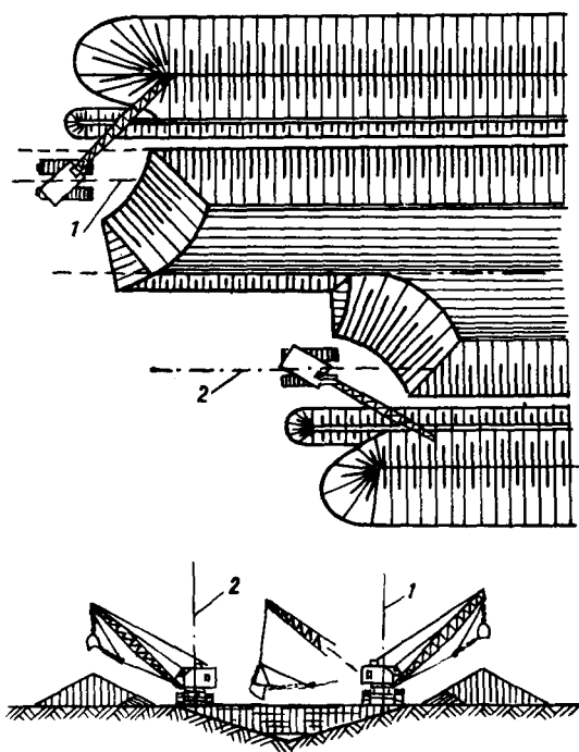
Рис. 29. Двухсторонняя разработка грунта:
