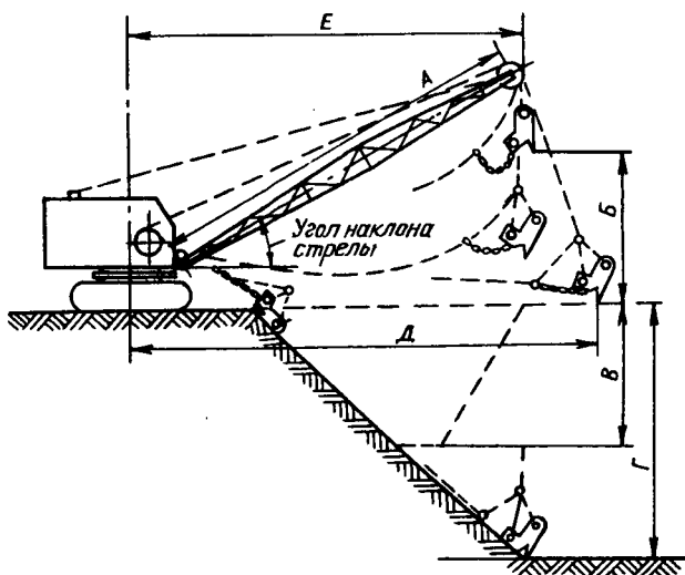
Рис. 40. Схема экскаватора Э-652Б с драглайном:
