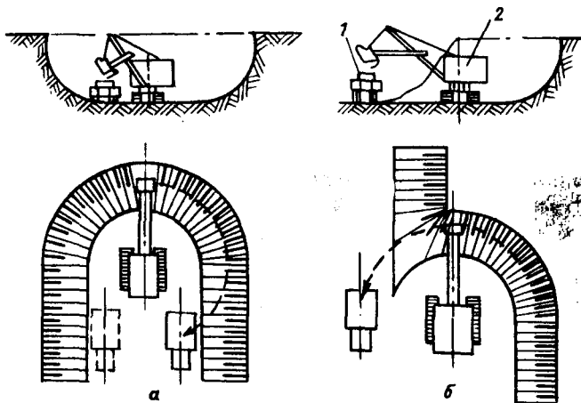
Рис. 31. Схема экскаваторного забоя при работе прямой лопатой с погрузкой и транспортными средствами:
