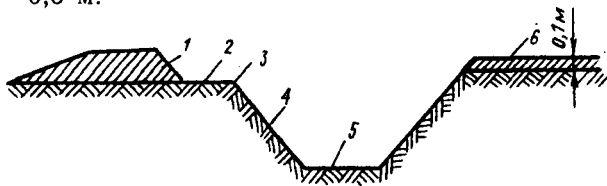
Рис. 38. Профиль осушительного канала:
