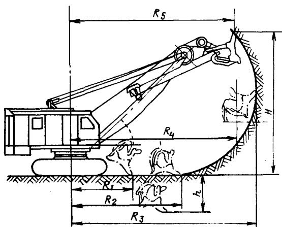
Рис. 42. Рабочие размеры экскаватора, оборудованного прямой лопатой:
