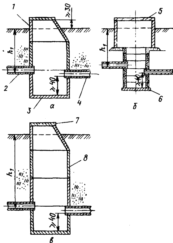
Рис. 20. Конструкции смотровых колодцев различных типов:
