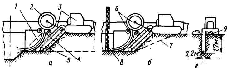
Рис. 47. Технологическая схема устройства узкотраншейного дренажа на осушительных системах:
