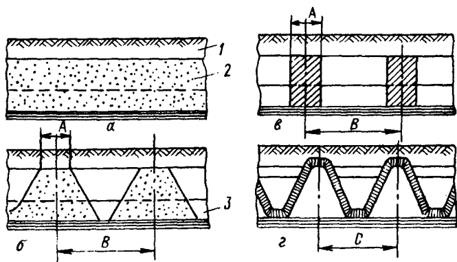
Рис. 51. Бестраншейный дренаж с фильтрующими элементами:
