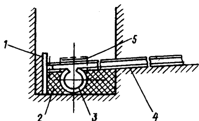
Рис. 48. Соединение дренажной линии с коллектором:
