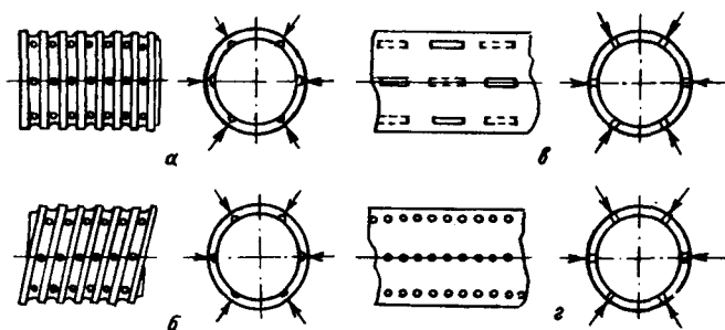
Рис. 24. Пластмассовые дренажные трубы:
