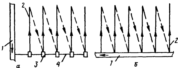
Рис. 50. Технологические схемы бестраншейной укладки дренажа:
