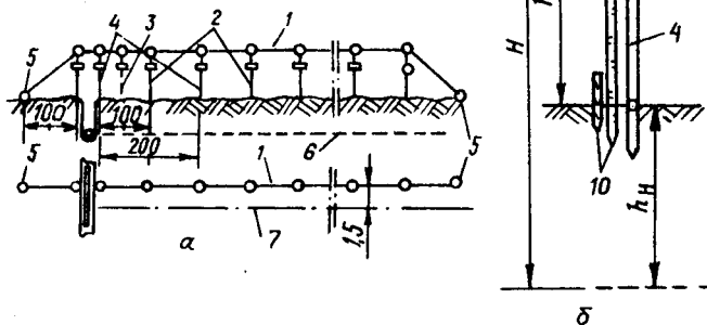
Рис. 45. Установка копирного троса на фиксирующие упоры:
