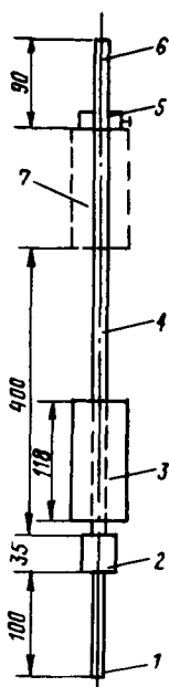
Рис. 57. Ударник ДорНИИ:
