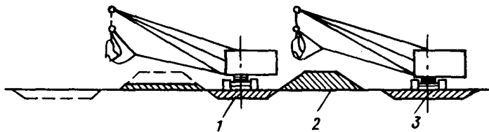
Рис. 36. Разработка канала драглайном в полунасыпи-полувыемке: 1 — канал; 2 — дамба; 3 — резерв
