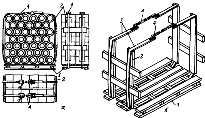
Рис. 26. Контейнеры для перевозки керамических труб:
