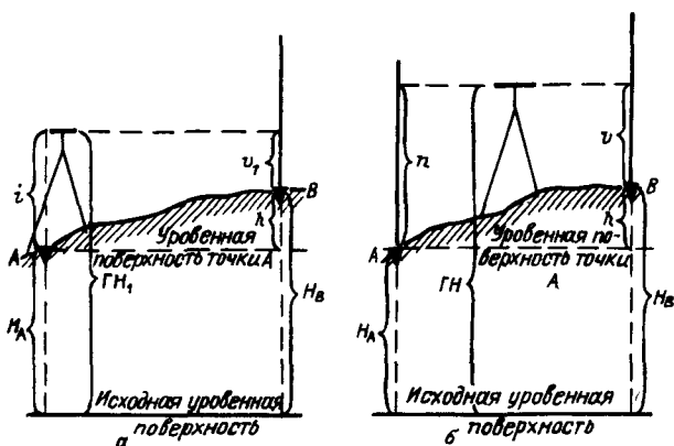
Рис. 12. Способы нивелирования:
