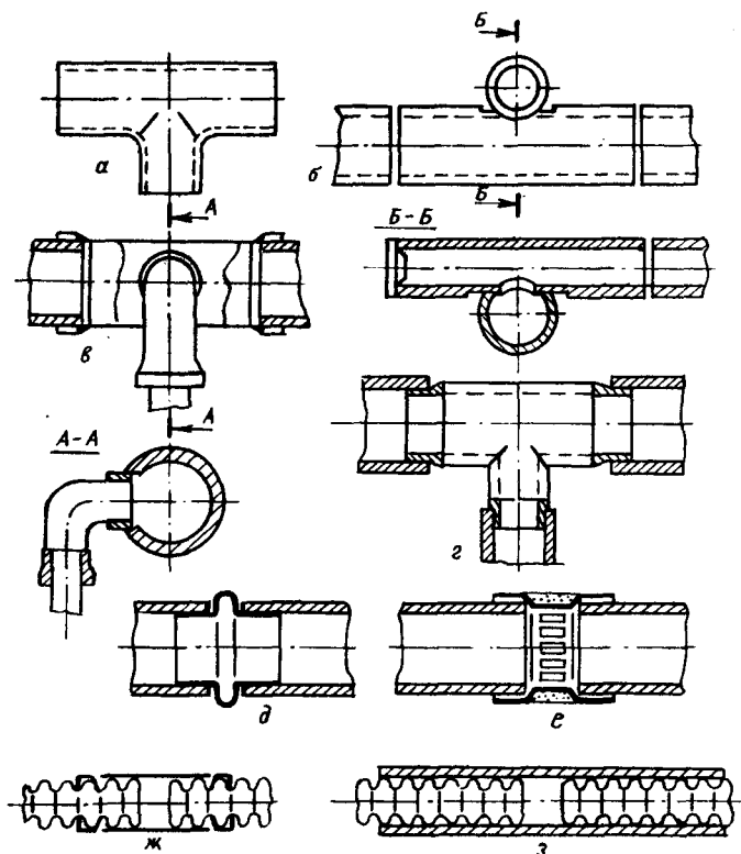
Рис. 25. Дренажная арматура:
