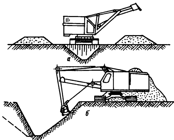
Рис. 33. Схема экскаваторного забоя при работе с обратной лопатой в отвал:
