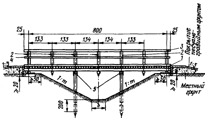
Рис. 17. Типовая конструкция деревянного пешеходного моста:
