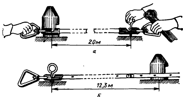
Рис. 1. Стальная мерная лента:
