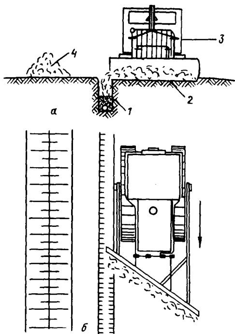
Рис. 49. Схема засыпки траншей гумусированным (растительным) грунтом:
