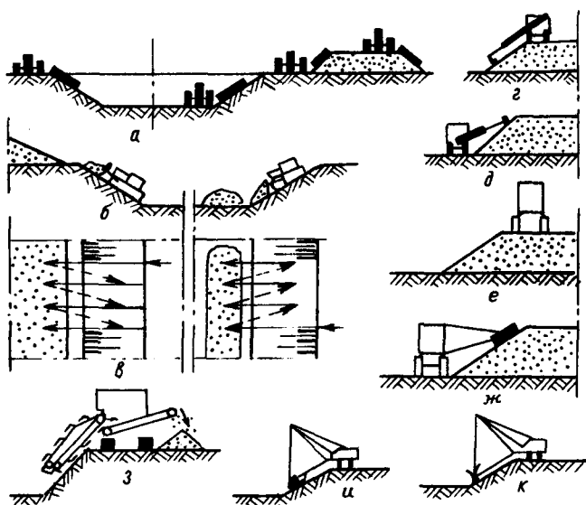
Рис. 43. Схема планировки откосов каналов:
