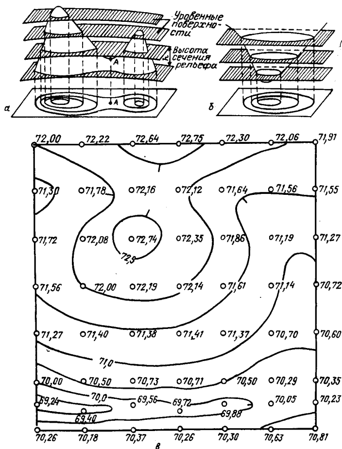
Рис. 9. Горизонталы:
