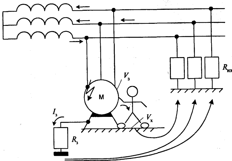
Рис. 20.3. Схема работы защитного заземления: R_{из} – сопротивление изоляции каждой из фаз относительно земли
