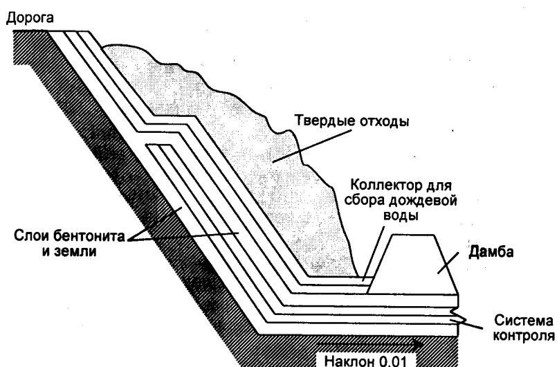
Рис. 4.7. Схема безопасного захоронения отходов
