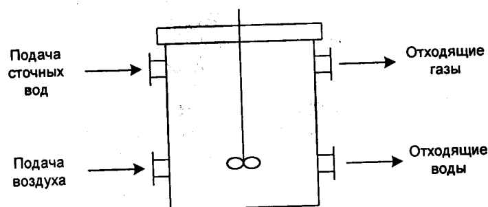
Рис. 4.5. Принципиальная схема окситенка
