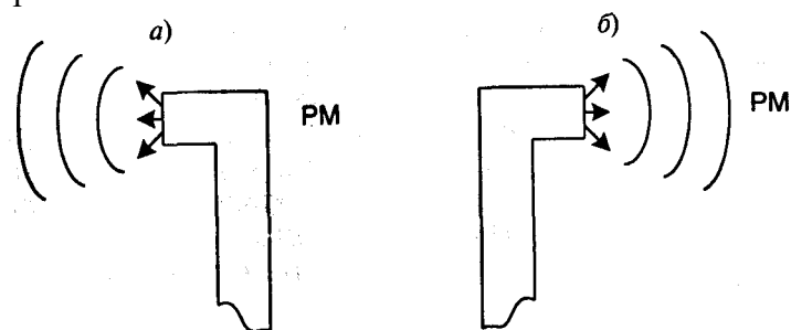
Рис. 17.3. Расположение трубы для сжатого воздуха в атмосферу: а) правильное; б) неправильное (PM — рабочее место)
