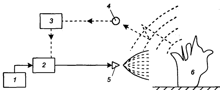
Рис. 22.1. Принципиальная схема автоматического пожаротушения: 1 — емкость для хранения огнетушащего вещества; 2 — оборудование для подачи огнетушащего вещества; 3 — система включения подачи огнетушащих веществ; 4 — устройство обнаружения пожара; 5 — устройство подачи огнетушащего вещества к очагу загорания (например, спринклерная и дренчерная головки); 6 — очаг загорания
