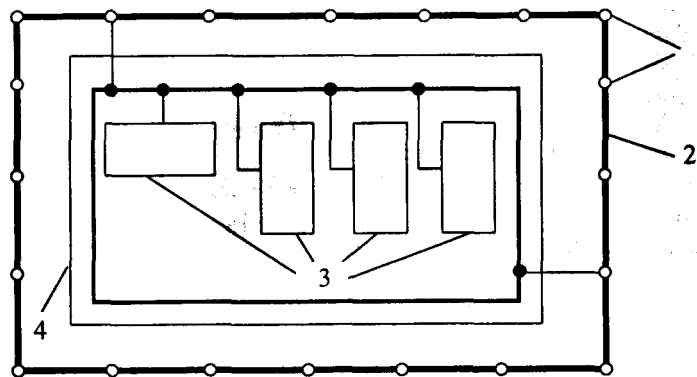
Рис. 20.5. Схема контурного заземления: 1 — заземлители; 2 — заземляющие проводники; 3 — заземляемое оборудование; 4 — производственное здание
