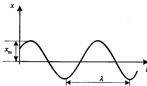
Рис. 17.1. Гармонические колебания
