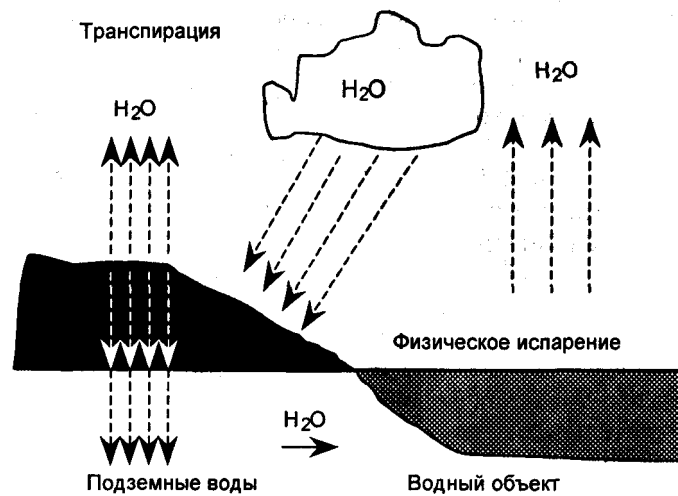
Рис. 1.3. Круговорот воды [21]
