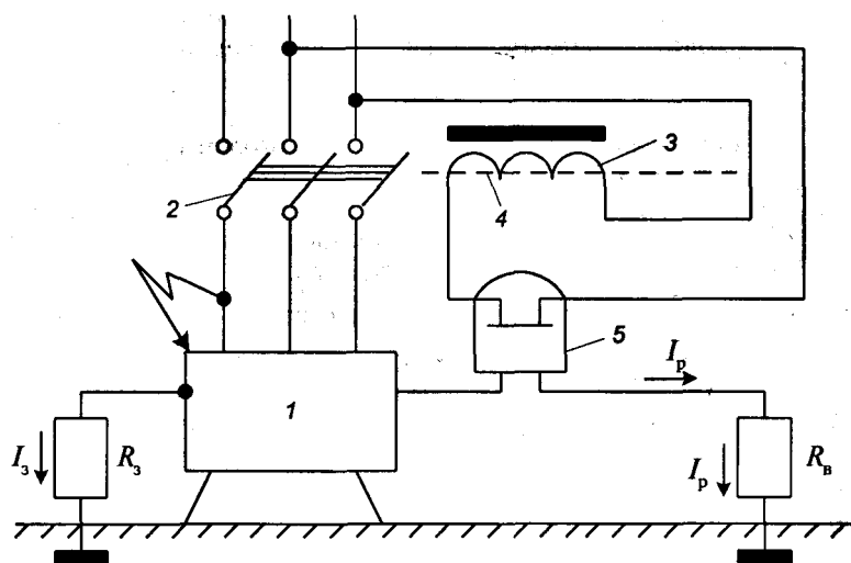
Рис. 20.8. Схема защитного отключения:
