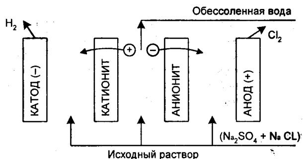
Рис. 4.6. Схема электродиализа
