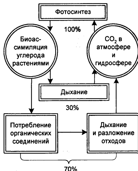
Рис. 1.2. Круговорот углерода [21]
