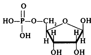
\beta -D-Рибозо-5-фосфат
