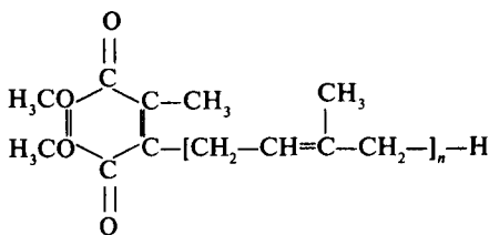
Убихинон
