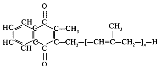
Менахинон (К 2 )
