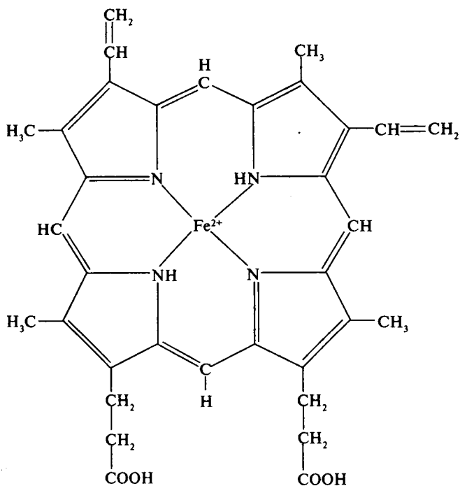
Рис. 6. Структура гема гемоглобина
