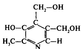
Пиридоксол
