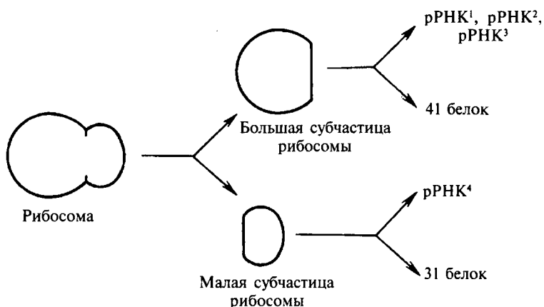
Рис. 17. Структура рибосомы
