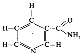
Никотинамид
