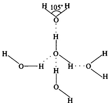
Рис. 1. Ассоциат молекул воды. Точками обозначены водородные связи
