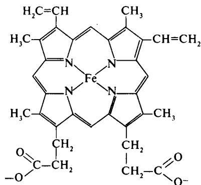
Рис. 25. Структура гема цитохрома b
