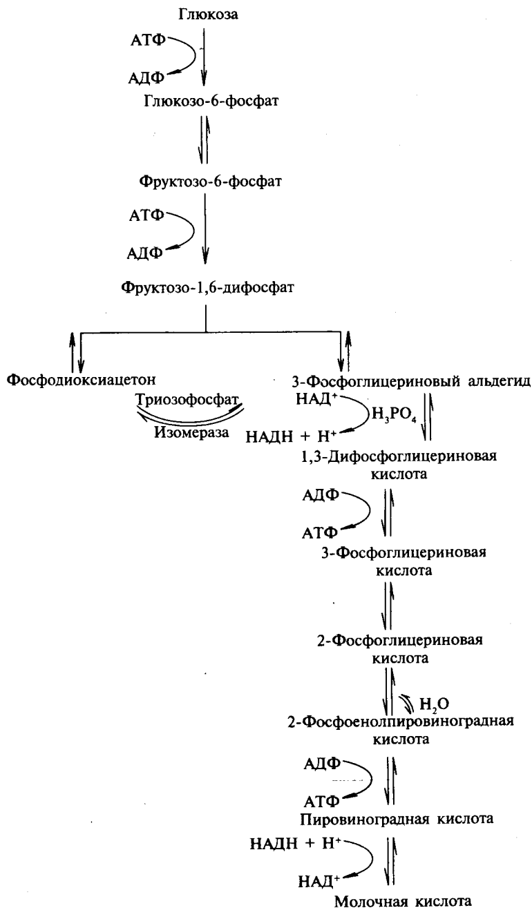
Схема 1. Гликолиз
