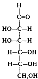
D -манноза
