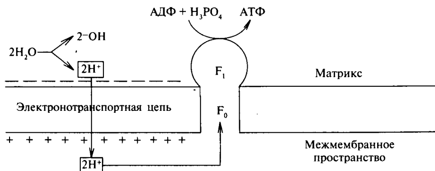
Рис. 26. Синтез АТФ, сопряженный с электронотранспортной цепью
