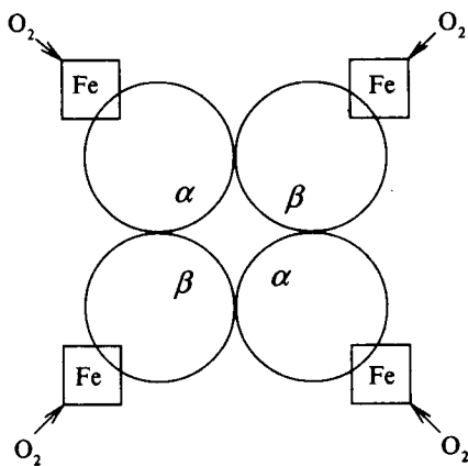
Рис. 7. Схематичное изображение четвертичной структуры гемоглобина: Fe — гем гемоглобина
