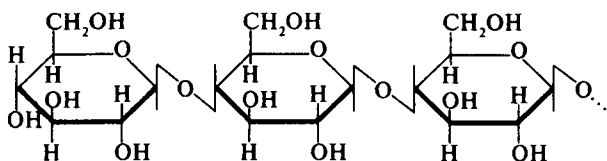
Целлюлоза
