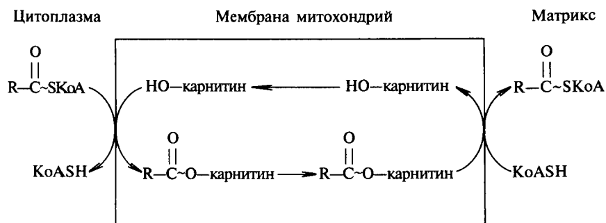
Рис. 16. Схема транспорта жирных кислот через митохондриальную мембрану
