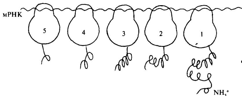
Рис. 20. Полирибосома
