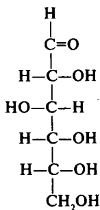
D -глюкоза
