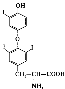
Триодтиронин
