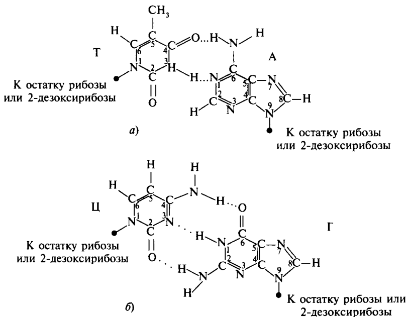
Рис. 18. Принцип комплементарности азотистых оснований нуклеиновых кислот: а) — образование водородных связей (---) между тиминем (Т) и аденином (А); б) — образование водородных связей (---) между цитозином (Ц) и гуанином (Г)
