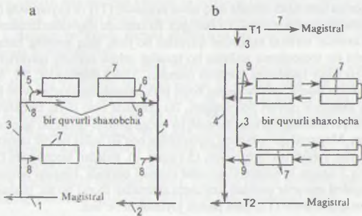
5.2-rasin Pastdan (a) va yuqoridan (b) uzatuvchi suvli gorizontal isitish tizimlari: 1, 2 – uzatuvchi va qaytaruvchi magistr; 3 va 4 – uzatuvchi va qaytaruvchi tirkak; 5 va 6 – uzatuvchi va qaytaruvchi ulama; 7 – isitish asboblari; 8 – bir quvurli shahobcha; 9 – bifilyar tarmoq
