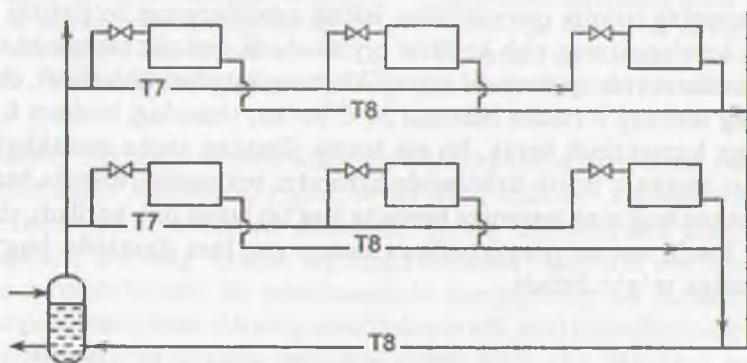
15.4-rasm. Gorizontaal ikki quvurli past haroratli bug'li isitish tizimining umumiy ko'rinishi
