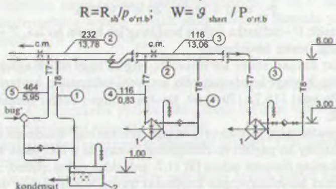
9.12-rasm. Yuqori bosim ta'sirida ishlaydigan isitish tizimining (kondensat idishi yopiq) hisobiy sxemasi
