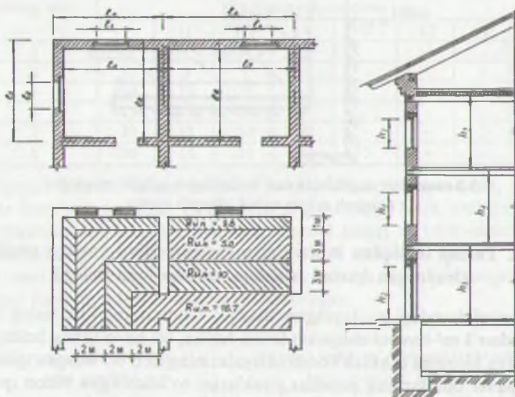
3.1-rasm. To'siqlarning hisobiy o'lchamini aniqlash
