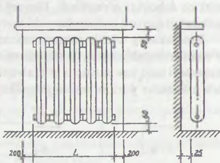
4.17-rasm. Radiatorlarning mehrobg'a o'rnatilishi
