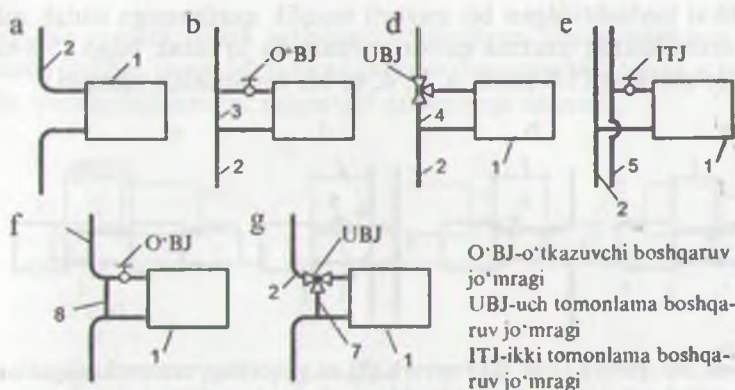
5.7-rasm. Bir (a-d) va ikki (e) quvurli vertikal isitish tizimida quvurlarning isitish asboblariга bir tomonlama ulanishi: 1 - isitish asboblari; 2 - bir quvurli tirkaklar, 3 - o'qi siljutilmagan birlashtiruvchi tirkaklar; 4 - o'qli aylanma uchastkasi; 5 va 6 - ikki quvurli tirkaklarda isitish tizimlariga issiqlik uzatuvchi va qaytaruvchi quvurlar; 7 - o'qdan siljutilgan tutashtiruvchi quvur; 8 - siljutilmagan tutashtiruvchi quvur
