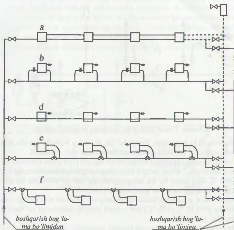
1.6-rasm. Sun'iy harakatlanuvchi suv bosimi ta'sirida ishlaydigan bir quvurli gorizontall isitish tizimlarining prinsipial sxemasi: a) issiq suvni to'g'ridan-to'g'ri to'liq miqdorda isitish asbobi orqali o'tish uslubi; b) birlashtiruvchi uzatma orqali isitish asboblarning ulanish uslubi; d) to'g'ridan-to'g'ri isitish asbobiga ulanish uslubi; e) boshqariluvchi, to'g'ridan-to'g'ri plintusgardishli ulash uslubi; f) to'g'ridan-to'g'ri, boshqariluvchi, deraza tagiga ulanuvchi gorizontall o'rnatilgan isitish asboblari
