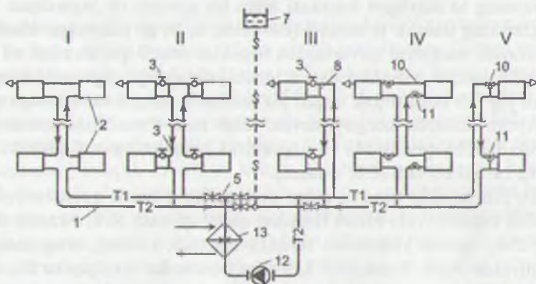
6.8, b-rasm. Quyidan taqsimlanuvchi bir quvurli va «Π» harfi shaklidagi tirkaklari turli konstruksiyali tirkakli isitish tizimlari: I – to‘g‘ri oqimli tirkak; II va III – siljirilgan va oxiri «Π» shaklida ulangan tirkak; IV-V – to‘g‘ri oqimli boshqariluvchi tirkak
