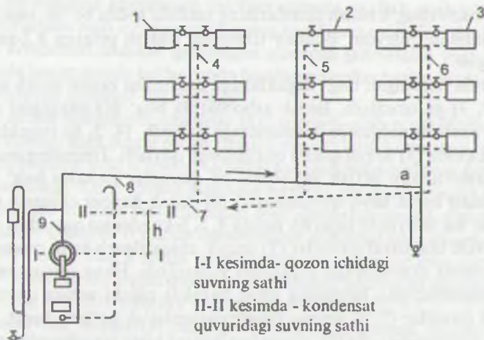
9.2-rasm. Quyidan taqsimlanuvchi va quruq kondensat quvurli bug'li bilan isitish tizimining prinsipl sxemasi
