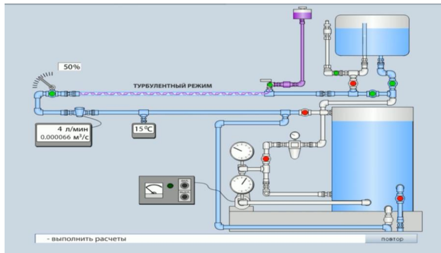
Рис.6.2 Схема лабораторной установки.
