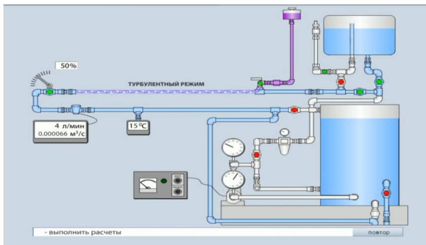
Рис.7.3 Схема лабораторной установки.
