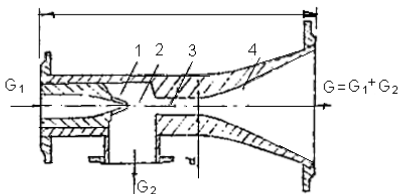
2.2- rasm. Elevatorning tuzilishi.
