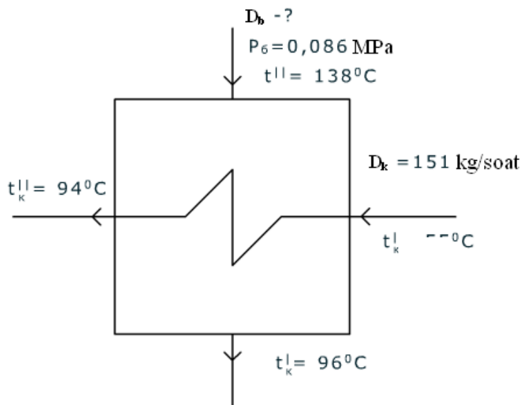
3.2 – rasm. Turbina kondensatoridan kelayotgan asosiy kondensat yo'liga o'rnatilgan PBI sxemasi.
