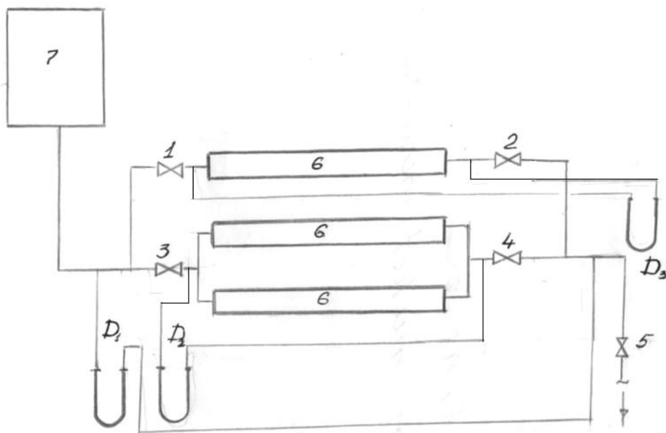
7.2-rasm. Tajriba qurilmasining chizmasi.
