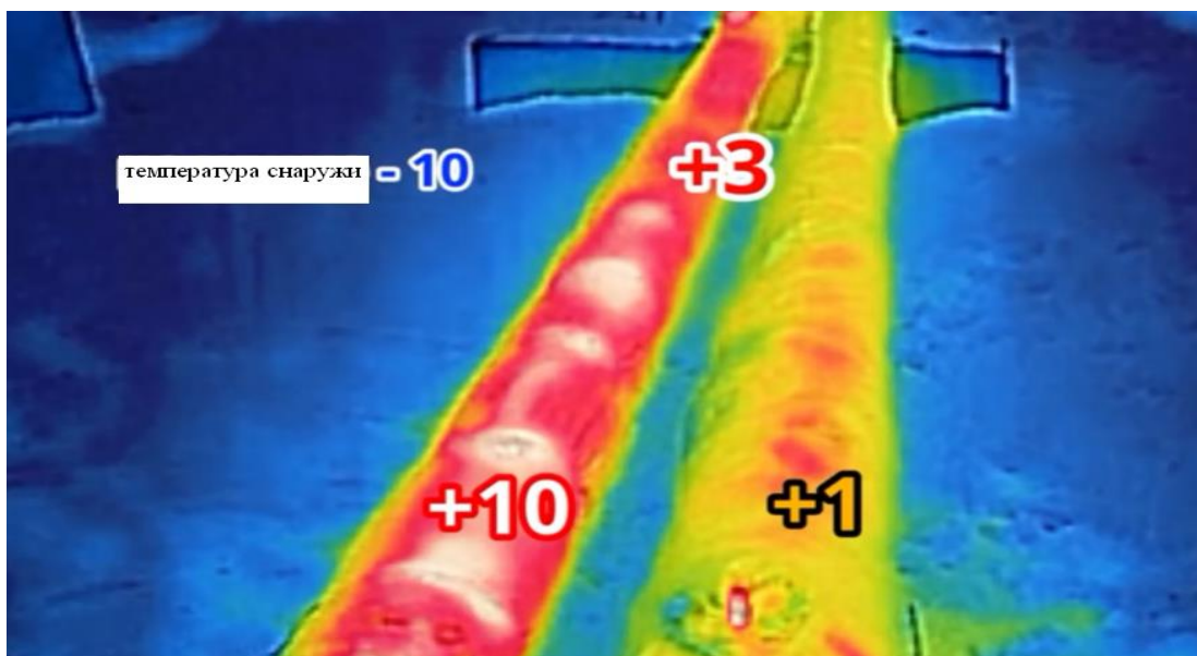
Рис.4.1. Система изолированных трубопроводов
