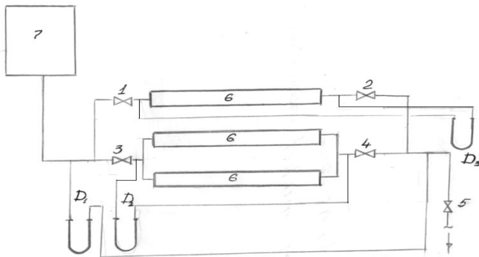
5.1-rasm tajriba bajarish qurilmasi.
