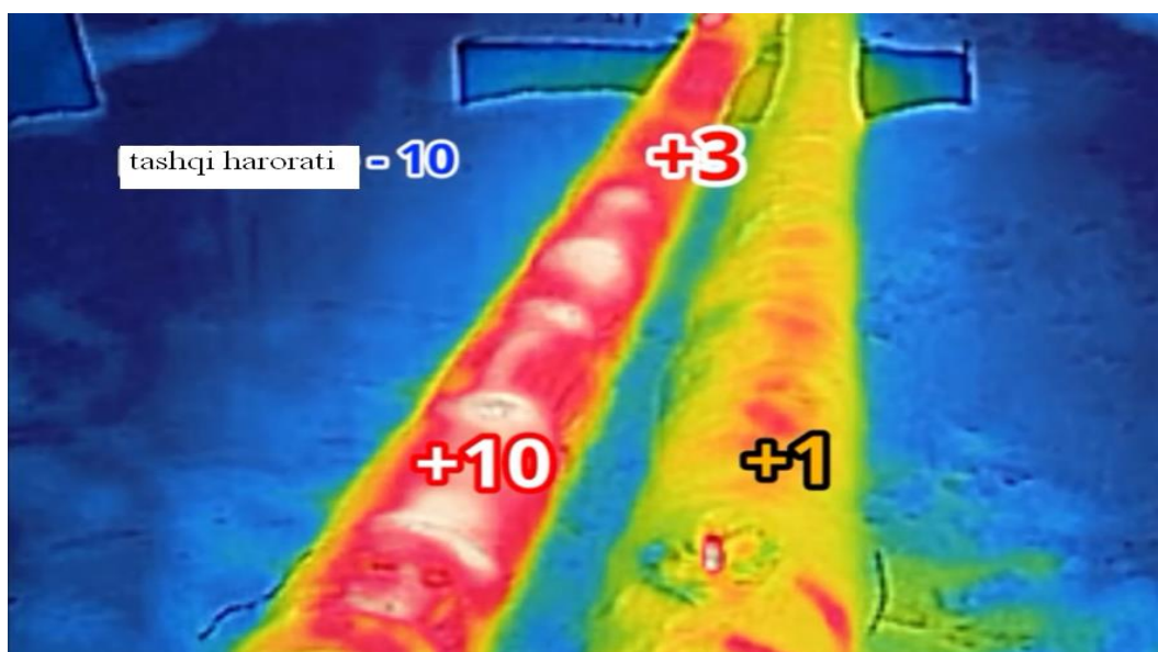
4.1-rasm. Issiqlik ta'minoti tizimi ko'rinishi.
