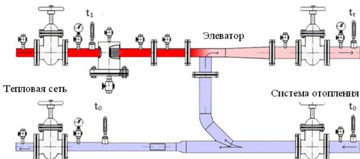
Рис.2.3 Схема элеваторного узла.
