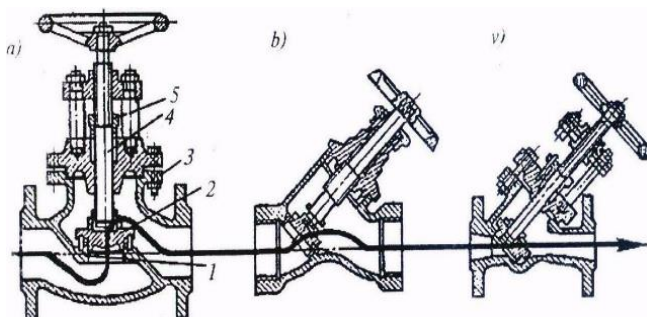
Рис 7.1. Вентили:
