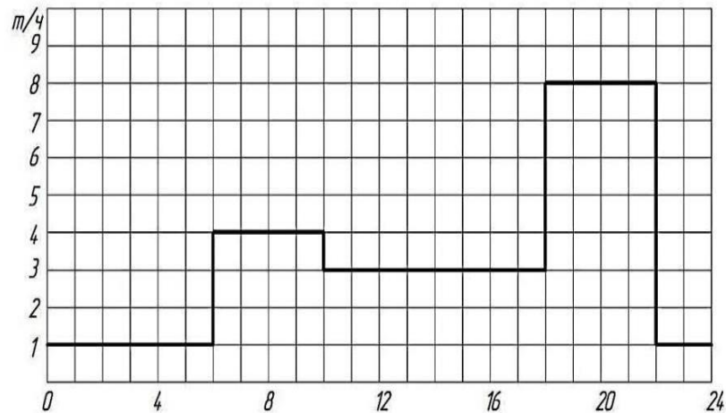
Рис. 1.3. График суточного потребления горячей воды (пример расчета)
