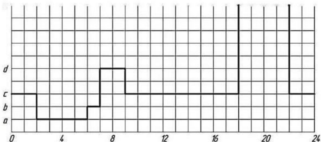
Рис.1.2. График суточного потребления горячей воды (задание)
