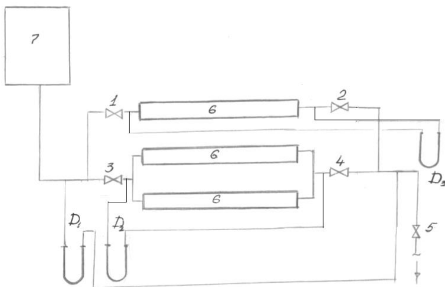
Рис.5.2 Схема опытной установки
