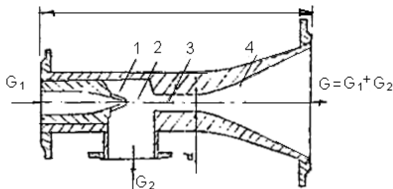
Рис.2.2. Конструкция элеватора.
