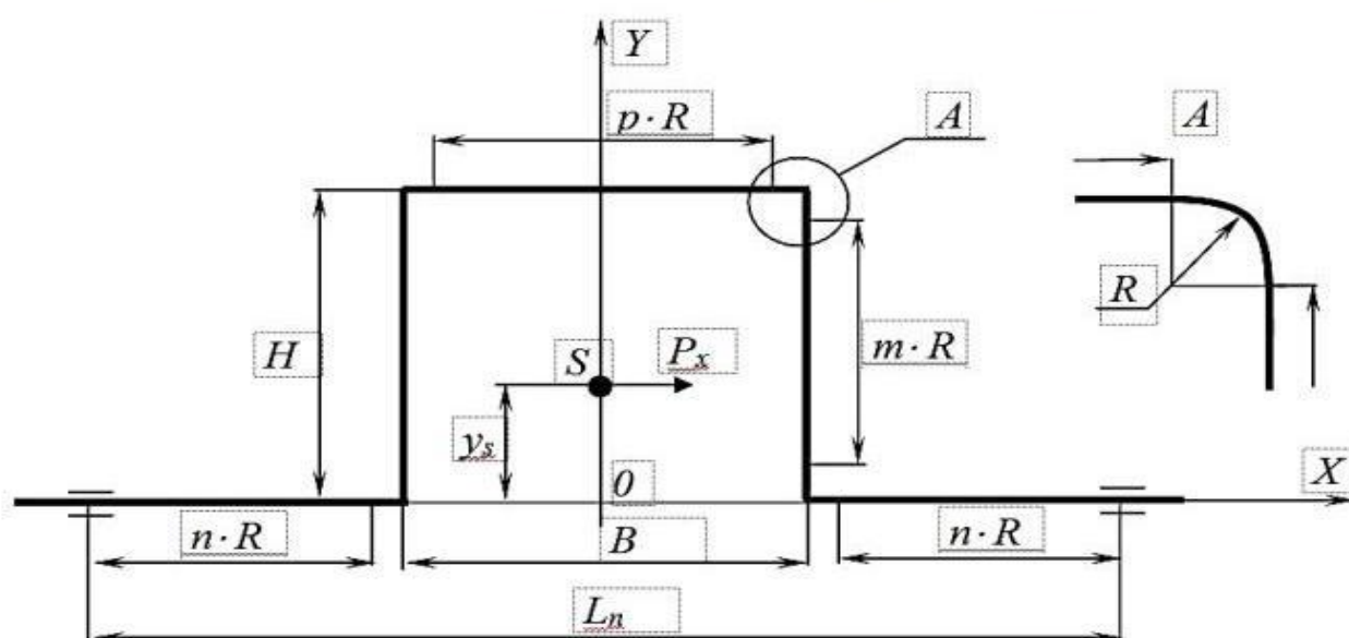
Рис. 8.2.Схема компенсатора
