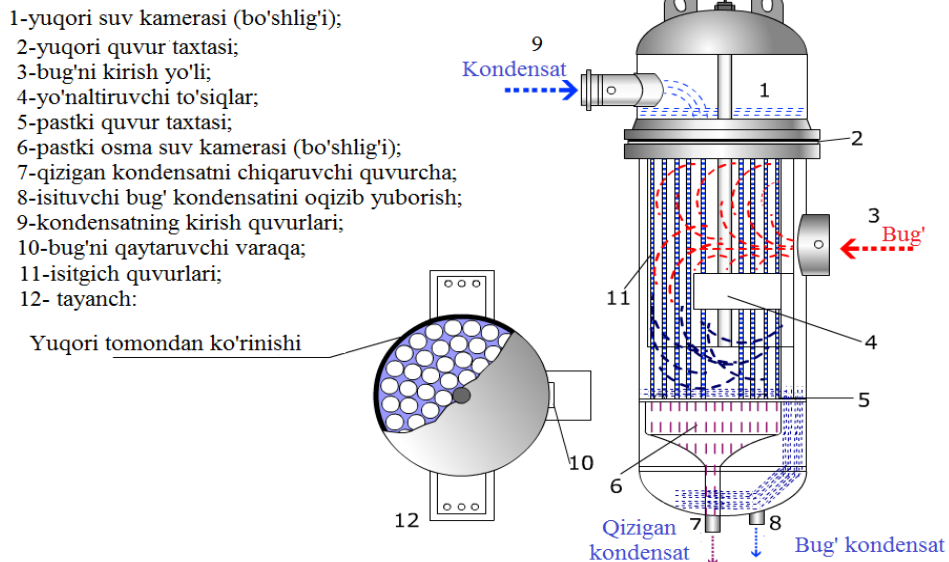
3.1– rasm. Past bosimli isitgichning sxemasi.
