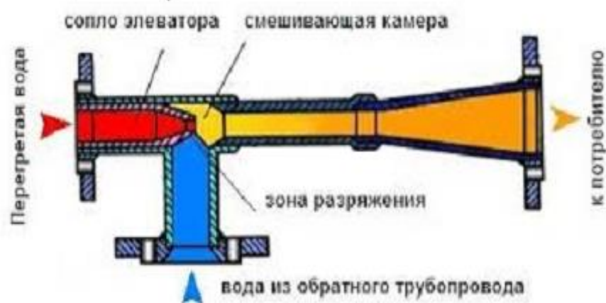
Рис.2.1. Схема водоструйного элеватора.
