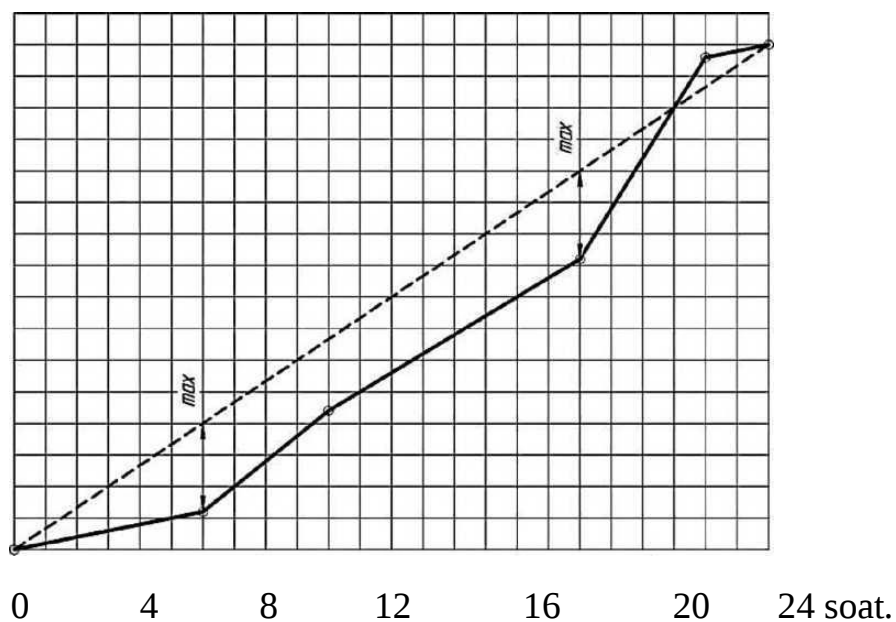
1.5- rasm. O'rtacha (punktir chizig'i) va haqiqiy (uzluksiz chizig'i) sarflar grafiklarini solishtirish chizmasi
