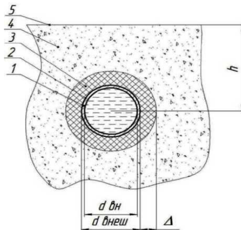
Рис.1.1. Схема прокладки трубопровода.
