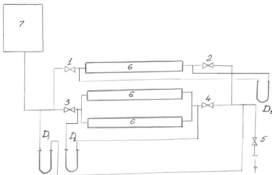
Рис.7.2 Схема лабораторной установки.
