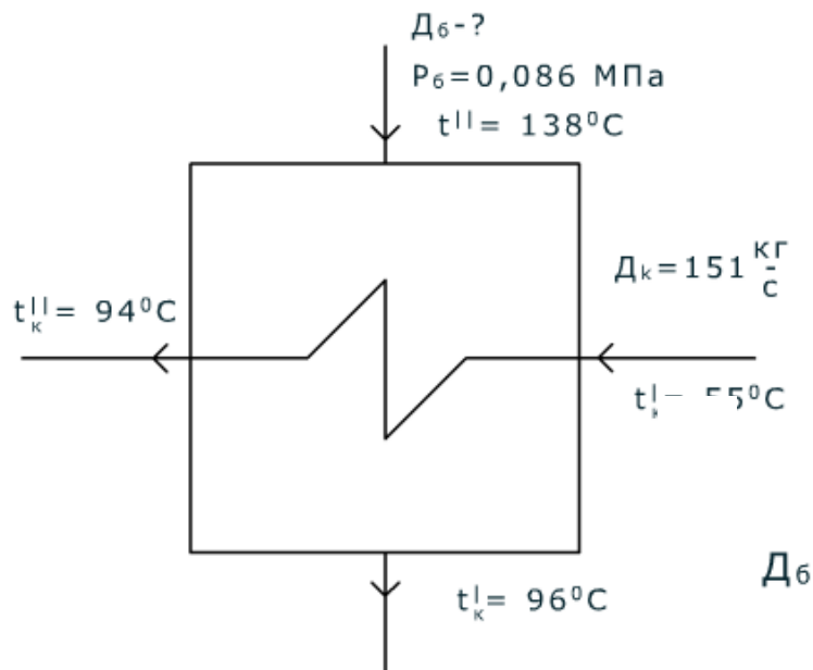
Рис.3.2 Расчетная схема подогревателя низкого давления.
