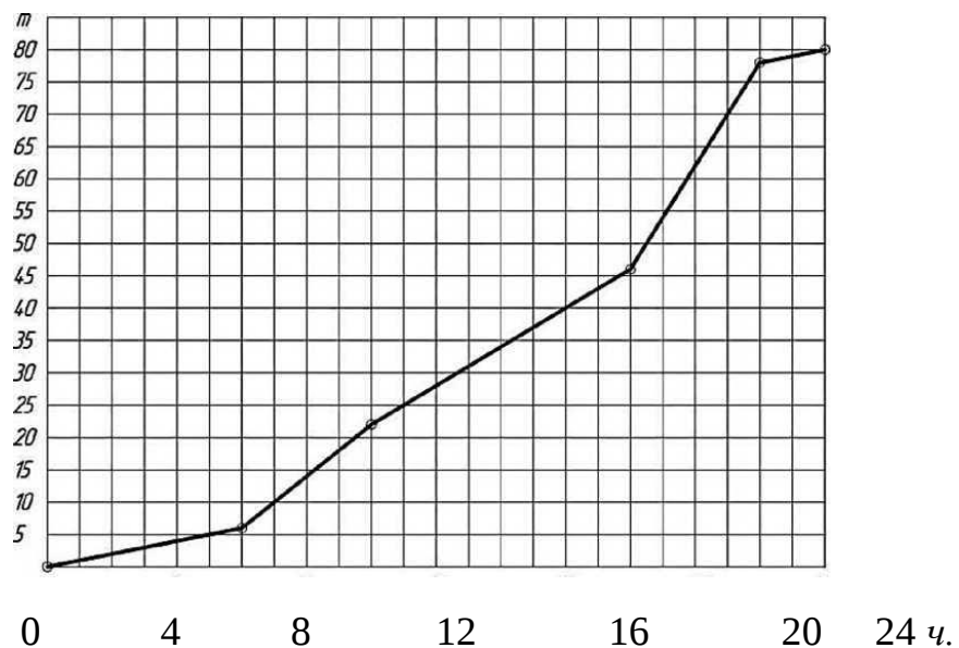
Рис. 1.4. Динамика потребления горячей воды в течение суток (пример расчета)
