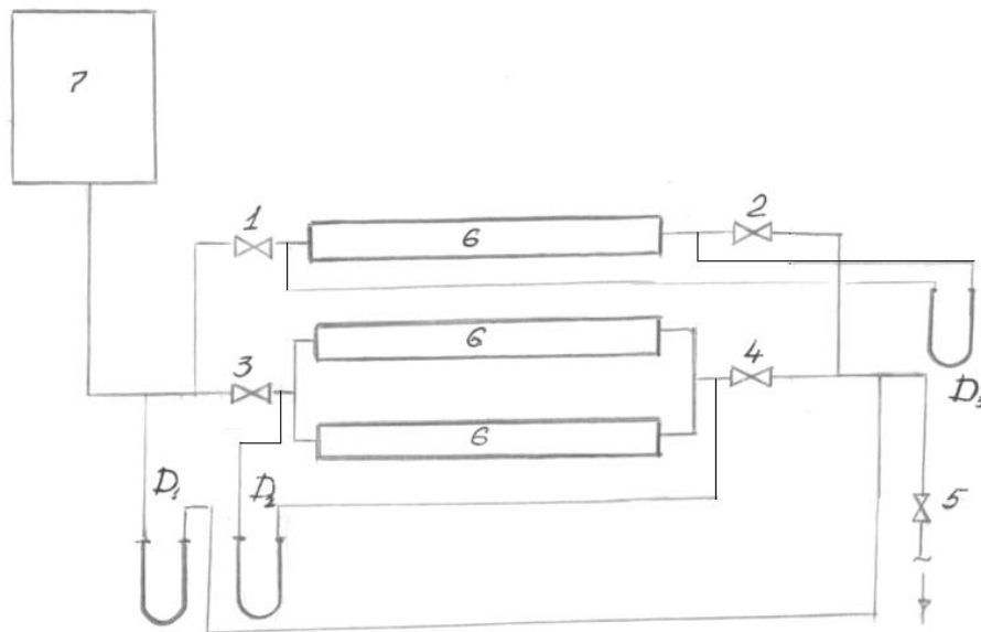
Рис.6.1 Схема лабораторной установки.
