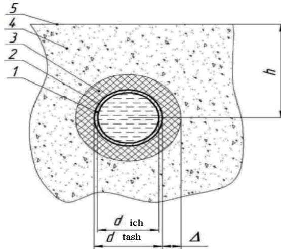
1.1-rasm. Issiqlik quvurni joylashish sxemasi.
