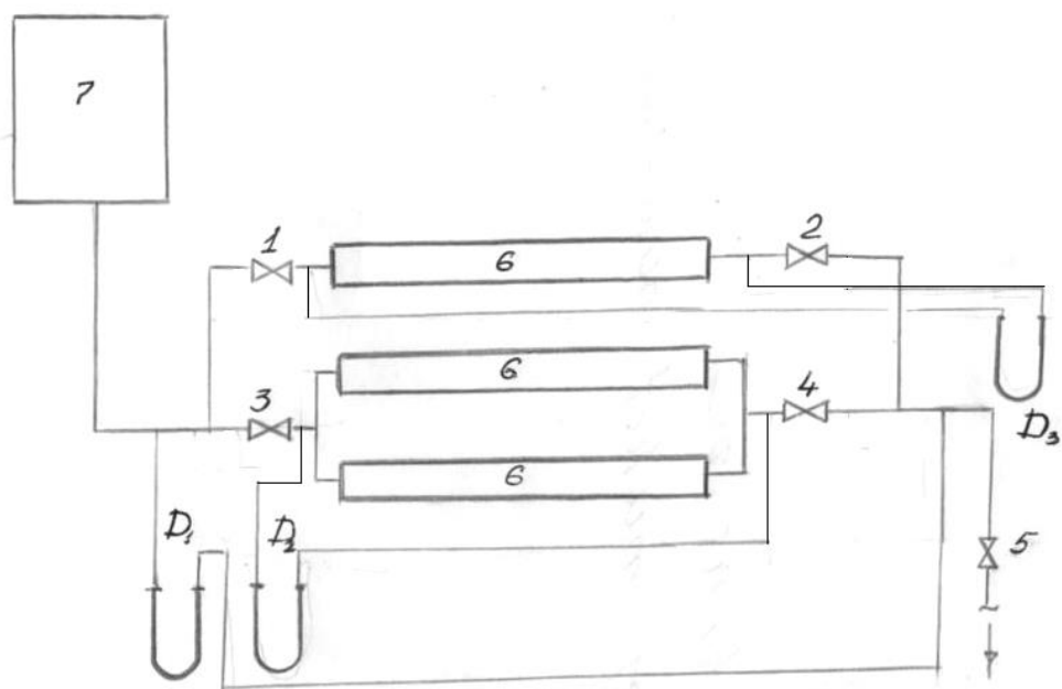
6.1.-rasm. Suvli issiqlik tarmog'ining sxemasi.
