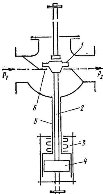
Рис. 9.6. Схема редукционного клапана
