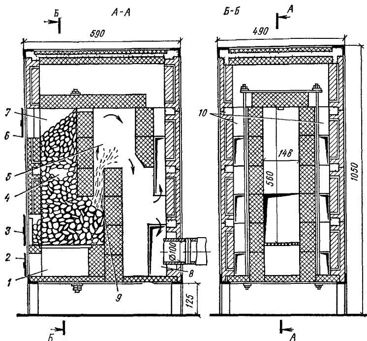
Рис. 12.8. Каркасная отопительная печь длительного горения АКХ-9 тепловой мощностью 2790 Вт
