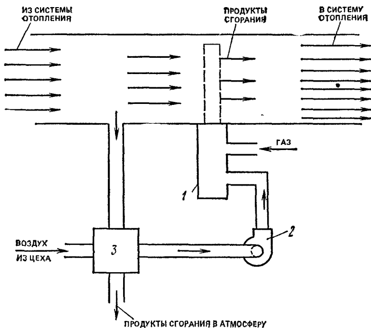
Рис. 13.10. Принципиальная схема погоков газа, воздуха и газовой смеси в теплогенераторе ТГЛ-0,5
