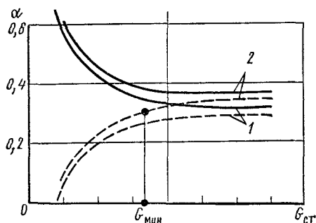
Рис. 8.5. Изменение коэффициента затекания воды в отопительные приборы однетрубных стояков с замыкающими осевыми (1) и смещенными (2) участками при движении воды в стояках в количестве G_{ст} сверху вниз (сплошные линии) и снизу вверх (пунктирные линии)
