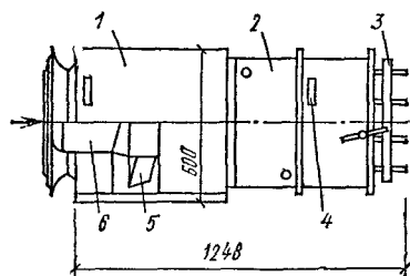
Рис. 10.3. Подвесной воздушно-рециркуляционный отопительный агрегат АО2-4 (боковой вид)
