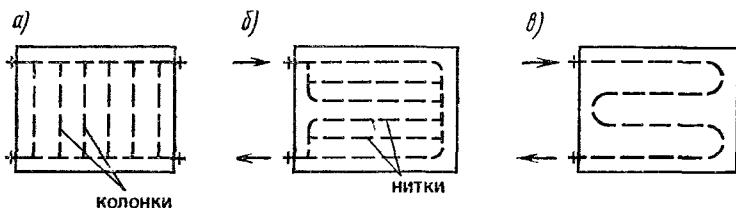
Рис. 4.4. Схемы каналов для теплоносителя в панельных радиаторах колончатой (а) формы (радиатор РСВ), змеевиковой двухходовой (б) и четырехходовой (в) форм (радиаторы РСГ-2 и РСГ-1)
