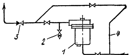
Рис. 9.8. Схема установки поплавкового конденсатоотводчика на магистрали
