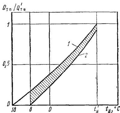
рис. 17.2. Изменение теплотребности здания в течение отопительного сезона без учета (1) и с учетом (2) технологических и внутренних теплоступлений и солнечной радиации
