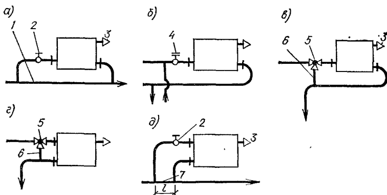
Рис. 5.10. Присоединение труб к отопительным приборам систем водяного отопления
