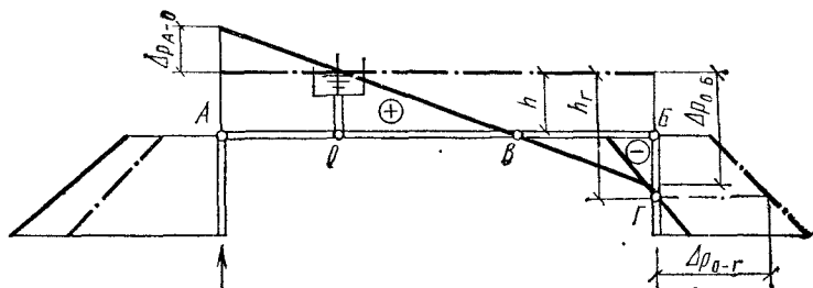
Рис. 7.7. Изменение гидростатического давления в верхней подающей магистрали системы отопления
