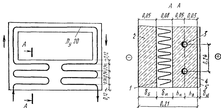
Рис. 11.8. Бифурканный стояк системы водяного отопления и греющие элементы змеевиковой формы, совмещенные с трехслойной наружной стеной
