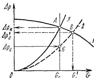
Рис. 6.14. Схема выбора циркуляционного насоса при \Delta p_n > \Delta p_c
