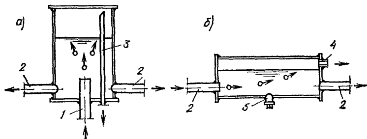
Рис. 5.17. Проточные воздухоборники
