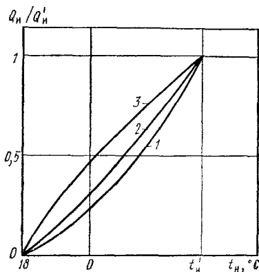
рис. 17.1. Изменение теплотребности на нагревание поступающего наружного воздуха в однотипные помещения многоэтажного жилого здания, расположенные на нижних этажах 5—12-этажного здания (1), на верхних этажах 5—12-этажного (2) и 16—22-этажного (3) здания, в течение отопительного сезона
