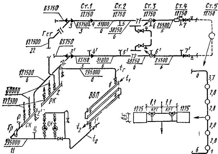
Рис. 8.11. Схема вертикальной однотрубной системы водяного отопления с верхней разводкой и тупиковым движением воды в магистралях (к примеру 8.12)
