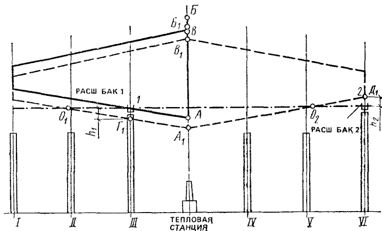
Рис. 7.17. Изменение гидростатического давления в теплопроводах районной системы водяного отопления (сплошные линии) при ее расширении (пунктирные линии) с установкой второго расширительного бака
