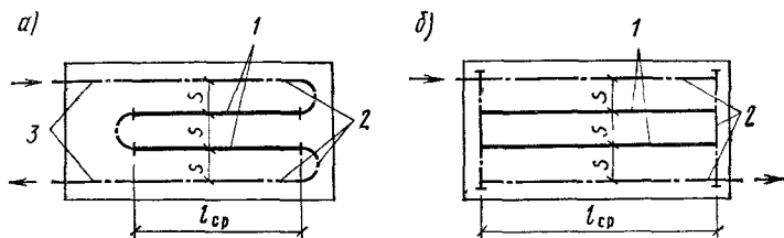
Рис. 11.2. Схемы нагревательных элементов отопительной панели змеевиковой (а) и регистровой (б) формы
