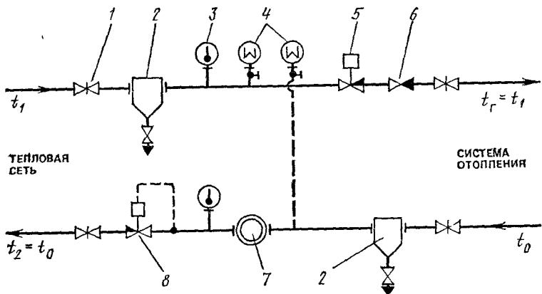
Рис. 6.11. Принципиальная схема местного теплового пункта при зависимом прямоточном присоединении системы водяного отопления к наружным теплопроводам
