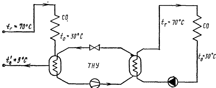
Рис. 19.5. Схема децентрализованного отбора теплоты из обратной магистрали системы центрального отопления (теплоснабжения) с помощью теплового насоса
