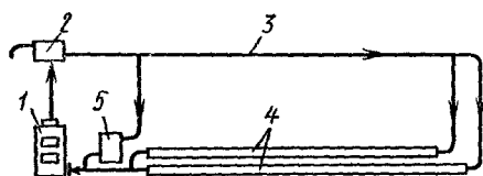
Рис. 6.25. Схема системы водяного отопления железнодорожного пассажирского вагона
