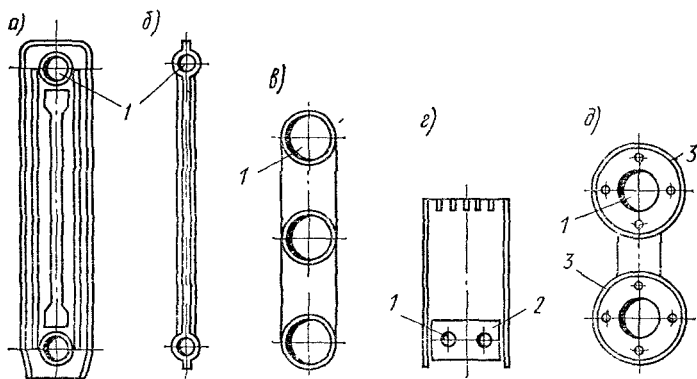
Рис. 4.2. Схемы отопительных приборов различных видов (поперечные разрезы) а — радиатор чугунный секционный; б — радиатор стальной панельный (РСб); в — гладкотрубный прибор из трех горизонтальных стальных труб; г — конвектор с кожухом; д — прибор из двух ребристых труб; 1 — канал для теплоносителя; 2 — стальная пластина; 3 — чугунный фланец
