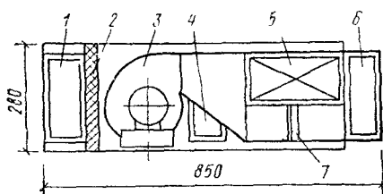
Рис. 10.8. Квартирный отопительно-вентиляционный агрегат
