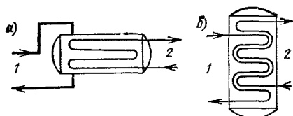
Рис. 20.2. Независимое включение теплоаккумулятора в контур системы отопления с зависимым подключением греющего контура (а) и с независимым (б) 1 — греющий контур; 2 — контур системы отопления
