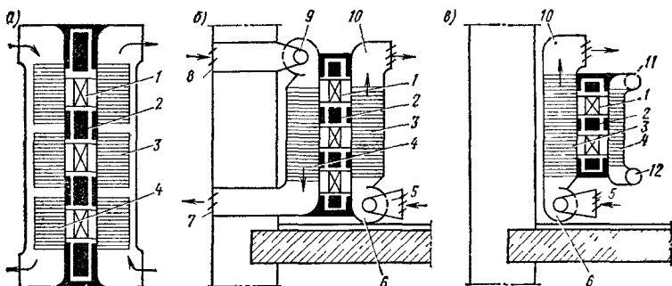
Рис. 14.14. Тепловой насос на полупроводниках (а), отопление помещения агрегатом типа «воздух — воздух» (б) и типа «воздух — вода» (в)
