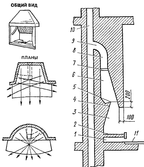
Рис. 12.9. Камин с односторонним излучением
