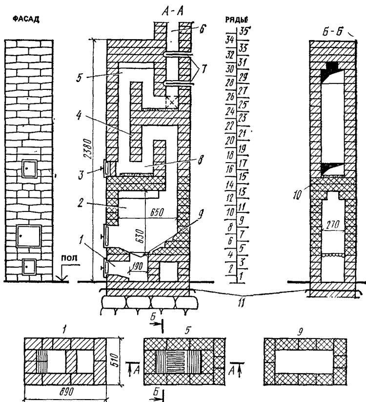
Рис. 12.4. Толстостенная отопительная печь умеренного прогрева марки ПТО-2500 с двумя последовательными дымооборотами
