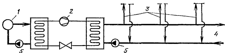
Рис. 20.12. Схема геотермальной теплосети с централизованным повышением температуры теплоносителя с помощью теплового насоса и закачкой отработанной воды в пласт
