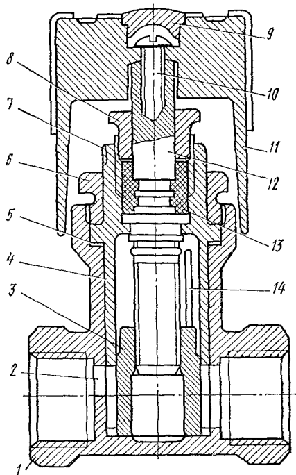
Рис. 5.11. Кран двойной регулировки шиберный типа КРДШ
