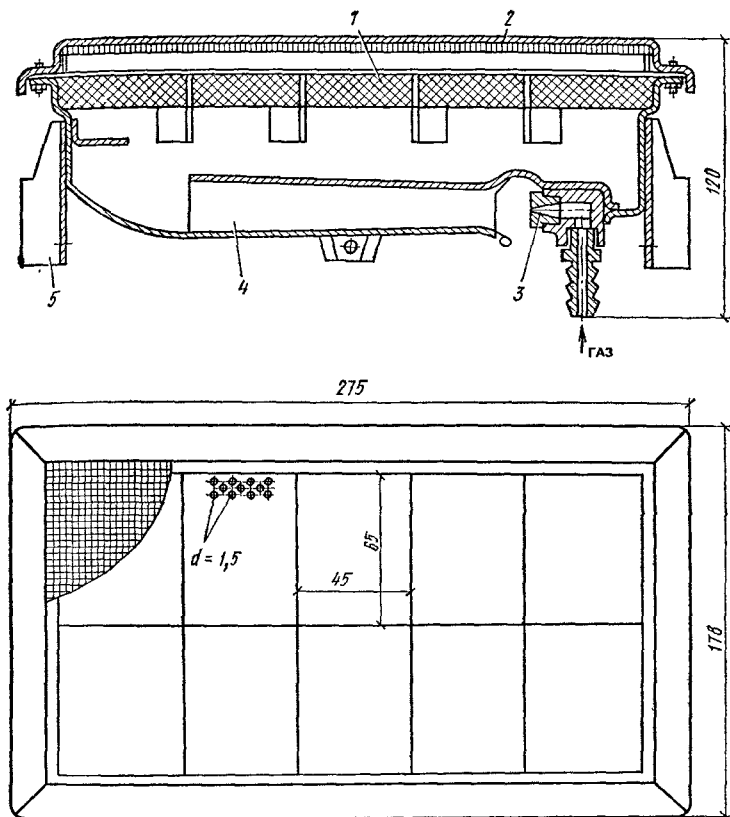
Рис. 13.11. Газовая горелка инфракрасного излучения
