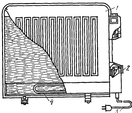
Рис. 14.6. Электрорадиатор панельного типа
