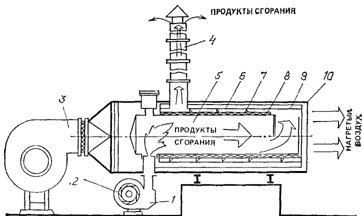
Рис. 13.7. Газовоздушный теплообменник ТГ-450
