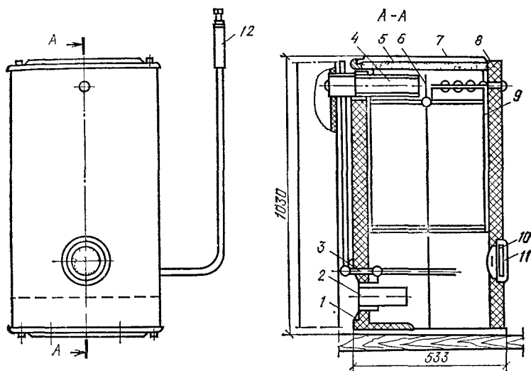
Рис 13.2. Отопительная печь заводского изготовления АКХ-СМ-1
