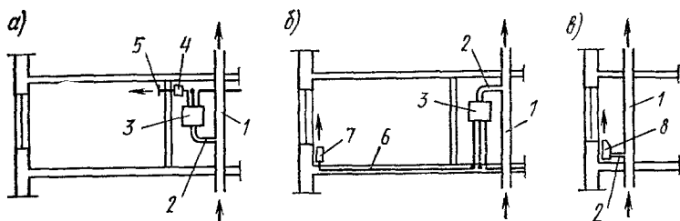
Рис. 18.1. Схемы комбинированного отопления многоэтажных зданий с централизованной подачей подогретого воздуха и местным дополнительным нагреванием а — в групповом нагревателе для выпуска воздуха под потолком помещений через шумоглушитель и регулятор подачи воздуха, б — то же, для выпуска воздуха под окнами помещений через подпольный воздуховод и регулятор подачи воздуха; в — в индивидуальном нагревателе-доводчике под окном каждого помещения
