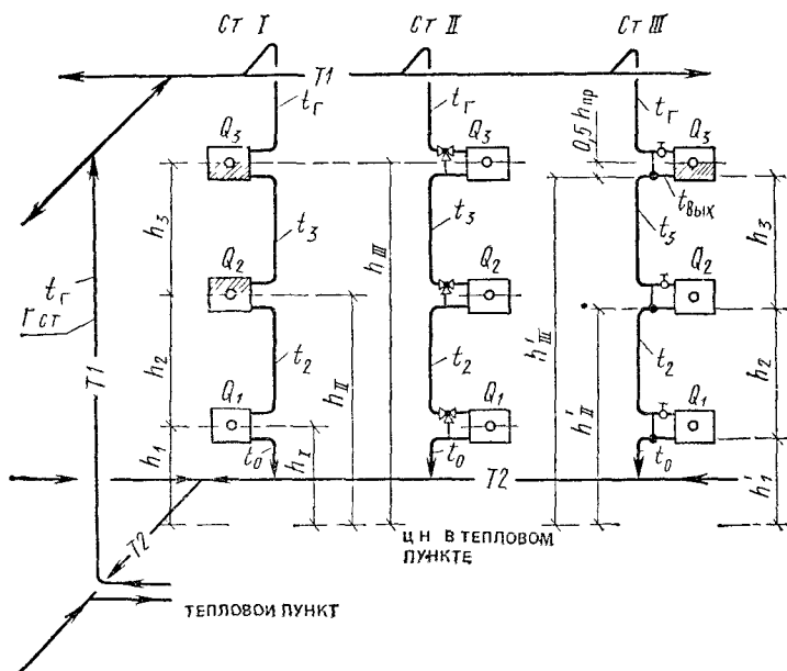
Рис. 7.20. Расчетная схема вертикальной однотрубной системы водяного отопления с верхней разводкой
