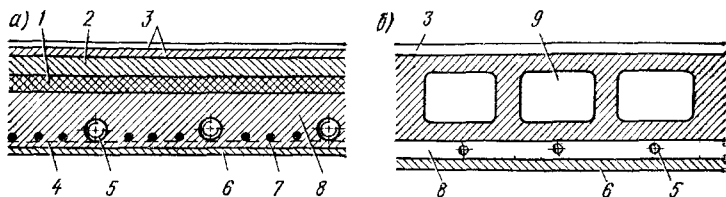
Рис. 11.5. Совмещенные потолочные бетонные отопительные панели с расположением греющих труб в несущем бетонном слое (а) и под несущими пустотелыми блоками (б)
