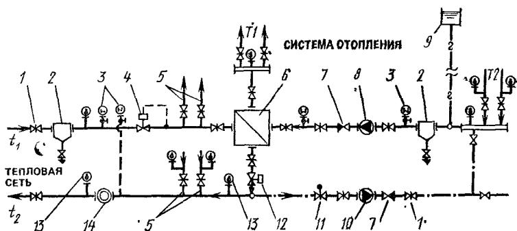
Рис. 6.9. Принципиальная схема местного теплового пункта при независимом присоединении системы водяного отопления к наружным теплотрассам
