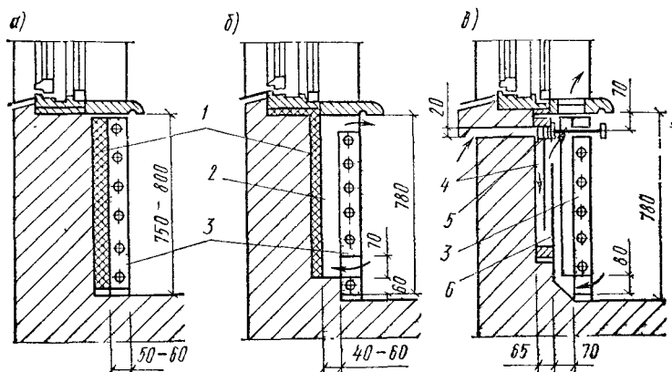
Рис. 11.10. Подоконные приставные бетонные отопительные панели с односторонней теплоотдачей (а), двусторонней теплоотдачей (б) и с двусторонней теплоотдачей и каналом для подачи подогретого наружного воздуха (в)
