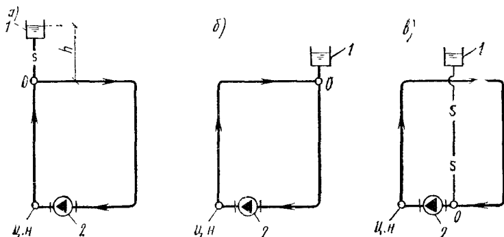
Рис. 7.8. Способы присоединения труб открытого расширительного бака к системе водяного отопления
