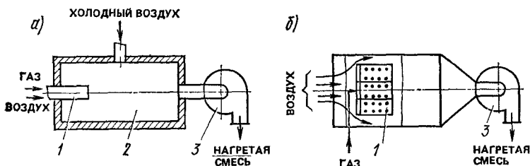
Рис. 13.8. Принципиальные схемы смесительных газозвудушных нагревателей ВГС с разбавлением продуктов сгорания в специальной камере (а) и сжиганием газа непосредственно в потоке воздуха (б)
