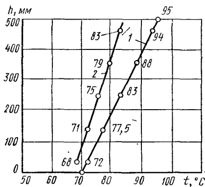
Рис. 4.14. Изменение температуры воды (1) и наружной поверхности (2) по высоте чугунного секционного радиатора при движении теплоносителя сверху вниз в двухтрубной системе отопления
