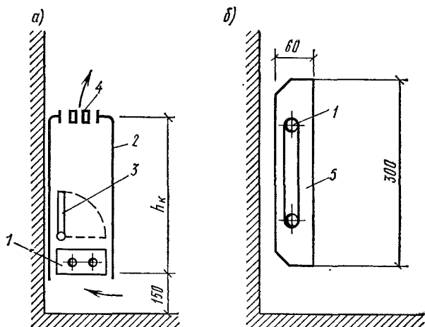
Рис. 4.6. Схемы конвекторов
