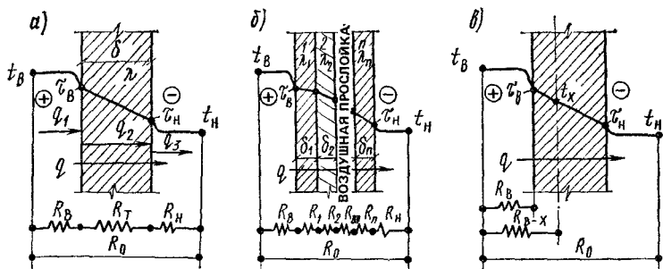
Рис. 2.4. Стационарная теплопередача через однослойное ограждение (а), многослойное с воздушной прослойкой (б) и определение температуры в произвольном сечении ограждения (в)
