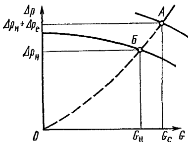
Рис. 7.26. Характеристики — насоса (рабочая точка Б) и суммарная (рабочая точка А с учетом естественного циркуляционного давления \Delta p_e ) применительно к вертикальной однотрубной системе отопления (расход воды изменяется от G_n до G_c )
