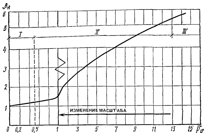
Рис. 3.4. Зависимость коэффициента \beta_n от относительного давления ветра \bar{p}_v для помещения с двусторонним остеклением
