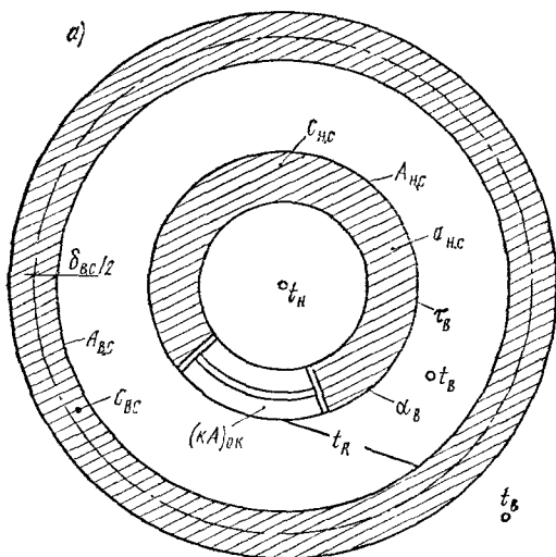
Рис. 2.10. Схема помещения (а) и аналоговая сетка теплообмена (б) общего решения охлаждения помещения
