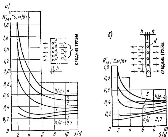
Рис. 4.15. Изменение термического сопротивления массива бетона R'_M , ^{\circ}\text{C}\cdot\text{м}/\text{Вт} , отнесенного к 1 м средних труб бетонного панельного радиатора [при теплопроводности бетона \lambda=1,0 Вт/(м \cdot^{\circ}\text{C} )], при односторонней теплоотдаче (а) и двусторонней (б)
