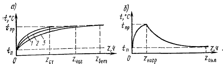
Рис. 4.18. Характер процессов изменения температуры поверхности отопительных приборов во времени
