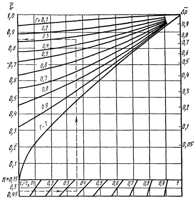
Рис. 17.5 Номограмма для определения показателя гидравлического разрегулирования системы водяного отопления
