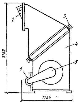
Рис. 10.4. Напольный воздушно-рециркуляционный агрегат STD-800M
