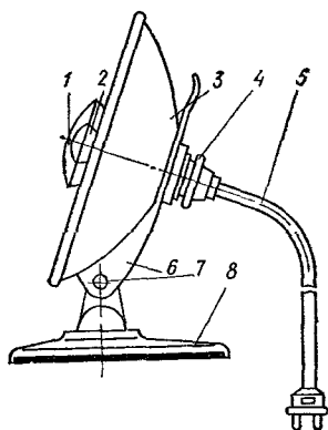
Рис. 14.4. Электрокамины со сферическим отражателем
