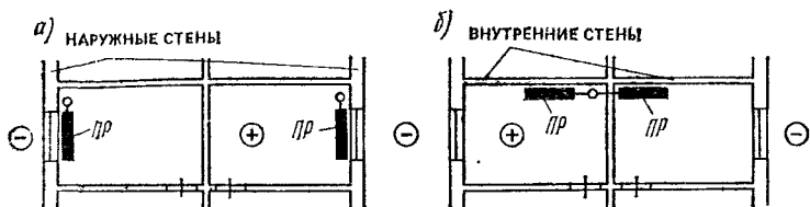
Рис. 4.8. Размещение отопительных приборов (пр) в помещениях (планы) под окнами (а), у внутренних стен (б)
