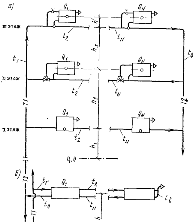
Рис. 7.24. Расчетные схемы горизонтальной однотрубной системы водяного отопления
