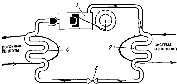
Рис. 14.13. Схема парокомпресссионного теплового насоса
