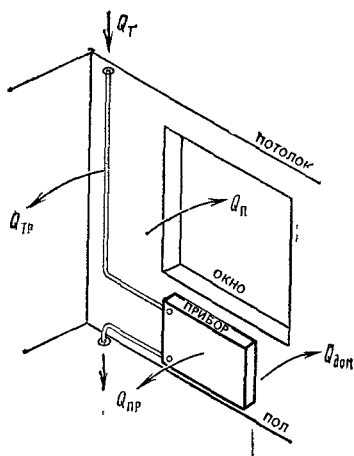
Рис. 4.1. Схема теплоотдачи отопительного прибора Q_{пр} и труб Q_{тр} для возмещения теплопотерь помещения Q_{п} и Q_{доп} при теплоподаче Q_T со стороны теплоносителя
