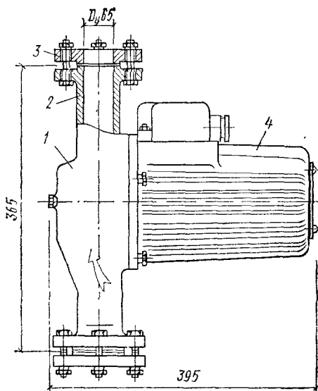
Рис. 6.12. Центробежный циркуляционный насос типа ЦВЦ 1 — корпус; 2 — нагнетательный патрубок; 3 — контрофланец для присоединения трубы; 4 — электродвигатель
