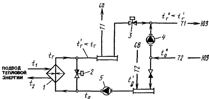
Рис. 17.4. Принципиальная схема автоматического регулирования температуры воды, направляемой в северо-восточную и юго-западную части системы отопления 1 — теплообменник; 2 — регулятор температуры по «возмущению»; 3 — регулятор температуры по «отклонению»; 4 — смесительный насос; 5 — циркуляционный насос
