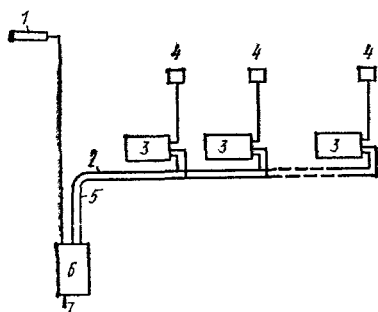
Рис. 14.9. Схема электротеплоаккумуляционной системы отопления одноквартирного дома
