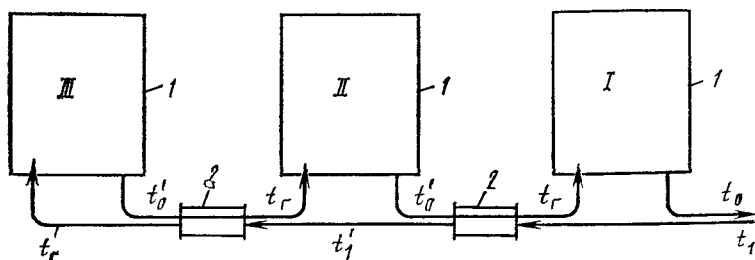
Рис. 8.29. Принципиальная схема системы водяного отопления СРТ, состоящей из трех подсистем I и двух регенераторов температуры 2
