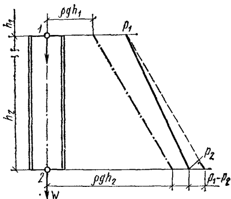
Рис. 7.2. Изменение гидростатического давления в вертикальной трубе при движении заполняющей ее воды сверху вниз (давление отложено справа от отрезка трубы)
