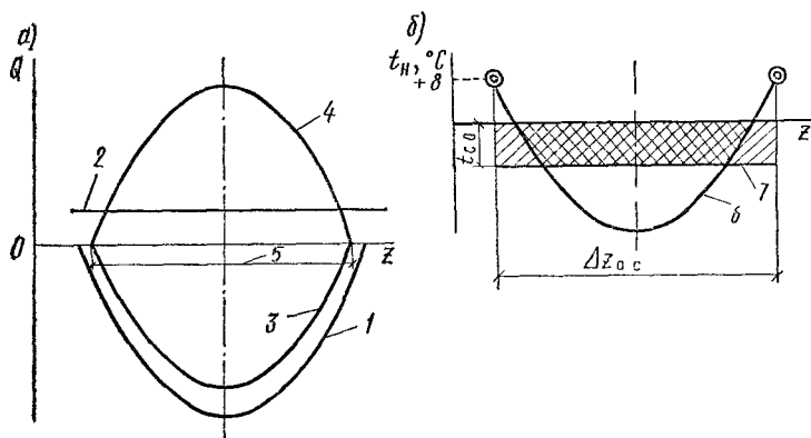
Рис. 2.2. Схема изменения тепловой нагрузки (а) и определения параметров отопительного сезона (б)
