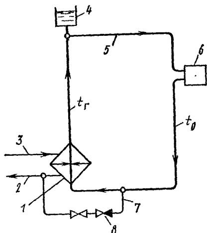
Рис. 6.24. Принципиальная схема гравитационной системы водяного отопления
