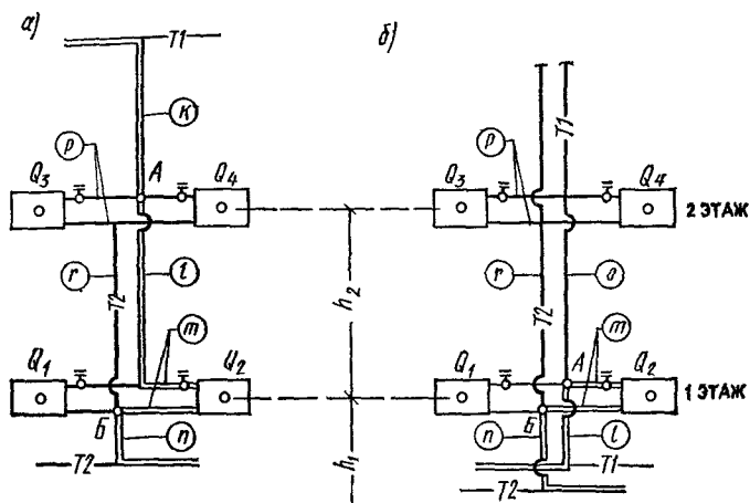
Рис. 8.10. Схемы двухтрубных стояков с расчетными участками в системах водяного отопления с верхней (а) и нижней (б) разводками
