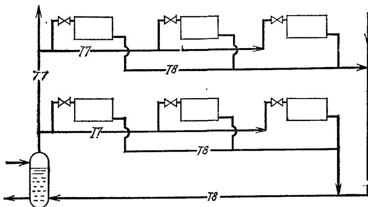
Рис. 20.4. Горизонтальная двухтрубная низкотемпературная система парового отопления
