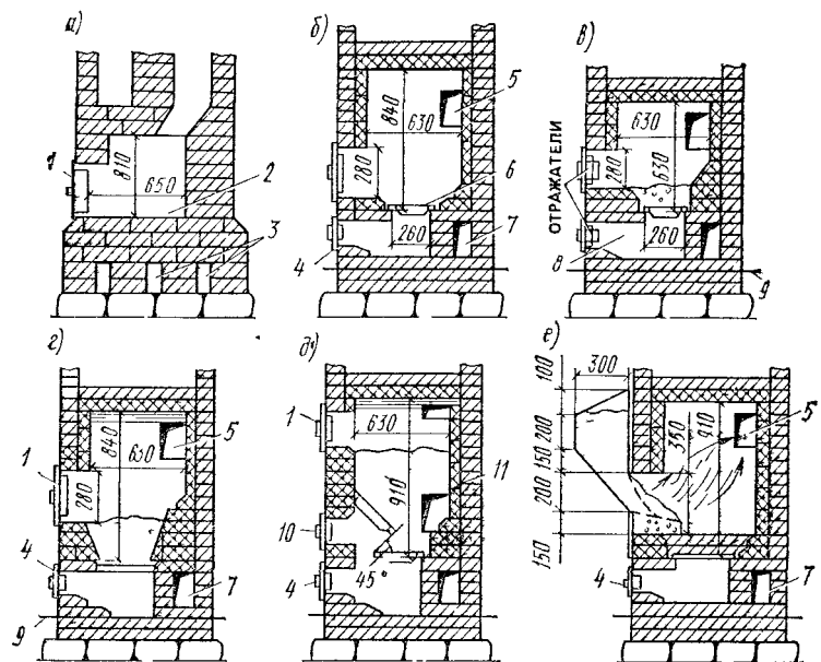
Рис. 12.3. Конструкции печных топливников с глухим подом (а), с колосниковой решеткой для сжигания дров (б), каменного угля (в), антрацита (г), влажного торфа (д), с бункром для сжигания местных горючих веществ (е)
