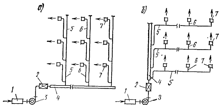
Рис. 18.2. Схемы высокоскоростных систем комбинированного воздушного отопления с доводчиками многоэтажных зданий
