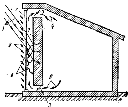
Рис. 20.5. Пассивная низкотемпературная система солнечного отопления «стена — коллектор»
