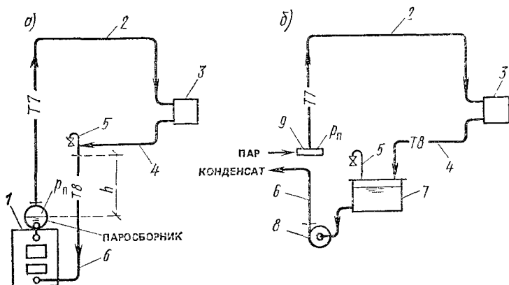
Рис. 1.6. Принципиальные схемы замкнутой (а) и разомкнутой (б) систем парового отопления
