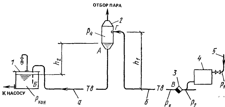
Рис. 9.11. Схема прокладки напорного (а) и двухфазного (б) конденсатопроводов 1 — конденсатный бак; 2 — бак-сепаратор; 3 — конденсатоотводчик; 4 — отопительные приборы системы парового отопления высокого давления; 5 — паропровод
