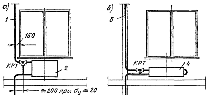
Рис. 5.3. Этажестояки вертикальной однетрубной системы водяного отопления с трехходовыми кранами у приборов
