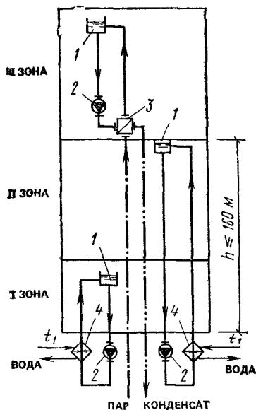
Рис. 6.26. Принципиальная схема водяного отопления высотного здания
