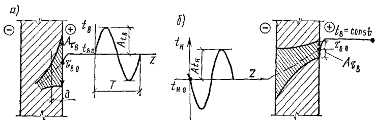
Рис. 2.6 Теплоустойчивость ограждения и ее два проявления — относительно колебаний температуры и теплового потока в помещении (а) и относительно сквозного проникновения через ограждение в помещение колебаний температуры наружного воздуха (б)
