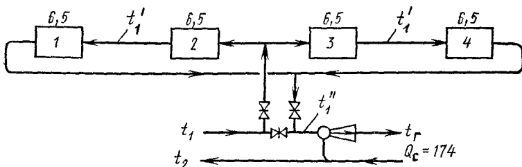
Рис. 10.12. Схема теплопроводов рециркуляционных воздухонагревателей для отопления лестничных клеток жилого здания с элеваторной системой водяного отопления (к примеру 10.9)
