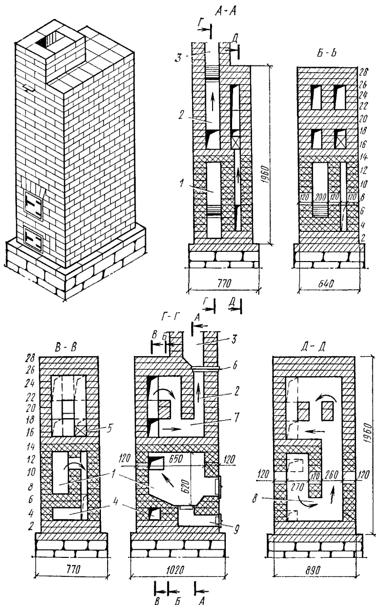
Рис. 12.5. Толстостенная отопительная печь умеренного прогресса марки ПТО-3300 с нижним прогревом
