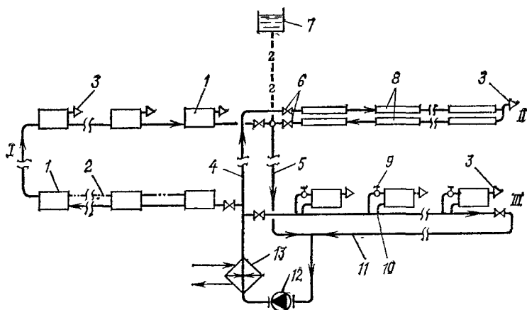
Рис. 6.6. Схема горизонтальной однотрубной системы отопления с ветвями различной (условно) конструкции
