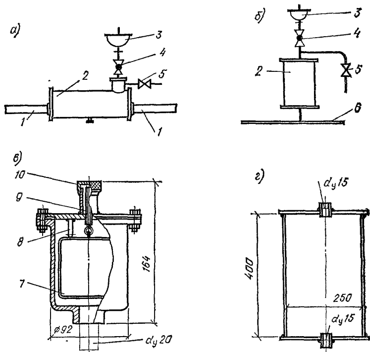
Рис. 5.18. Схемы установки воздухоборников и воздухоотводчиков
