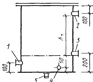
Рис. 6.20. Открытый расширительный бак с патрубками для присоединения труб
