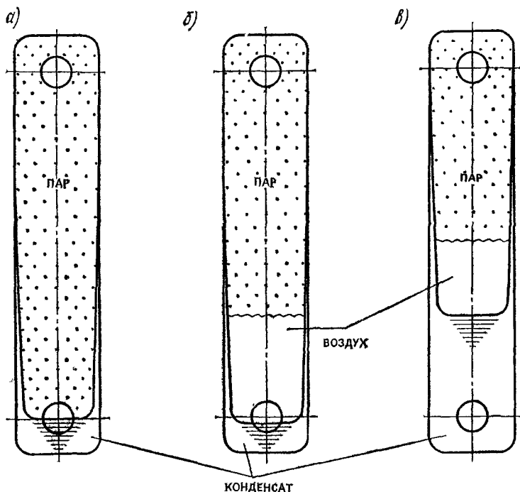
Рис. 9.1. Распределение пара, конденсата и воздуха в отопительном приборе при подаче пара в расчетном количестве (а) и в уменьшенном (б, е)
