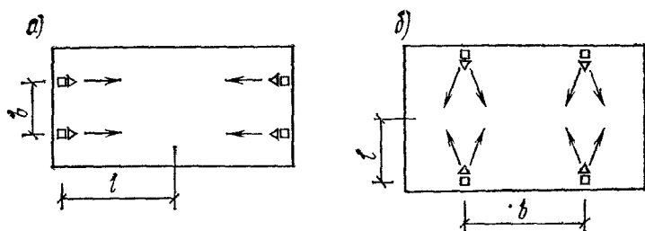
Рис. 10.6. Схемы расположения отопительных агрегатов в плане помещения при параллельных воздушных струях (а) и при неполных весовых воздушных струях (б)
