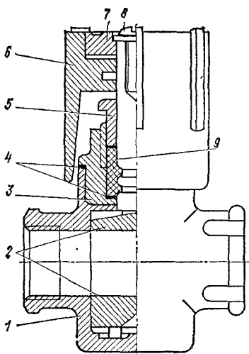
Рис. 5.14. Кран регулирующий трехходовой типа КРТП
