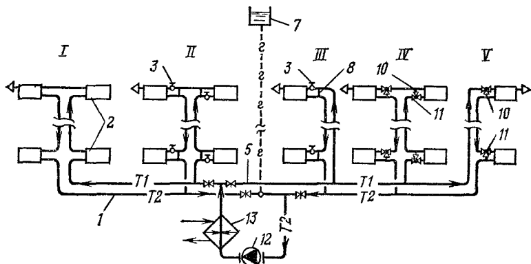
Рис. 6.3. Схема вертикальной однотрубной системы водяного отопления с нижней разводкой и П-образными стояками различной (условно) конструкции
