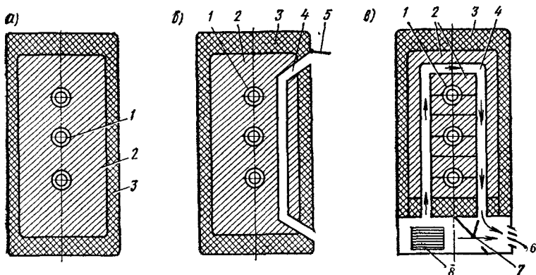
Рис. 14.8. Электрические теплоаккумуляционные печи различных типов
