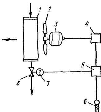
Рис. 10.7. Принципиальная схема автоматизации работы воздушного отопительного агрегата
