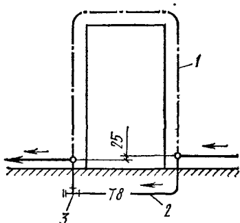
Рис. 9.4. Обвод сухим конденсатопроводом дверного проема
