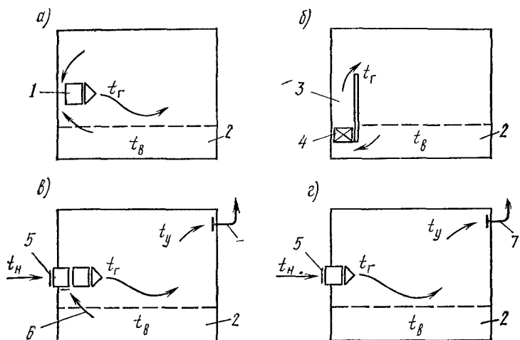
Рис. 10.1. Принципиальные схемы местной системы воздушного отопления а, б — полностью рециркуляционные; в — частично рециркуляционная; г — проточная; 1 — отопительный агрегат; 2 — рабочая зона; 3 — канал нагретого воздуха; 4 — теплообменник-калорифер; 5 — воздухозабор; 6 — рециркулирующий воздух; 7 — канал вытяжной вентиляции
