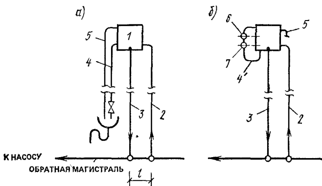
Рис. 6.21. Присоединение открытого расширительного бака к обратной магистрали в системе отопления с ручным контролем (а) и с автоматизированным сигнализацией и регулированием уровня воды в баке (б)
