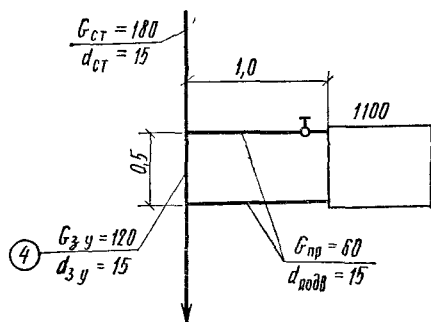
Рис. 8.7. Схема малого циркуляционного кольца в стояке с замыкающими участками вертикальной однотрубной системы водяного отопления с верхней разводкой (к примеру 8.5); 1100 — тепловая нагрузка, Вт
