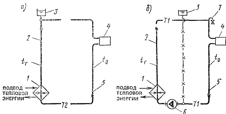
Рис. 1.5. Принципиальные схемы водяного отопления с естественной циркуляцией (гравитационная) (а) и с механическим побуждением циркуляции воды (насосная) (б)
