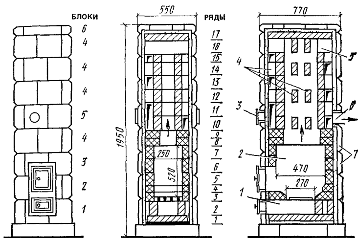
Рис. 12.7. Тонкостенная сборно-блочная отопительная печь повышенного прогрева марки ПТИ-3500
