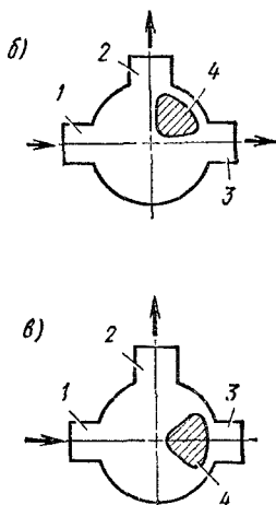
Рис. 5.15. Регулирование расхода воды в отопительном приборе трехходовым краном
