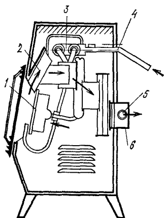
Рис. 13.5. Газовый отопительный камин «Амра» радиационного действия
