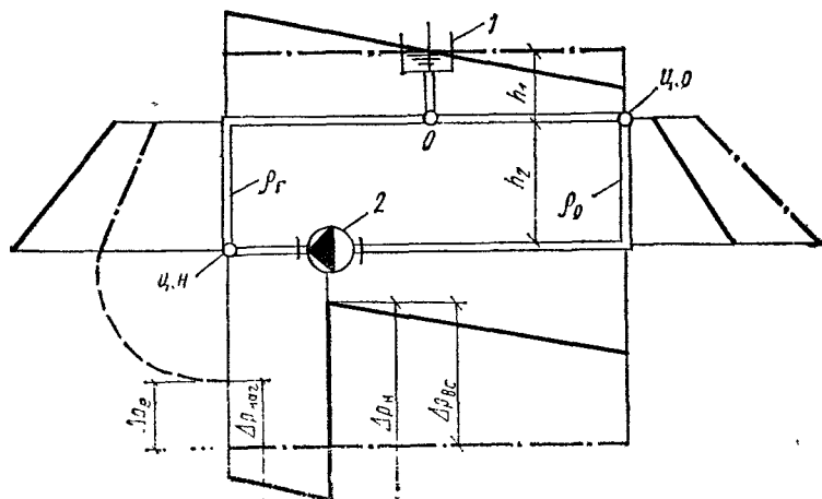
Рис. 7.6. Эпюра гидростатического давления в системе водяного отопления при действии насоса
