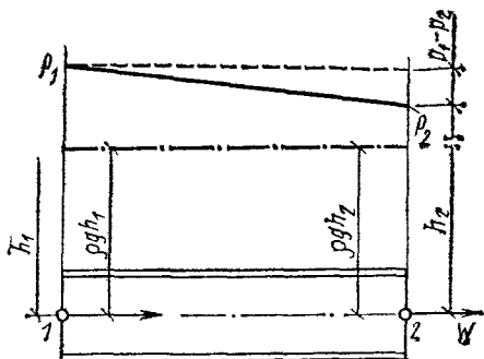
Рис. 7.1. Изменение гидростатического давления в горизонтальной трубе при движении заполняющей ее воды с постоянной скоростью слева направо (давление отложено над трубой)
