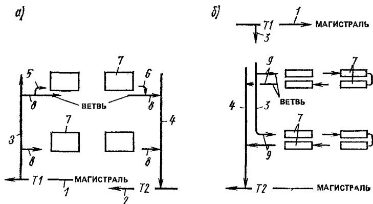
Рис. 5.2. Теплопроводы горизонтальных систем водяного отопления с нижней (а) и верхней разводкой (б)
