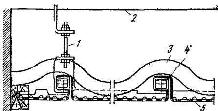
Рис. 11.6. Подвесная потолочная отопительная панель 1 — подвеска, 2 — перекрытие, 3 — тепловая изоляция, 4 — труба для теплоносителя, 5 — перфорированный металлический лист
