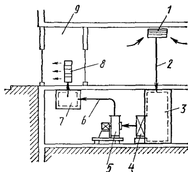
Рис. 10.14. Смесительная воздушно-тепловая завеса у наружного входа здания с двойными тамбуром
