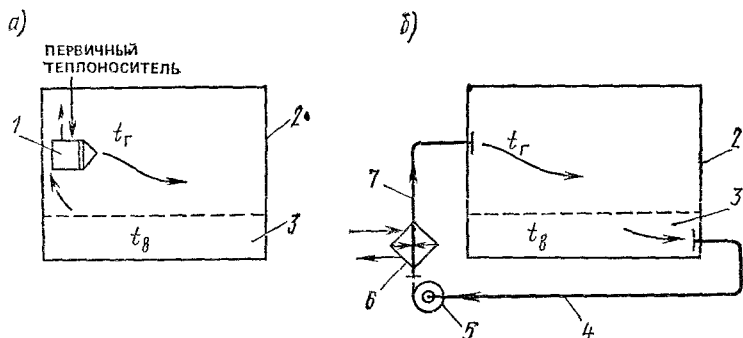
Рис. 1.7. Принципиальные схемы местной (а) и центральной (б) систем воздушного отопления
