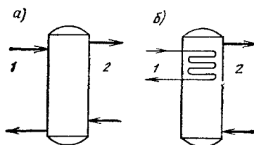
Рис. 20.1. Зависимое включение теплоаккумулятора в контур системы отопления с зависимым подключением греющего контура (а) и с независимым (б) 1 — греющий контур; 2 — контур системы отопления
