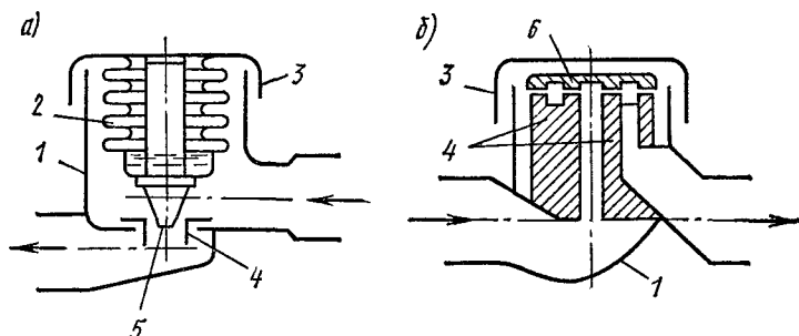
Рис. 9.7. Схемы термостатического (а) и термодинамического (б) конденсатоотводчиков
