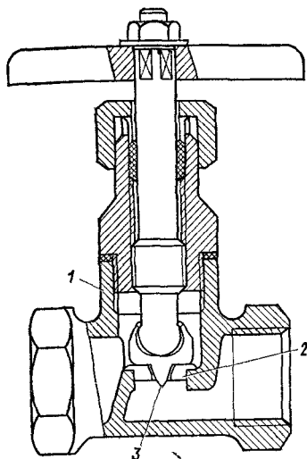
Рис. 5.13. Кран регулирующий с дросселирующим устройством
