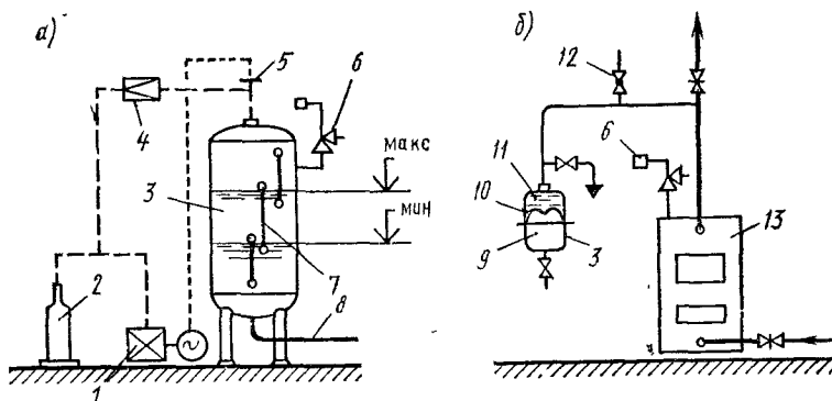
Рис. 6.22. Установка закрытого расширительного бака без мембраны (а) и с мембраной (б)
