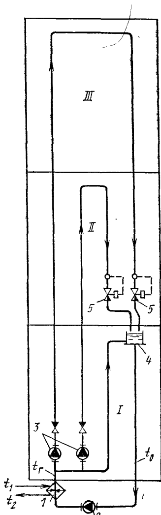
Рис. 6.27. Принципиальная схема единой системы водо-водяного отопления высотного здания
