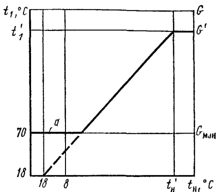
Рис. 17.3. Схема графика регулирования температуры t и расхода G теплоносителя в системе водяного теплоснабжения в течение отопительного сезона
