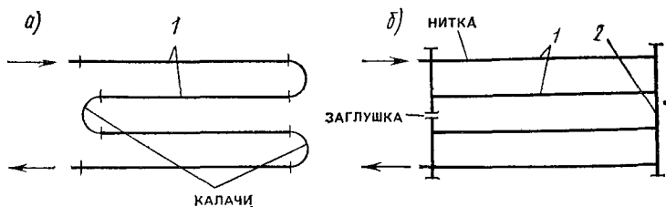
Рис. 4.5. Змеевиковая (а) и регистровая (б) формы соединения стальных труб в гладкотрубные отопительные приборы
