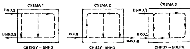
Рис. 4.17. Основные схемы присоединения радиаторов к теплопроводам систем водяного отопления
