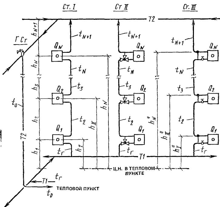
Рис. 7.22. Расчетная схема вертикальной однотрубной системы водяного отопления с «опрокинутой» циркуляцией воды в стояках (с нижней разводкой подающей магистрали и верхней прокладкой обратной магистрали)
