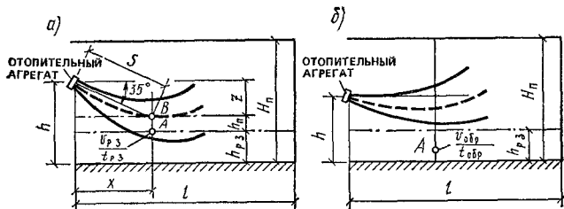
Рис. 10.5. Схемы наклонной (а) и сосредоточенной (б) подачи нагретого воздуха отопительным агрегатом, установленным на высоте h
