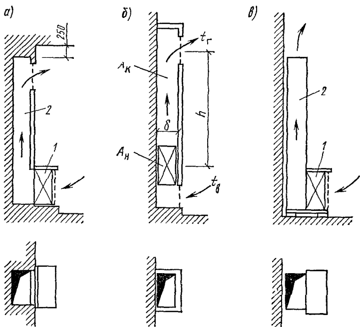
Рис. 10.10. Конструкции рециркуляционных воздушонагревателей
