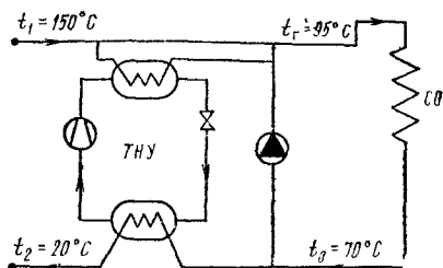
Рис. 19.4. Схема централизованного охлаждения воды системы отопления в обратном теплопроводе центрального теплоснабжения с помощью теплового насоса
