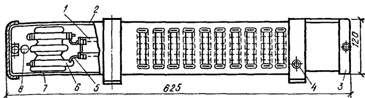
Рис. 14.3. Печь электронагревательная ПЭТ (боковой вид)
