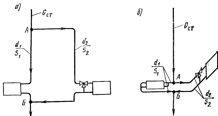
Рис. 8.4. Схемы нетиповых однетрубных узлов
