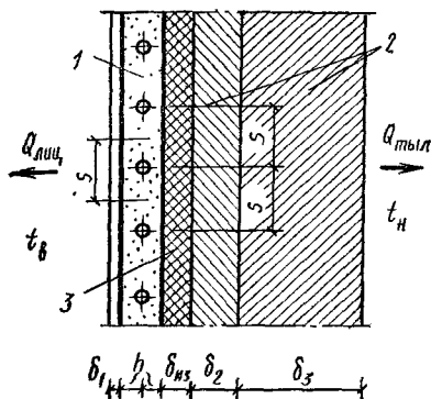
Рис. 11.14. Разрез наружного ограждения с приставной бетонной отопительной панелью
