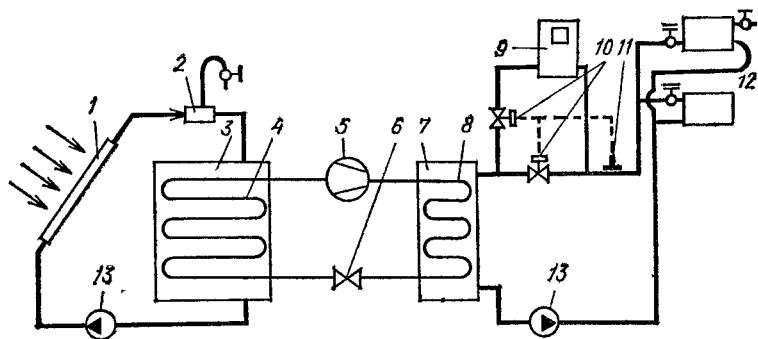
Рис. 20.10. Жидкостная двухконтурная комбинированная низкотемпературная система солнечного отопления с плоскими коллекторами, тепловым насосом и двумя жидкостными теплоаккумуляторами
