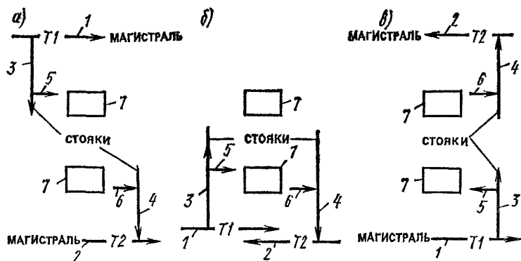
Рис. 5.1. Теплопроводы вертикальных систем центрального отопления с верхней разводкой (а), с нижней разводкой (б), с «опрокинутой» циркуляцией воды (в) 1 и 2 — подающие (T1) и обратные (T2) магистрали; 3 и 4 — подающие и обратные стояки; 5 и 6 — подающие и обратные подводки; 7 — отопительные приборы (стрелками показано направление движения теплоносителя)
