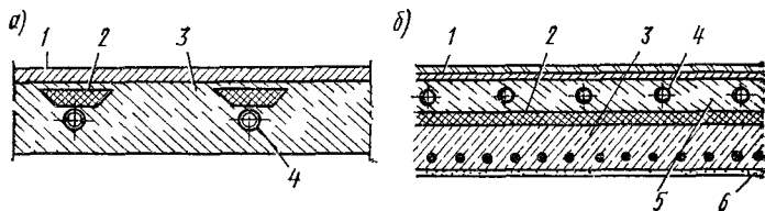
Рис. 11.7. Напольные бетонные отопительные панели с расположением греющих труб в несущей части перекрытия (а) и над ней (б)
