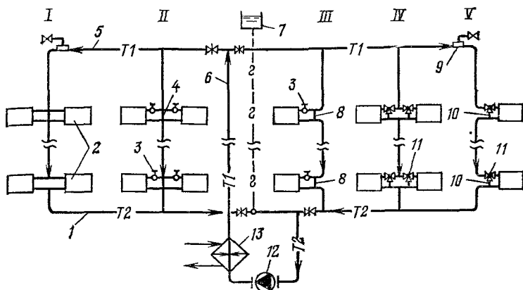
Рис. 6.2. Схема вертикальной однотрубной системы водяного отопления с верхней разводкой и стояками различной (условно) конструкции
