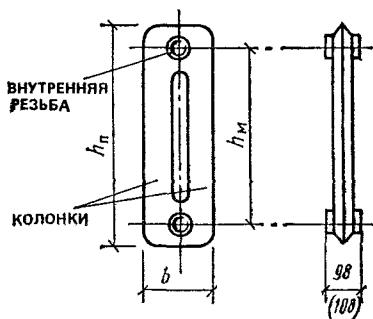
Рис. 4.3. Двухколончатая секция чугунного радиатора h_n — полная высота; h_m — монтажная высота; b — строительная глубина, 98 (108) — длина секции, мм
