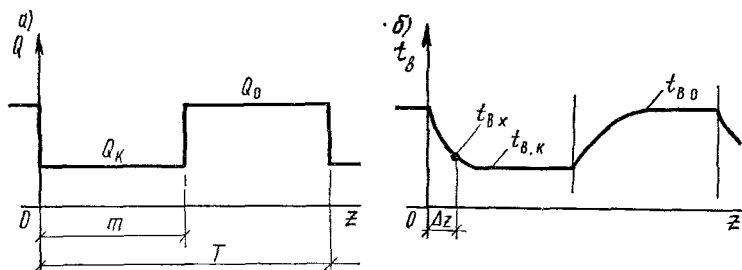
Рис. 2.8. Охлаждение помещения в интерпретации теории теплоустойчивости как часть периодического процесса длительного охлаждения и нагревания а — периодические длительные прекращения и подача теплоты, б — соответствующее изменение температуры воздуха в помещении
