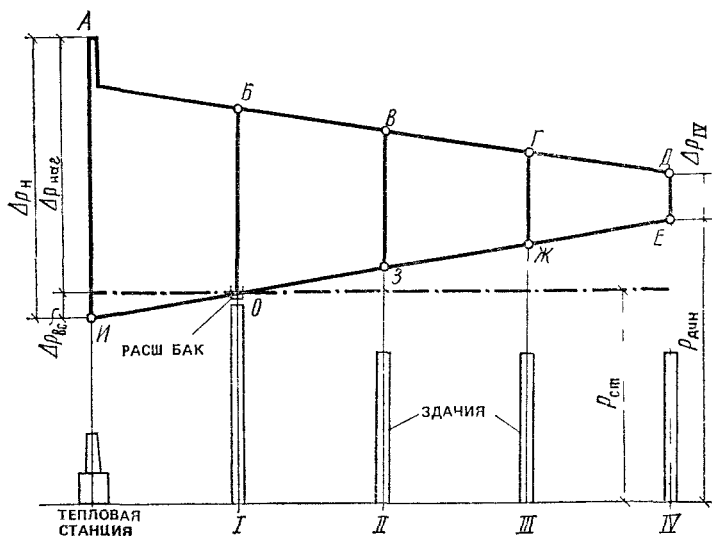
Рис. 7.12. Изменение гидростатического давления в наружных тепловых трубах районной системы отопления четырех зданий с расширительным баком в ближайшем здании (I) к тепловой станции
