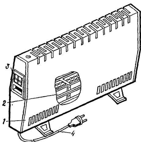
Рис. 14.7. Электроконвектор 1 — корпус прибора; 2 — нагревательный элемент из стальных пластин; 3 — выключатель; 4 — шнур
