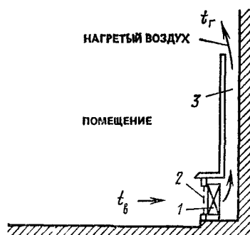
Рис. 4.11. Схема рециркуляционного воздухонагревателя
