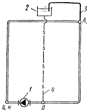
Рис. 7.15. Схема системы водяного отопления с верхней разводкой и воздушной трубой, выведенной в открытый расширительный бак
