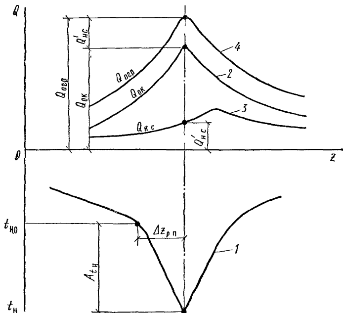
Рис. 3.1. Определение наибольших теплотерь помещения в период резкого похолодания
