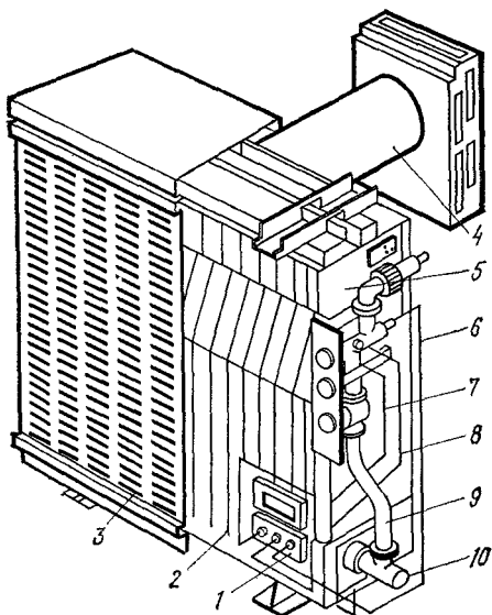
Рис. 13.6. Газовый отопительный камин АОГ-5 конвективного действия
