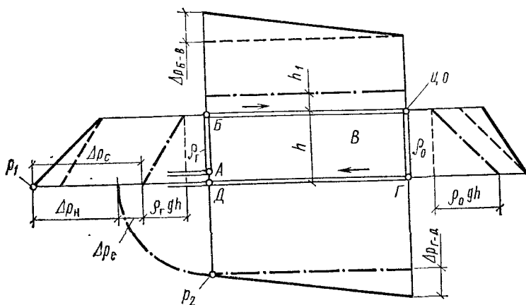
Рис. 7.13. Эпюра гидростатического давления в системе водяного отопления, непосредственно соединенной с наружными теплопроводами (без расширительного бака) D — точка постоянного давления P_2
