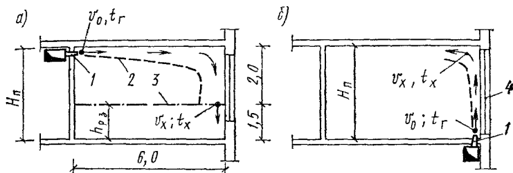
Рис. 10.13. Центральное воздушное отопление помещения с подачей нагретого воздуха через подпотолочный (а) и напольный (б) щелевой воздухораспределитель 1 — воздухораспределитель; 2 — граница настилающейся воздушной струи; 3 — граница рабочей зоны; 4 — наружное ограждение
