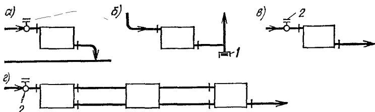
Рис. 5.9. Разностороннее присоединение труб к отопительным приборам при движении теплоносителя в приборах сверху вниз
