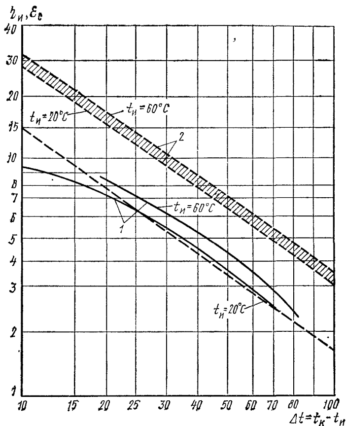
Рис. 19.1. Зависимость коэффициента использования (1) реальных теплонасосных установок и коэффициента преобразования (2) идеального термодинамического цикла \epsilon_c от разности температуры \Delta t в конденсаторе t_k и испарителе t_n
