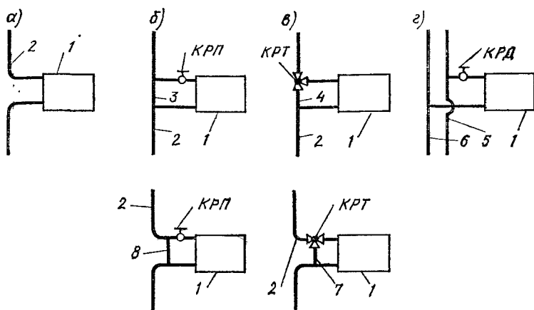
Рис. 5.7. Одностороннее присоединение труб к отопительным приборам вертикальных систем отопления однотрубных (а—г), двухтрубных (з)
