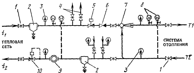
Рис. 6.10. Принципиальная схема местного теплового пункта при зависимом присоединении системы водяного отопления к наружным теплопроводам со смещением воды с помощью водоструйного элеватора
