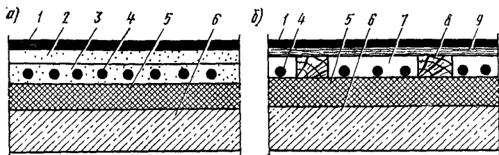
Рис. 14.1. Греющий кабель в перекрытиях зданий
