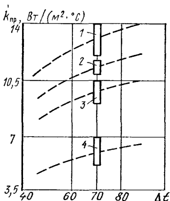
Рис. 4.16. Области значений коэффициента теплопередачи отопительных приборов при \Delta t_{\text{ср}} = 70^\circ\text{C}
