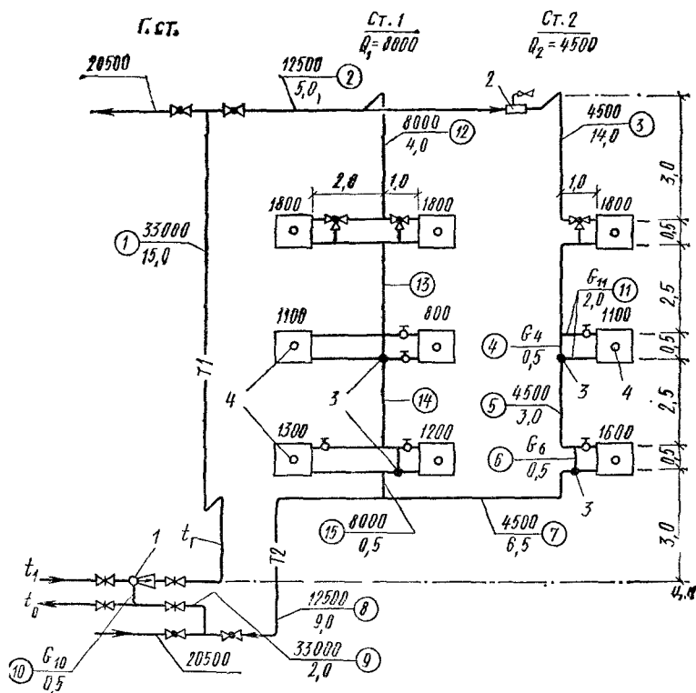
Рис. 8.6. Схема вертикальной однотрубной системы водяного отопления с верхней разводкой и тупиковым движением воды в магистралях (к примеру 8.3)
