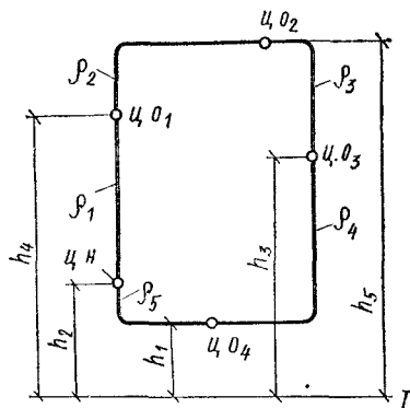
Рис. 7.19. Схема вертикального циркуляционного кольца теплопроводов с произвольно расположенными центрами нагревания (ц. н.) и охлаждения (ц. о.) теплоносителя воды
