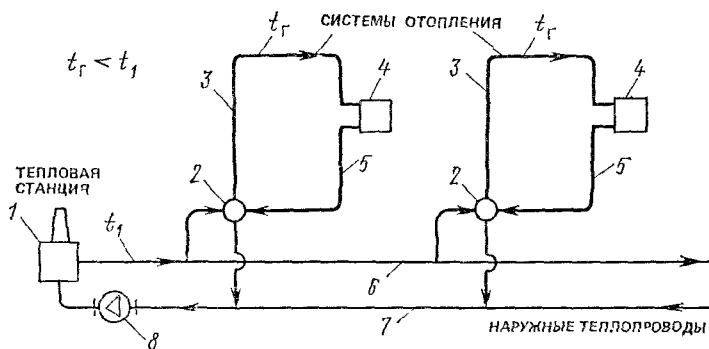
Рис. 1.4 Принципиальная схема районной системы отопления
