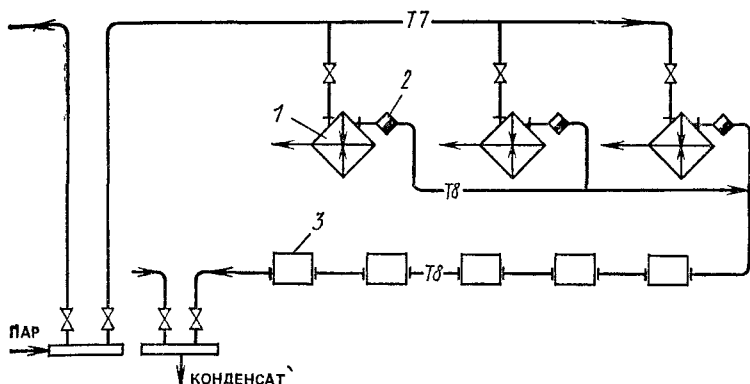
Рис. 9.13. Схема системы парового отопления высокого давления с использованием пароконденсатной смеси в местных отопительных приборах
