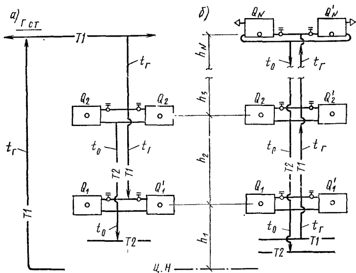
Рис. 7.23. Расчетные схемы вертикальной двухтрубной системы водяного отопления с верхней разводкой (а) и нижней разводкой магистралей (б)
