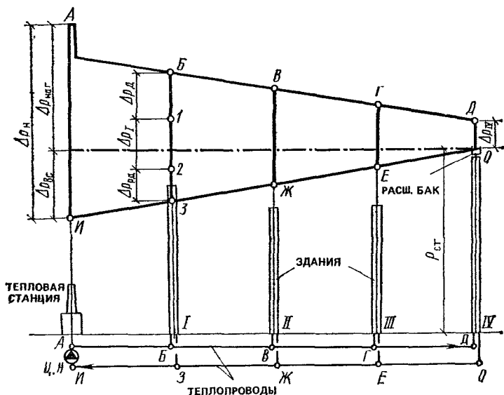
Рис. 7.11. Изменение гидростатического давления в наружных теплопроводах районной системы отопления четырех зданий с расширительным баком в удаленном здании (IV) от тепловой станции
