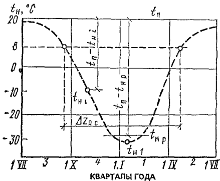
Рис. 1.2. Схема изменения среднесуточной температуры наружного воздуха в течение года в Москве
