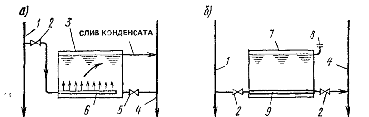
Рис. 9.14. Радиаторы децентрализованной пароводяной системы отопления а — стандартный чугунный; б — безнапорный стальной; 1 — паровой стояк; 2 — паровой вентиль; 3 — чугунный радиатор; 4 — конденсатный стояк; 5 — вентиль (нормально закрыт); 6 — перфорированная труба; 7 — стальной радиатор; 8 — водоналивной патрубок; 9 — водонагревательная труба
