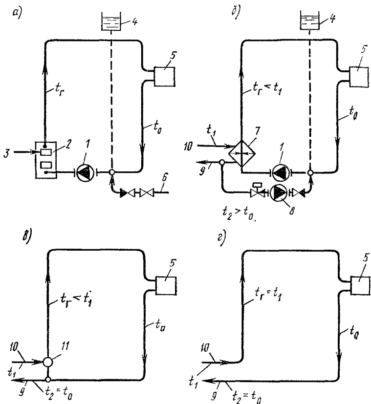
Рис. 6.1. Принципиальные схемы системы насосного водяного отопления при местном теплоснабжении (а) и присоединении к наружным теплопроводам централизованного теплоснабжения (б, в, г)
