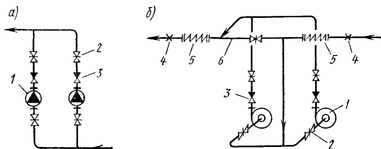
Рис. 6.15. Схемы присоединения труб к циркуляционным бесфундаментным (а) и общепромышленным (б) насосам
