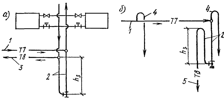
Рис. 9.3. Схема системы осушки пара при нижней разводке паропроводов (а) и верхней (б)
