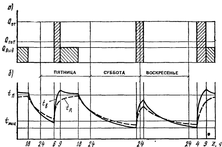
Рис. 19.6. Изменение теплоступлений Q(a) , температуры (б) воздуха t_v (сплошные линии) и радиационной температуры t_R (пунктирные линии) рабочего помещения в течение четырех дней недели в зимнее время
