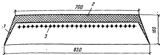
Рис. 14.2. Подвесная панель с электрообогревом изолированным кабелем 1 — стальной кожух; 2 — теплоизоляция из пенопласта; 3 — нагреватель
