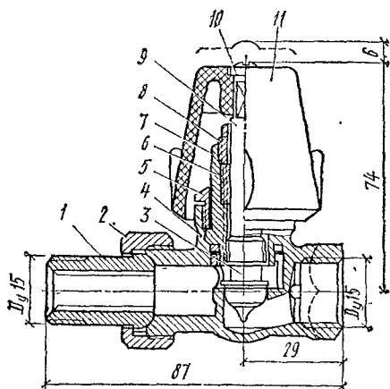
Рис. 5.12. Кран двойной регулировки типа «Термис»
