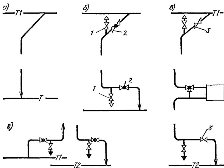
Рис. 5.4. Схемы присоединения стояков к магистралям систем водяного отопления двух-трехэтажных (а), четырех-семизэтажных при верхней разводке (б) и нижней разводке (г), восьмиэтажных и более высоких (в) зданий.
