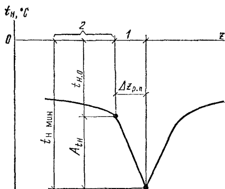
Рис. 2.1. Характерная расчетная кривая изменения температуры наружного воздуха в период резкого похолодания 1 — период резкого похолодания; 2 — период устойчивой зимней температуры
