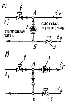
Рис. 6.16. Принципиальные схемы смесительной установки с насосом на перемычке между магистралями (а), на обратной магистрали (б), на подающей магистрали (в)
