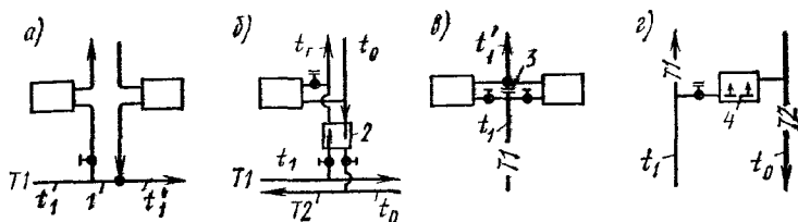
Рис. 6.28. Узлы систем отопления с децентрализованным смешением воды в основании однотрубных и двухтрубных стояков (а и б), в приборах одно- и двухтрубных стояков (в и г)
