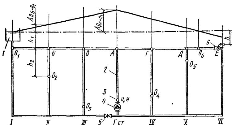
Рис. 7.10. Изменение гидростатического давления в верхней подающей магистрали системы водяного отопления, состоящей из двух частей, при действии насоса 1 — открытый расширительный бак; 2 — главный подающий стояк; 3 — центр нагрева; 4 — циркуляционный насос 5 — задвижка, 6 — проточный воздухоотборник с воздушным краном
