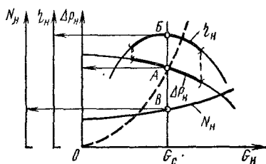
Рис. 6.13. Характеристики циркуляционного насоса (КПД, давление, мощность) и характеристика системы отопления (пунктирная линия)
