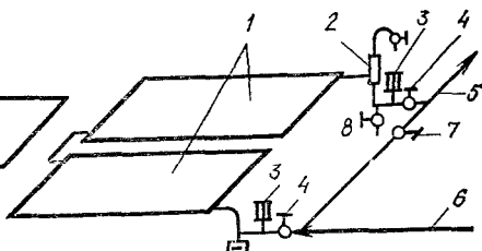
Рис. 11.12. Схема присоединение напольных панелей к обратной магистрали системы водяного отопления
