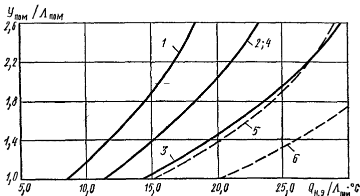
Рис. 14.12. График для подбора теплоаккумулирующих отопительных приборов 1, 4 — \gamma_{э} = 7,9 ; 2, 5 — \gamma_{э} = 10 ; 3, 6 — \gamma_{э} = 12,8 ; 1, 2, 3 — зарядка 8 ч; 4, 5, 6 — зарядка 8 + 2 ч
