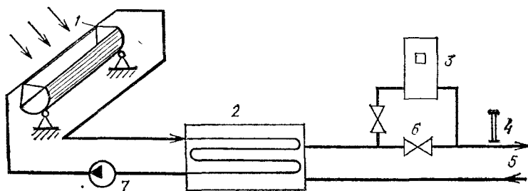
Рис. 20.7. Жидкостная комбинированная двухконтурная низкотемпературная система отопления с параболическим концентратором и жидкостным теплоаккумулятором
