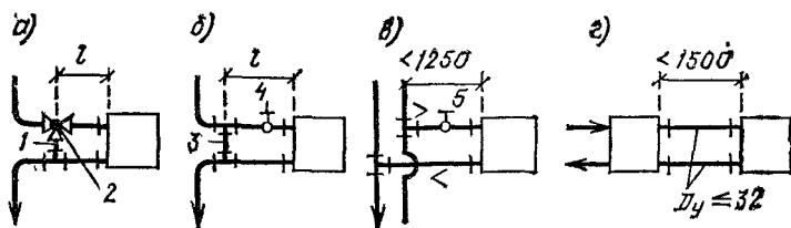
Рис. 5.8. Унифицированное присоединение труб к отопительным приборам вертикальных систем отопления однотрубных (а и б), двухтрубных (в) и в «сцепке» двух приборов (г)
