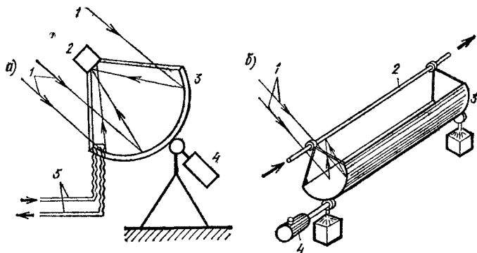
Рис. 20.6. Концентрирующие гелиоприемники
