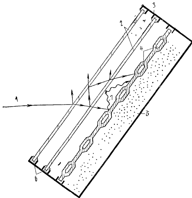
Рис. 20.8. Плоский солнечный коллектор
