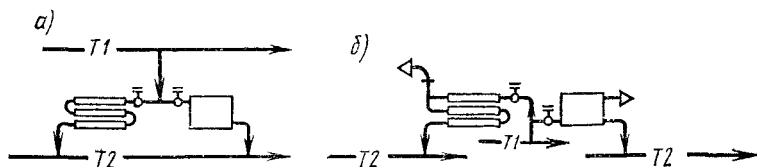
Рис. 6.7. Приборные узлы горизонтальной двухтрубной системы водяного отопления с верхней (а) и нижней (б) разводкой магистралей
