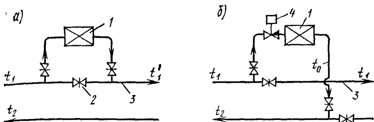
Рис. 10.11. Последовательная (а) и параллельная (б) схемы присоединения воздухонагревателя к теплопроводам
