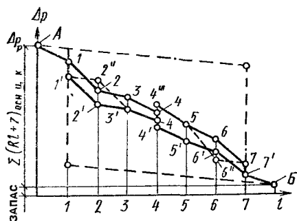
Рис. 8.3. Эюра циркуляционного давления в двухтрубной системе отопления с попутным движением воды в магистралях (1—7 — номера стояков)
