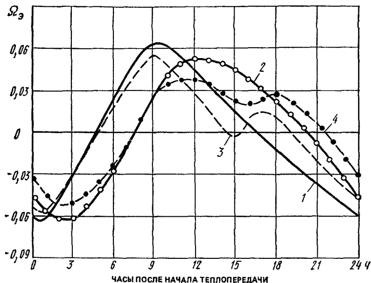
Рис. 14.11. Расчетные значения показателя \Omega_{э} при периоде зарядки аккумулирующей печи, равном 8 ч (кривые 1, 2) и 8 + 2 ч (3, 4); для приборов с \gamma_{э} = 7,9 (1, 3) и 10 (2, 4)
