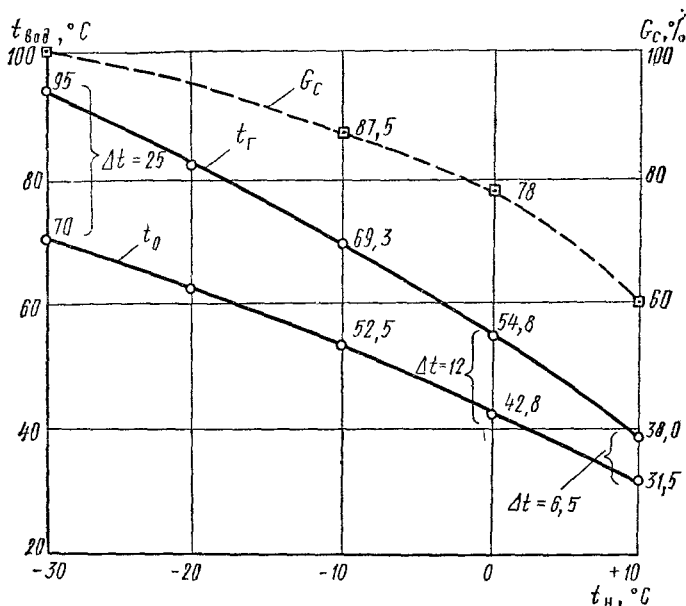
Рис. 7.25. График изменения температуры t_r , t_o и расхода воды G_c в вертикальной однетрубной системе отопления в течение отопительного сезона (расчетные t_r = 95^\circ\text{C} и t_o = 70^\circ\text{C} соответствуют t_n = -30^\circ\text{C} )
