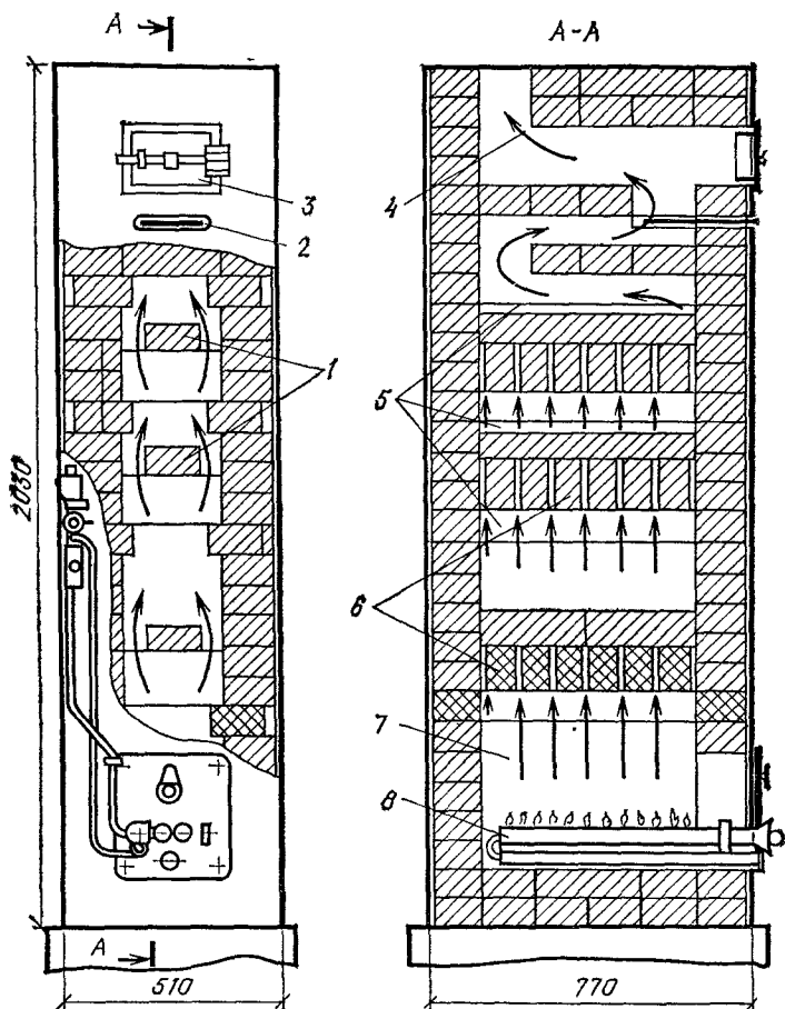
Рис. 13.1. Газовая отопительная печь АКХ-14
