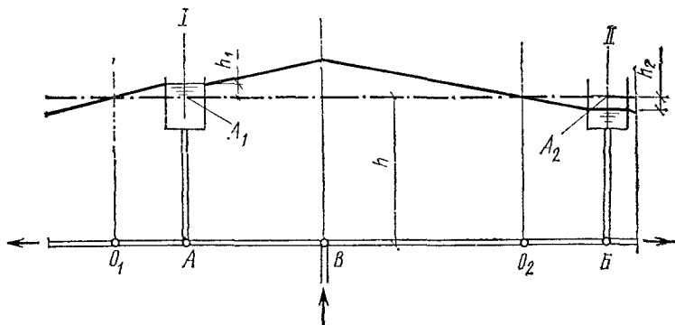
Рис. 7.16. Эпюра гидростатического давления в системе водяного отопления с двумя открытыми расширительными баками, параллельно присоединенными к теплопроводам
