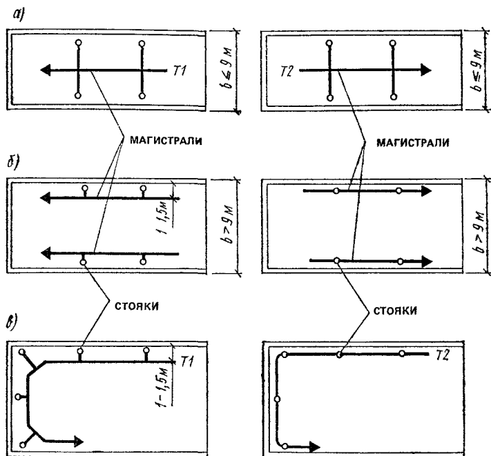
Рис. 5.5. Размещение магистралей систем отопления в чердачных (слева), подвальных и технических (справа) помещениях зданий шириной 9 м (а), шириной более 9 м при тупиковом (б) и попутном (в) движении теплоносителя в трубах
