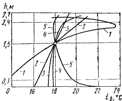
Рис. 3.7. Кривые распределения температуры воздуха по высоте помещения при различных видах отопления (за реперную точку принята температура 18 °С на высоте 1,5 м от пола для всех видов отопления)
