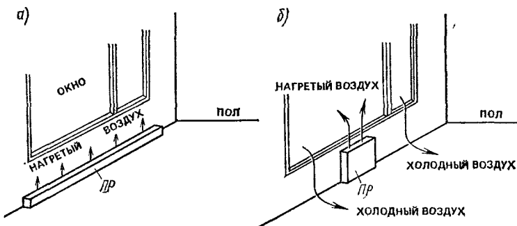
Рис. 4.10. Размещение под окном помещения отопительного прибора (пр) низкого и длинного (желательно) (а), высокого и короткого (нежелательно) (б)
