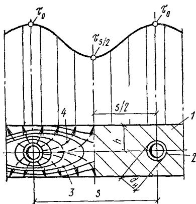
Рис. 11.13. Схема изотерм и тепловых потоков в массиве бетона и график изменения температуры поверхности отопительной панели с двухсторонней теплоотдачей
