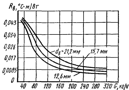
Рис. 4.13. Зависимость сопротивления теплообмену на внутренней поверхности стенки R_B от расхода теплоносителя G и внутреннего диаметра трубы d_B
