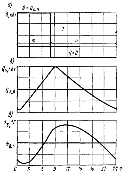
Рис. 14.10. Изменение теплового потока от нагревательных элементов (а), теплопоступлений от наружной поверхности теплоаккумулирующего прибора (б), температуры воздуха при 8-часовой зарядке (в)
