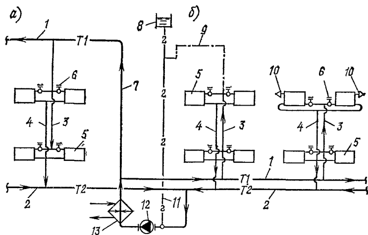
Рис. 6.5. Схемы вертикальной двухтрубной системы водяного отопления с верхней (а) и нижней (б) разводкой (при нижней разводке стояки условно различной конструкции)
