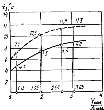
Рис. 19.7. Зависимость минимальной температуры воздуха после ночного охлаждения (без отопления) от теплоустойчивости помещений, имеющих окна с двойным (сплошная линия) и тройным (пунктирная линия) остеклением, при t_n = -20^\circ\text{C} .
