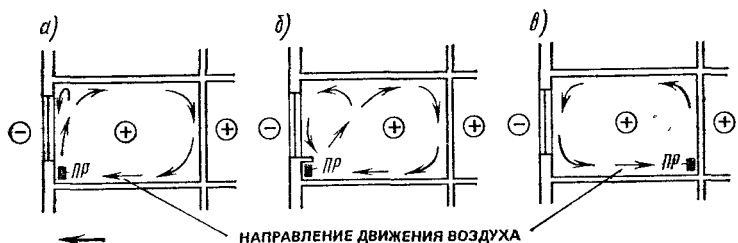
Рис. 4.9. Схемы циркуляции воздуха в помещениях (разрезы) при размещении отопительных приборов (пр) под окнами без подоконника (а), под окнами с подоконником (б), у внутренней стены (в)
