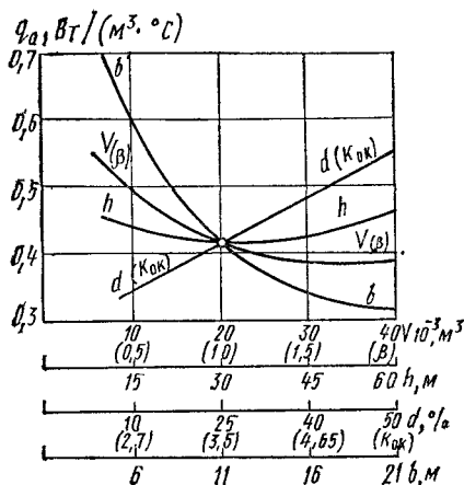
Рис. 3.6. Зависимость удельной тепловой характеристики здания q_0 от объема здания V(\beta) , степени остекленности наружных стен d(k_{ок}) , ширины здания b и высоты h [реперная точка на графике с q_0=0,415 Вт/(м³·°C) соответствует зданию объемом V=20 \cdot 10^3 м³ ( \beta=0 ), шириной b=11 м, остекленностью наружных стен d=0,25 при сопротивлении теплопередаче наружных стен R_0=0,86 ( \beta=0 ), коэффициент теплопередачи окон k_{ок}=3,48 ]
