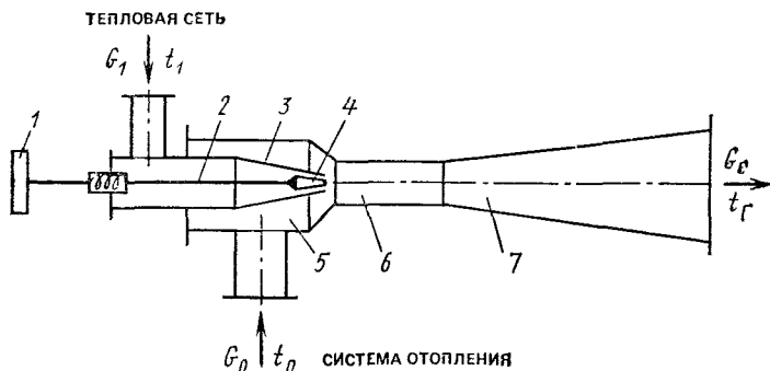
Рис. 6.19. Схема водоструйного элеватора с регулируемым соплом
