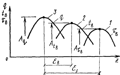
Рис. 2.6 Теплоустойчивость ограждения и ее два проявления — относительно колебаний температуры и теплового потока в помещении (а) и относительно сквозного проникновения через ограждение в помещение колебаний температуры наружного воздуха (б)
