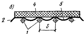
Рис. 11.3. Подвешенная металлическая отопительная панель с плоским экраном (а) и с экраном волнообразной формы (б)
