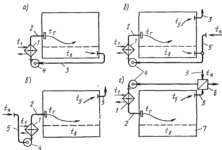
Рис. 10.2. Принципиальные схемы центральной системы воздушного отопления а — полностью рециркуляционная; б — частично рециркуляционная; в — проточная; г — рекуперативная; 1 — теплообменник-калорифер; 2 — канал нагретого воздуха с воздухораспределителем на конце; 3 — канал внутреннего воздуха; 4 — вентилятор; 5 — канал наружного воздуха; 6 — воздухо-воздушный теплообменник; 7 — рабочая зона
