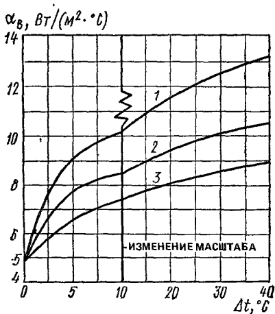
Рис. 2.3. Зависимость коэффициента теплообмена \alpha_v для плоской нагретой поверхности, расположенной в помещении, от разности температуры на поверхности и помещения \Delta t
