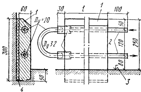
Рис. 11.9. Плинтусная представная бетонная отопительная панель
