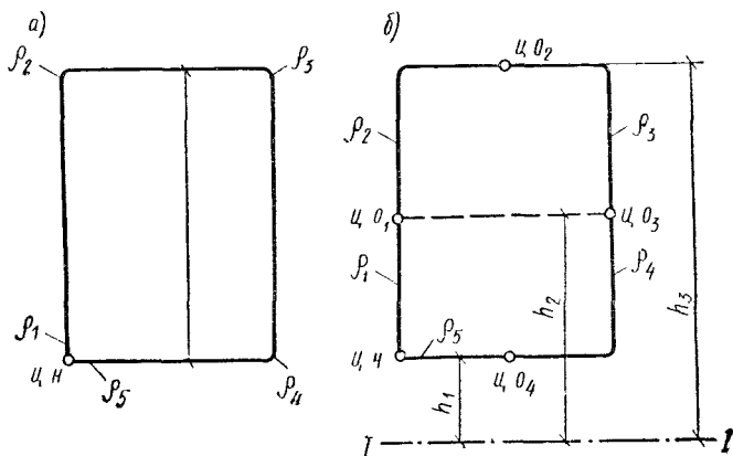
Рис. 7.18. Схемы вертикального циркуляционного кольца теплопроводов без отопительных приборов с центром нагревания (ц. н.)
