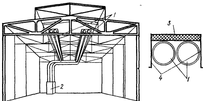
Рис. 13.9. Схема системы воздушного лучистого отопления с теплоизлучающими трубами в межферменном пространстве цеха
