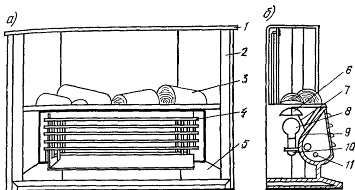
Рис. 14.5. Декоративно-функциональный электрокамин
