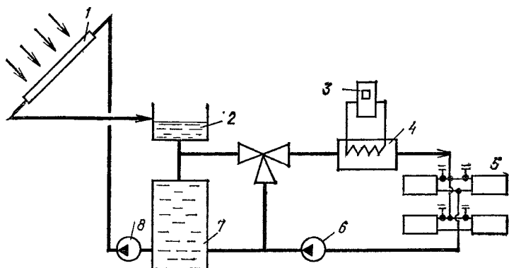
Рис. 20.9. Схема водяной низкотемпературной системы солнечного отопления с плоскими коллекторами и их автоматическим дренажем при прекращении циркуляции
