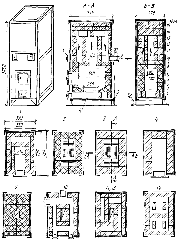
Рис. 12.6. Тонкостенная каркасная отопительная печь повышенного прогрева марки ПТК-3000
