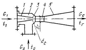
Рис. 6.18. Принципиальная схема водоструйного элеватора
