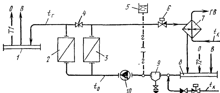
Рис. 6.8. Принципиальная схема тепловых пунктов местной водогрейной котельной 1 — распределительный коллектор, 2 — котел теплоснабжения систем отопления и вентиляции; 3 — котел теплоснабжения системы горячего водоснабжения; 4 — задвижка (нормально закрыта), 5 — расширительный бак; 6 — регулирующий клапан, 7 — теплообменник системы горячего водоснабжения; 8 — сборный коллектор, 9 — грязевик; 10 — циркуляционный насос
