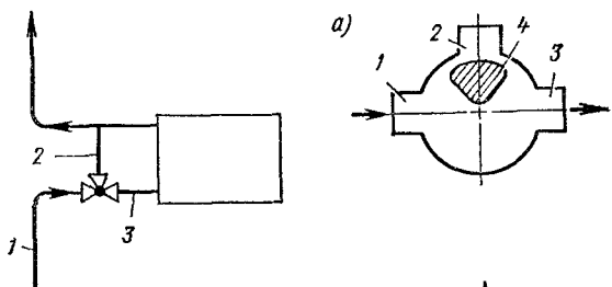
Рис. 5.15. Регулирование расхода воды в отопительном приборе трехходовым краном
