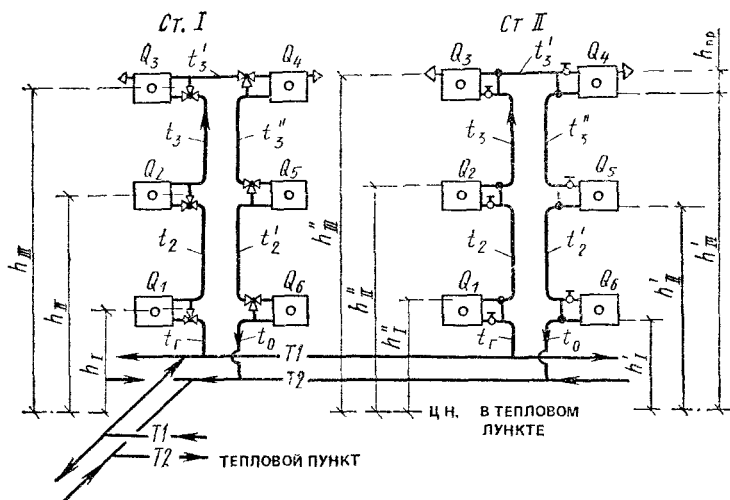
Рис. 7.21. Расчетная схема вертикальной однотрубной системы водяного отопления с нижней разводкой обеих магистралей (с П-образными стояками)
