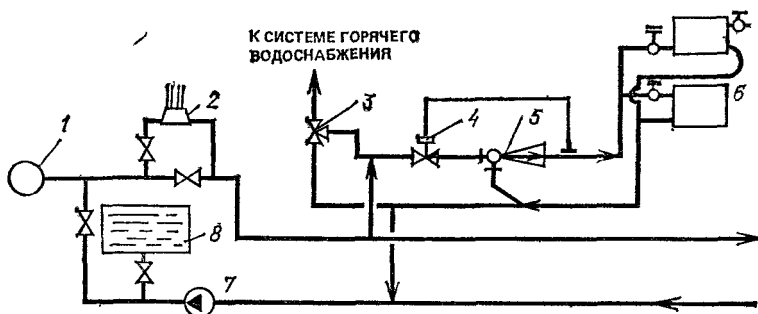
Рис. 20.11. Бессливная комбинированная геотермальная система теплоснабжения с «пиковым» догревом
