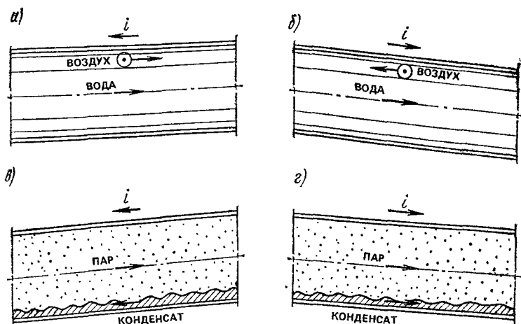
Рис. 5.6. Направление движения теплоносителя и уклон i труб в системах отопления
