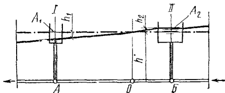
Рис. 7.14. Эпюра гидростатического давления в системе водяного отопления с двумя открытыми расширительными баками, последовательно присоединенными к теплопроводу
