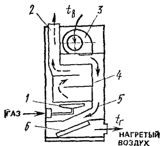
Рис. 1.3. Схема газовоздушного отопительного агрегата
