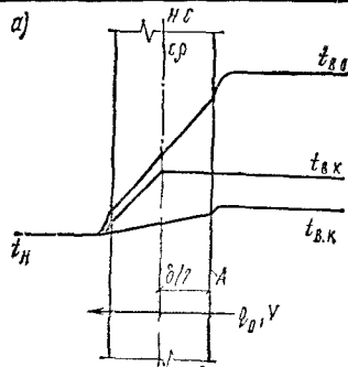
Рис. 2.9. Принятое распределение температур в наружном ограждении (а) и схема теплообмена (б) при выводе формулы (2.86) для расчета охлаждения помещения
