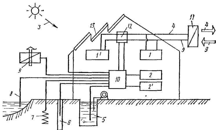
Рис. 19.3. Сопряжение потоков энергии различных сред внутри и вне здания 1, 1' — отапливаемые, кондиционируемые и вентилируемые помещения; 2, 2' — прочие потребители теплоты и холода; 3 — солнечные лучи; 4 — внутренний удаляемый воздух; 5 — бытовые и технологические воды; 6 — грунтовые воды; 7 — геотермальные источники; 8 — водоемы; 9 — наружный воздух; 10 — холодильная машина и тепловой насос; 11 — регенераторы, рекуператоры и другие теплоутилизаторы; 12 — смесители; 13 — солнечные коллекторы и абсорберы
